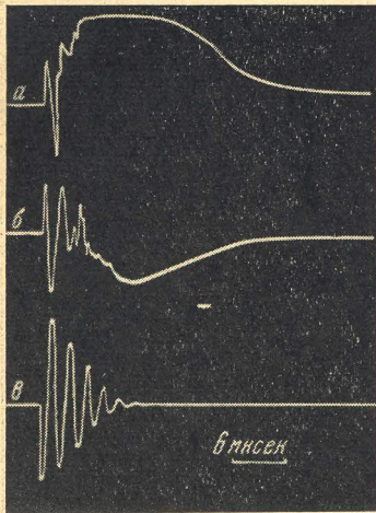
Фиг. 2 Сигналы с магнитных зондов, установленных в плазме под витком на расстояниях: а — \sim 0.25R , б — \sim 0.9R от оси камеры, в — ток ударного витка.
