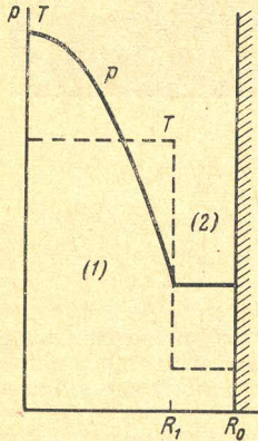
Фиг. 5. Распределение давления и температуры в каналовой модели
