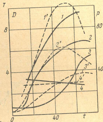
Фиг. 6. Сравнение экспериментальных данных с расчетными. Максимум основного тока соответствует 37 мксек. Сплошные кривые — экспериментальные, пунктирные — расчетные; 1 и 1' — температура, 2 и 2' — давление на оси, 3 и 3' — давление в пристеночной области, 4 и 4' — диаметр токового канала
