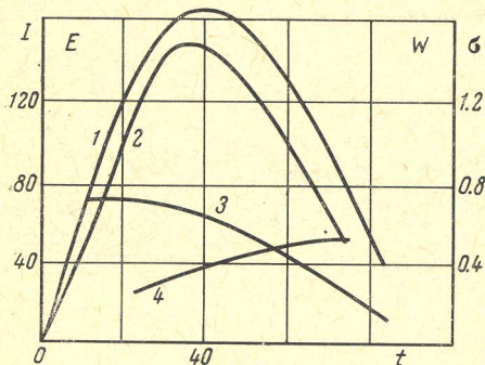
Фиг. 2. Электрические характеристики разряда ( t , мксек); p_0 = 20 \text{ мм рт. ст.} Водород. 1 — ток I , кА; 2 — мощность W , Мвт/см 3 , вкладываемая в плазму; 3 — напряженность электрического поля E , в/см; 4 — проводимость плазмы \sigma , мо/см
