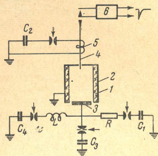
Фиг. 1. Схема установки
