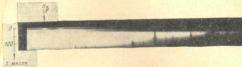
Фиг. 4. Развертка спектра излучения во времени; H_\beta — водородная линия серии Бальмера (4861 Å)
