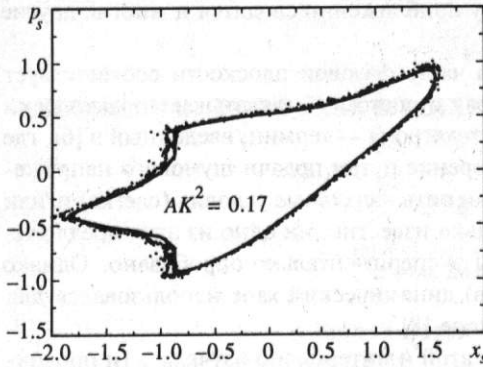
Рис. 1. Универсальная граница микро- тронных областей в безразмерных перемен- ных (4): n = 2-20000 ; время движения для каждого n равно 3000 итераций отображе- ния (1). Область внутри границы соответ- ствует регулярному движению, а вне ее — хаотическому. Вблизи неподвижной точки x_s = p_s = 0 частота малых колебаний \omega_0 = \pi/2 , а на границе \omega_b = 2\pi r_b (6)
