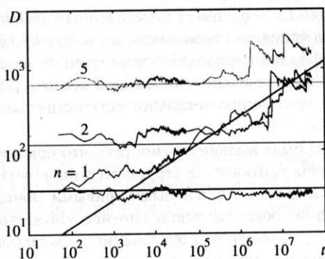
Рис. 3. Аномальная диффузия для модели (1) в микротронном режиме (3): ломаные линии — численные данные для n = 1, 2, 5 и контрольного счета \bar{c} K = 2\pi (см. текст); горизонтальные прямые показывают (постоянную) скорость нормальной диффузии; наклонная прямая — зависимость (19) с теоретическим значением c_D = 1/3 и эмпирическим b = 11 (для n = 1, M = 40 )
