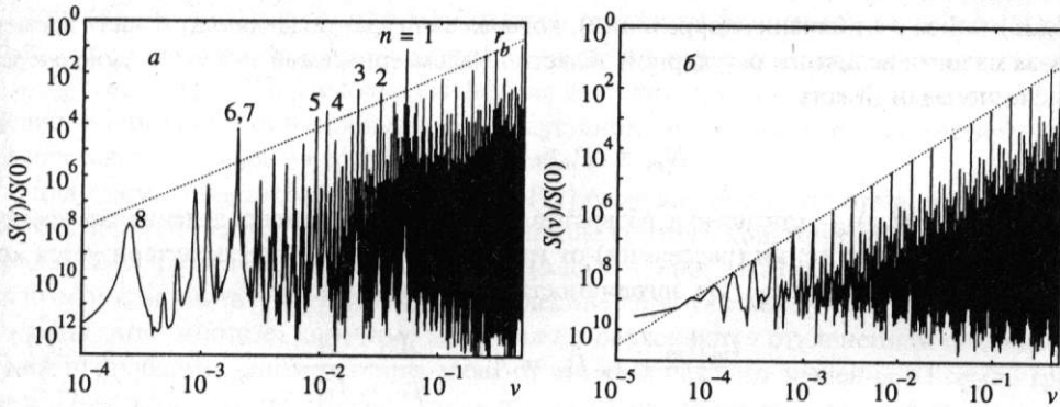
Рис. 2. Пример спектра движения на границе хаоса: частота \nu \pmod{1} , S(\nu)/S(0) — относительный модуль фурье-амплитуды; полное время движения T = 65536 итераций. а — Статистическое подобие (хаотическая ренормгруппа) на грубой границе хаос–порядок: n = 1 ; r_b = 0.23713 \dots (пик r_b ), что несколько отличается от асимптотического значения (6). Цифры у кривой — порядковый номер m основных резонансов, а пунктирная прямая — теория (8). б — Точное подобие (неподвижная точка ренормгруппы) на негрубой границе хаос–хаос для специального r_b = (3 - \sqrt{5})/2 = [2, 1, 1, 1, \dots] и K = 0.9716 \dots
