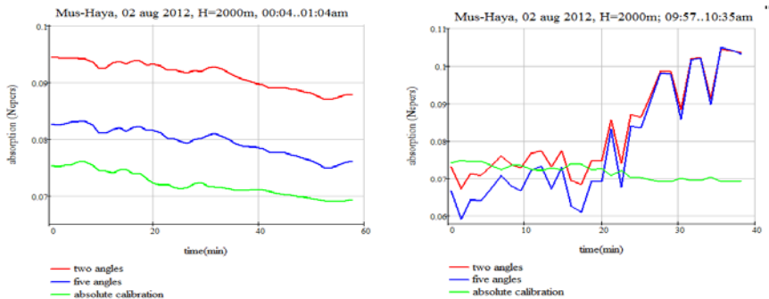
Измерение атмосферного поглощения
