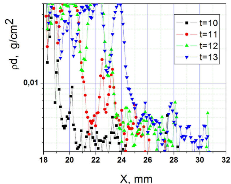
Динамика распределений массы струи от времени. Прямой стык. 10-13 мкс.
