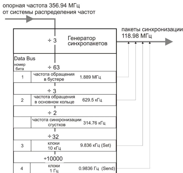
Рисунок 3.6.3.3. Схема генерации тактовых частот в блоке RMO.
