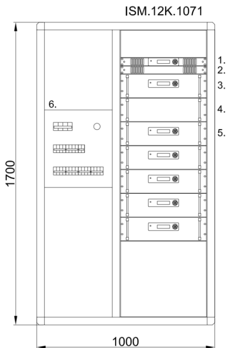
Рисунок 3.4.2.1. Эскиз усилителя мощности ISM.12K.1071 для ВЧ питания резонатора третьей гармоники накопительного кольца (вид спереди). На рисунке цифрами обозначены: 1 – Блок управления, 2 – Блок дистанционного контроля СДК-5, 3 – Предварительный усилитель 500 Вт, 4 – Делитель на 4, 5 – Усилитель мощности 3.6 кВт, 6 – Распределительный щит.
