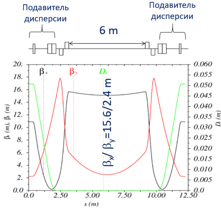
Рисунок 2.1.3.1. Магнитная структура секций подавления дисперсии (dispersion suppressor) и прямолинейного промежутка.
