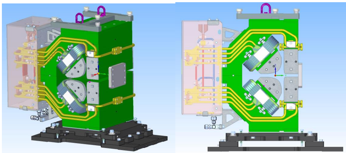
Рисунок 3.1.2.4. Модель диполя BDC.
