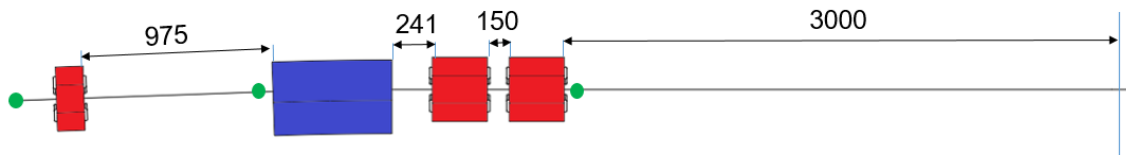
Рисунок 2.1.3.2. Компоновка прямолинейного прожегута и секции зануления дисперсионной функции (показана половина).
