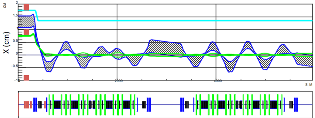
Рисунок 2.8.4. Огибающая впущенного пучка (синие линии, заштриховано) и огибающая циркулирующего пучка (зеленые линии) для согласованной инжекции.
