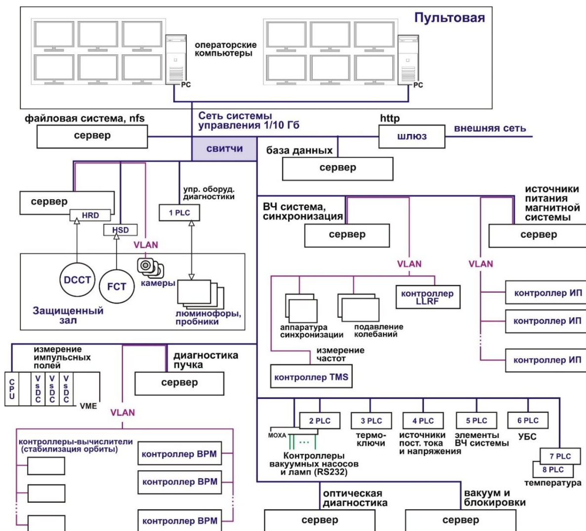
Рисунок 3.6.1.2. Блок-схема компьютеров и аппаратуры СУ SKIF.
