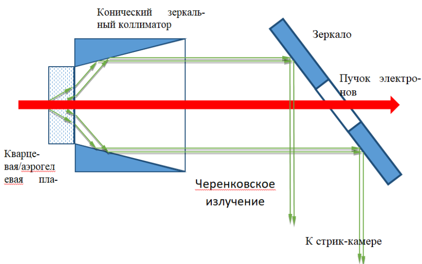
Рисунок 1.1.8.5. Схема черенковского датчика для измерения продольного профиля пучка.
