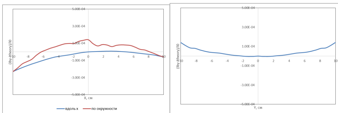
Рисунок 3.1.2.3. Слева – относительное отличие интеграла вертикального поля V_y вдоль оси x и на окружности радиуса R = 10 мм от такового на орбите. Справа – то же для координаты y .
