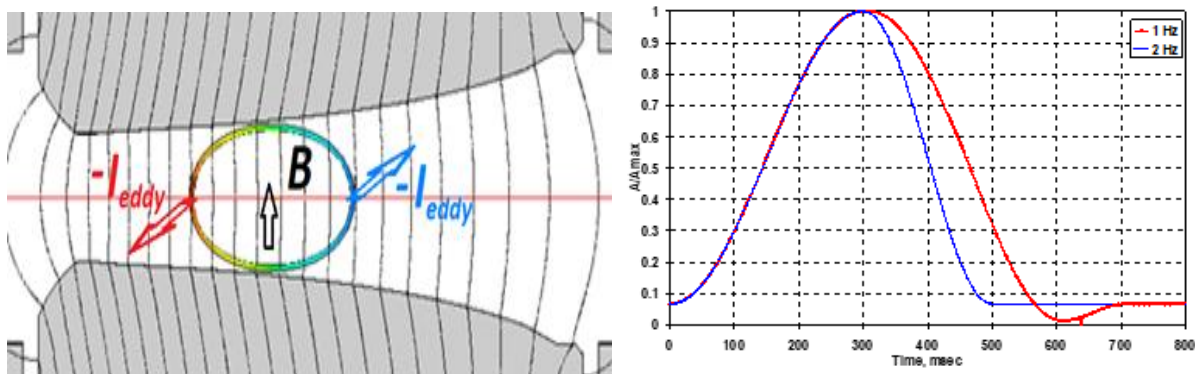
Рисунок 1.2.4.1. Слева – направление и плотность (показана цветом) вихревых токов в вакуумной камере диполя ВД (схематично). Справа – относительное изменение тока питания магнитов бустера во времени для частоты инжекции 1 Гц (красная кривая) и 2 Гц (синяя кривая).
