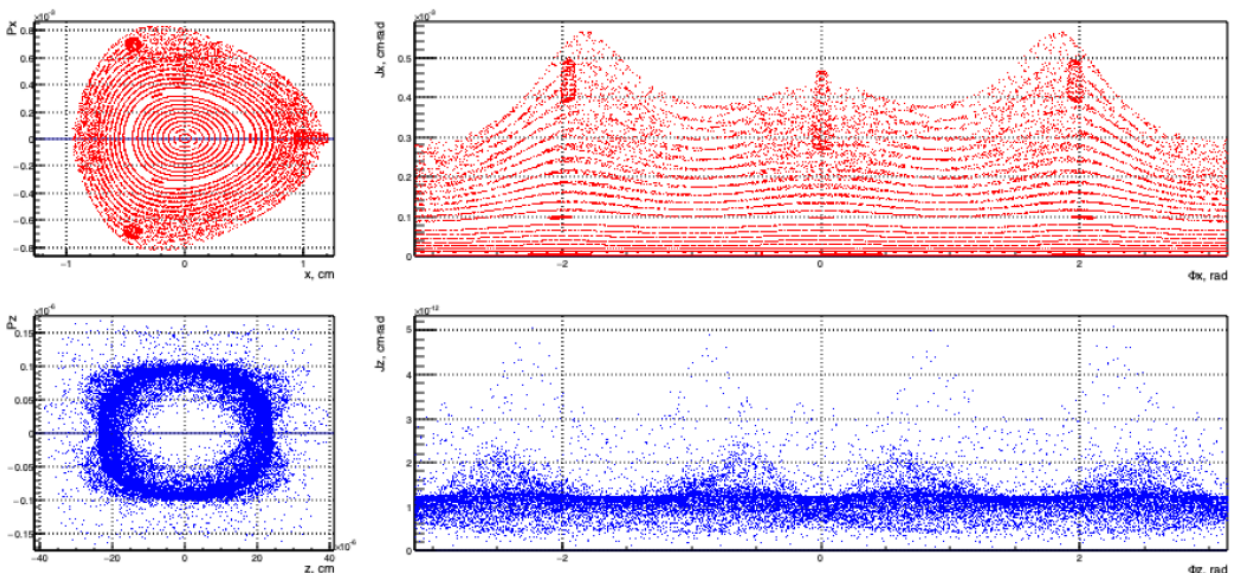
Рисунок 2.2.6. Фазовые траектории: горизонтальные (вверху) и вертикальные с учетом малых синхротронных колебаний.
