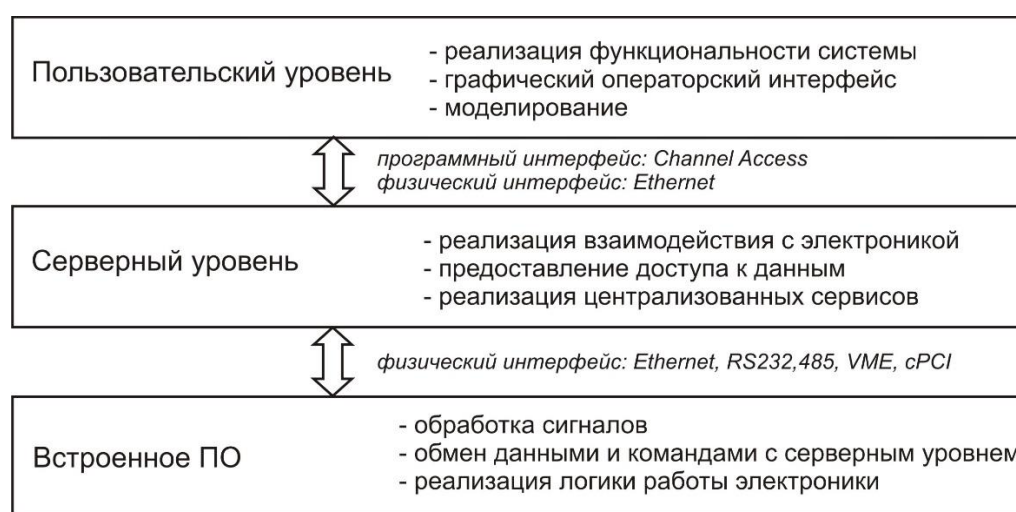
Рисунок 3.6.1.1. Трёхуровневая схема построения системы управления.
