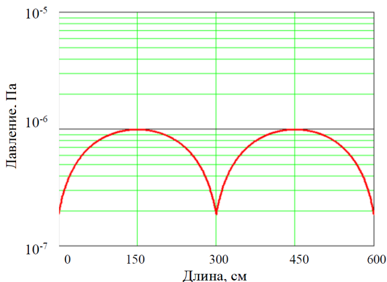
Рисунок 3.2.1.2. Распределение давления остаточного газа на шестиметровом участке вакуумной камеры линейного ускорителя. При расчетах коэффициент термического газовыделения 4 \times 10^{-8} м 3 ·Па/с/м 2 , эффективная быстрота откачки насосов 50 л/с по азоту.
