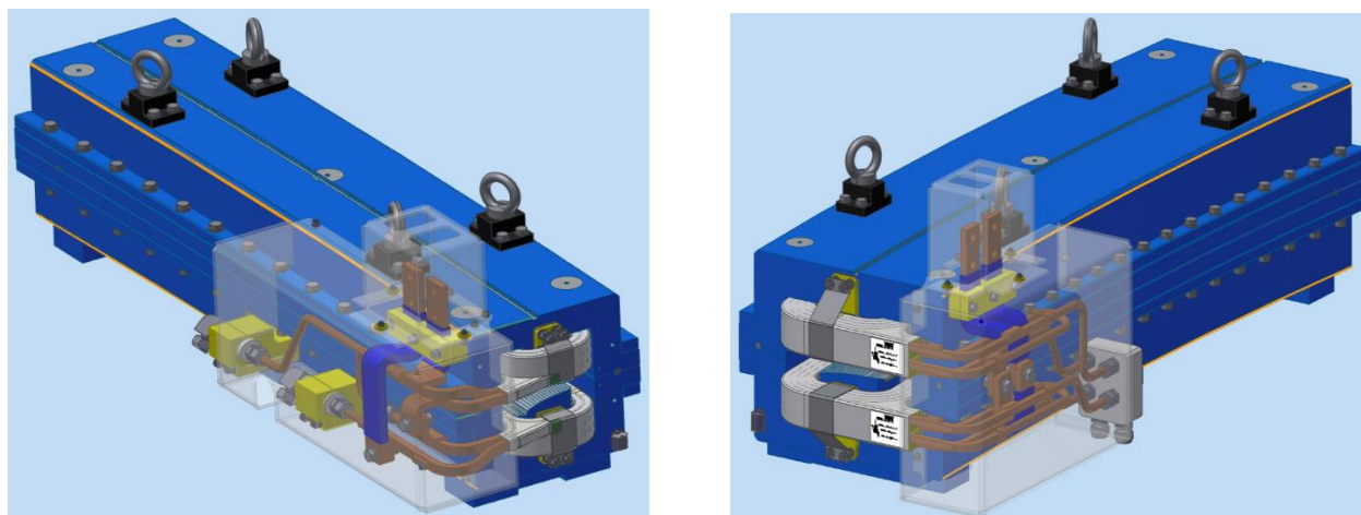
Рисунок 1.2.7.1. Внешний вид дипольных магнитов BF и BD.
