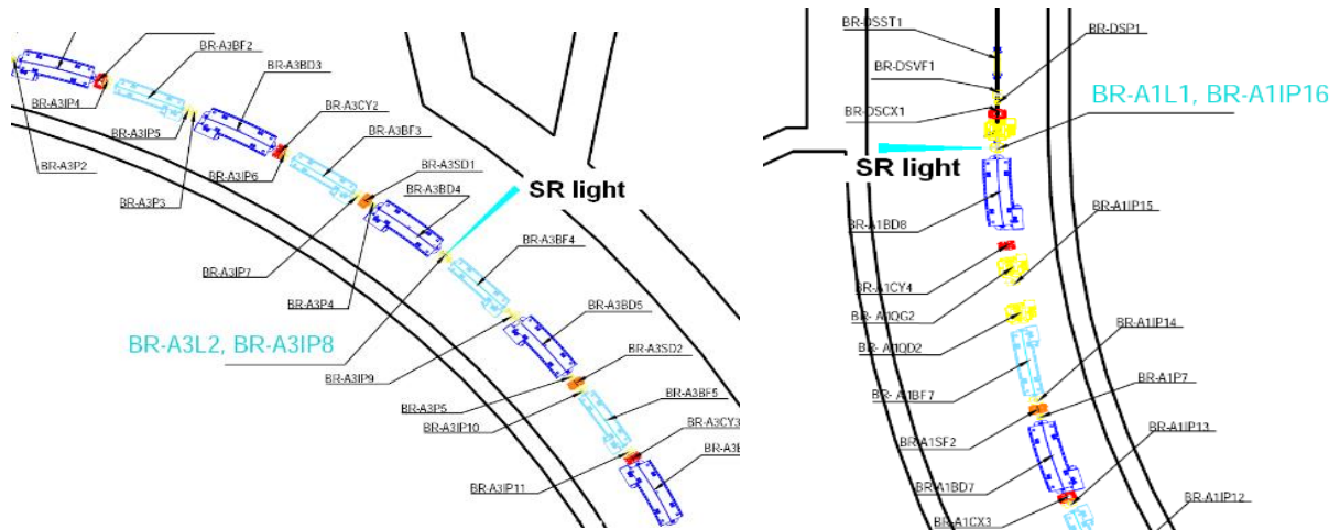
Рисунок 3.7.2.1. Расположение мест вывода СИ из вакуумной камеры бустера.
