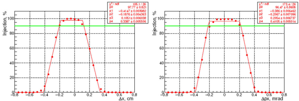
Рисунок 2.8.11. Зависимость эффективности инъекции от ошибки нацеливания пучка на впуске по горизонтали (слева – по координате, справа – по углу). 10^3 частиц, 1000 оборотов. Здесь и ниже зеленая линия показывает эффективность инъекции 90 %.
