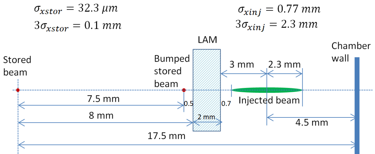
Рисунок 2.8.3. Схематичное положение пучков в момент инжекции.
