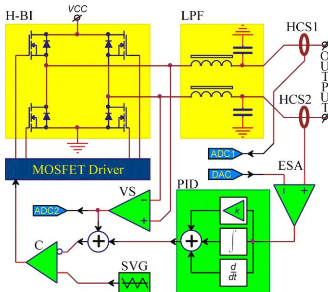
Рисунок 3.5.1.7. Структурная схема MPS-6. H-BI – мостовой инвертор. LPF – фильтр низких частот.
