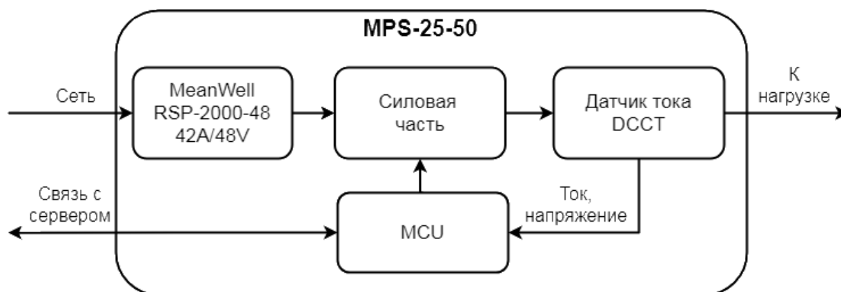
Рисунок 3.5.5.5. Структурная схема усилителя мощности MPS-25-50.
