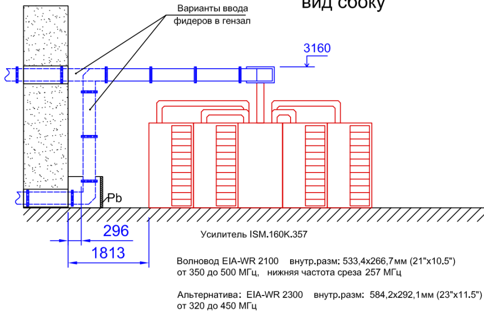
Рисунок 3.4.2.4. Вариант размещения ВЧ усилителей в генераторном зале 1 основного кольца.
