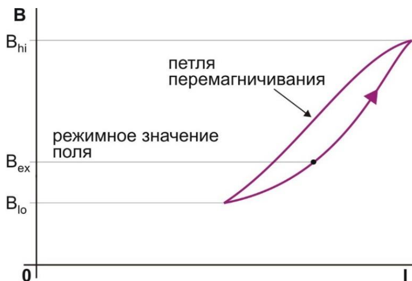
Рисунок 3.6.4.1. Диаграмма цикла перемагничивания.
