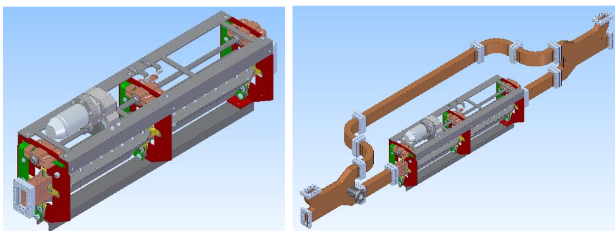
Рисунок 1.1.5.3. Волноводные фазовращатель (слева) и аттенюатор (справа).
