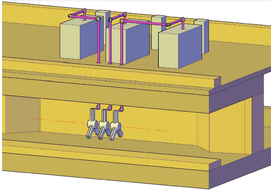
Рисунок 3.3.11. Схема размещения резонаторов и усилителей мощности бустера: внизу – резонаторы в радиационно-защищенном туннеле, вверху – усилители мощности и стойки управления в генераторном зале.
