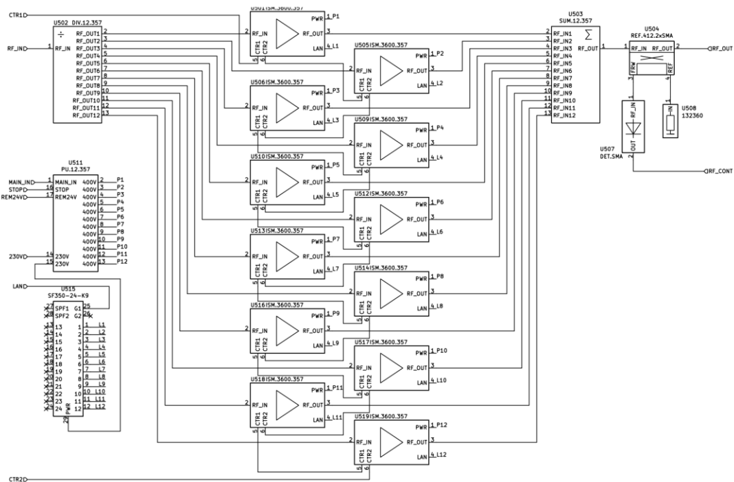
Рисунок 3.4.1.4. Блок схема усилительной стойки усилителя мощности ISM.160K.357.
