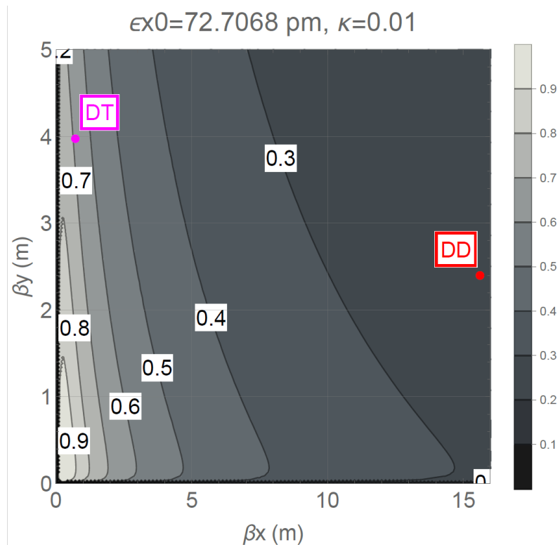
Рисунок 2.3.1.5. Нормализованная яркость ( V_t/V_{t_{\max}} ) в зависимости от бета-функций в центре вставного устройства. В более светлой зоне яркость выше.
