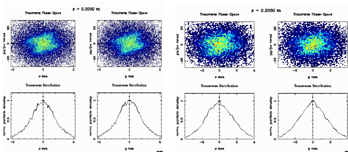
Рисунок 1.1.2.4. Поперечные фазовые профили пучка с зарядом сгустка 1 нКл (слева) и 0.3 нКл (справа).
