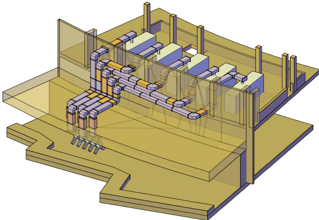
Рисунок 3.3.12. Схема размещения резонаторов и усилителей мощности накопителя: внизу – резонаторы в радиационно-защищенном туннеле, вверху – усилители мощности и стойки управления в генераторном зале.
