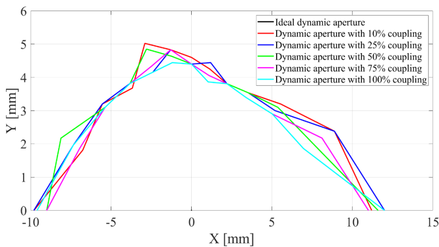
Рисунок 2.5.3.8. Поперечная динамическая апертура накопителя СКИФ для различных значений отношения вертикального и горизонтального эмиттансов (вплоть до 100%), управляемого скью-квадрупольными корректорами в бездисперсионных промежутках.
