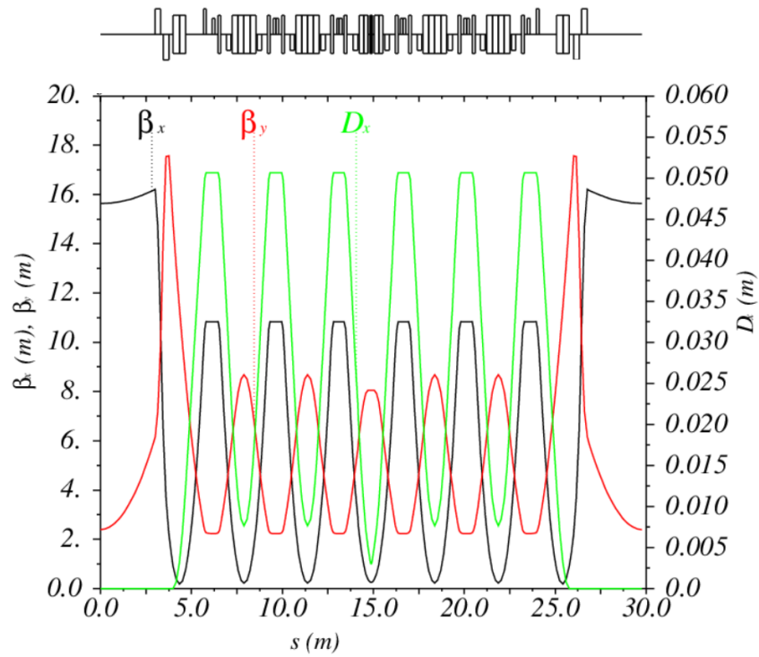
Рисунок 2.1.3.3. Структура и оптические функции суперпериода СКИФ.
