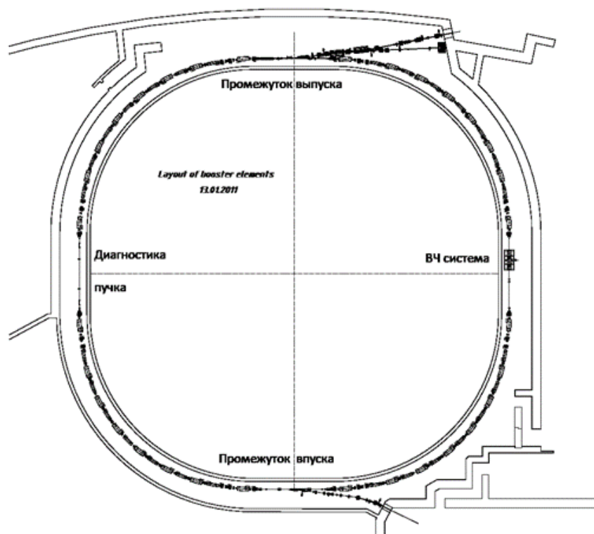
Рисунок 1.2.1.2. Схема магнитной системы синхротрона-бустера проекта SKIF.
