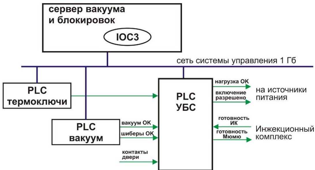
Рисунок 3.6.11.1. Блок-диаграмма системы блокировок.
