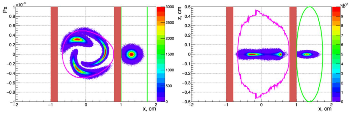
Рисунок 2.8.8. Горизонтальная фазовая плоскость (слева) и поперечное сечение на азимуте септумаламбертсона. Показаны впускаемый пучок на выходе из канала и три последовательных оборота впущенного пучка в накопителе. Статистика – 10^7 частиц. Размеры вакуумной камеры канала (зеленый эллипс на правом рисунке) \Delta x \times \Delta y = 7.5 \times 10 мм 2 . Розовая линия показывает границы динамической апертуры.
