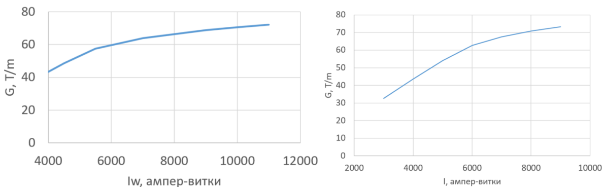
Рисунок 3.1.3.2. Зависимость градиента в центре линзы QFB (слева) и QDA, QFA (справа) от ампервитков питания.
