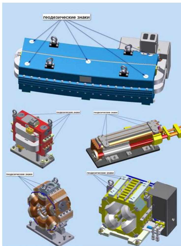
Рисунок 3.8.1. Геодезические знаки на элементах бустера.
