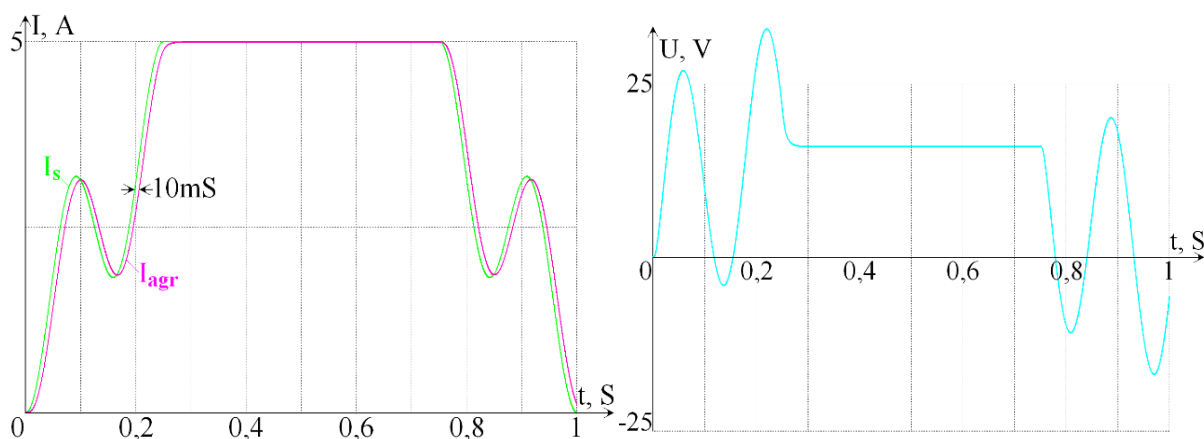
Рисунок 3.5.3.9. Временная зависимость выходного тока и напряжения источников питания корректоров. I_s – Заданное значение тока (сигнал ЦАП), I_{agr} – измеренное значение тока (сигнал LEM-датчика).
