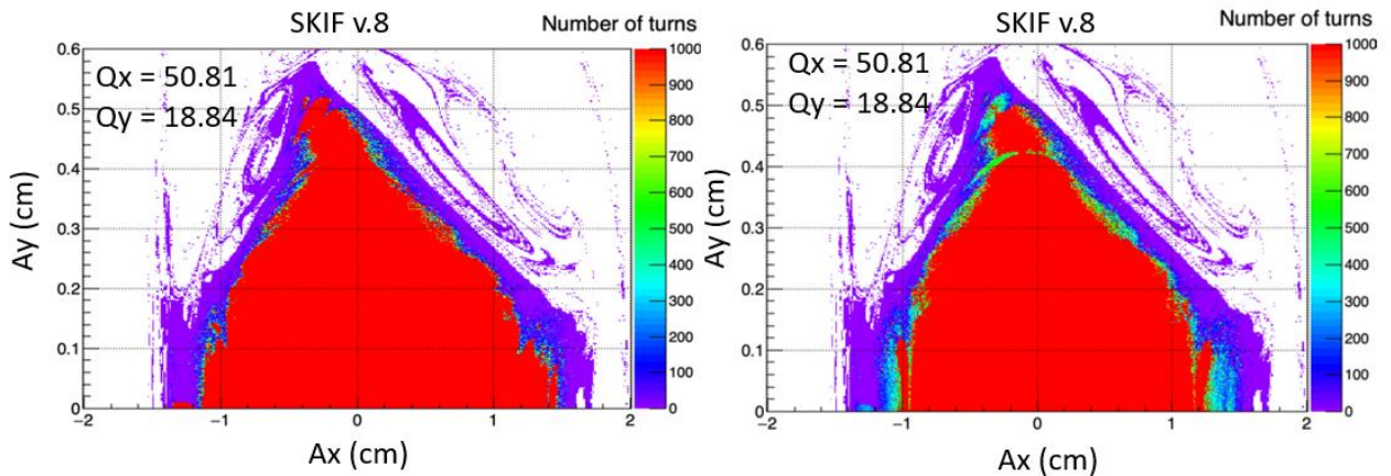
Рисунок 2.2.4. Поперечная динамическая апертура в выбранной рабочей точке. Слева без, справа с синхротронными колебаниями. Цвет показывает число оборотов устойчивого движения (Survival plot, Acceleraticum).
