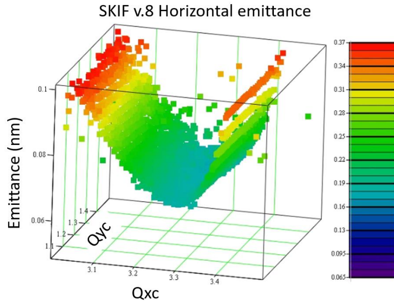
Рисунок 2.2.3. Изменение горизонтального эмиттанса накопителя в зависимости от выбранной рабочей точки частот.
