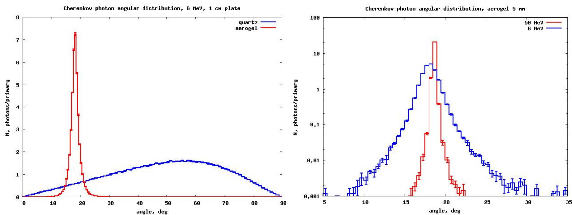
Рисунок 3.7.3.7. Слева – угловое распределений черенковских фотонов, испущенных при прохождении электроном с энергией 6 МэВ через аэрогель и кварц толщиной 10 мм. Справа – угловое распределение черенковских фотонов, испущенных электронами с энергиями 6 МэВ и 50 МэВ при прохождении аэрогеля толщиной 5 мм.
