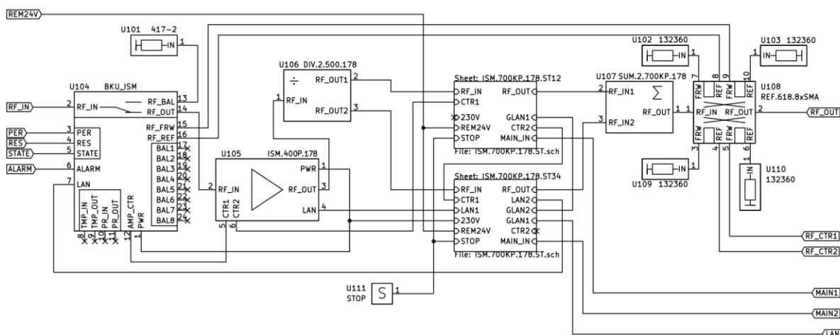
Рисунок 3.4.3.3. Блок схема усилителя мощности ISM.700KP.178.100.
