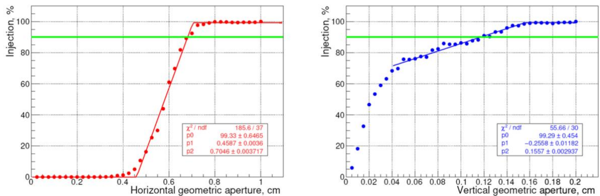
Рисунок 2.8.10. Зависимость эффективности инъекции от ограничения горизонтальной (слева) и вертикальной геометрических апертур в центре прямолинейного промежутка ( 10^3 частиц, 1000 оборотов).
