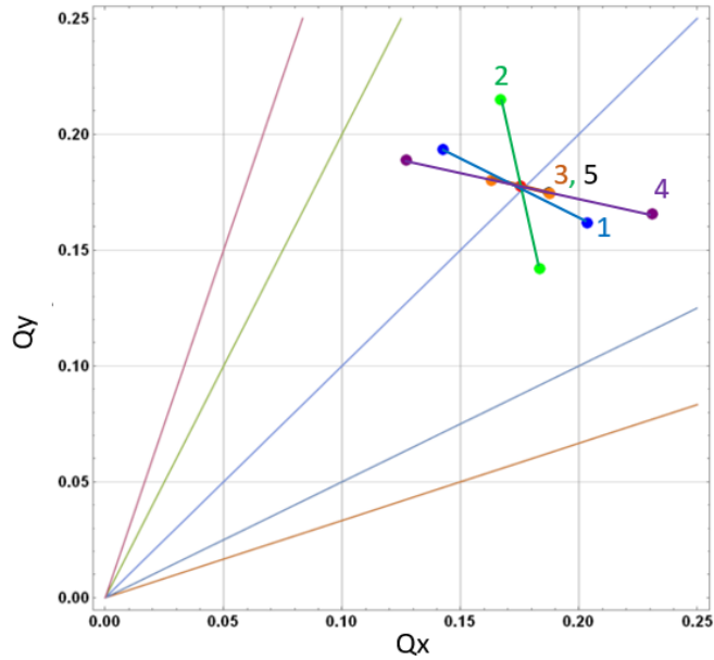
Рисунок 2.1.4.7. Девияция бетатронных частот при изменении градиента квадрупольных линз на \pm 1\% . Действие третьей и пятой квадрупольных линз совпадает.
