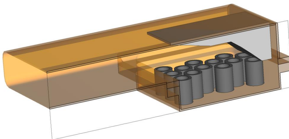
Рисунок 3.3.7. Эскиз нагрузки ВМ с СВЧ поглотителями.
