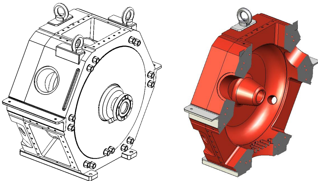
Рисунок 3.3.5. Корпус резонатора.
