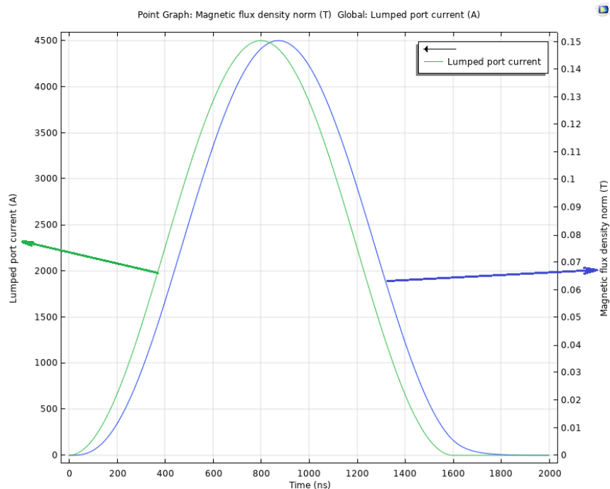
Рисунок 1.3.3.4. Импульс магнитного поля в центре на оси кикерного магнита (синий), и импульс тока на пластинах, длительностью 1600 нс по основанию (зеленый). Толщина напыления чистого титана 2.5 мкм.
