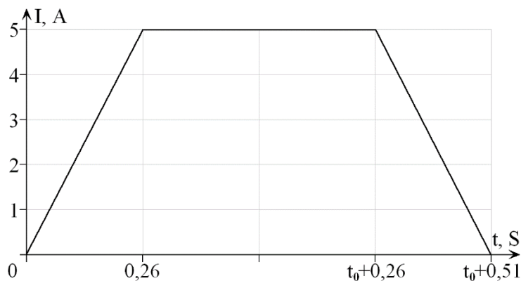
Рисунок 3.5.3.6. Временная зависимость тока в секступольной линзе бустера.
