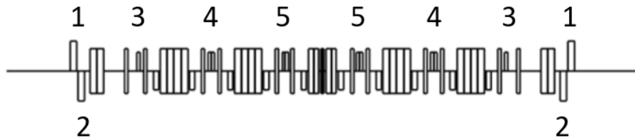
Рисунок 2.1.4.1. Линзы, используемые для настройки оптики.
