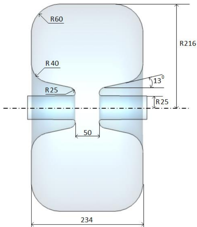
Рисунок 3.3.1. Внутренняя геометрия резонатора.
