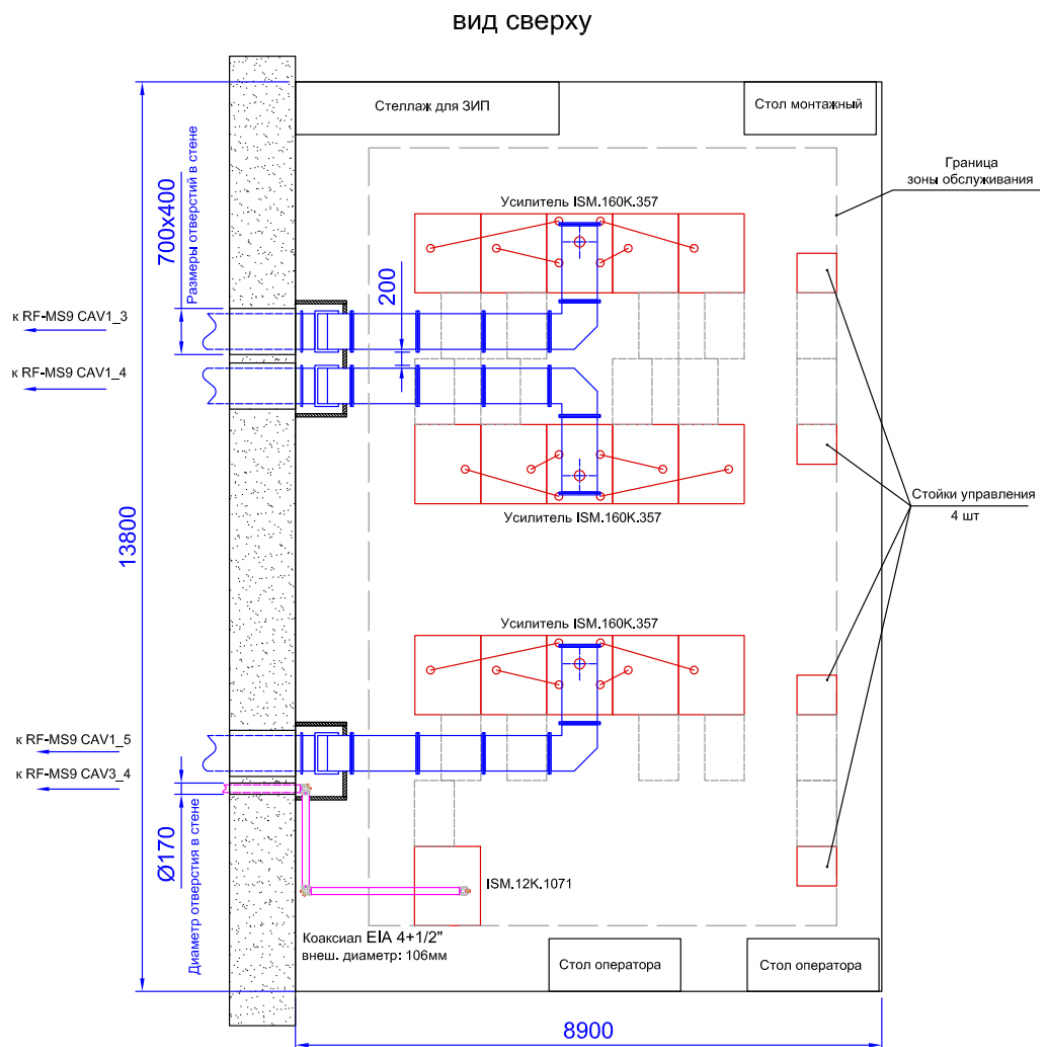
Рисунок 3.4.2.5. Вариант размещения ВЧ усилителей в генераторном зале 2 основного кольца.
