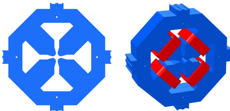
Рисунок 3.1.3.1. Квадрупольная линза QFB. Профиль ярма – слева, трехмерная модель – справа.
