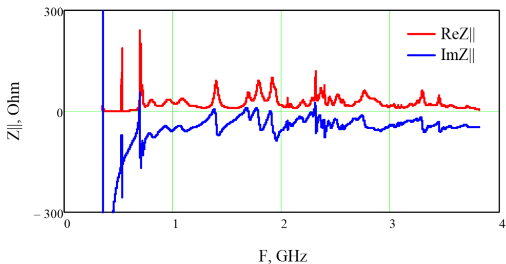
Рисунок 2.7.1.4. Спектр продольного импеданса ВЧ-резонатора основной гармоники.
