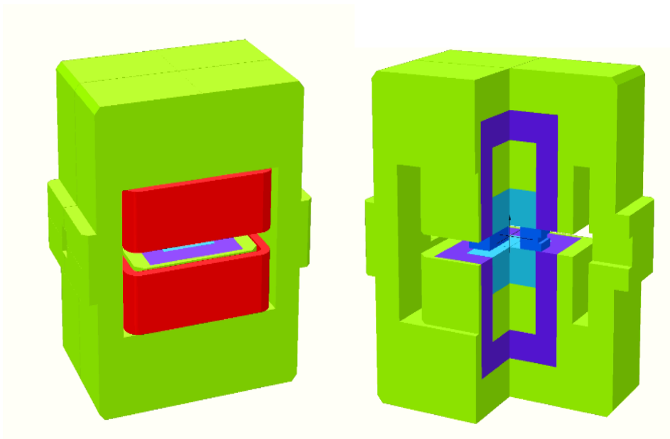
Рисунок 3.1.2.7. Дипольный магнит ВРС. Ярмо магнита показано зеленым цветом, постоянные магниты – синим, пермендюрный полюс – голубым и корректирующая обмотка – красным.
