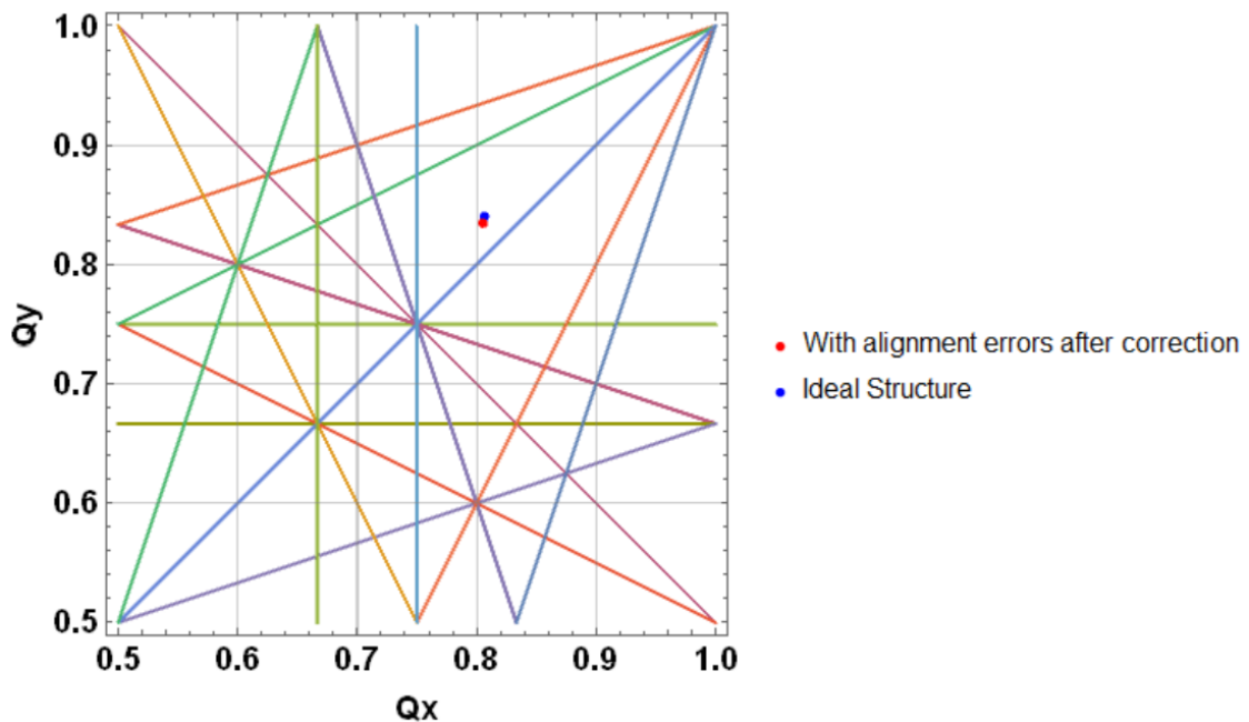
Рисунок 2.5.3.2. Сетка резонансов для структуры SKIF. Синяя точка – рабочие частоты в идеальной структуре без связи и ошибок выставки элементов; красная точка – частоты, соответствующие вертикальному смещению секступолей 40 \mu м (горизонтальное смещение отсутствует) и повороту квадруполей на 150 \mu рад.
