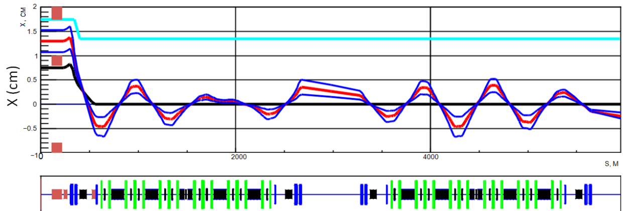
Рисунок 2.8.5. Центральные траектории впускаемого (красный) и накопленного (черный) пучков при «идеальной» инжекции. Синим цветом показаны центральные траектории впускаемого пучка, отклоненного по горизонтали на \Delta x_{inj} = \pm 2.3 \text{ мм} = \pm 3\sigma_{xinj} .
