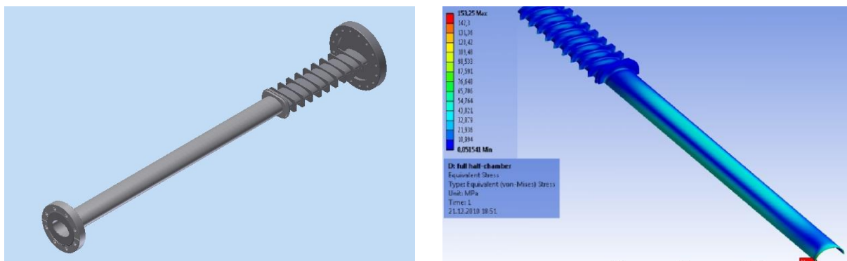
Рисунок 3.2.2.6. Вакуумная камера импульсного BUMP-магнита (слева). Распределение напряжении (МПа) в камере из-за СИ (справа).
