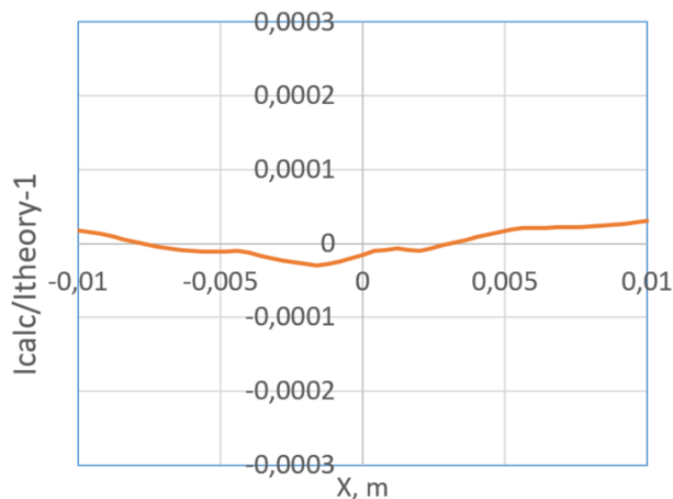
Рисунок 3.1.2.6. Качество интеграла поля на орбите магнита BDC.
