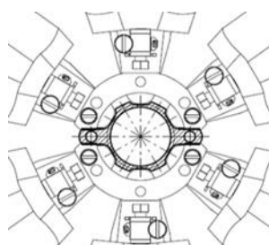
Рисунок 3.2.3.7. Профиль вакуумной камеры в секступольных магнитах.
