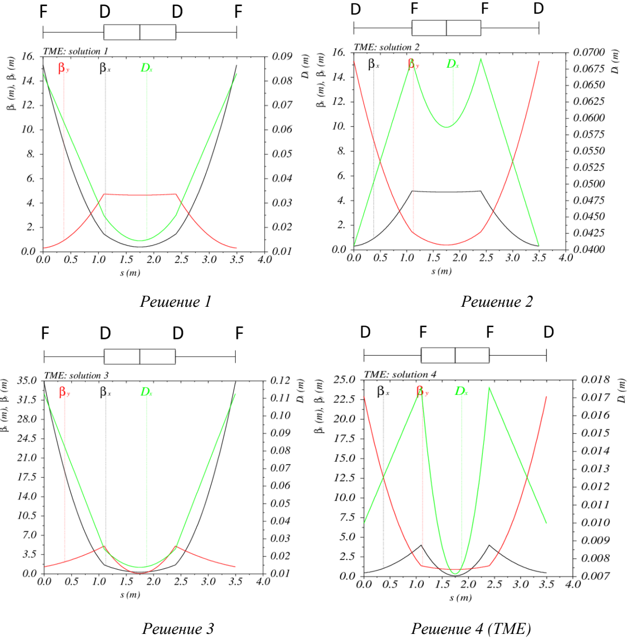
Рисунок 2.1.2.2. Четыре периодических решения для магнитной ячейки с Рисунка 2.1.2.1 . F и D обозначают фокусирующие и дефокусирующие квадрупольные линзы. Решение 4 соответствует минимально достижимому эмиттансу (TME).
