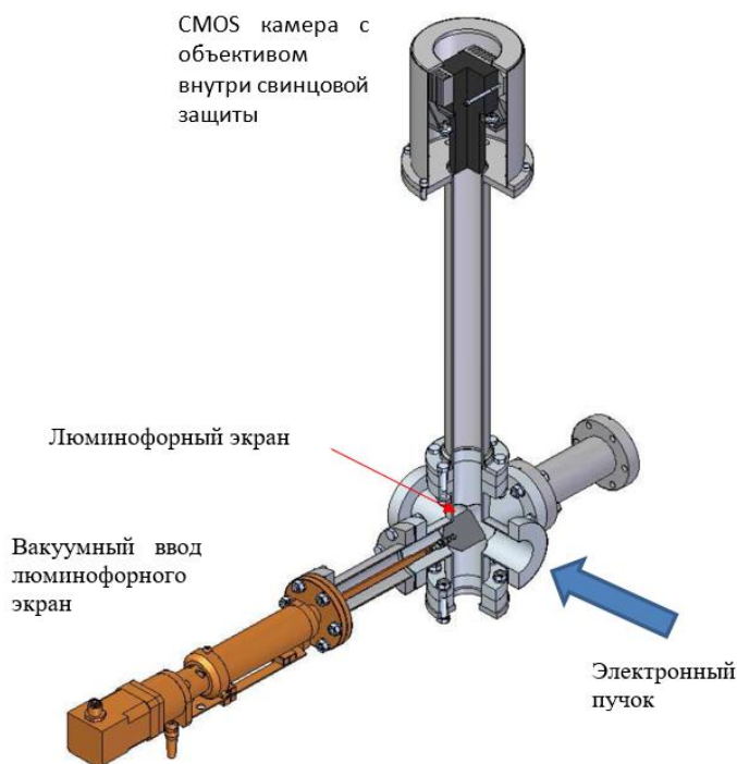
Рисунок 3.7.3.1. Схема люминофорного экрана линейного ускорителя
