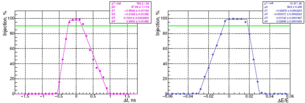
Рисунок 2.8.13. Зависимость эффективности инжекции от ошибки времени влета пучка (слева) и отклонения средней энергии пучка (справа). 10^3 частиц, 1000 оборотов.
