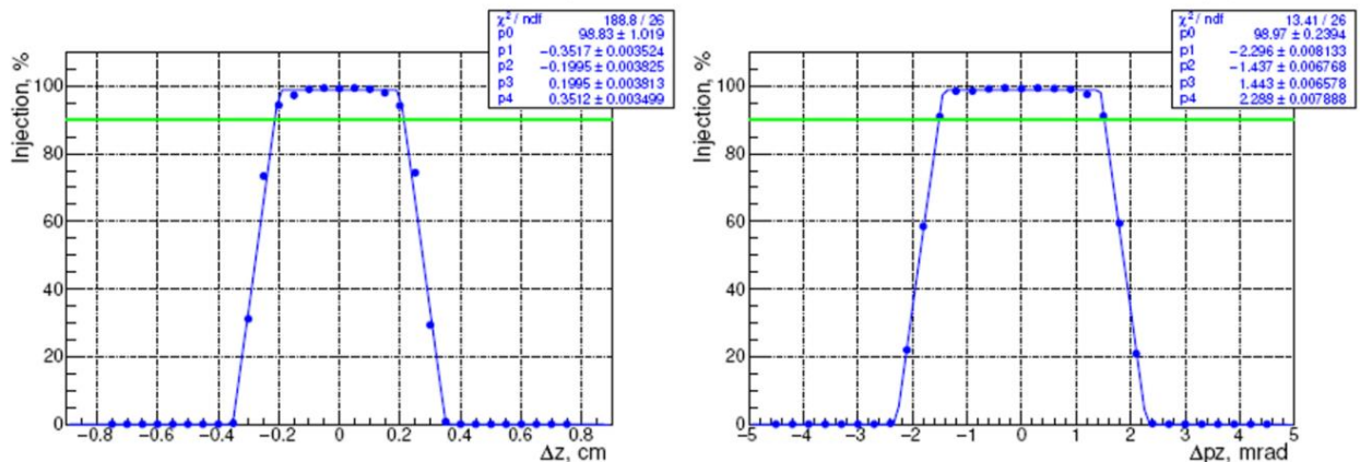
Рисунок 2.8.12. Зависимость эффективности инъекции от ошибки нацеливания пучка на впуске по вертикали (слева – по координате, справа – по углу). 10^3 частиц, 1000 оборотов.
