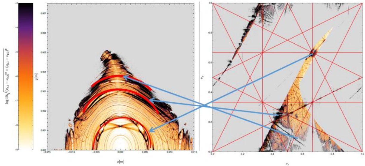
Рисунок 2.2.11. FMA для динамической апертуры источника СИ SKIF. Слева – в пространстве поперечных координат, справа – в пространстве бетатронных частот («футпринт», footprint). Темные и светлые области показывают стохастические и регулярные траектории соответственно.
