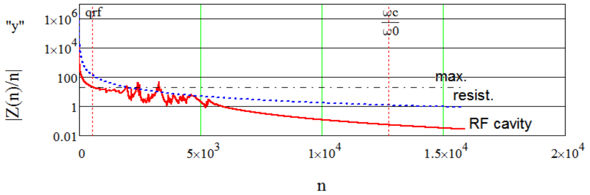
Рисунок 3.3.10. Нормализованный продольный (вверху) и поперечный (x, y) импеданс для пяти ускоряющих ВЧ резонаторов и для резистивного импеданса вакуумной камеры; max - максимальное значение нормализованного импеданса по МВН; \omega_c – частота среза, выше которой возможно развитие МВН.
