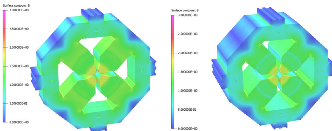
Рисунок 3.1.3.3. Цветом показана карта насыщения ярма линз QFB (слева) и QDA, QFA (справа) при максимальном градиенте.
