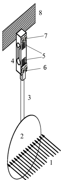
Рисунок 1. Тягомер на основе тензометрической балки. 1- поток плазмы, 2 – мишень, 3 – алундовый стержень, 4 – тензобалка, 5 – тензодатчики, 6, 7 – зажимы, 8 - консоль.
