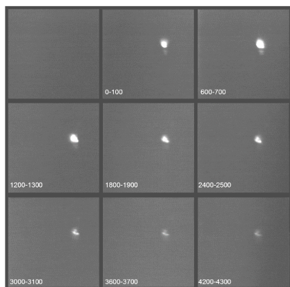
Рис. 1. Девятикадровое изображение поверхностного скользящего разряда в потоке с наклонной ударной волной. Число Маха потока 1.58, плотность 0.06 кг/м 3 . Время на кадрах указано в наносекундах.
