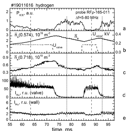
Рис.1. Эволюция мощности ICE в диапазоне 5-80 МГц – окно a, \bar{n}_e(0,574) и \bar{n}_e(0,718) – усредненная плотность, измеренная по вертикальным хордам на больших радиусах 0,574 м (вблизи магнитной оси) и 0,718 м (крайний канал СВЧ интерферометра) – окна b и c, U_{valve} – напряжение, подаваемое на пьезоэлектрический клапан напуска – окно b, сигналы мониторов H_\alpha вблизи клапана напуска водорода – окно d и вдали от клапана – окно e.
