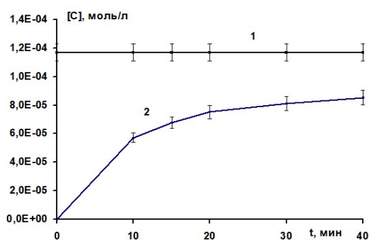
Рис. 1 [С] – концентрация продуктов, моль/л; t, мин – время, в течение которого активировалась излучением проба воды. Цифрами обозначены: (1) – исходная концентрация пробы фенола 25 мг/л в смеси с дистиллированной водой 1:1; (2) – концентрация 4-нитрофенола в смеси исходного фенола 25 мг/л и воды 1:1, активированной излучением в течение времени t через два дня после обработки.
