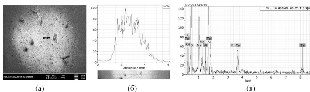
Рис. 1. Пленка тантала на стеклянной подложке (растровый микроскоп EVO-40): (а) – область осаждения Ta; (б) – относительная концентрация Ta в области напыления; (в) – элементный состав пленки.
