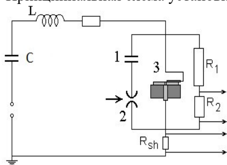
Рис. 1. Схема капиллярного плазмотрона. 1 – иницирующая емкость, 2 – коммутатор, 3 – капилляр, R_1 , R_2 – сопротивления делителя напряжения, R_{sh} – сопротивление шунта для определения тока разряда, C – батарея конденсаторов.
