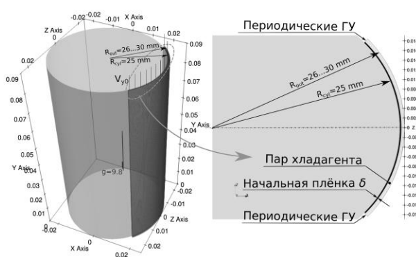
Рис. 1. Схема течения.
