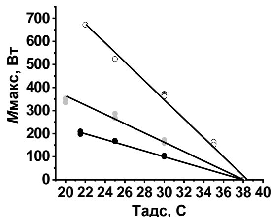
Рис. 1. Зависимость максимальной мощности от температуры адсорбции для АТО с различной геометрией.
