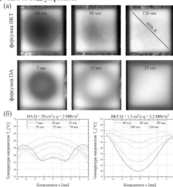
Рис. 1. (а) Термограммы поверхности нагревателя при спрейнго охлаждении для различных форсунок и на различных расстояниях; (б) Профили температуры поверхности вдоль диагонали нагревателя.
