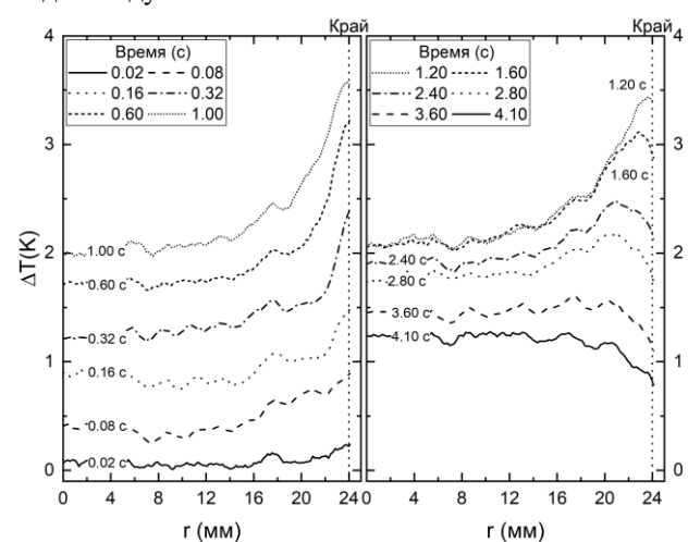
Рис. 1 Распределение температуры вдоль (X, 0) торцевой вставки в различные моменты времени.
