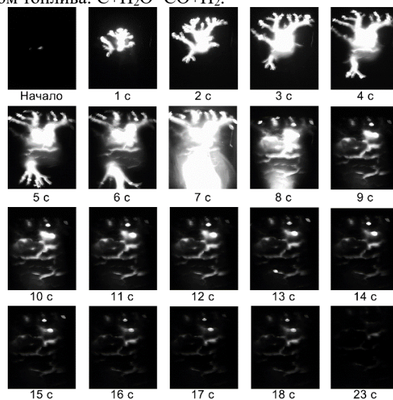
Рис. 2. Визуализация процесса СВЧ-пиролиза с момента иницирования по 23 с.
