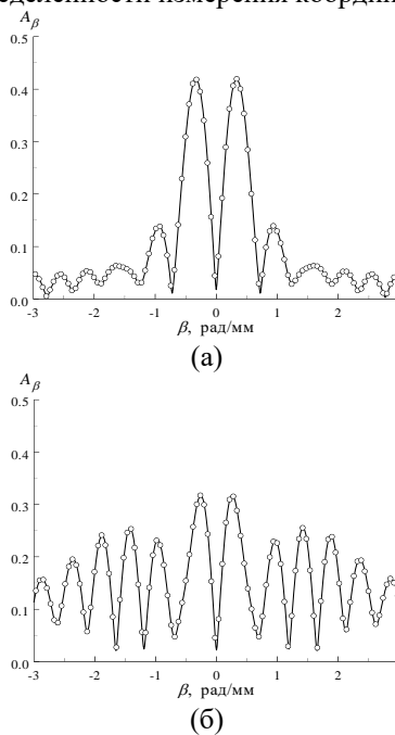
Рис. 3. Волновой спектр амплитуды стационарного возмущения, порожденного в пограничном слое пластины с радиусом притупления (а) 0,04 мм; (б) 0,5 мм.
