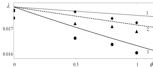
Рис. 1. Зависимость коэффициента теплопроводности [ \text{Вт}/(\text{м}\cdot\text{К}) ] наногазовзвесей от объемной концентрации наночастиц ( \phi \cdot 10^3 ).
