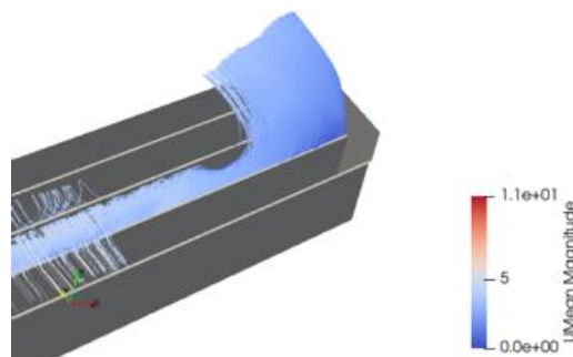
Рисунок 3. Структура течения в случае циклических граничных условий на боковых стенках.
