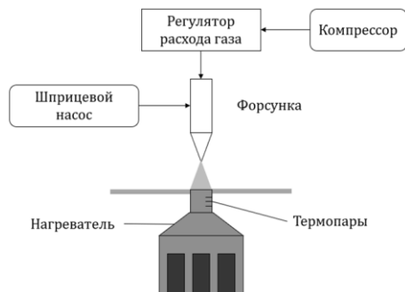
Рис. 1. Схема установки для измерения теплового потока, отводимого спреем.
