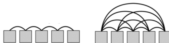
Рис. 2. Схемы использования соседних кадров при расчете поля скорости двухкадровым кросскорреляционным и многокадровым кросскорреляционным методом.
