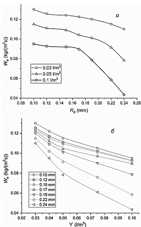
Рис. 1. Значения скоростей испарения капель воды с учетом их разных начальных размеров и концентраций.
