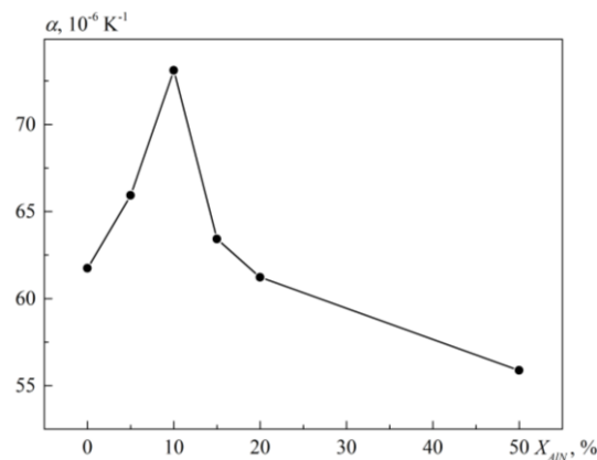
Рис. 3. Концентрационная зависимость ТКЛР ПКМ при T = 300 К.
