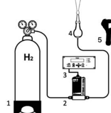
Рис. 1. Экспериментальная установка: 1 – баллон со сжатым водородом, 2 – клапан расходомера MKS 1179B (MKS Instruments), 3 – 2- каналный контроллер расходомера MKS PR4000B (MKS Instruments), 4 – пара сопел d_1 = d_2 = 200 мкм, 5 – тепловизор CEM DT-9897H.
