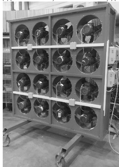
Рис.1 Аэродинамическая стена.
