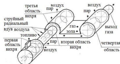
Рис.1. Схема четырехкамерного реактора.
