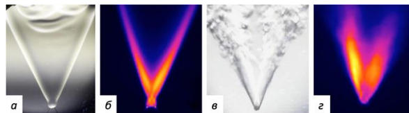
Рис. 2. Взаимодействие двух факелов при истечении микроструи водорода из сопел с d_1 = d_2 = 200 мкм, а), б): U_1 = U_2 = U = 457 м/с ( Re = 932 ); в), г): U_1 = U_2 = U = 914 м/с ( Re = 1865 ).
