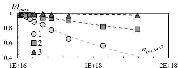
Рис.1. Зависимость относительной амплитуды сигнала I/I_{max} , регистрируемого масс-спектрометром, от плотности газа в послескimmerной секции n_{pst} для атомов (1), димеров (2) и тримеров (3) аргона при среднем размере кластеров в потоке \langle S \rangle \sim 50 .
