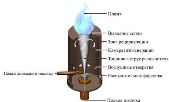
Рис 1. Схема горелочного устройства.
