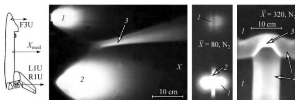
Рис. 1. Структура поля течения для модели Space Shuttle. Зона свободной струи (1), зоны взаимодействия двух (2) и трех (3) струй.
