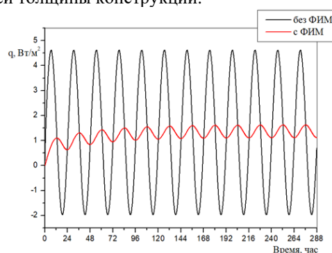
Рис. 1. Сравнение плотности теплового потока на внутренней поверхности без ФИМ и с ФИМ.
