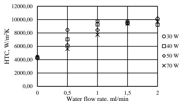
Рис. 2. Зависимость коэффициента теплообмена от расхода жидкости для форсунки с капилляром 0,25 мм при расходе газа 5 л/мин.
