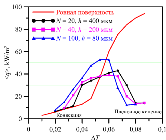
Рис. 2. Кривые кипения на ровной (сплошная линия) и шероховатых поверхностях (размер каверн: круги – 400 мкм, квадраты – 200 мкм, треугольники – 80 мкм).
