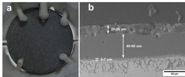
Рисунок 1. Образцы сплава с покрытием перед термоциклированием. (а) Оптические изображения подложки после нанесения геленитового покрытия; (б) СЭМ-изображения поперечного сечения образца, покрытого геленитом.
