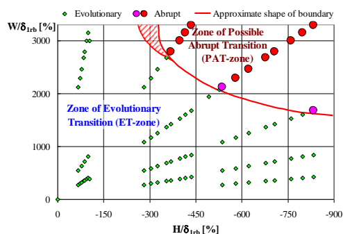
Рис. 1. Сценарии перехода в зависимости от ширины W и глубины H канавки. Оба параметра нормированы на местную толщину вытеснения d_{1rb} . Эволюционные режимы — ромбики, внезапный переход — кружки.
