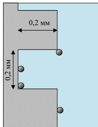
Рис. 1. Схема вариантов расположения парового зародыша на начальной стадии численного моделирования роста пузыря.
