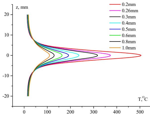
Рис. 1. Распределение температуры в алмазном стекле по высоте в сечении x=0, y=0, -20\text{мм} \leq z \leq 20\text{мм} . Толщина алмазного стекла: от 0.2 мм до 1 мм.
