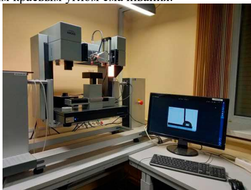
Рис. 1. Установка KRUSS DSA 100 для измерения краевых углов смачивания.
