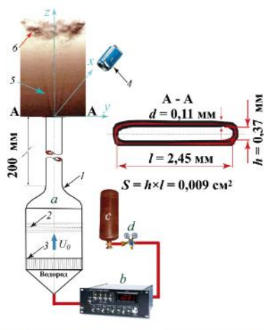
Рис. 1. Схема эксперимента: а – сопловой аппарат; б – блок управления электромагнитным клапаном расхода; с – баллон сжатого водорода (100 атм.); д – редуктор. Сопловой аппарат (а) состоит из форкамеры (1), набора детурбулизирующих сеток (2), хонейкомба (3) и микротрубки длиной 200 мм с щелевым микросоплом. С помощью цифровой видеокамеры или тепловизора (4) фиксировались теневые картины сверхзвуковых ячеек (5) или топология пламени (6).
