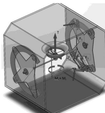
Рис.2 Измерение сил на ячейке в аэродинамической установке АТ-324 ИТПМ.
