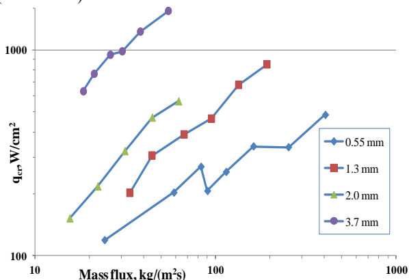
Рис. 1. Влияние удельного массового расхода (массовой скорости) воды и высоты канала (указана в легенде) на критический тепловой поток q_{cr} для нагревателя 3x3 мм 2 (ширина канала 30 мм).
