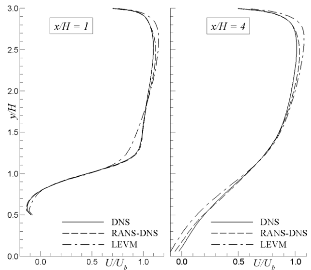
Рис. 2. Профили средней скорости в PH-течении.
