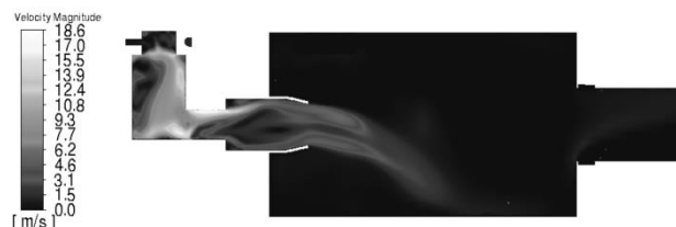
Рис.2 Магнитуда скорости в тангенциальном горелочном устройстве и топочной камере.
