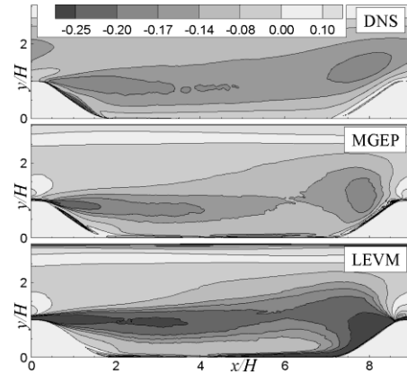
Рис. 1. Изолинии b_{12} , полученные из данных DNS [2] и из априорных оценок моделей MGEP и LEVM в PH-течении.
