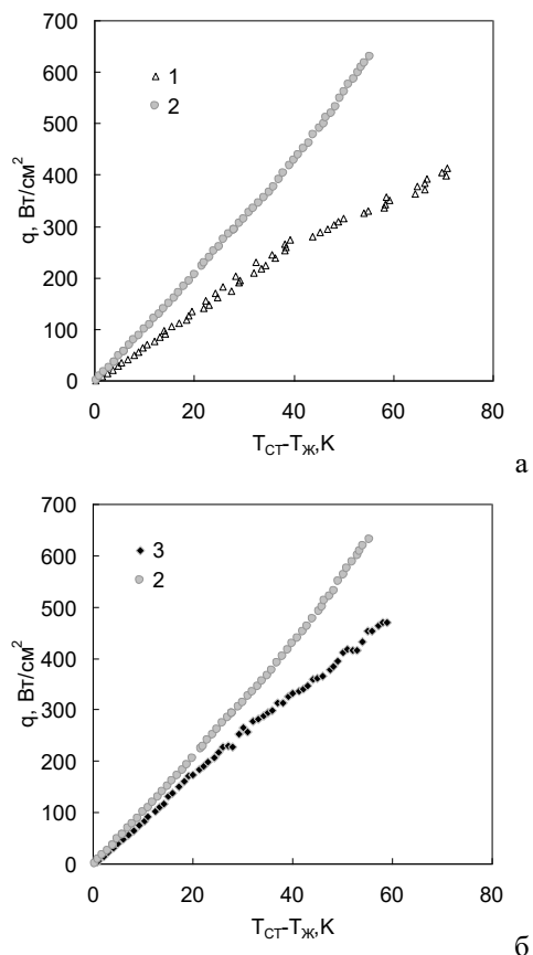
Рис.1. Зависимость снимаемого теплового потока от перегрева температуры стенки. (а) V струй=7,4 м/с, (б) \Gamma = 12,6 г/см 2 сек; 1- D =10мм V =7,4 м/с, 2- D =8мм V =7,4 м/с, 3- D =10мм V =11,5 м/с.
