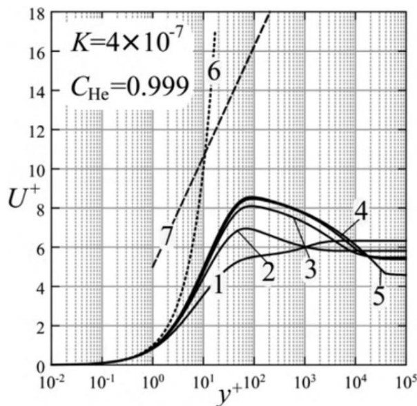
Рис. 2. Профили скорости при K = 4 \times 10^{-7} : 1 - 5 – профили скорости при Re \times 10^6 = 0.5, 1, 5, 10, 60 соответственно; 6 – ламинарный подслой; 7 – логарифмический закон.
