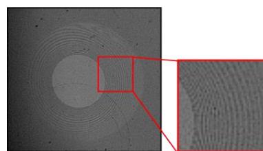
Рис. 2. Полученный с помощью LED интерферометрии кадр роста парового пузыря при кипении воды ( p_s = 101,3\ \text{kPa} , q_{input} = 60\ \text{kW/m}^2 ).
