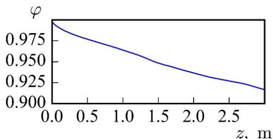
Рис. 1. Распределение истинного объемного паросодержания по длине канала при конденсации R113, p = 0.33 МПа, массовая скорость 180 кг/(м 2 с).
