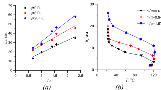
Рис. 2. Высоты поднятия струи в зависимости от отношения скорости струи и потока v/u , а также частоты пульсаций f струи (а); профили температуры потока в зависимости от удаления от среза сопла струи (б).
