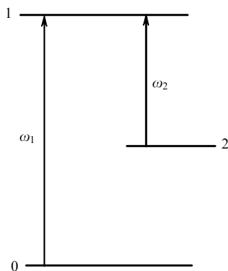
Рис.2. Энергетическая диаграмма трехуровневого атома, взаимодействующего со слабым пробным (частота \omega_1 ) и сильным управляющим (частота \omega_2 ) лазерными полями.
