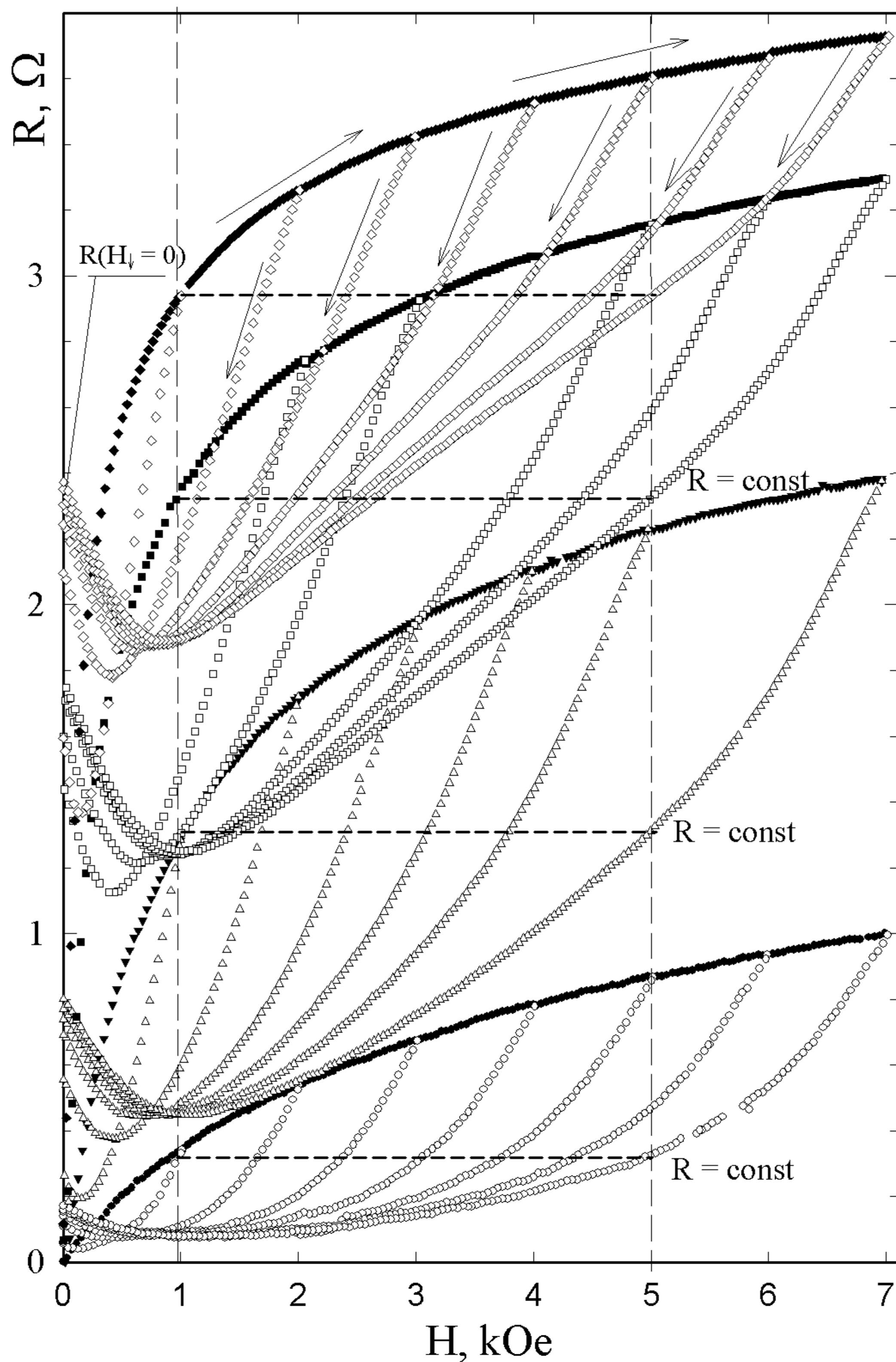
Рис.10. Гистерезисные зависимости R(H) образца YBCO + 30CuO при различных значениях I (2, 4, 7, 10 мА – снизу вверх) и различных величинах H_{max} = 1, 2, \dots, 7 кОе при T = 4.2 К. Зависимости R(H\uparrow) (поле возрастает) показаны закрытыми символами, а зависимости R(H\downarrow) (поле убывает) – открытыми символами. Каждое измерение для нового значения H_{max} и I проведено после снятия магнитной предыстории. Штриховые линии поясняют определение значения полевой ширины гистерезиса \Delta H_{R=const} = H\downarrow - H\uparrow при H\downarrow = 5 кОе. В этом случае при H_{max} = 7 кОе величина \Delta H(H\downarrow = 5 \text{ кОе}) \approx 4 кОе для всех зависимостей R(H) на этом рисунке).
