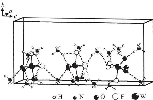
Рис. 6. Система водородных связей (\text{NH}_4)_3\text{WO}_3\text{F}_3 в триклинной фазе G_2 .
