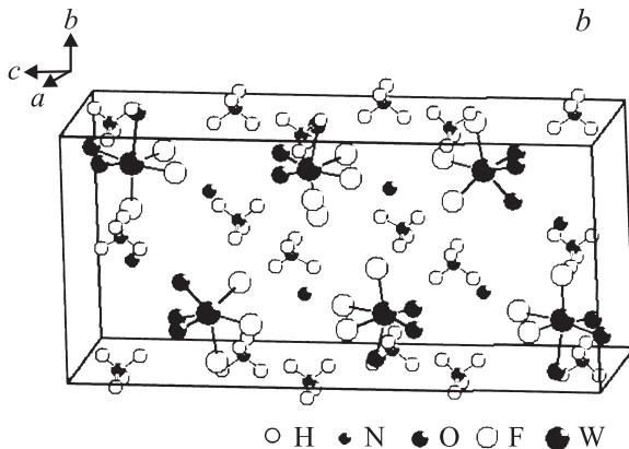
Рис. 5. Структуры фаз (\text{NH}_4)_3\text{WO}_3\text{F}_3 : а — кубической G_0 при T = 298 ; б — триклинной G_2 при T = 133 .
