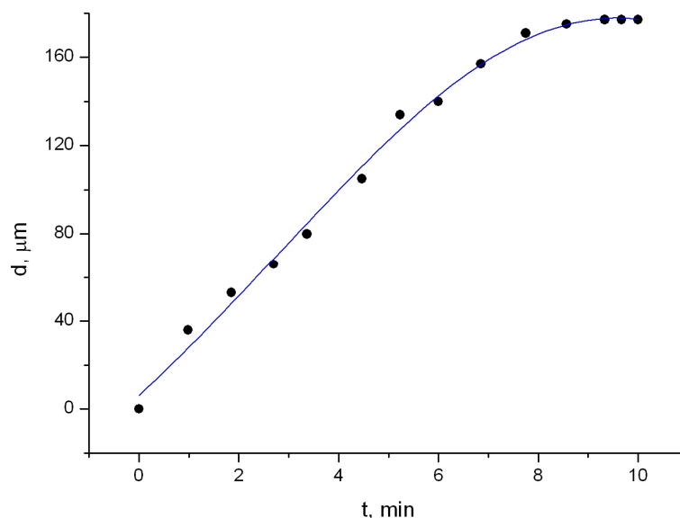
Рис. 5. Зависимость диаметра растущего домена МББА, нанесенного через 1 мин на пленку ПК, растворенного в дихлорметане, от времени при температуре 23 °С (точки). Сплошная линия – интерполяция
