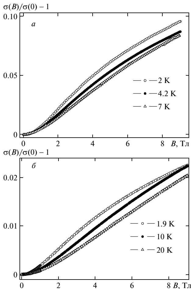
Рис. 3. Зависимости поправки к проводимости \sigma(B)/\sigma(0) - 1 от магнитного поля B при различных температурах для бумаги (а) и многослойных углеродных нанотрубок диаметром (20-22) \pm 8 нм (б)
