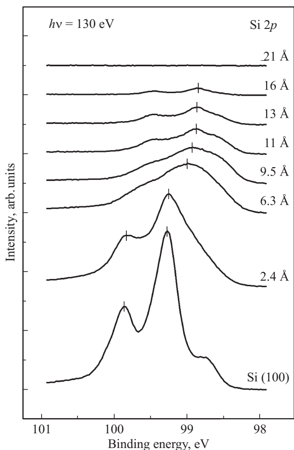
Рис. 1. Спектры 2 p -электронов кремния, полученные для разных доз напыления марганца на поверхность Si(100) 2 \times 1 при комнатной температуре.
