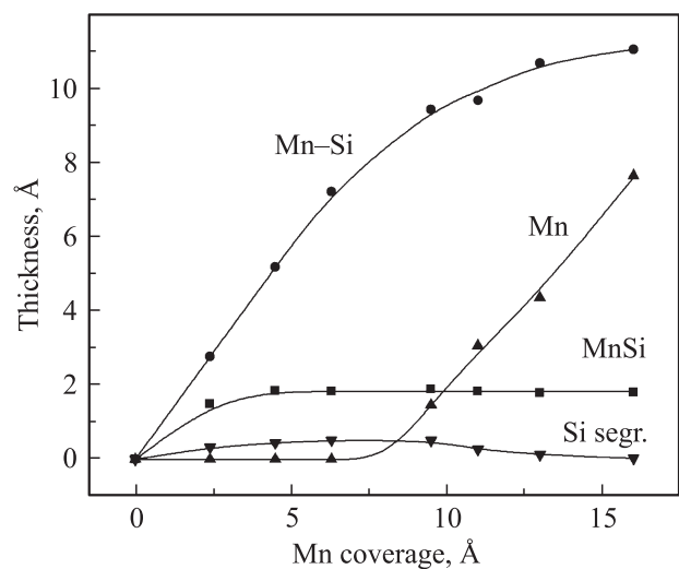
Рис. 5. Зависимости средней толщины слоев различных химических фаз, образующихся в области интерфейса Mn/Si, от величины покрытия.
