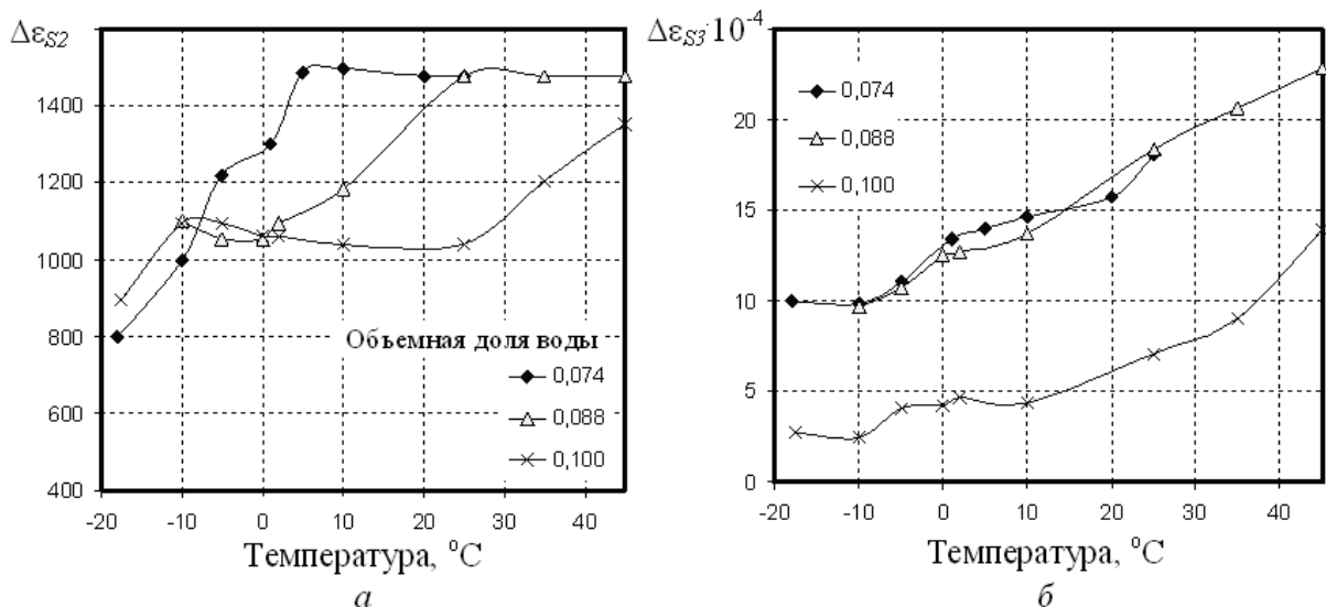
Рис. 6. Температурная зависимость параметров \Delta\epsilon_{S2} и \Delta\epsilon_{S3} для второй (а) и третьей (б) областей релаксации
