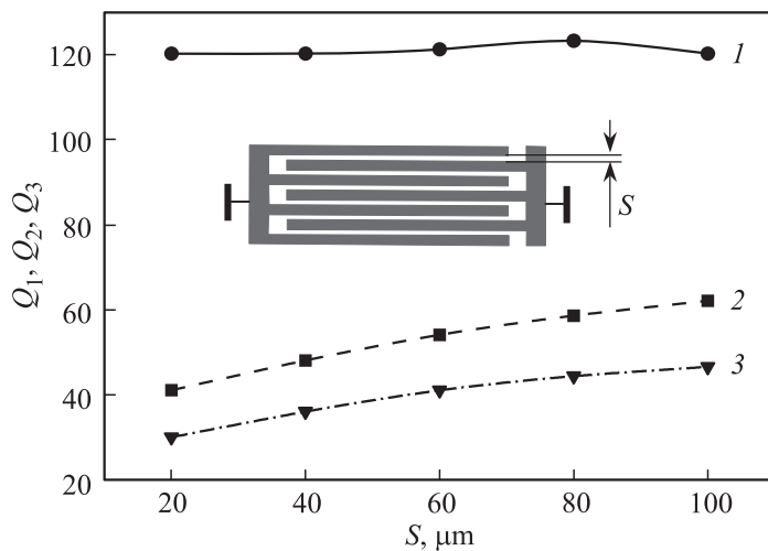
Рис. 2. Зависимости собственных добротностей первых трех мод колебаний многопроводного микрополоскового резонатора ( N = 7 ) от зазора между полосковыми проводниками встречно-штыревой структуры.
