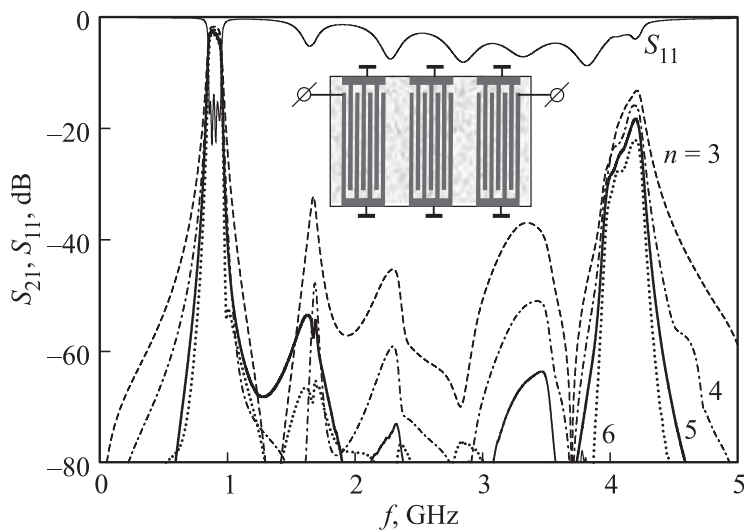
Рис. 1. АЧХ многорезонансных фильтров ( n = 3-6 ) на многопроводных микрополосковых резонаторах ( N = 7 ), полученные численным электродинамическим анализом 3D-моделей. На вставке конструкция фильтра третьего порядка.
