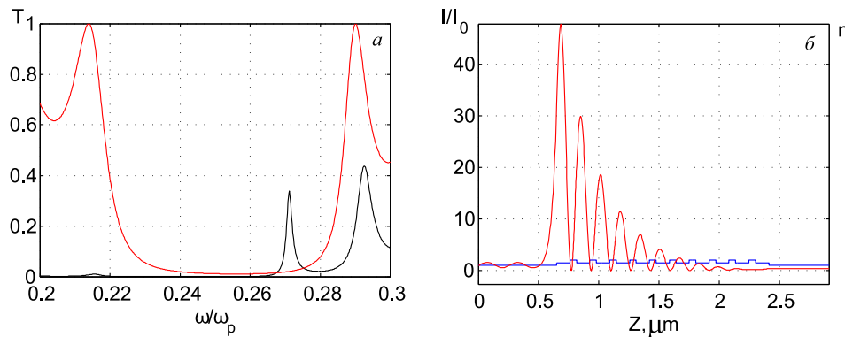
Рис. 3: Спектр пропускания при нормальном падении света на ПК (красная линия) и на ПК сопряженный со слоем НК (черная линия) с диспергированными вытянутыми наночастицами для волн -поляризации (а) и локализация поля на частоте таммовского состояния \omega = 0.2709\omega_p (б). Толщина слоя НК d_{mix} = 150 нм, фактор заполнения f = 0.3 , \xi = 10 , толщина слоя d_b = 55 нм и d_a = 110 нм. Остальные параметры такие же как для рис. 2.
