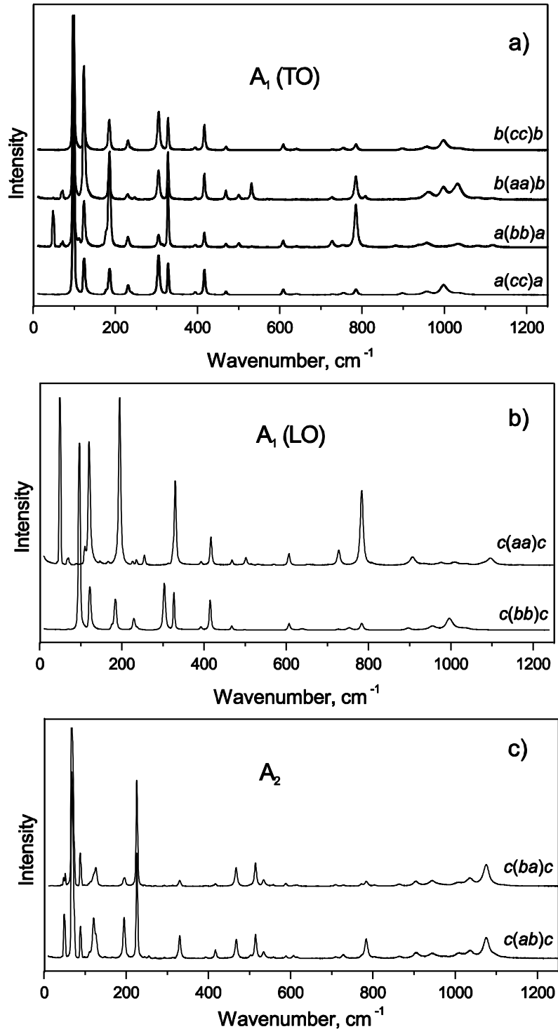
Figure 2. Raman spectra of the \delta - \text{BiB}_3\text{O}_6 crystal at: a) b(cc)b , b(aa)b , a(bb)a , a(cc)a b) c(aa)c , c(bb)c , c) c(ba)c , c(ab)c geometries
