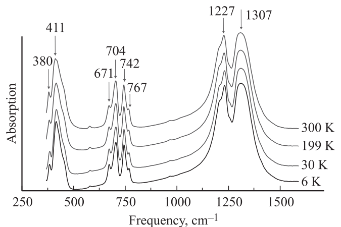
Рис. 1. Температурная трансформация спектров поглощения в диапазоне частот 375\text{--}1700\text{ cm}^{-1} .
