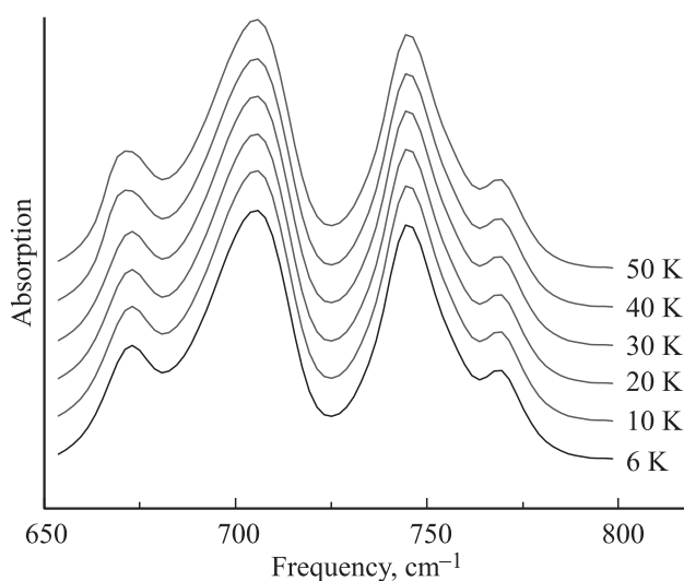
Рис. 3. Спектральная область 650–800\text{ cm}^{-1} .
