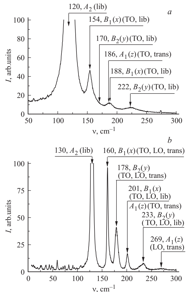
Рис. 3. Низкочастотный участок спектра КР нитрита натрия при комнатной температуре (а) и при T = 123 \text{ K} (б).
