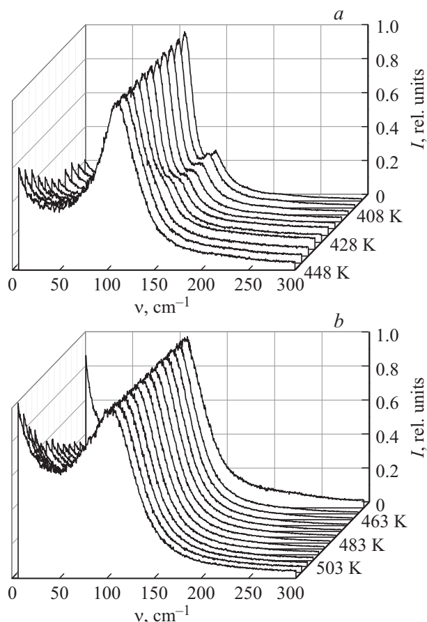
Рис. 5. Температурная зависимость низкочастотных спектров КР вблизи температуры сегнетоэлектрического фазового перехода: а — 398–448 К, б — 453–513 К.
