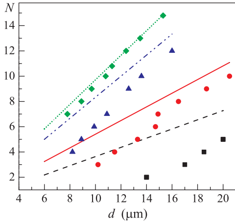
Рис. 2. (Цветной онлайн) Экспериментальные зависимости N(d) для концентраций C хиральной добавки 3.0% (■), 4.5% (●), 6.7% (▲) и 7.7% (◆). Линиями показаны зависимости N_0 = 2d/p_0 для концентраций 3.0% (---), 4.5% (—), 6.7% (· · · · ·) и 7.7% (· · · · ·)
