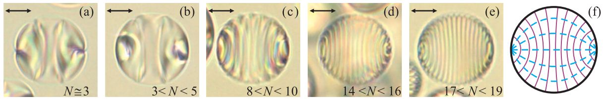
Рис. 1. (Цветной онлайн) Фотографии капель ХЖК, сделанные без анализатора, для концентраций C : 3.0% (a), (b); 4.5% (c); 6.7% (d); 7.7% (e). N – число интервалов между линиями оптической текстуры. Размер капель ХЖК 17 мкм (a), 18–19 мкм (b)–(e). (f) – Схематическое представление структуры с биполярным распределением оси ХЖК для N \approx 12 , расстояние между сплошными линиями соответствует половине шага спирали, штриховыми линиями показана ориентация оси геликоида в различных участках капли. Направление поляризатора показано двойными стрелками
