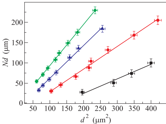
Рис. 3. (Цветной онлайн) Зависимости величин N \cdot d от d^2 для концентраций хиральной добавки 3.0% (■), 4.5% (●), 6.7% (▲) и 7.7% (◆) и линейные аппроксимации соответствующих экспериментальных данных
