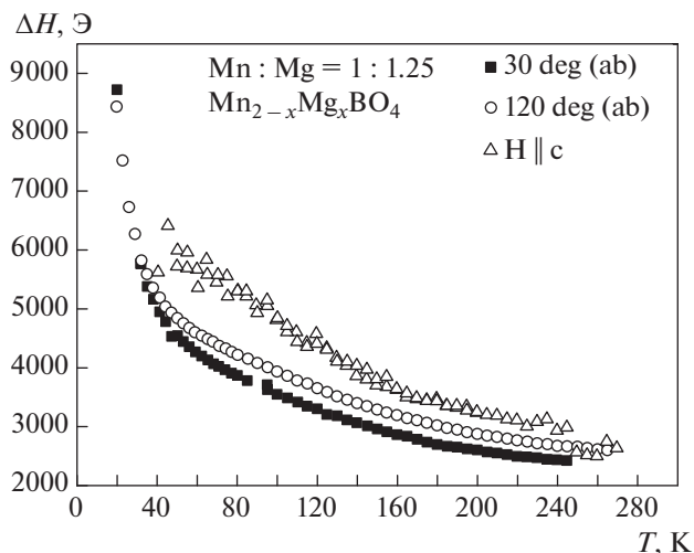
Рис. 3. Температурные зависимости ширины линии ЭПР в монокристалле \text{Mn}_{0.89}\text{Mg}_{1.11}\text{BO}_4 вдоль трех перпендикулярных направлений.
