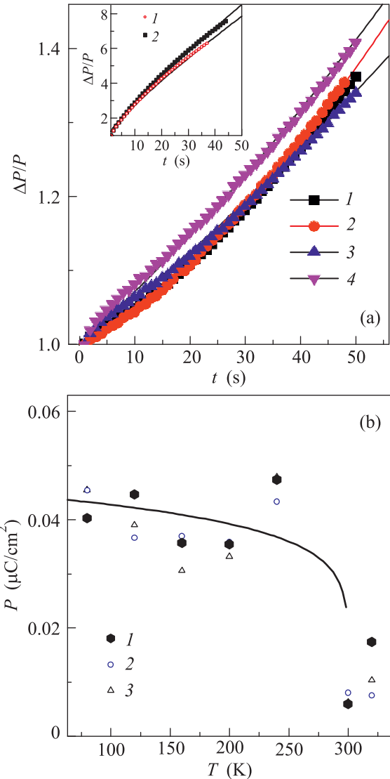
Рис. 2. (Цветной онлайн) Относительное изменение электрической поляризации вдоль пленки на подложке из граната от времени, после включения постоянного электрического поля E = 600 В/см при T = 80 К (1), 120 К (2), 160 К (3), 200 К (4). На вставке \Delta P/P при T = 360 К, H = 0 кЭ (1), H^z = 12 кЭ (2) (а). Остаточная поляризация при t = 200 с в магнитных полях H = 0 кЭ (1), H^z = 12 кЭ (2), H^x = 12 кЭ (3) от температуры (б)
