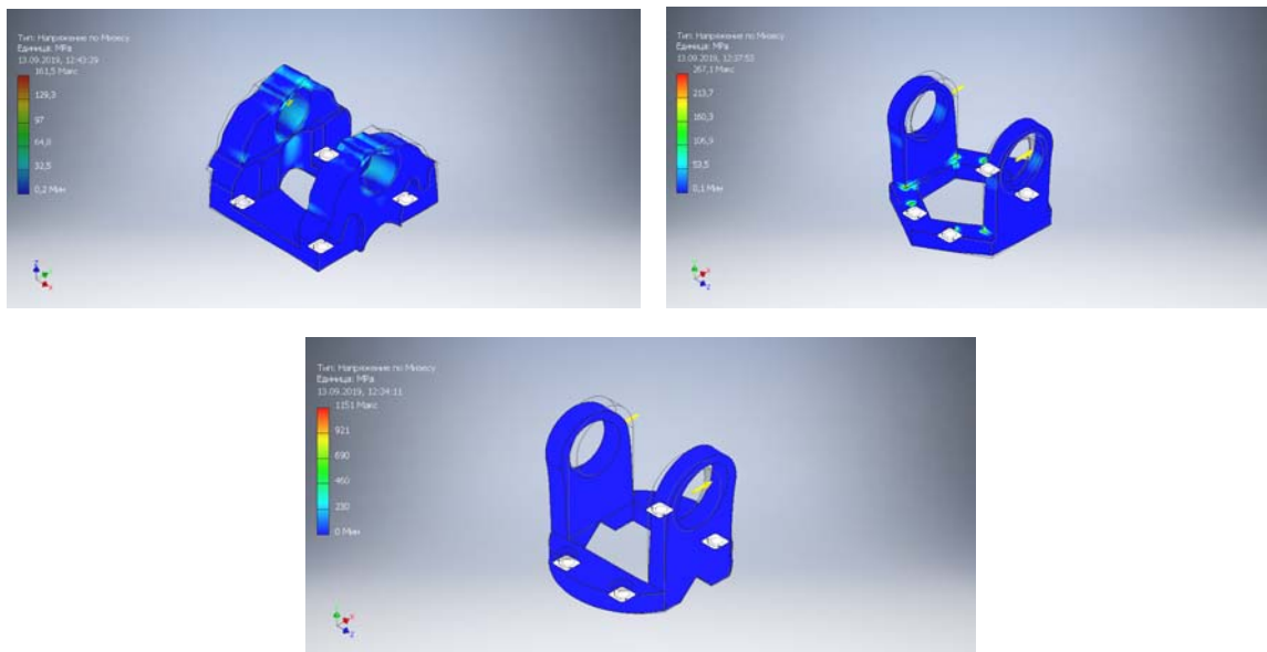
Рис. 2. Конечно-элементный анализ вилок карданных передач
