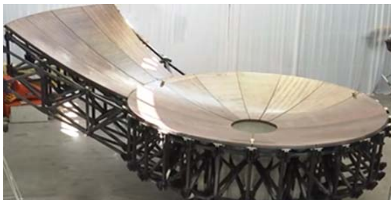
Рефлектор из полимерных композитов
