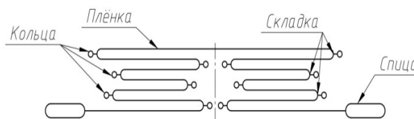
Рис. 3. Схема образования складок
