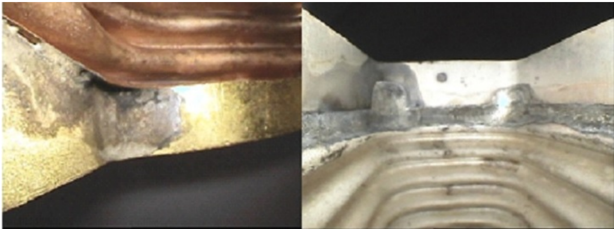
Рис. 1. Дефекты паяного соединения – непроай и наплывы
