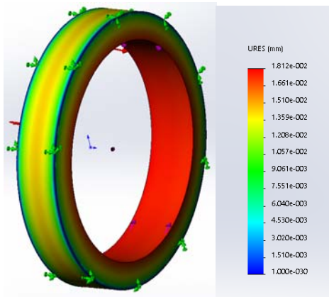
Рис. 3. Результат статического анализа на перемещение нейлонового кольца
