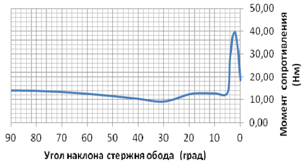
Рис. 1. График изменения момента сопротивления
