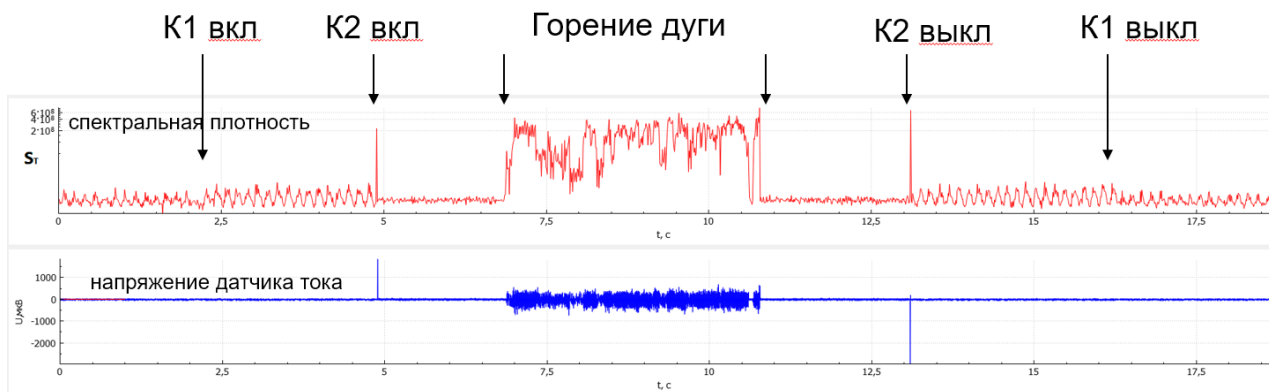
Рис. 3. Результаты экспериментального определения дугообразования
