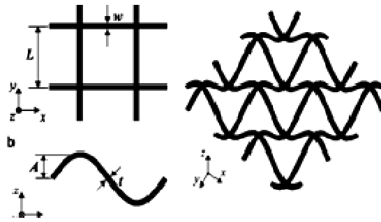
Рис. 1. Структурная схема модели ауксетичного материала
