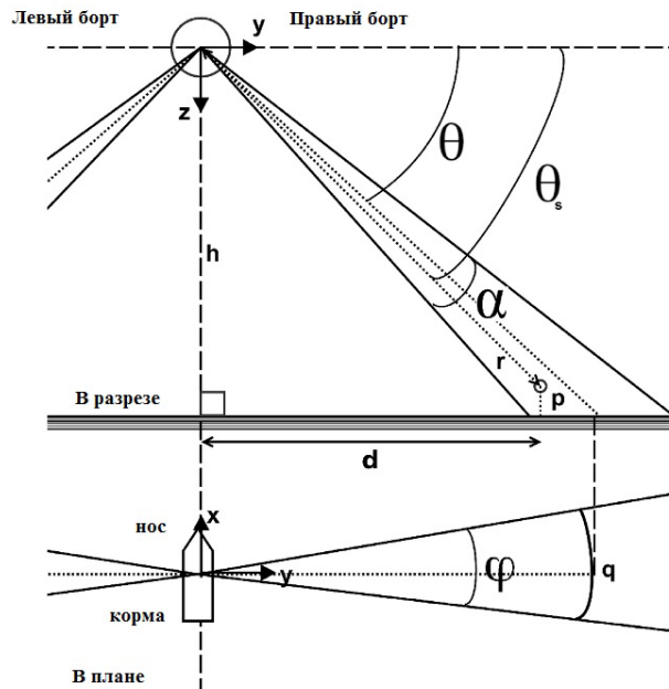
Рис. 1. Принцип работы гидролокатора бокового обзора: h – глубина от трансьюера до дна; \theta – угол луча относительно условного горизонта водоема; \alpha , \phi – углы луча трансьюера; точка p определяется на удалении r по дуге q и выражается парой координат xy [2]
