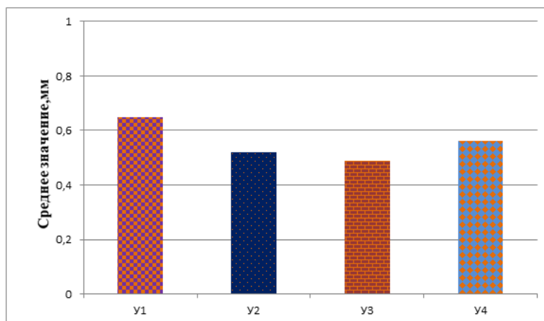
Среднее значение размера зерна макроструктур сплава АК12 в зависимости от технологии плавки
