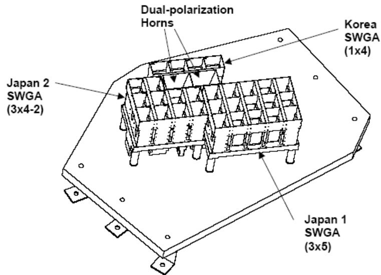
Рис. 1. Многолучевая решетка
