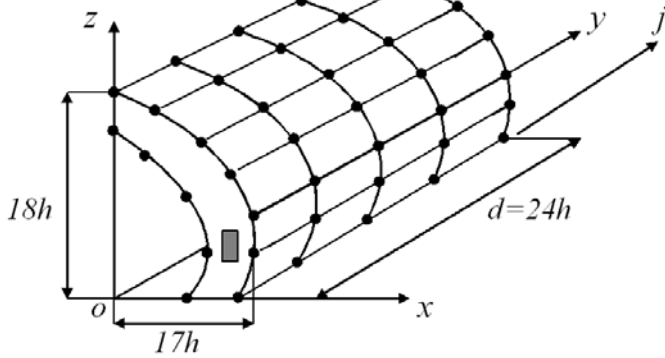
Рис. 1. Двухсеточный КЭ V_d^a
