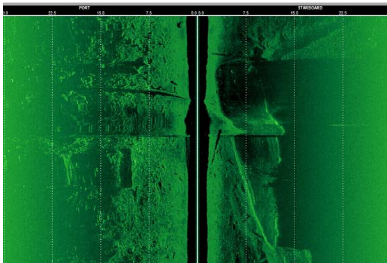
Рис. 3. Пример гидроакустического снимка с резким волнообразным искажением донного объекта (затонувшего судна). Причина – резкий подъем буксируемого модуля с целью предотвращения его зацепления за донный объект
