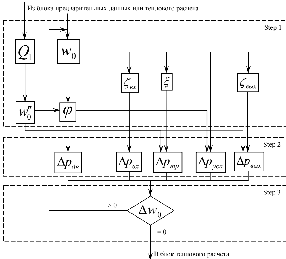
Схема расчетной последовательности гидравлического блока
