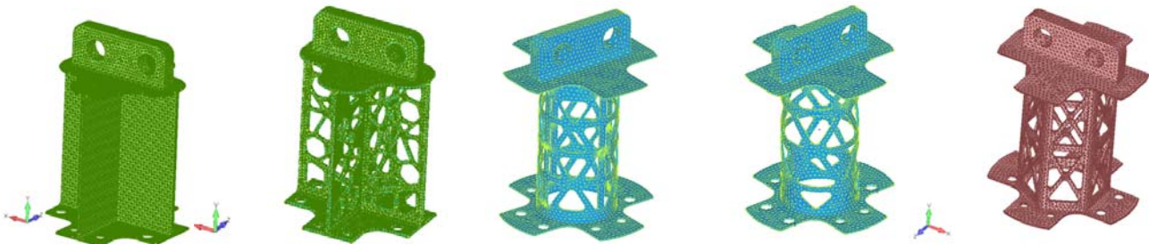
Рис. 3. Конечноэлементные модели вариантов стойки
