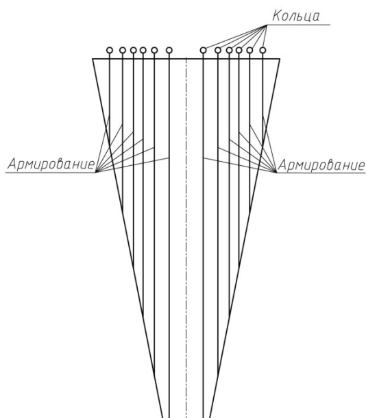
Рис. 4. Схема армирования пленки
