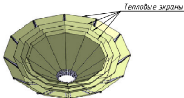
Рис. 1. Система пассивного охлаждения космического телескопа «Миллиметрон»
