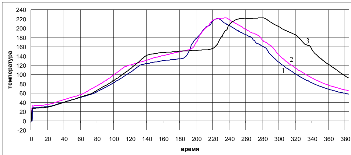
Рис. 1. Термопрофили оплавления паяльной пасты
