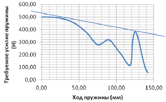
Рис. 2. Требуемое усилие в КПМ и характеристика пружины сжатия
