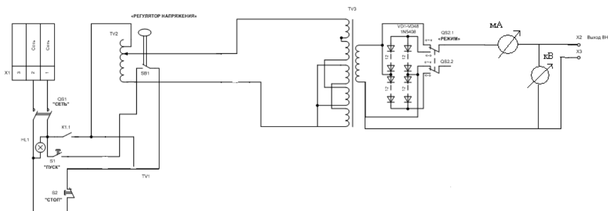
Структурная схема пробойной установки УПУ-6
