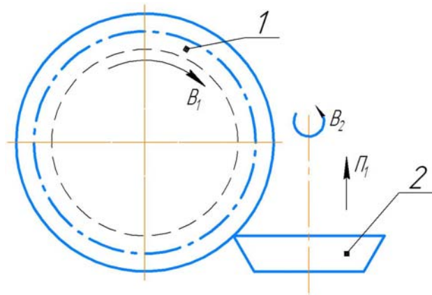
Схема распределения элементарных движений 1 – заготовка глобоидного червяка; 2 – многолезвийный инструмент; B_1 – движение червяка в форме вращения; B_2 – движением инструмента в форме вращения; \Pi_1 – поступательное движение инструмента (вертикальная подача)
