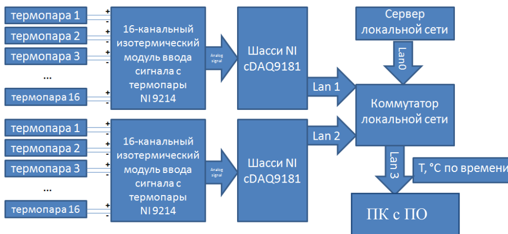
Рис. 2. Автоматизированная система фиксации данных на основе контролеров National Instruments
