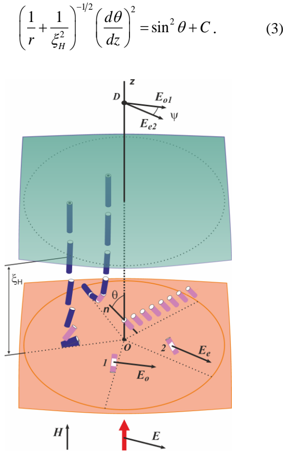
Рис. 1. Ориентационная структура домена HANL в магнитном поле H . Лазерный луч направлен вдоль оси z . Линия дисклиниции на схеме не показана
