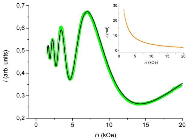
Рис. 4. Интенсивность света I в зависимости от магнитного поля H : экспериментальная (зеленая линия) и теоретическая (черная сплошная линия). Разность фаз \delta в зависимости от H приведена на вставке
