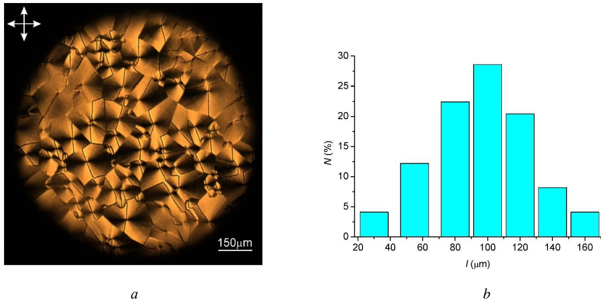
Рис. 3. Фрагмент HANL, ограниченный диафрагмой диаметром 1 мм; направления скрещенных поляризаторов показаны стрелками (а). Статистическое распределение длин линий дисклинаций в HANL (b)
