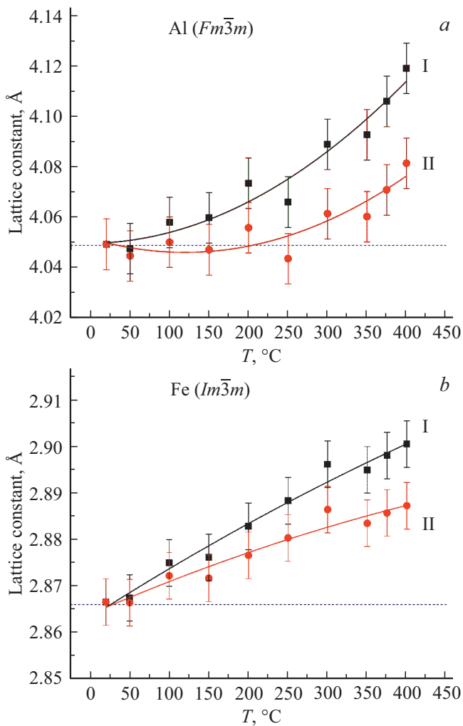
Рис. 3. Изменение параметра решетки алюминия (а) и железа (б) в процессе нагрева тонкопленочной наносистемы Al/Fe до 400°C (кривые I — без учета ТКЛР, кривые II — с учетом ТКЛР).
