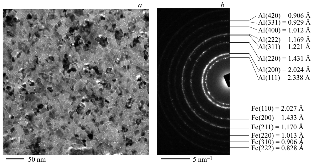
Рис. 1. Электронно-микроскопическое изображение (а) и картина дифракции электронов (б), полученные от тонкопленочной наносистемы Al/Fe в исходном состоянии.
