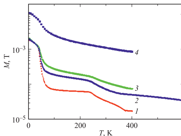
Рис. 3. Температурные зависимости намагниченности компонента \text{DyMn}_2\text{O}_5\text{-Mn}_3\text{O}_4 . H = 1 - 0.04, 2 - 0.4, 3 - 0.8, 4 - 4 MA/m.
