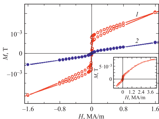
Рис. 4. Полевые зависимости намагниченности: 1, 2 — T = 20, 70 К. На вставке приведена петля намагниченности при T = 4.2 К, полученная до полей H = 4 MA/m.
