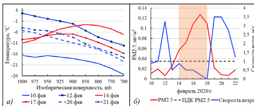
Рис. 1. Метеорологические условия в Красноярске в феврале 2020 г. а) – температуры воздуха на изобарических поверхностях; б) – концентрации PM 2.5 и скорости ветра, оранжевым цветом выделен период НМУ.
