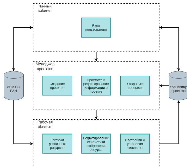
Рис. 1. Модульная система веб-приложения для быстрой развертки веб-ГИС
