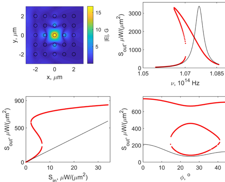
Рис. 1. а) Резонансная мода на линейном дефекте в центре массива с \epsilon=11,56 , \epsilon_{def}=3 , радиус цилиндров r=0.18 \mu\text{m} , \nu = 1,077 \cdot 10^{14} \text{ Hz} ; б) отклик по частоте для ФК из (а), черная кривая для дефекта с линейным по полю \epsilon , красная для дефекта с постоянной Керра n_2=1.81 \cdot 10^{-11} \text{ cm}^2/\text{W}^2 ( S_{in}=12 \mu\text{W} , \phi=0 ); в) и г) отклик по интенсивности внешнего поля ( \nu=1,068 \cdot 10^{14} \text{ Hz} , \phi=0 ) и углу падения ( \nu=1,068 \cdot 10^{14} \text{ Hz} , S_{in}=12 \mu\text{W} ) соответственно, черным цветом – линейный случай, красным - n_2=8.47 \cdot 10^{-11} \text{ cm}^2/\text{W}^2 .
