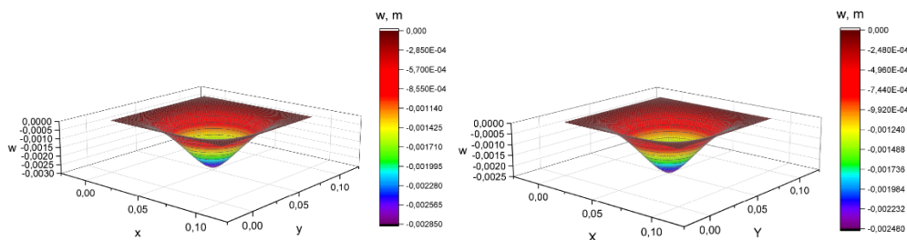
Рис. 1. Изгиб однослойной композитной пластинки под действием поперечной нагрузки.
