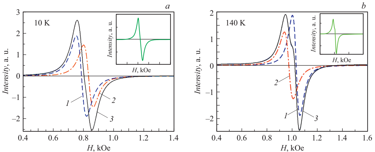
Рис. 1. Подгоночная кривая (линия 3) экспериментальных СВЧ-спектров для пленки с толщиной Dy t_{Dy} = 5 nm, измеренных при 10 (a) и 140 K (b). 1 и 2 — акустическая и оптическая мода соответственно. На вставках представлены экспериментальные кривые.
