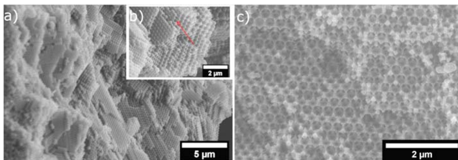
Рис. 1. Электронная микрофотография: a – темплата из ПММА; b – пропитанного образца; c – инверсного опала
