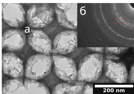
Рис. 5. ПЭМ изображения:
