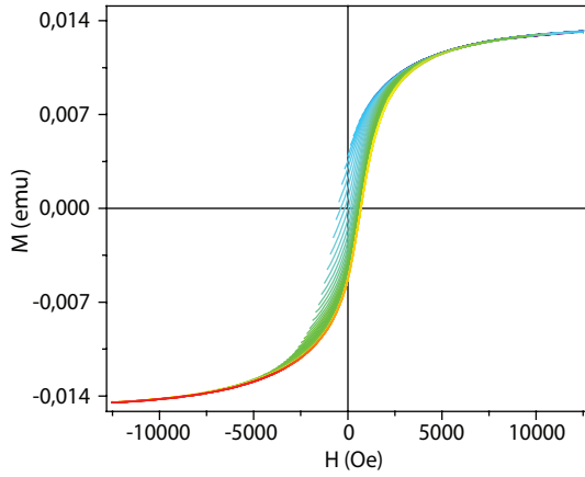
BTO/ZCFO/PVDF-TrFE
