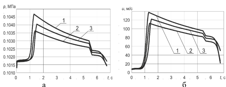
Рис. 2. Зависимость изменения давления (а) и скорости истечения (б) продуктов горения через выходное сечение канала от времени: 1 – прямоугольный канал (рис. 1, а); 2 – прямоугольный канал (рис. 1, б); 3 – треугольный канал (рис. 1, в)
