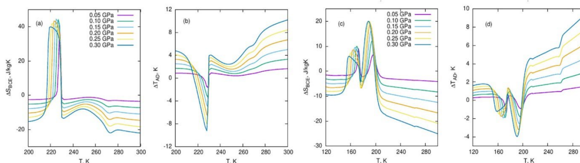
Рис. 1. Температурные зависимости экстенсивного (а, с) и интенсивного (b, d) БКЭ в (NH 4 ) 3 GeF 7 (а, b) и (NH 4 ) 3 SiF 7 (с, d)
