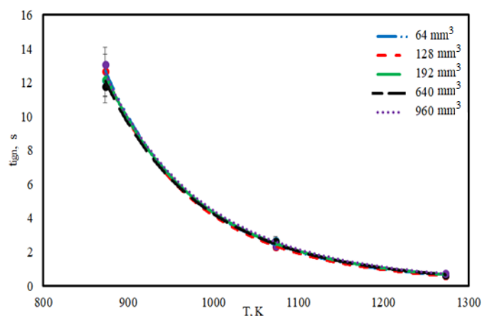
Рис. 1. Зависимости времени задержки зажигания частицы древесной биомассы в форме куба от температуры внешней среды при различных характерных размерах
