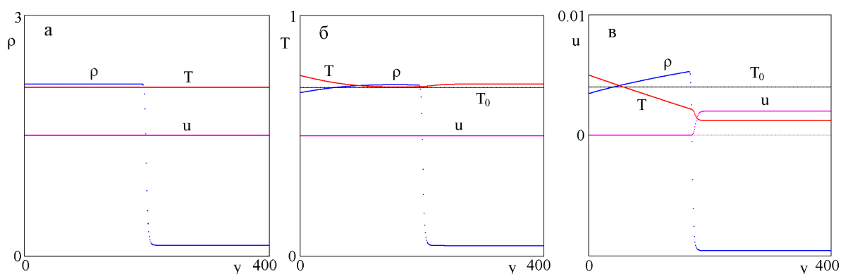
Рис. 1. Моделирование: а – начальное состояние, T_0 = 0.7T_{кр} , u = 0 ; б – включены нагрев подложки \Delta T = 0.05T_{кр} и теплопроводность жидкости; в – квазистационарный режим течения при оттоке пара на границе u_0 = 0.002 . Температура и плотность даны в приведенных переменных
