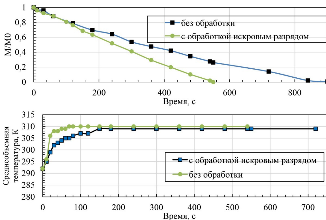
Рис. 2. Кривая изменения массы капли воды и среднеобъемной температуры, подвешенной капли воды при обтекании слаботочным плазменным каналом искрового разряда и без
