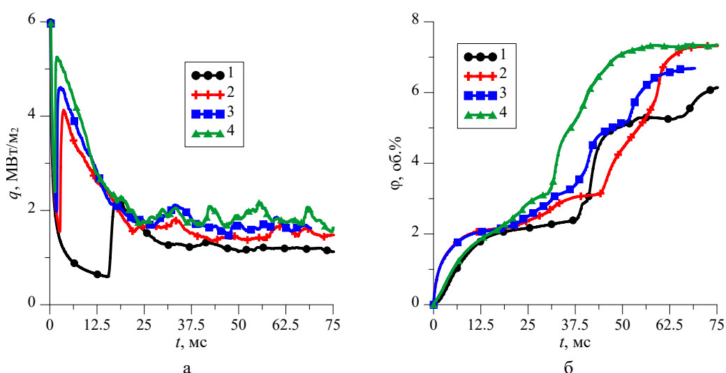
Рис. 1. Зависимость от времени плотности теплового потока на нагревателе (а) и объёмной концентрации пара (б) при различной t_{II} : 1 – 105°C; 2 – 115°C; 3 – 120°C; 4 – 126°C. Re_l = 33,2 , Re_g = 912,8
