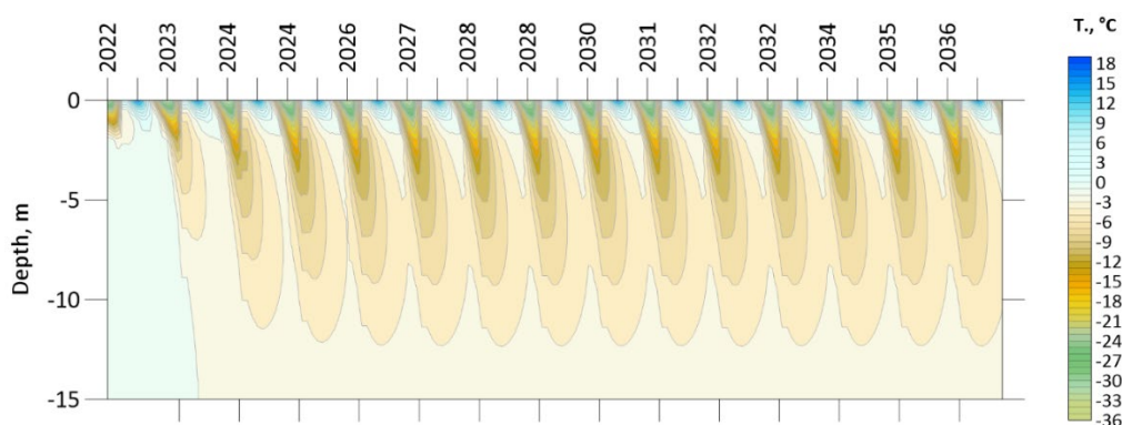
Рис. 2. Динамика температуры грунтов варианта 1 по II сценарию
