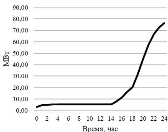
Рис. 2. Пиковые мощности во время зарядки электрокаров, МВт
