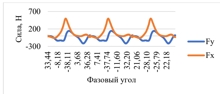
Рис. 2. График обобщенной силы, действующей на лопасть
