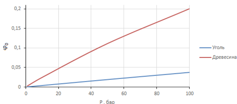
Рис. 1. Зависимость объемной плотности твердых частиц от давления
