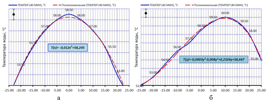
Рис. 2. Экспериментально определённые распределения температуры воды в поперечном сечении РПН \varnothing 51 мм на 40-й минуте остывания: a – горизонтальное сечение гидростолба; б – вертикальное сечение гидростолба
