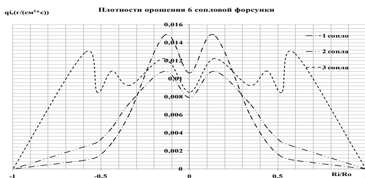
Рис. 1. Изменение плотности орошения по сечению факела жидкости при увеличении количества шнеков
