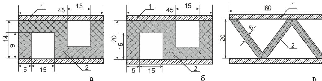
Рис. 1. Геометрические конфигурации и размеры элементов ГО, включающих обшивку из органопластика 1 и твердое топливо 2: а – прямоугольный канал 15 \times 9 мм; б – прямоугольный канал 15 \times 15 мм; в – треугольный канал высотой 20 мм
