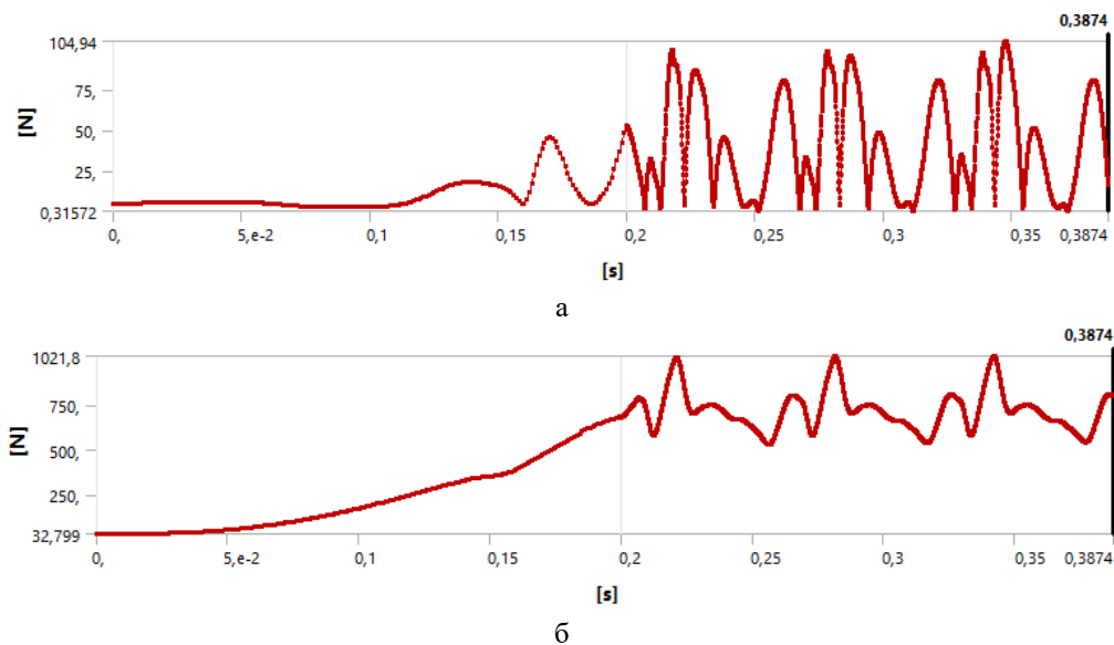
Рис. 4. Графики реакций для одной лопасти при скорости набегающего потока 50 м/с: а – в управляющей тяге; б – в оси крепления лопасти
