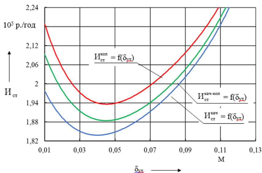
Рис.1. Зависимости I_{ст}^{кач} , I_{ст}^{кач-кол} и I_{ст}^{кол} от \delta_{ут} : I_{ст}^{кач} – затраты по утеплению наружных ограждающих конструкций стен здания при качественном регулировании отпускаемой тепловой энергии, р./год; I_{ст}^{кач-кол} – затраты по утеплению наружных ограждающих конструкций стен здания при качественно-количественном регулировании отпускаемой тепловой энергии, р./год; I_{ст}^{кол} – затраты по утеплению наружных ограждающих конструкций стен при количественном регулировании отпускаемой тепловой энергии, р./год
