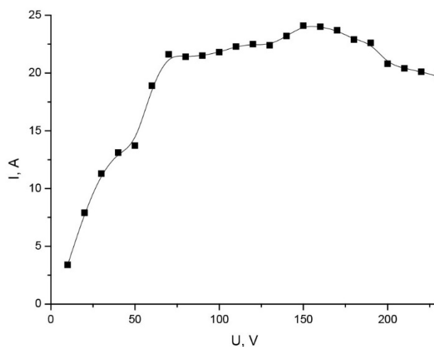
Рис. 1. ВАХ плазменно-электролитного хромирования
