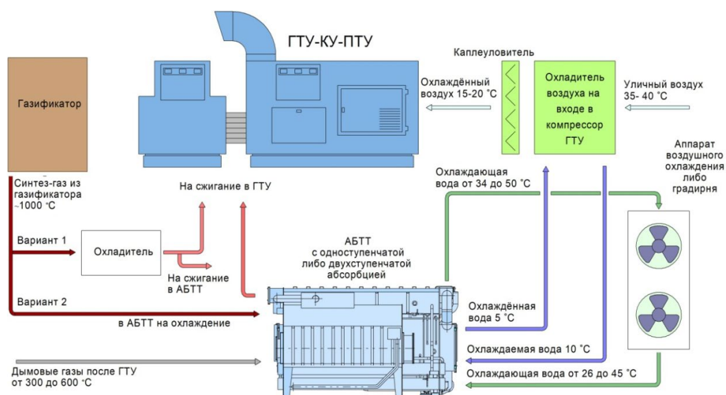
Рис. 1. Схема охлаждения воздуха на входе ГТУ с помощью АБТТ, установленного на ПГУ-ВЦГ
