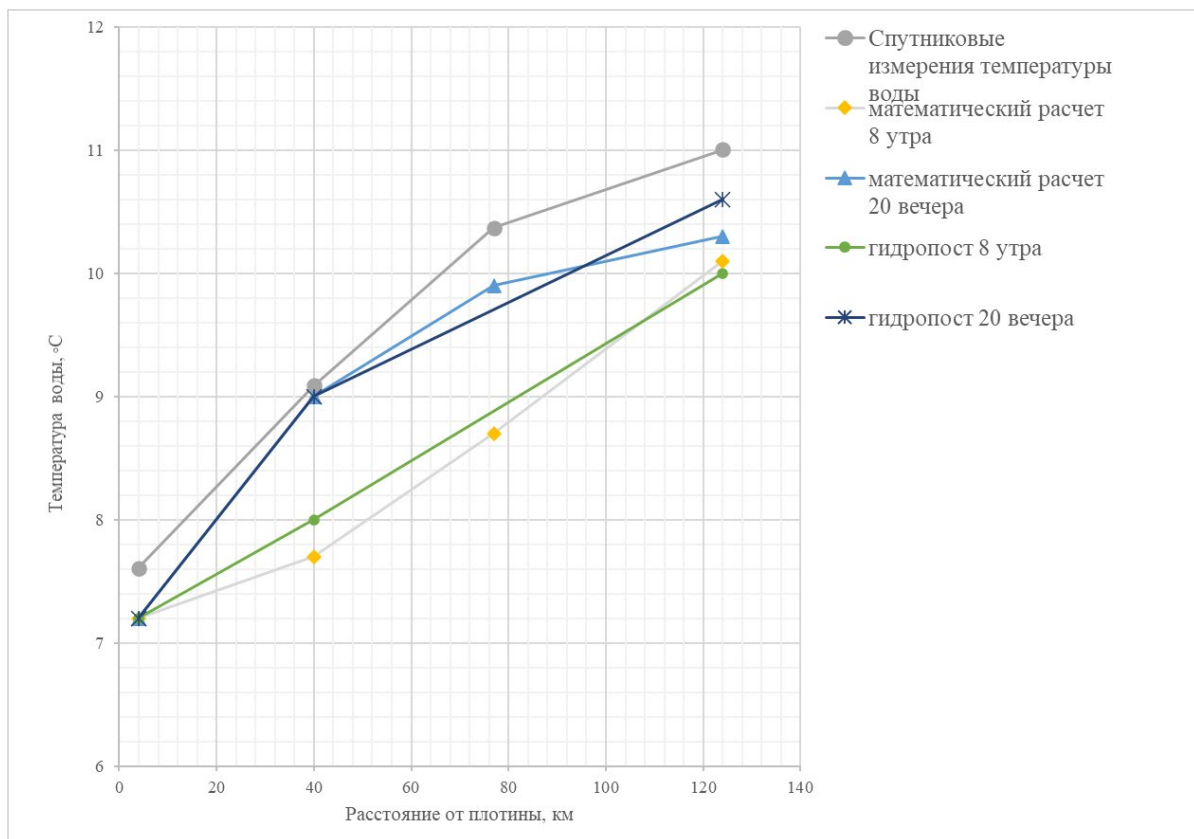
Рис. 1. Температура воды в нижнем бьефе Красноярской ГЭС, полученная разными способами
