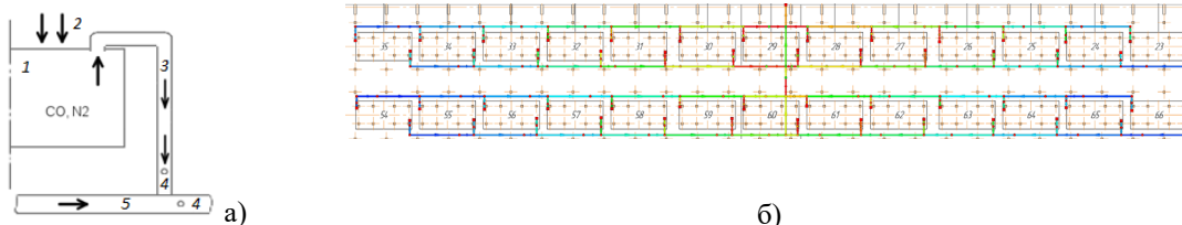
Рис. 1. Система газоходов электролизного производства: а) подключение электролизера; 1 – электролизер; 2 – присосы воздуха; 3 – спуск; 4 – точки замера расхода; 5 – сборный газоход; б) сеть
