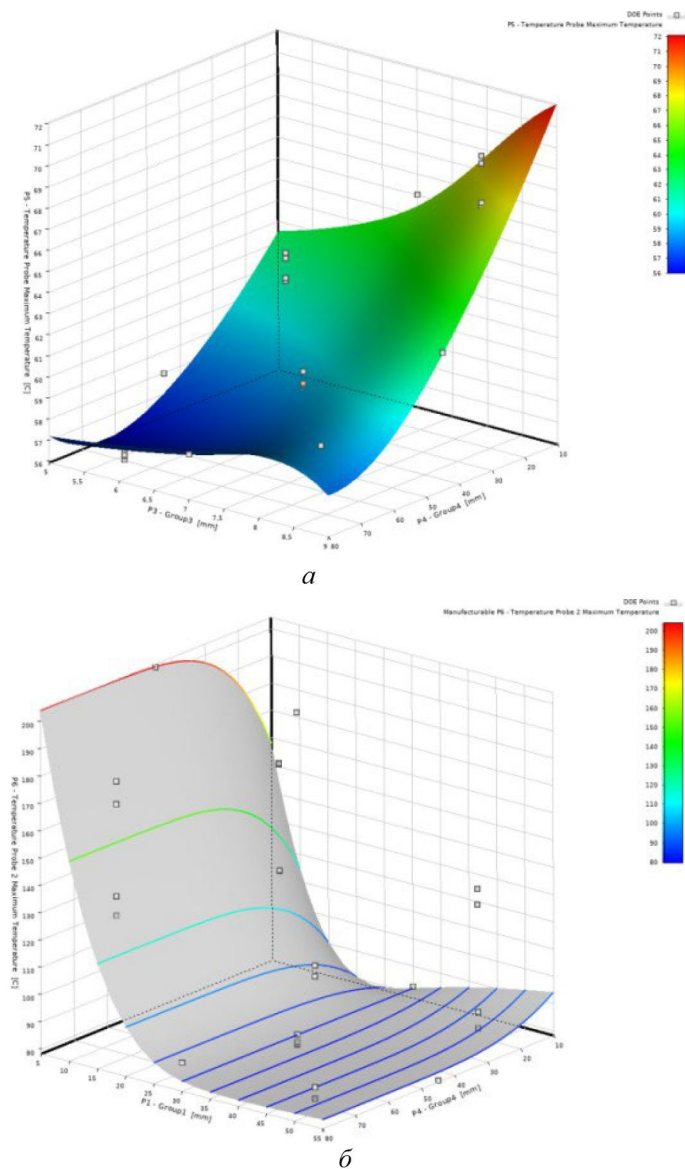
Рис. 2. Поверхности отклика по трем параметрам: а – температура резисторов от толщины основания несущей конструкции и расположения ГТПС; б – температура МС в зависимости от её перемещения по поверхности ПП и перемещения ГТПС
