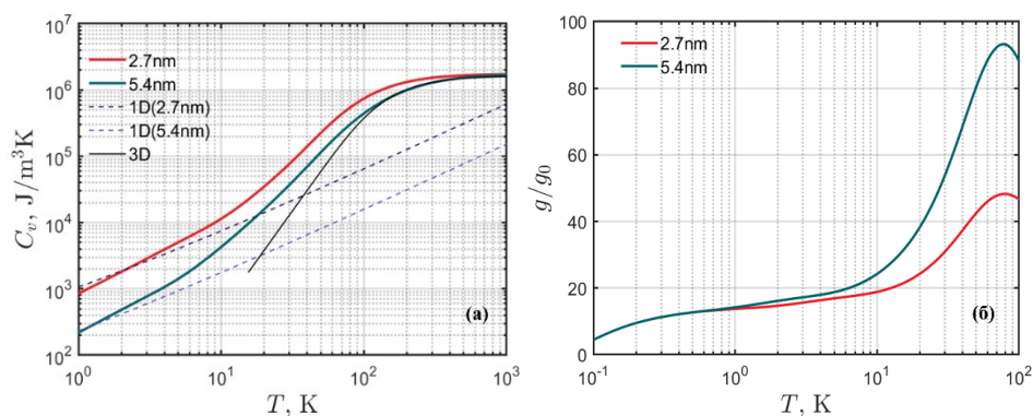
Рис. 2. Теплоемкость (а) и баллистическая теплопроводность (б) нанонитей. Линии – результаты расчета авторов для диаметров 2,7 и 5,4 нм; 1D, 3D – модель Дебая [3].
