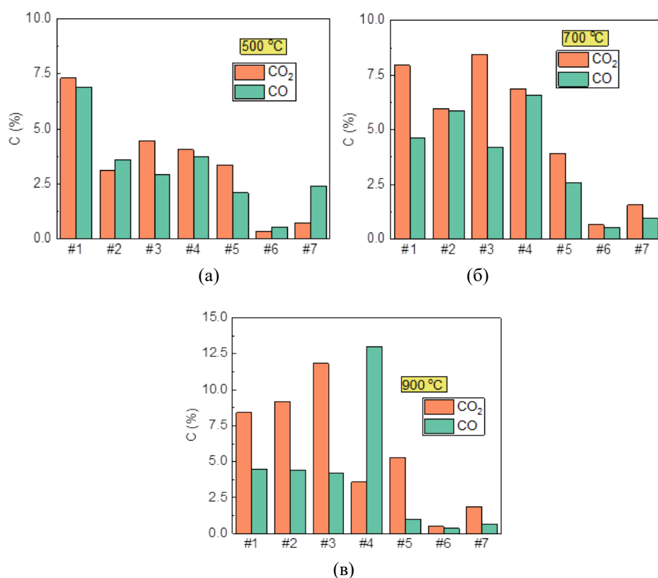
Рис. 2. Концентрации оксидов углерода в зависимости от температуры окислителя: а – 500\text{ }^\circ\text{C} ; б – 700\text{ }^\circ\text{C} ; в – 900\text{ }^\circ\text{C} (#1 древесина, #2 линолеум, #3 ПВХ, #4 полипропилен, #5 стекломagnesитовый лист, #6 минеральная вата, #7 гипсокартон)
