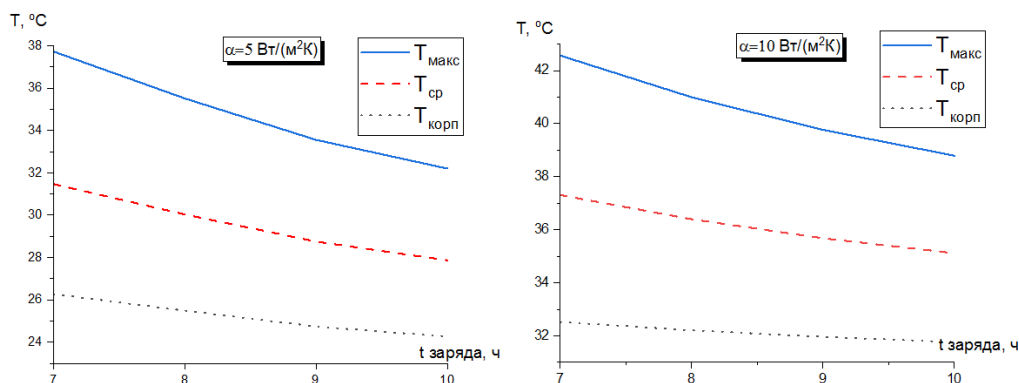
Рис. 2. Характерные температуры элемента свинцово-кислотной батареи при T_{\text{окр}} = 20\text{ }^{\circ}\text{C}
