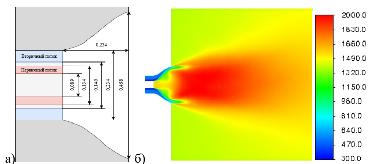
Рис. 1. Схема горелочного устройства (а), размеры указаны в миллиметрах; распределение температуры (б) в пылеугольном факеле при кислородном сжигании (К)
