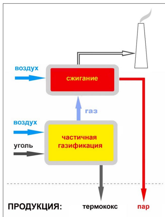
Рис. 1. Принципиальная схема технологии «ТЕРМОКОКС»
