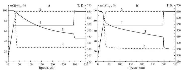
Рис. 1. Изменение температуры (1, 2) и относительной массы образца (3, 4) для двух режимов нагрева: a – расчет, b – эксперимент
