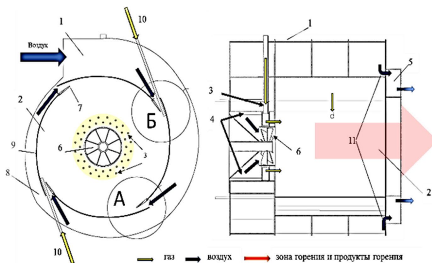
1 – распределительный короб; 2 – камера сгорания; 3 – осевой ввод газа; 4 – торцевая вихревая камера; 5 – пережим; 6 – завихритель; 7 – сопла тангенциального ввода воздуха; 8 – «улитка»; 9 – стенки камеры сгорания; 10 – тангенциальный ввод газа; 11 – переток воздуха в пережим Рис. 2. Схема лабораторной модели ЦВП. Поперечный (слева) и продольный (справа) разрезы
