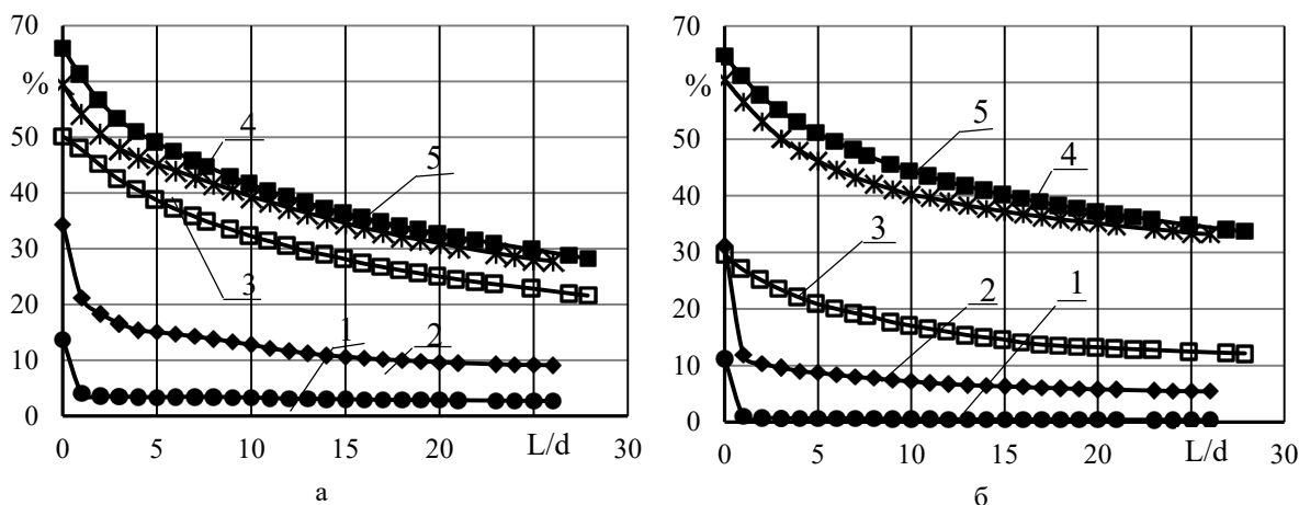
Рис. 1. Изменение концентрации охладителя по поверхности: а) при m = 1 ; б) при m = 2 : 1 – цилиндрическое отверстие; 2 – веерное отверстие с коротким диффузорным участком; 3 – laidback отверстие с коротким диффузорным участком; 4 – веерное отверстие с длинным диффузорным участком; 5 – комбинированное отверстие
