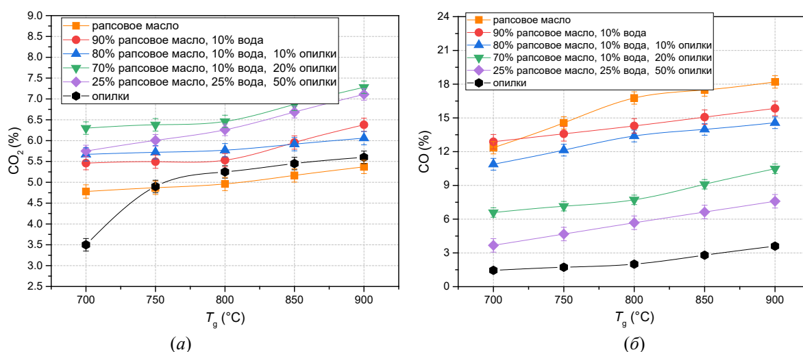
Рис. 2. Концентрации оксидов углерода в зависимости от температуры в камере сгорания
