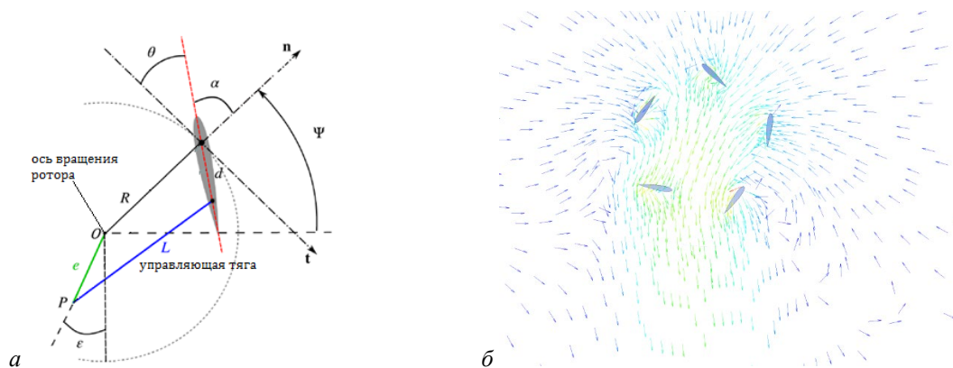
Рис. 2. Циклический ротор: a – кинематическая схема движения лопасти циклического движителя; б – пример течения, индуцируемого циклическим ротором (численное моделирование)
