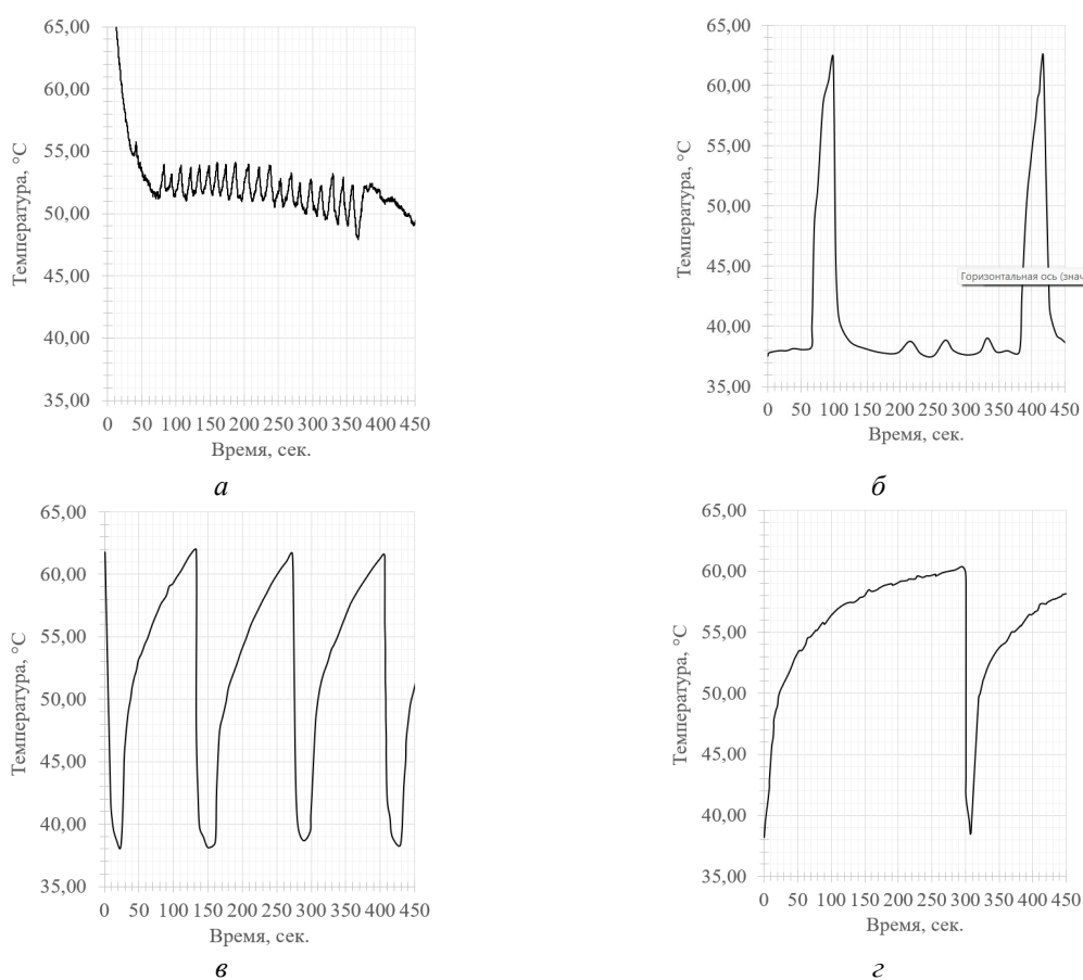
Рис. 2. Фрагмент колебания температуры стенки поверхности при следующих значениях теплового потока: а – данные, полученные авторами статьи; б – q = 23 \text{ Вт/см}^2 ; в – q = 12,2 \text{ Вт/см}^2 ; г – q = 9,4 \text{ Вт/см}^2 [0]
