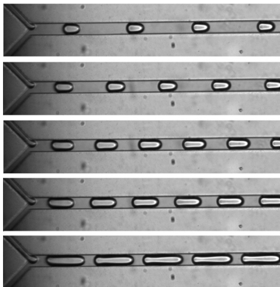
Рис. 1. Снарядный режим течения при фиксированном расходе нефти Q_o = 1,7 \cdot 10^{-11} \text{ м}^3/\text{с} и варьируемом расходе воды (сверху вниз) Q_w = 8,3 \cdot 10^{-12} \text{ м}^3/\text{с} ; Q_w = 1 \cdot 10^{-11} \text{ м}^3/\text{с} ; Q_w = 1,3 \cdot 10^{-11} \text{ м}^3/\text{с} ; Q_w = 1,7 \cdot 10^{-11} \text{ м}^3/\text{с} ; Q_w = 3,3 \cdot 10^{-11} \text{ м}^3/\text{с} .
