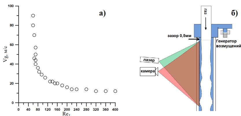
Рис. 1. Граница перехода к уносу для воды (а); схема работы ЛИФ-метода (б)
