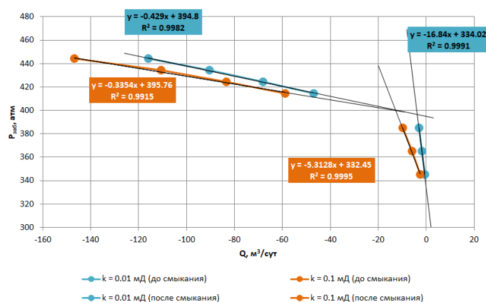
Рис. 2. Зависимости расхода закачиваемой жидкости от давления закачки в скважине при различных проницаемостях пласта 0.01 \cdot 10^{-15} и 0.1 \cdot 10^{-15} \text{ м}^2
