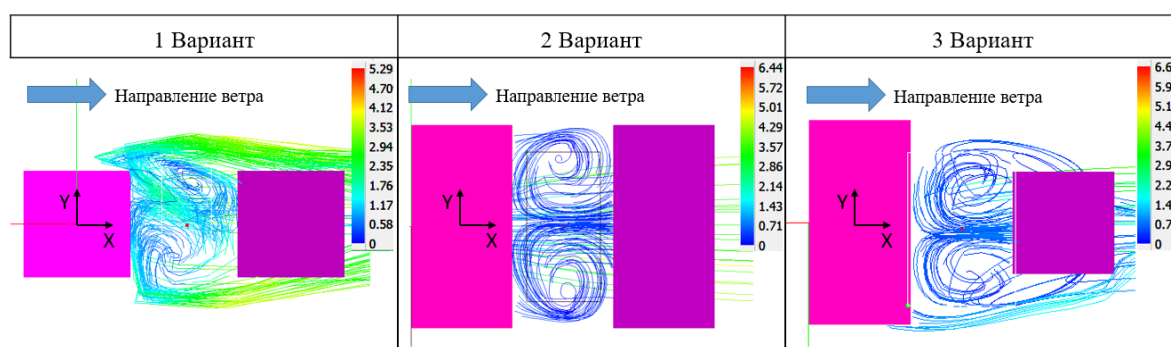
Рис.1. Образовавшиеся вихревые структуры между зданиями, отрисовка треками
