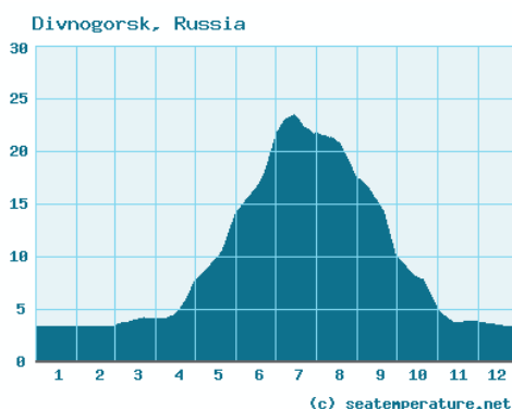
Рис. 1. Годовой график средней температуры воды реки Енисей вблизи Дивногорска [2]
