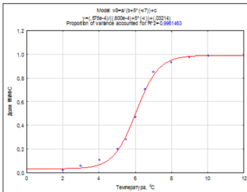
Рис. 2. Зависимость относительной доли модельного МИФС в исследуемой конструкции в зависимости от принятой температуры фазового перехода
