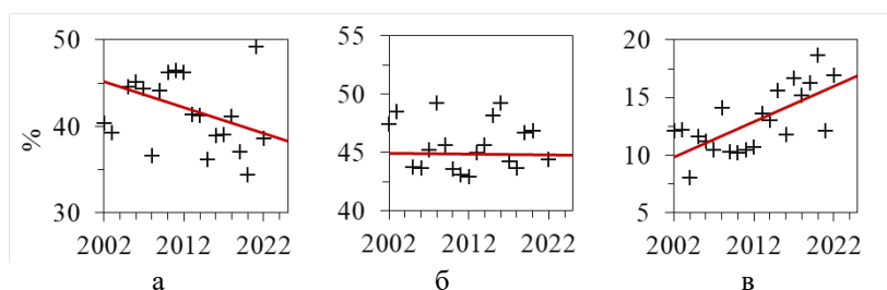
Рис. 1. Многолетние тренды площадей пожаров в Сибири с учётом интенсивности горения по мощности теплоизлучения (FRP): а – низкоинтенсивные; б – средней интенсивности; в – высокоинтенсивные
