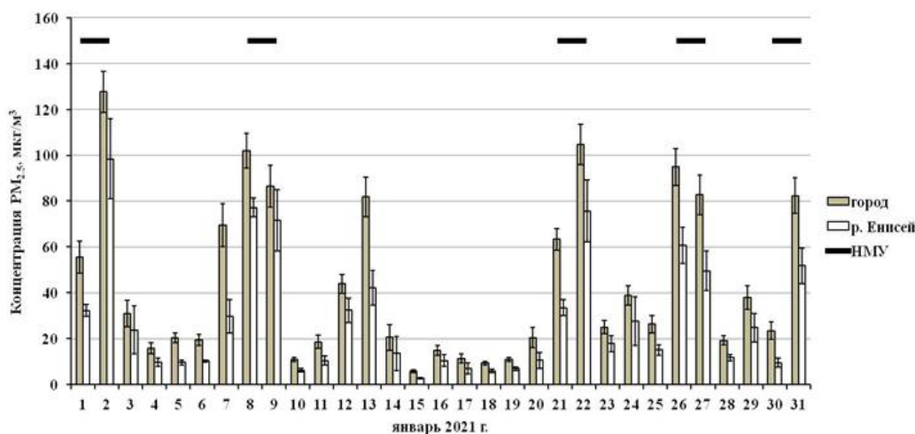
Рис. 1. Среднесуточные концентрации PM 2,5 в приземной атмосфере над рекой Енисей и прилегающей к ней территории города Красноярска в январе 2021 г. Черные горизонтальные линии обозначают периоды НМУ
