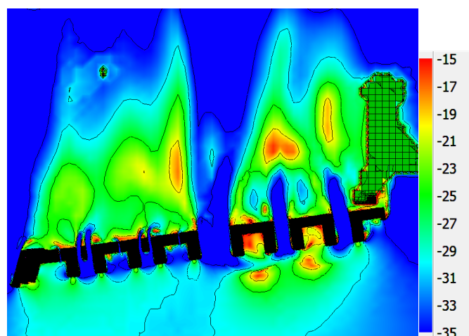
Рис. 1. Поле ЭЭТ на высоте 2 м
