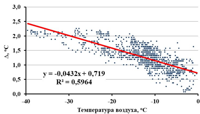
Рис. 1. Разность температуры воды у плотины ГЭС и в центре Красноярска в зависимость от температуры воздушной среды над поверхностью реки зимой 2022/2023
