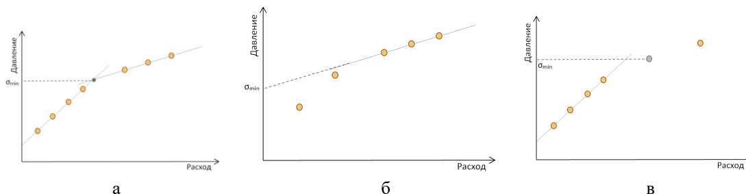
Рис. 1. Способы определения давления смыкания трещины автоГРП
