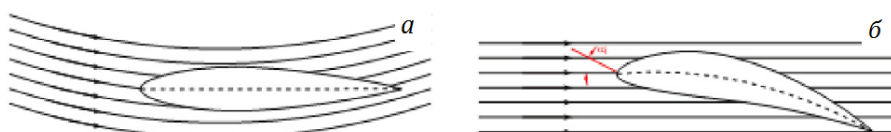
Рис. 1. Обтекание крылового профиля при вращательном движении: a – симметричный профиль при вращательном движении; б – аналогия, криволинейный профиль в прямолинейном потоке
