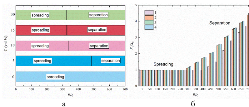
Рис. 1. Связь режимов соударения капли с твердой поверхностью при варьируемой концентрации воды в топливе ( T_f=80 °C) и числе Вебера (а); отношение площадей свободной поверхности после и до взаимодействия (б): 1 – 94,5 % мазута, 5 % воды, 0,5 % Tween 80; 2 – 89,5 % мазута, 10 % воды, 0,5 % Tween 80; 3 – 84,5 % мазута, 15 % воды, 0,5 % Tween 80; 4 – 69,5 % мазута, 30 % воды, 0,5 % Tween 80.
