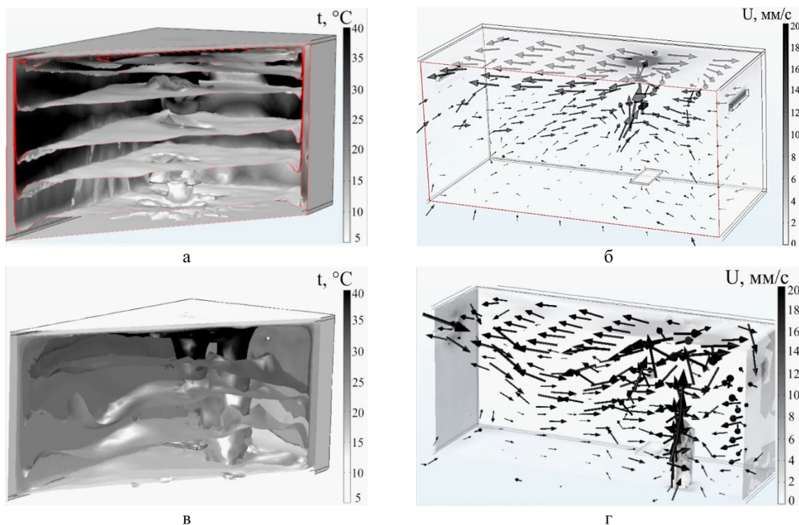
Рис. 2. Температурные поля (а, в) и векторы скорости (б, г) в помещении после одного часа работы ГИИ: без учёта (а, б) и с учётом (в, г) фигуры работающего
