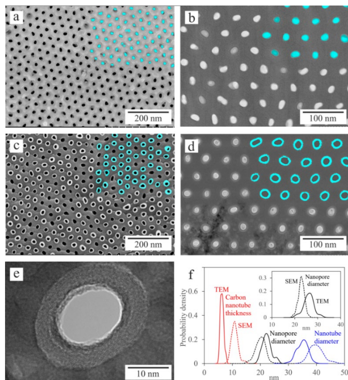
Рис. 1. РЭМ (a, c) и ПЭМ (b, d) изображения поперечного сечения мембраны ПАК до осаждения углерода (a, b) и после осаждения углерода (c, d). ПЭМ-изображение одной нанопоры с углеродной нанотрубкой (e). Распределение диаметра нанотрубок, диаметра нанопор и толщины нанотрубок (f). Результаты для мембран до осаждения углерода (вставка)
