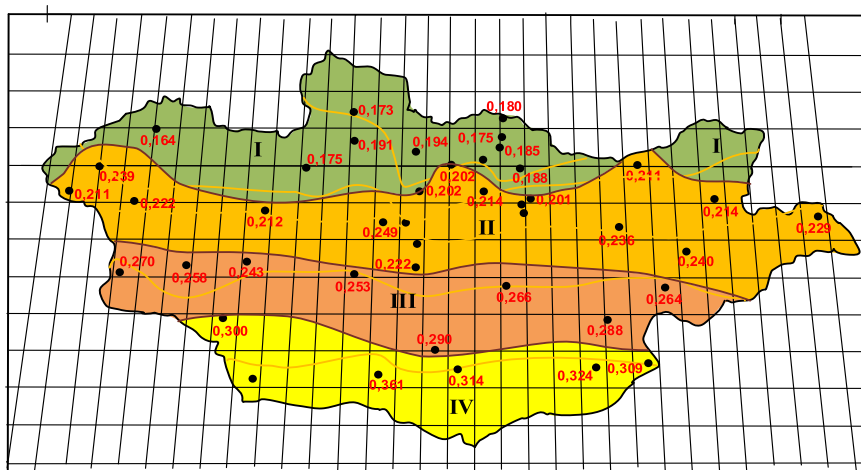
Рис. 1. Зонирование территории Монголии по эффективности использования солнечной энергии для обогрева зданий
