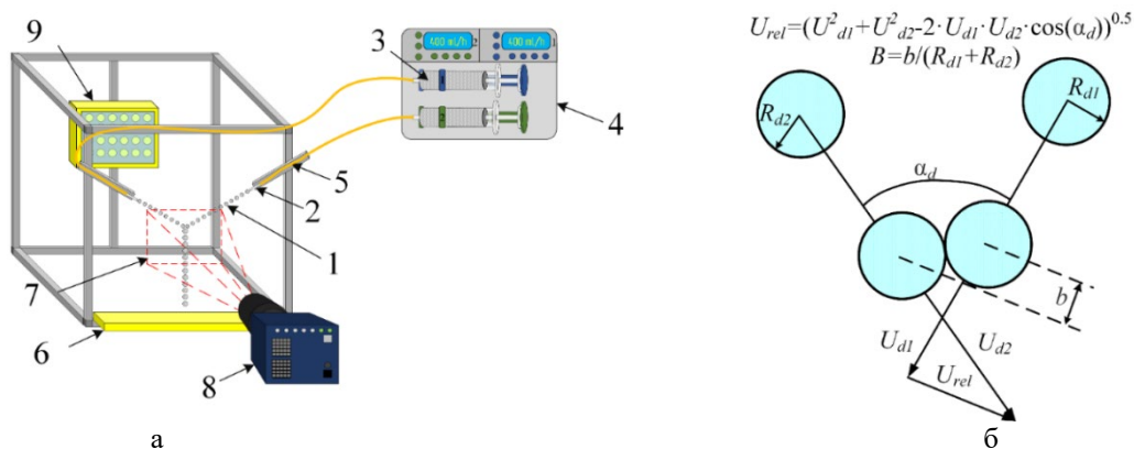
Рис. 1. Схемы стенда с основными элементами (а) и регистрации характеристик соударения капель (б): 1 – капли, содержащие твердые частицы; 2 – сменные сопла различного диаметра; 3 – шприц с жидкостью; 4 – шприцевой насос; 5 – силиконовые трубки; 6 – емкость для сбора жидкости; 7 – область регистрации; 8 – высокоскоростная видеокамера; 9 – диодный прожектор
