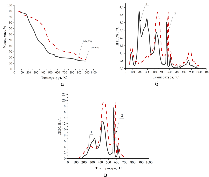
Рис. 1. Данные ТГ (а), ДТГ (б) и ДСК (в) : 1 – биомасса банановой кожуры; 2 – биоуглерод из банановой кожуры
