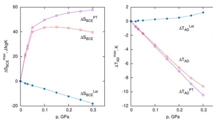
Рис. 2. Зависимости от давления максимальных значений экстенсивного (а) и интенсивного (b) БКЭ в (NH 4 ) 3 GeF 7 вблизи фазового перехода первого рода при T 4
