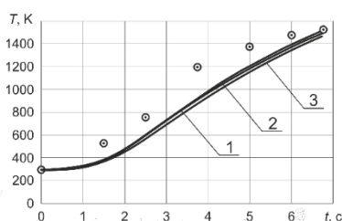
Рис. 3. Наружная температура обшивки к моменту завершения горения: 1 – прямоугольный канал (рис. 1, а); 2 – прямоугольный канал (рис. 1, б); 3 – треугольный канал (рис. 1, в); \odot – экспериментальные данные
