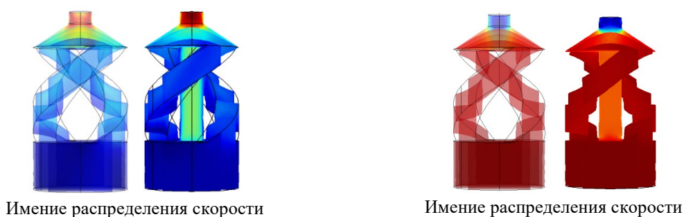
Рис. 3. Изменение параметров потока при отсутствии или наличии канала в шнеке.
