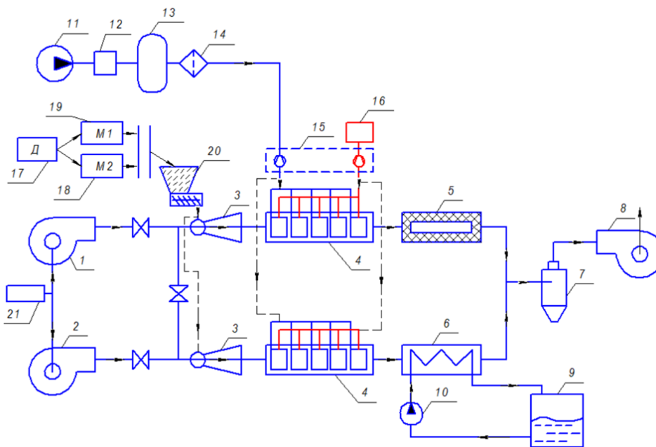
Рис. 1. Технологическая схема экспериментальной установки:
