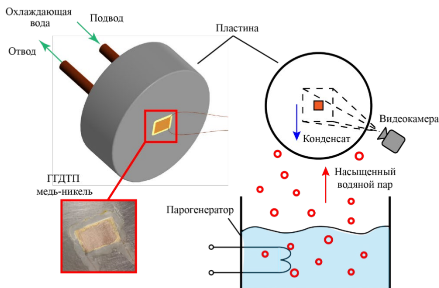
Рис. 1. Экспериментальная установка
