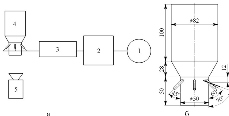
Рис. 1. Схема экспериментальной установки (а) и геометрические размеры диффузора (б): 1 – компрессор; 2 – ресивер для стабилизации потока; 3 – каналный нагреватель; 4 – вертикальный диффузор с визуализирующей сеткой; 5 – тепловизор
