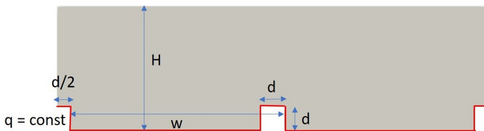
Рис. 1. Расчетная область
