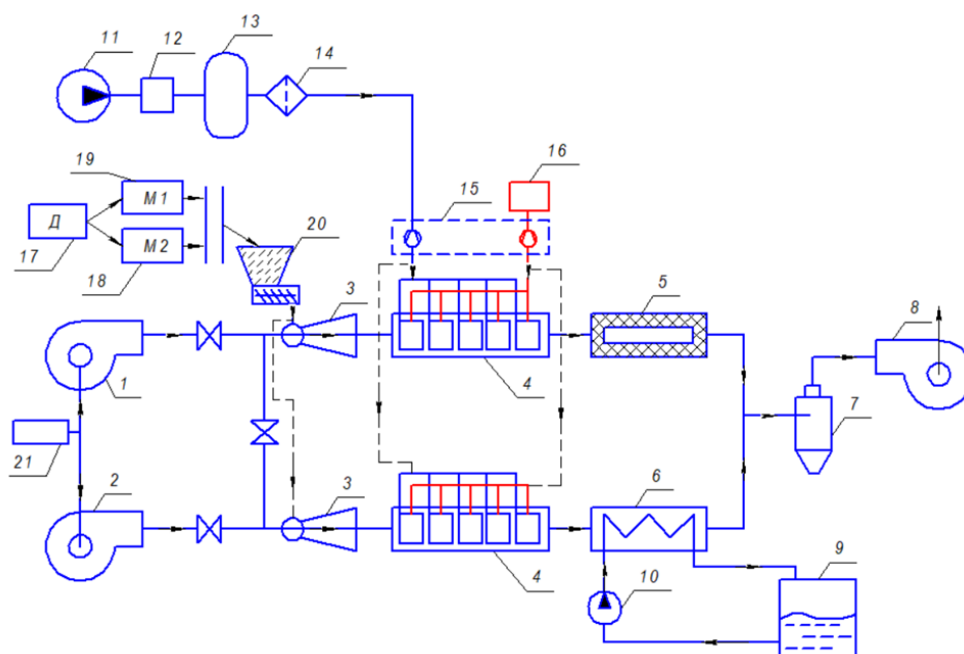
Рис. 1. Технологическая схема экспериментальной установки: 1 – вентилятор высоконапорный; 2 – вентилятор низконапорный; 3 – эжектор; 4 – модуль для розжига пыли; 5 – футерованная труба; 6 – водоохлаждаемая труба; 7 – золоуловитель; 8 – дымосос; 9 – бак охлаждающей воды; 10 – насос; 11 – компрессор; 12 – осушитель; 13 – ресивер; 14 – блок фильтрации; 15 – узел регулирования к радиационным горелкам; 16 – баллон с пропаном; 17 – дробилка; 18, 19 – дисковый истиратель; 20 – питатель пыли; 21 – калорифер
