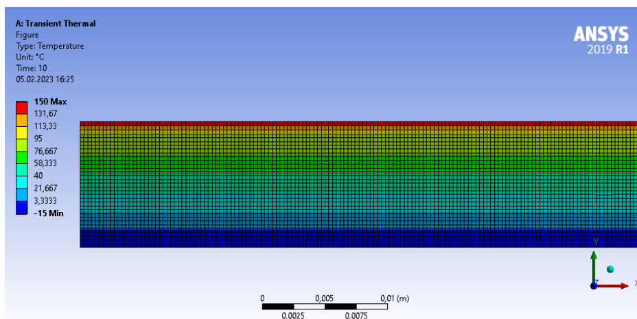
Рис. 2. Температурные поля при нестационарном режиме нагрева для алюминиевого сплава с покрытием на основе МДО ( t = 10 с)
