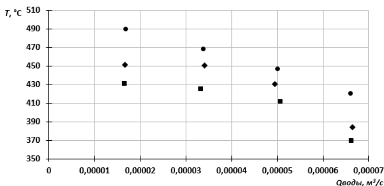
Рис. 3. Зависимости показаний одной из термопар от объемного расхода водяной компоненты дисперсного потока: \blacksquare — Q_{\text{возд}} = 0,0005 \text{ м}^3/\text{с} , \blacklozenge — Q_{\text{возд}} = 0,00091 \text{ м}^3/\text{с} , \bullet — Q_{\text{возд}} = 0,00133 \text{ м}^3/\text{с}
