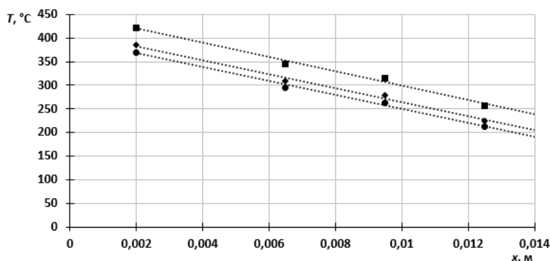
Рис. 2. Распределение температуры стенки по толщине рабочего участка ( Q_{\text{воды}} = 0,000065 \text{ м}^3/\text{с} ) при различных значениях объемного расхода рабочего газа: \blacksquare — Q_{\text{возд}} = 0,0005 \text{ м}^3/\text{с} , \blacklozenge — Q_{\text{возд}} = 0,00091 \text{ м}^3/\text{с} , \bullet — Q_{\text{возд}} = 0,00133 \text{ м}^3/\text{с}
