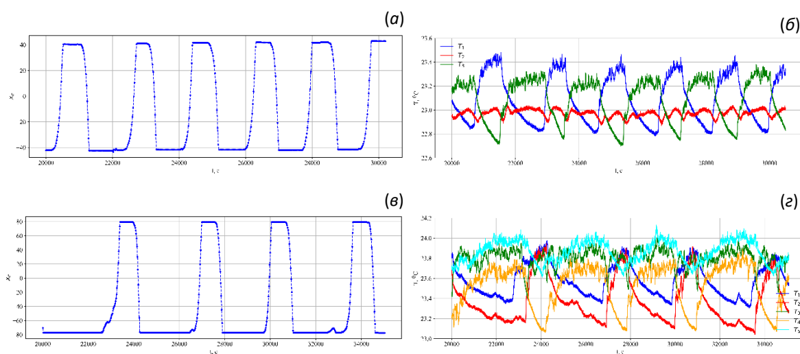
Рис. 1. Временная эволюция координаты центра диска x_c (а, в) и температуры на нижней поверхности (б, з) в случае фольгированного диска: а, б – L = 180 мм, h = 4 мм; в, з – L = 250 мм, h = 4 мм
