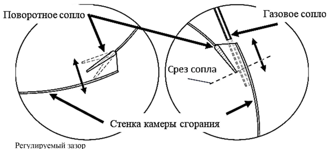
Регулируемый зазор Регулируемое положение газового ввода относительно тангенциального воздушного сопла срез тангенциального воздушного сопла
