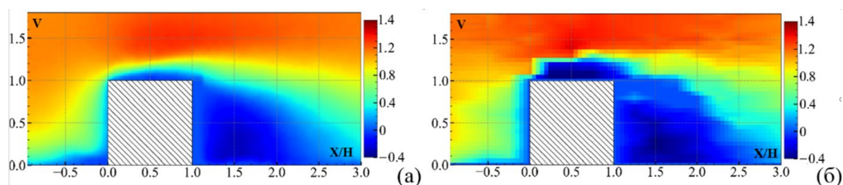
Рис. 1. Поля продольной компоненты скорости при обтекании кубов H = 50 мм, Re = 18\,000 (а) и H = 500 мм, Re = 225\,000 (б)
