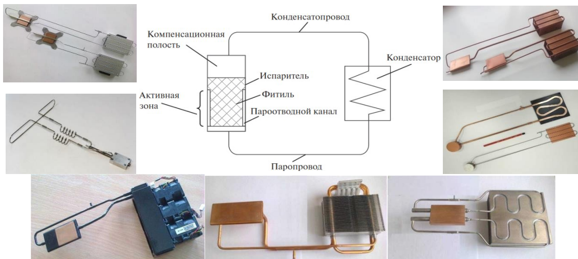
Рис. 1. Принципиальная схема и внешний вид КТТ
