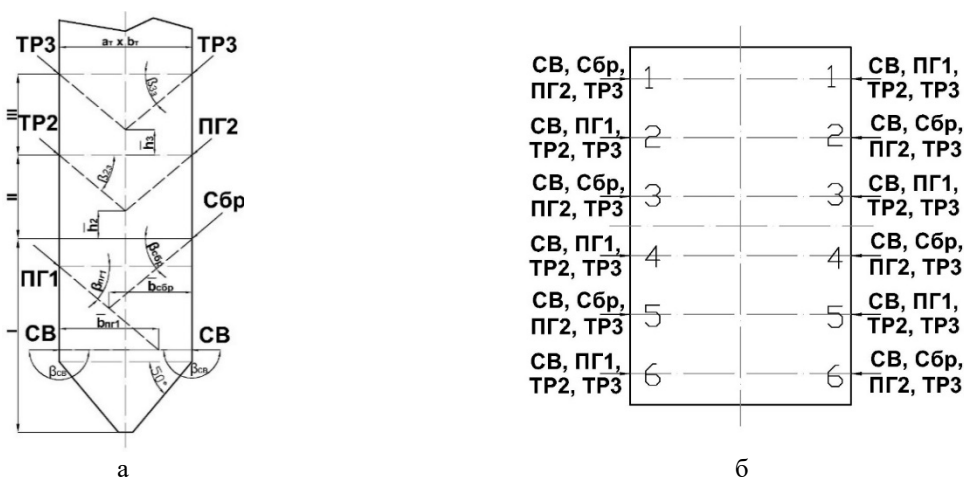
Рис. 1. Принципиальная схема расположения горелочных устройств и сопел в общем виде: а – вид в вертикальных сечениях 2-2, 4-4, 6-6; б – вид сверху; ПГ1 и ПГ2 – пылеугольная горелка I и II зоны соответственно; Сбр – сопло сбросного агента пылесистем; СВ – сопло вторичного воздуха; ТР1 и ТР2 – сопло третичного воздуха II и III зоны соответственно
