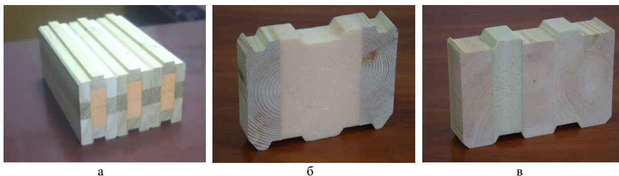
Рис. 1. Профилированный брус с утепляющими вставками: 1 – из трех элементов (ТГАСУ); 2 – фирмы «Сибрэкс» с утепляющей вставкой ПОЛИСТЕН; 3 – брус ОАО «Томская ДСК» с одной или двумя утепляющими вставками из пенополистирола
