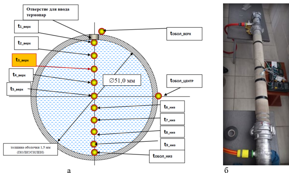
Рис. 1. Схема размещения спаев термопар по вертикальному диаметру гидростолба в РПН \varnothing 51 мм: а – схема; б – общий вид установки
