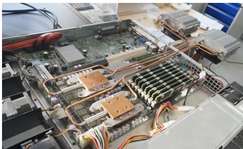
Рис. 2. Компьютерный сервер с контурными тепловыми трубами
