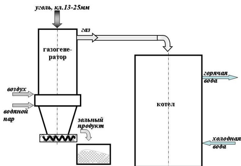
Рис. 1. Технологическая схема экологически чистого локального теплоисточника, работающего на топливном генераторном газе
