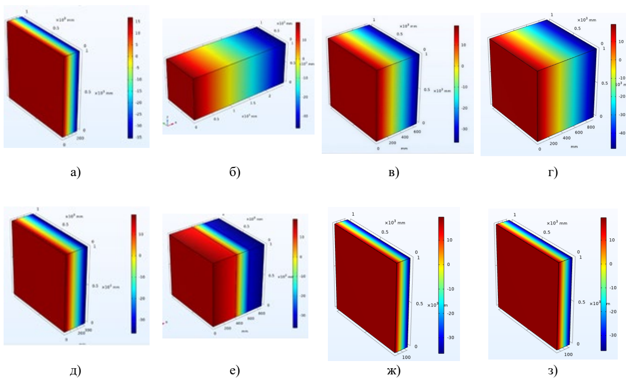
Рис.1. Распределение температуры в ограждающей конструкции: а) дерево; б) обыкновенный глиняный кирпич; в) арболит; г) саман; д) дерево, утеплитель (прессованная солома), дерево; е) кирпич, утеплитель (прессованная солома), кирпич; ж) СИП-панель; з) цементная EPS сэндвич-панель
