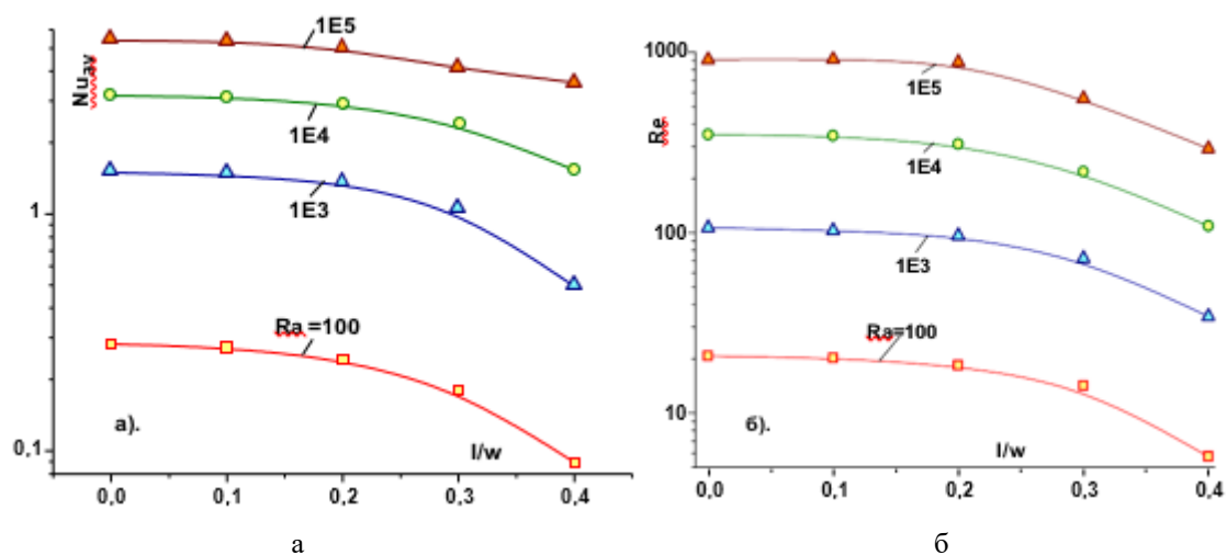
Рис. 1. Влияние высоты ребра на теплообмен (а) и конвективную тягу (б) в вертикальном канале
