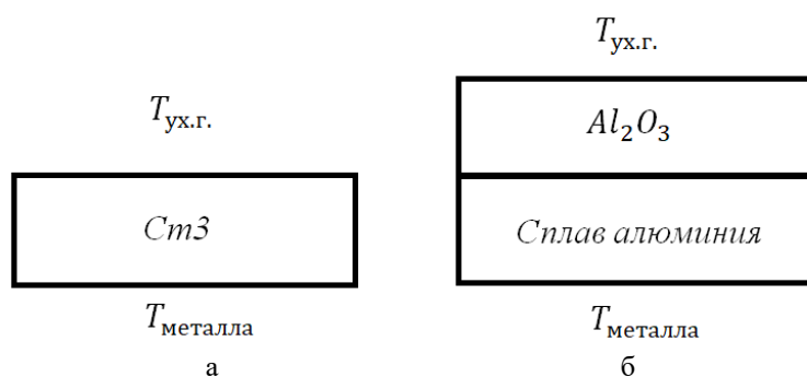
Рис. 1. Геометрия модельного образца: а – Ст3; б – сплав алюминия с покрытием по методу МДО
