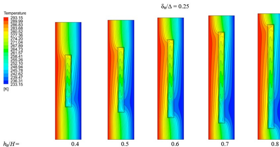
Рис. 2. Изотермы для одного ряда воздушных полостей
