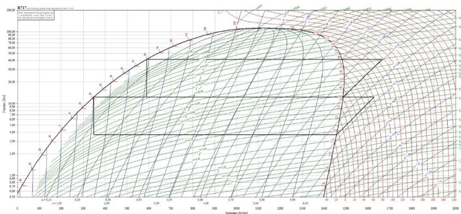
Рис. 1. Пример энергоэффективности двухступенчатого цикла аммиачного (R717 NH 3 ) теплового насоса при температуре испарения и конденсации -4\text{ }^{\circ}\text{C} и 80\text{ }^{\circ}\text{C} соответственно
