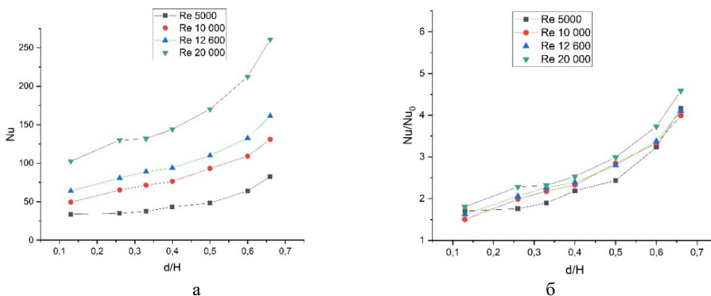
Рис. 2. Зависимость: а – среднего по поверхности числа Нуссельта; б – отношения Nu/Nu_0 , где Nu_0 – среднее по поверхности число Нуссельта в плоском канале
