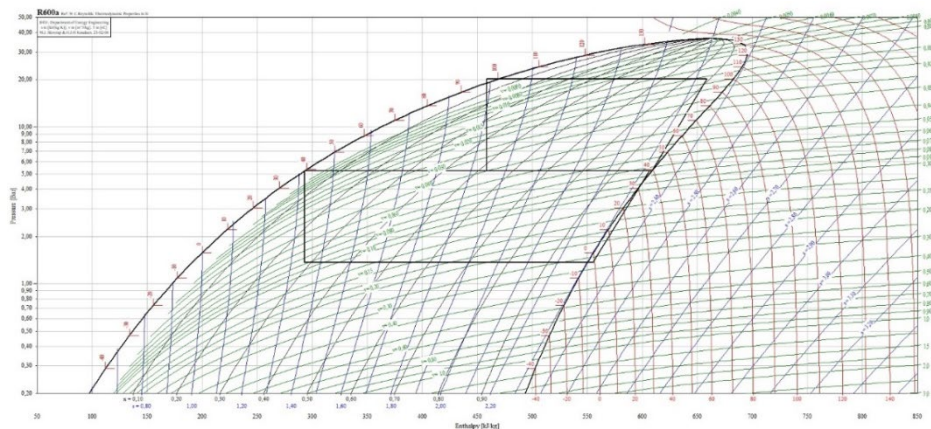
Рис. 2. Пример двухступенчатого цикла высокотемпературного теплового насоса с рабочим телом R600a (C4H10 изобутан). Температура испарения и конденсации -4^{\circ}\text{C} и 100^{\circ}\text{C} соответственно. Перегрев 3К, переохлаждение 3К
