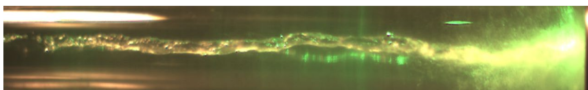
Рис. 2. Структура потока в патрубке за диафрагмой вихревой камеры на режиме 2
