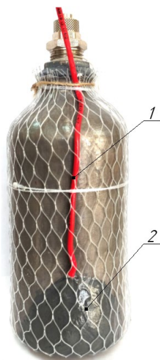
Рис. 1. Экспериментальная емкость: 1 – термопара со слоем тепловой изоляции; 2 – слой эпоксидного компаунда
