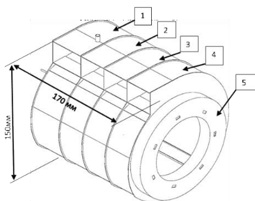
1 – торцевая вихревая камера; 2 – обечайка № 1; 3 – обечайка № 2; 4 – обечайка № 3; 5 – пережим
