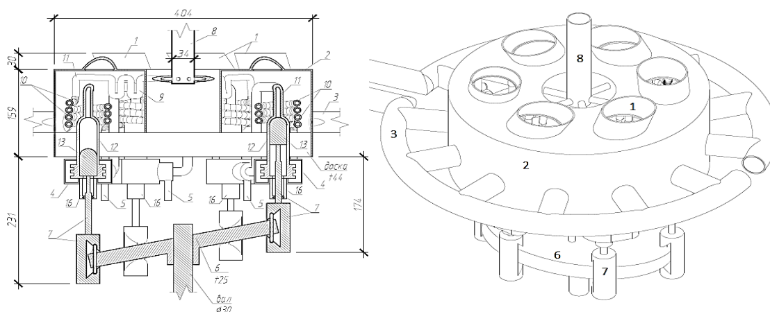
Рис. 1. Чертеж двигателя Стирлинга вид сбоку с разрезом (слева) и общий вид (справа): 1 – отверстия для горелок; 2 – камера сгорания; 3 – выхлопная труба; 4 – водный радиатор; 5 – патрубки для подачи оборотной воды; 6 – косая шайба; 7 – кривокопфный механизм; 8 – выходная труба горячей оборотной воды; 9 – ширма; 10 – экономайзер (акцептор); 11 – трубка нагревателя; 12 – цилиндр; 13 – поршень; 16 – уплотнительная втулка
