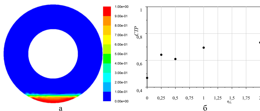
Рис. 1. Распределение второй фазы в поперечном сечении канала вблизи выхода (а) и график зависимости СТР от содержания наночастиц в базовом растворе (б)
