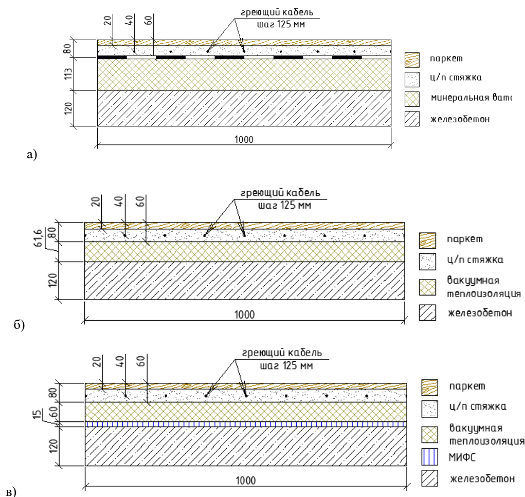
Рис. 1. Принятые к расчету конструкции полов: а – образец для сравнения; б – конструкция с вакуумной теплоизоляцией; в – конструкция с вакуумной теплоизоляцией и МИФС
