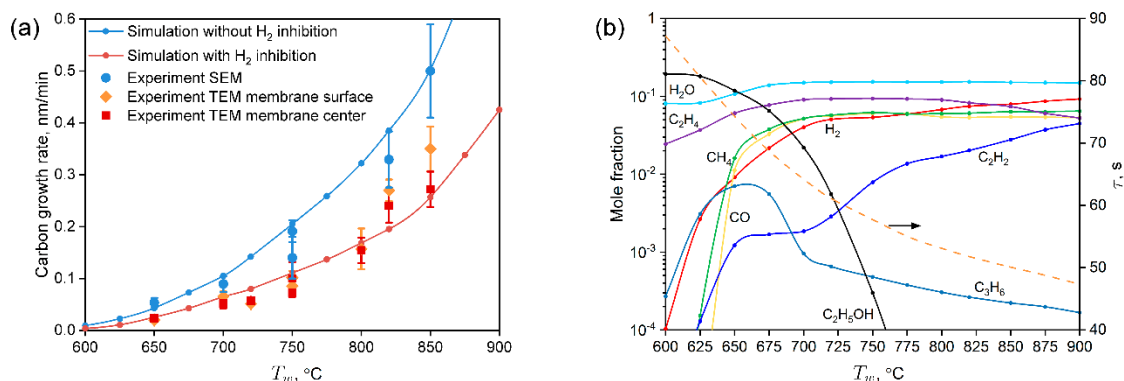
Рис. 2. Зависимость скорости роста стенок углеродных нанотрубок (a) и молярных долей частиц, усредненных по поверхности мембраны / времени пребывания (b) от температуры стенки реактора. Давление 0,5 бар, расход аргона 200 мл / мин, расход этанола 0,083 мл / мин.
