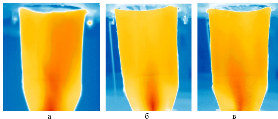
Рис. 2. Термограммы структуры потока в вертикальном диффузоре при подаче воздуха (средняя скорость около 6,5 м/с) через трубки, установленные под разными углами: а – 45^\circ ; б – 60^\circ ; в – 70^\circ
