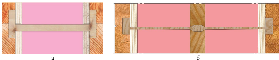
Рис. 2. Профилированный брус с утепляющими вставками: 1 – с П-образным коллектором; 2 – с Ж-образным коллектором
