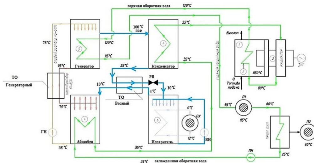
Рис. 2. Система тригенерации на основе представленного типа двигателя и одноступенчатой АТТ: 1 – камера сгорания; 2 – акцептор; 3 – двигатель Стирлинга; 4 – гидропетля; 5 – жаротрубный пучок; 6 – охлаждаемый контур; П1(2) – потребитель тепла; ПХ – потребитель холода; ПН, ГН, ВН – питательный, генераторный и водяной насосы соответственно
