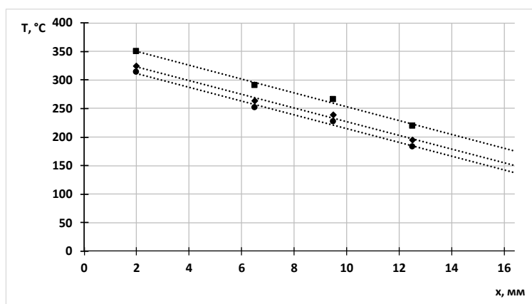
Рис. 2. Температура поверхности рабочего участка в зависимости от продольной координаты
