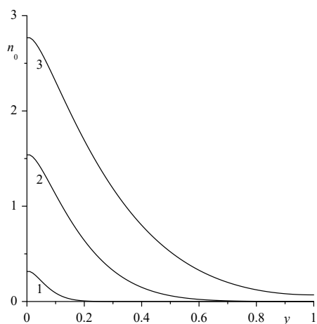
Рис. 3. Безразмерные профили бензоата лития в разные моменты времени: 1 – t = 2 ; 2 – t = 15 ; 3 – t = 50
