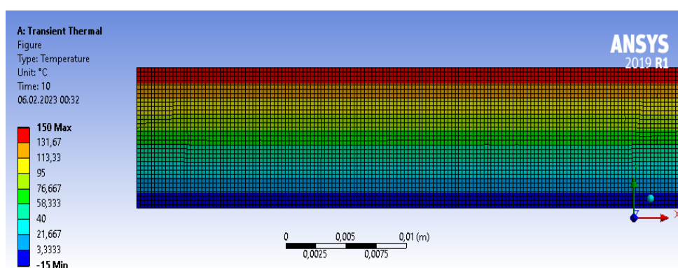
Рис. 3. Температурные поля при нестационарном режиме нагрева для Ст3 ( t = 10 с)
