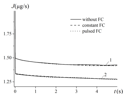
Рис. 2. Временные зависимости скорости испарения для различных режимов вынужденной конвекции: 1 – \text{CH}_4 ; 2 – \text{N}_2
