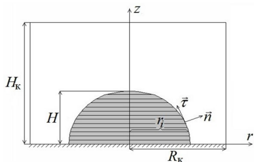
Рис. 1. Схема эксперимента
