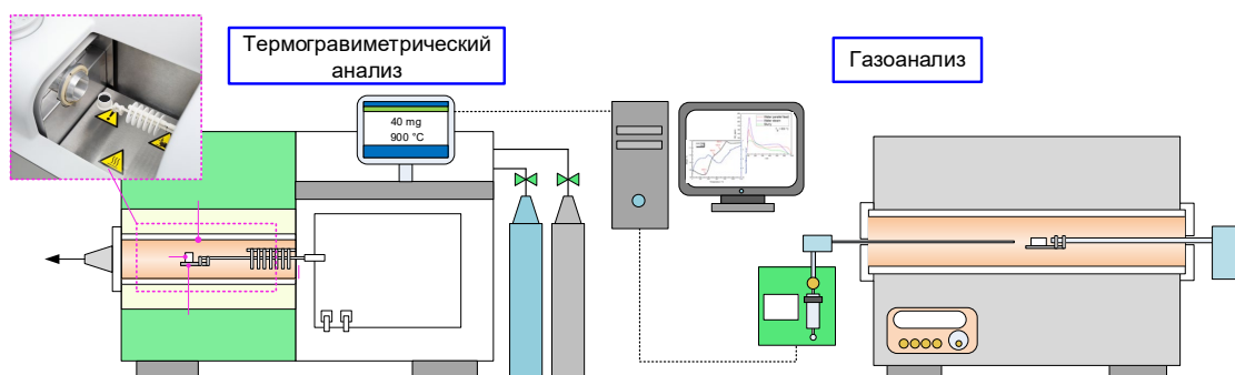
Рис. 1. Схема экспериментального стенда
