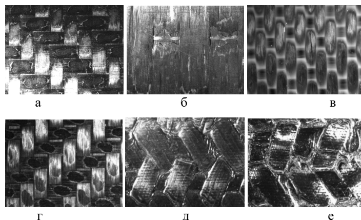
Рис. 1. Структуры ПКМ с различным армированием: а – образец 1; б – образец 2; в – образец 3; г – образец 4; д – образец 5; е – образец 6
