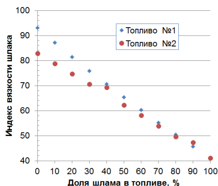
Рис. 2. Зависимость индекса вязкости шлака от доли шлака в композиционном топливе
