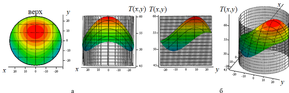
Рис. 3. Азимутально-радиальные распределения температуры воды в РПН \varnothing 51 мм, полученные по экспериментальным точкам: a – изотермы (карта) распределения T(x,y) ; б – 3D-график распределения T(x,y)
