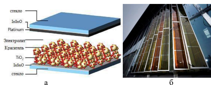
Рис. 1. Функциональная структура и компоненты DSSC (а) и общий вид солнечного модуля (б)
