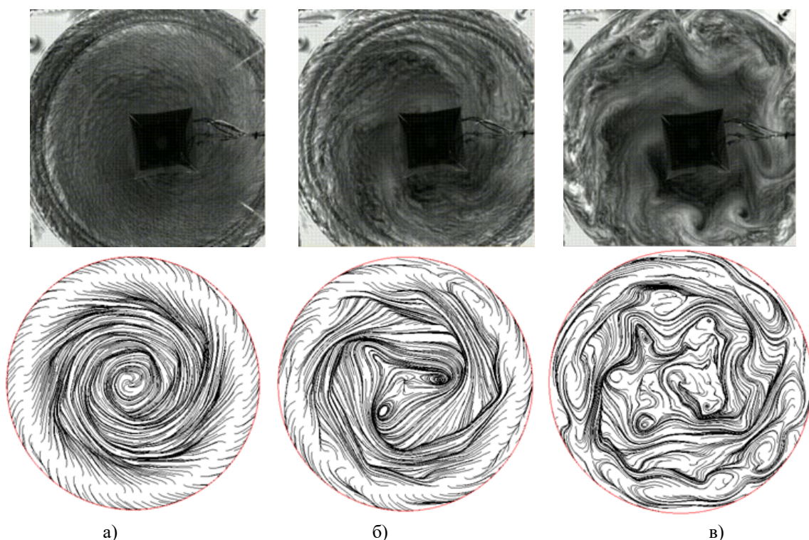
Рис. 1. Мгновенное течение. Верхний ряд – лабораторный эксперимент, нижний ряд – траектории частиц в относительном движении, численный расчёт. Период вращения Trot , с: а – 77; б – 47; в – 17
