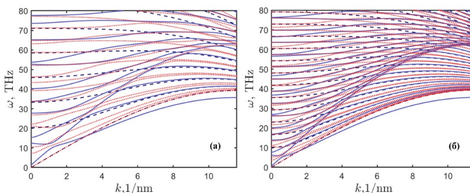
Рис. 1. Дисперсионные соотношения для квантовых нитей диаметром 2,7 нм (а) и 5,4 нм (б).
