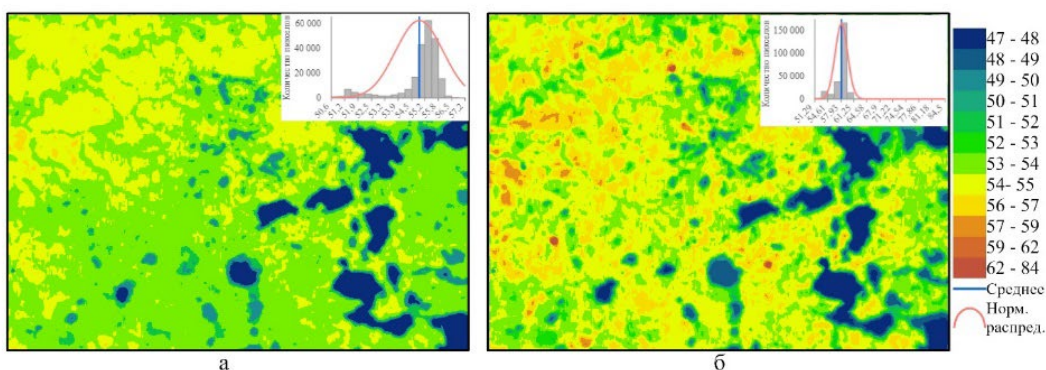
Рис. 2. Исследуемая территория в температурном градиенте на основании индекса LST. Распределение пикселей индекса LST на основании данных Landsat-8: а – в 2014 г.; б – в 2022 г.
