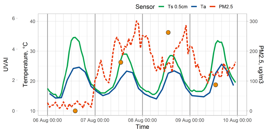
Рис. 1. Температура деятельного слоя почвы TS (на глубине 0,5 см), температура воздуха ТА, концентрация PM2.5 (на высоте 2 м), значение индекса UVAI в д. Минино
