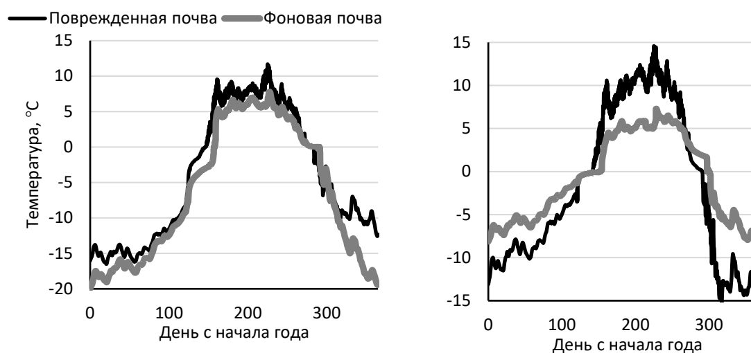
Рис. 1. Изменение температуры на глубине 1 м в течение года. Слева: условия лиственничников в криолитозоне Среднесибирского плоскогорья. Справа: модельные условия на широте Красноярска
