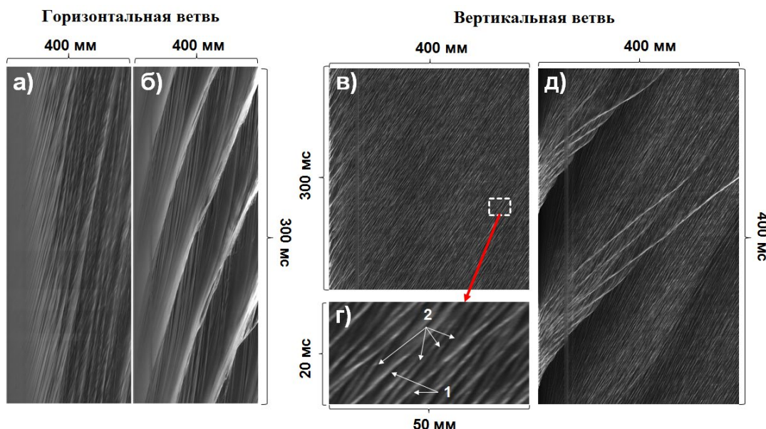
Рис. 2. а, б) Re = 300 , V_g = 8 \text{ м/с} , f = 0 \text{ Гц} (а), f = 10 \text{ Гц} (б); в-д) Re = 50 , V_g = 43 \text{ м/с} , f = 0 \text{ Гц} (в, г), f = 5 \text{ Гц} (д)
