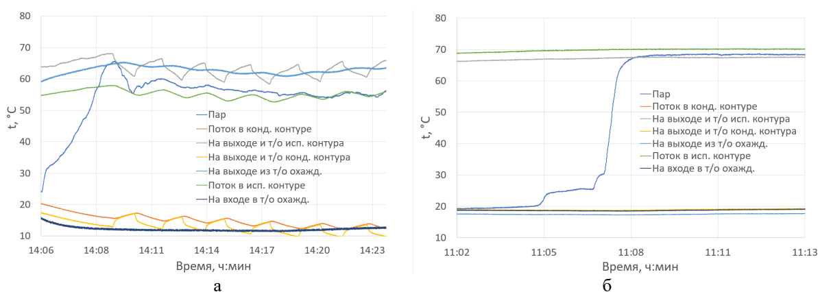
Рис. 2. Графики изменения температуры: а – с включенным тепловым насосом; б – без запуска теплового насоса
