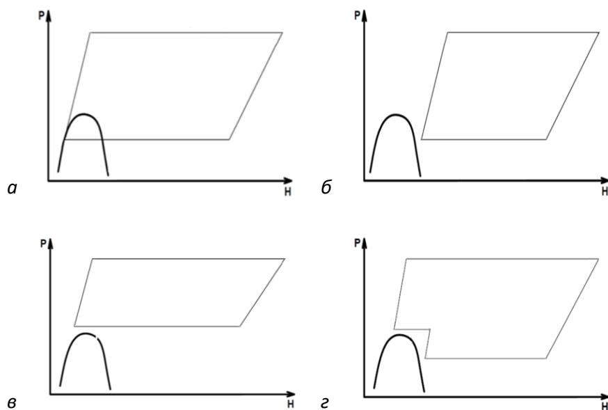
Рис. 1. P-h-диаграммы \text{CO}_2 -циклов: а – с конденсацией рабочего тела; б – с одноступенчатым компрессорным повышением давления; в – с одноступенчатым повышением давления насосом; з – с двухступенчатым повышением давления компрессором и насосом
