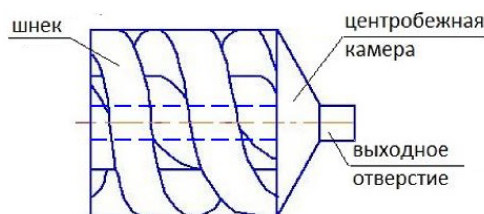
Рис. 2. Шнек, основной элемент центробежной форсунки
