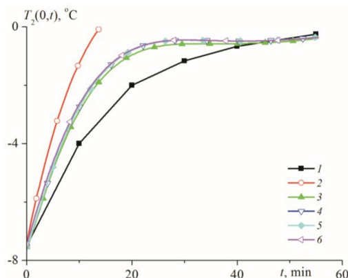
Рис. 1. Динамика роста температуры левой поверхности льда на разных подложках: 1 – данные [3], 2 – A = \Lambda = 0,01 , 3 – подложка из бакелита, 4 – при A = \Lambda = 1 , 5 – при A = \Lambda = 100 , 6 – расчет по [6]
