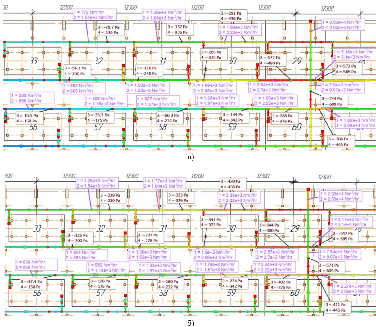
Рис. 2. Сравнение эксперимента с расчетом: а) до идентификации; б) после идентификации; 1 – расход, рассчитанный сетевой моделью; 2 – замеры расхода; 3 – статическое давление, рассчитанное сетевой моделью; 4 – замеры давления
