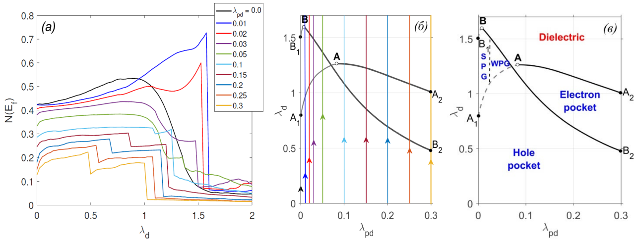
Рис. 1 (а) Плотность состояний на уровне Ферми слабодопированной системы. (б) Соответствие типов перехода металл-диэлектрик областям плавного и резкого изменения функций полярона и биполярона в кластере. А и В – точки разрыва функций полярона и биполярона в основных состояниях соответственно. A_1A и B_1B – линии перегиба поляронных и биполяронных свойств как функции диагонального \lambda_d электрон-фононного взаимодействия при фиксированном недиагональном \lambda_{pd} . AA_2 и BB_2 – линии резкого кроссовера для полярона и биполярона. (в) Обобщающая фазовая диаграмма поляронной системы: WPG и SPG – слабая и сильная псевдощель, hole pocket и electron pocket – дырочные и электронные карманы на поверхности Ферми.
