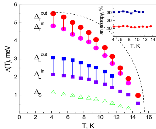
Рис. 2. Температурные зависимости СП энергетических параметров \text{LiFeAs} . Цвета для \Delta_j соответствуют таковым с Рис. 1. Вставка – температурные зависимости анизотропии большой \Gamma - (красные кружки) и средней L - (синие квадраты) СП щелей.
