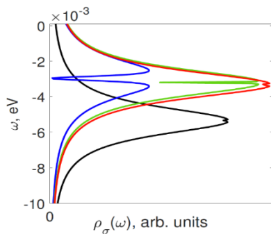
Рис. 1. Плотность состояний Андерсоновской КТ для различных температур и напряжений
