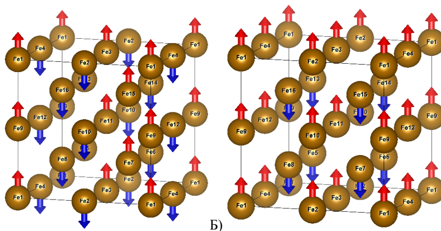
Рис. 1. Конфигурации атомов в суперячейке для ОЦК Fe. Стрелками обозначены направления магнитных спинов.
