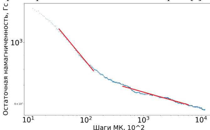
Рис. 1 Логарифм релаксации захваченного магнитного потока. Диаметр 3 мкм, температура 10 К
