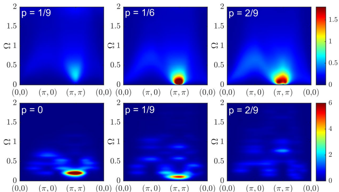
Рис 1. Динамическая спиновая восприимчивость вдоль симметричных направлений зоны Бриллюэна в рамках СРТ-RPA (сверху) и spin-СРТ (снизу) для различных значений допирования p [2]
