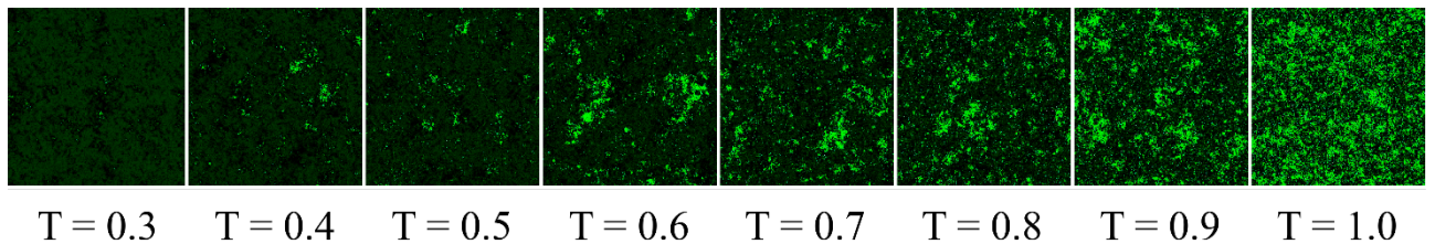
Рис. 1. Корреляционные матрицы XY-модели для 0.3 \leq T \leq 1.0 .
