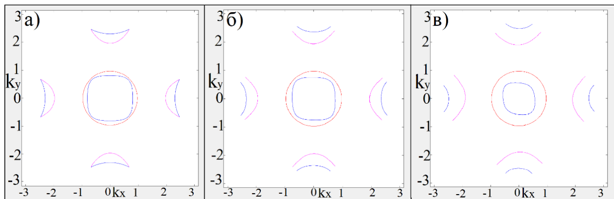
Рис. 2. Ферми-поверхность пниктида железа при наличии z-компоненты спин-орбитального взаимодействия: а) \lambda = \lambda' = 0 ; б) \lambda = \lambda' = 0,2 ; в) \lambda = \lambda' = 0,4 .
