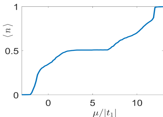
Рис 1. DMRG расчеты зависимости концентрации фермионов от химпотенциала в цепочке Китаева с сильным кулоновским межузельным отталкиванием фермионов. Расщепление затравочной зоны фермионов с образованием двух подзон свидетельствует о реализации в системе зоны флуктуационных состояний.
