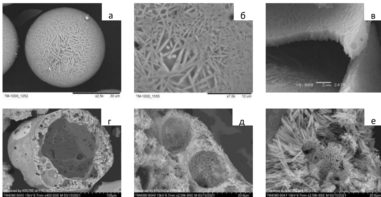
Рисунок 2. СЭМ-снимки узких фракций ценосфер кольцевого строения -0,063 \pm 0,05 (а–в) и сетчатого строения -0,25 \pm 0,2 (г–е)
