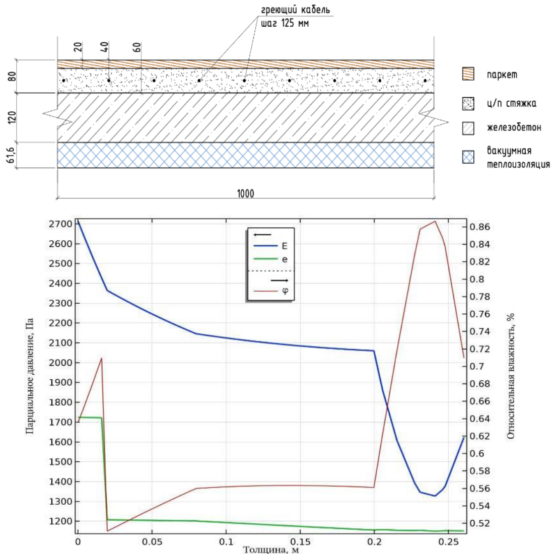
Рисунок 2. Вакуумная теплоизоляция на поверхности перекрытия подземной автостоянки. E – давление водяного пара, Па; e – парциальное давление насыщенного водяного пара, Па; φ – относительная влажность, %
