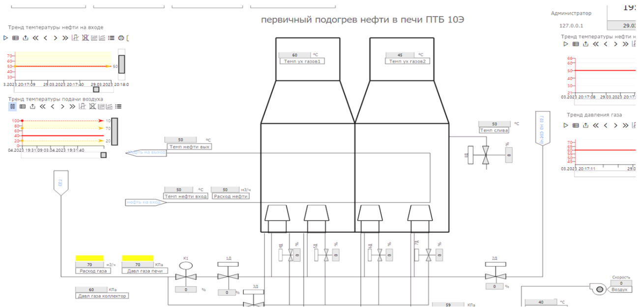
Рисунок 7. Экран процесса подогрева нефти
