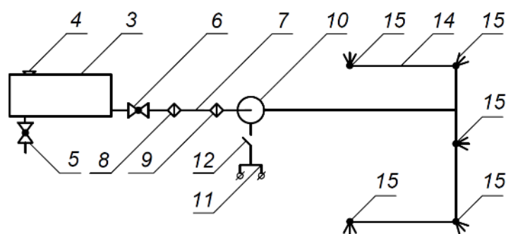
Рисунок 1. Гидравлическая схема подвесной системы для подавления пылегазовых выбросов карьерного самосвала
