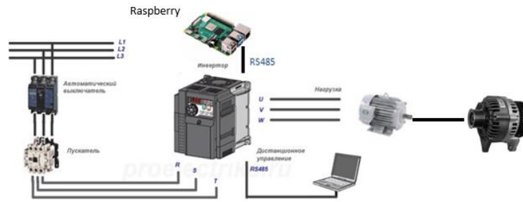
Рисунок 1. Лабораторный стенд
