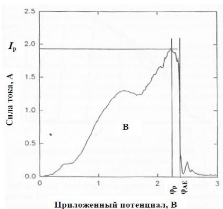
Рисунок 1. Типичный вид вольтамперограммы: I_p – ток пика, \varphi_p – потенциал при токе пика, \varphi_{AE} – потенциал при анодном эффекте, B – площадь вольтамперограммы [4,5].
