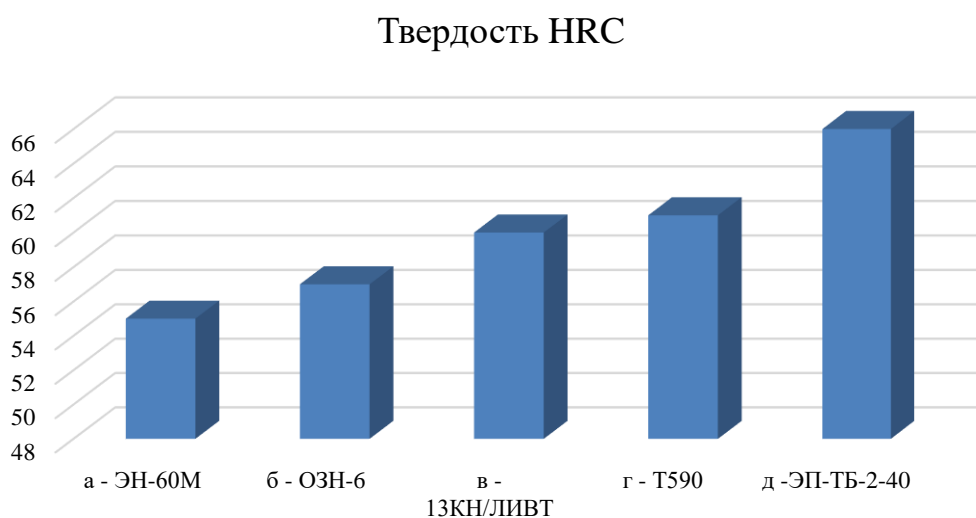
Рисунок. Сравнение твердости наплавленного слоя электродов: а - ЭН-60М, б - ОЗН-6, в - 13КН/ЛИВТ, г - Т590, д - ЭП-ТБ-2-40
