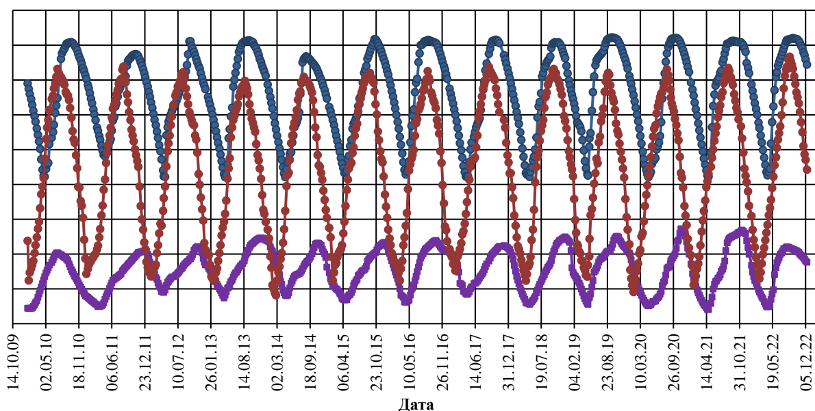
Рисунок 1. Связь уровней воды в пьезометре с УВБ.
