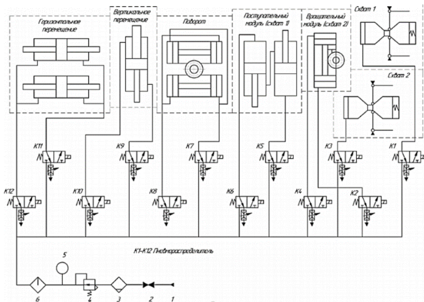
Рисунок 5 - Пневматическая схема МП–11
