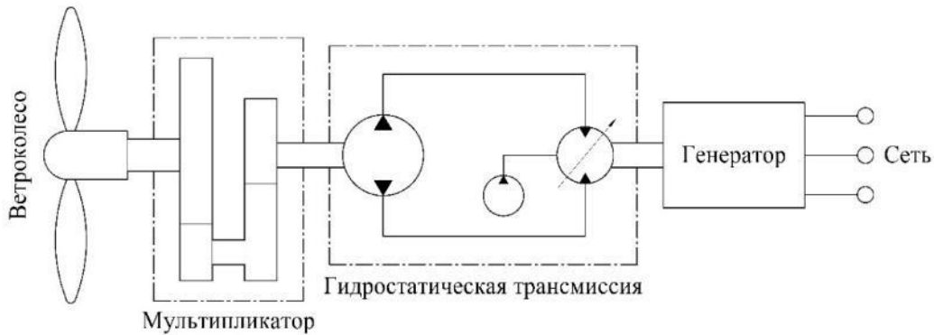
Рисунок 1. Схема ВЭУ с гидромеханической передачей
