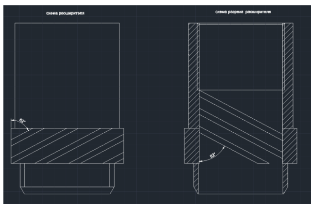
Рисунок 3. Схема предлагаемого расширителя
