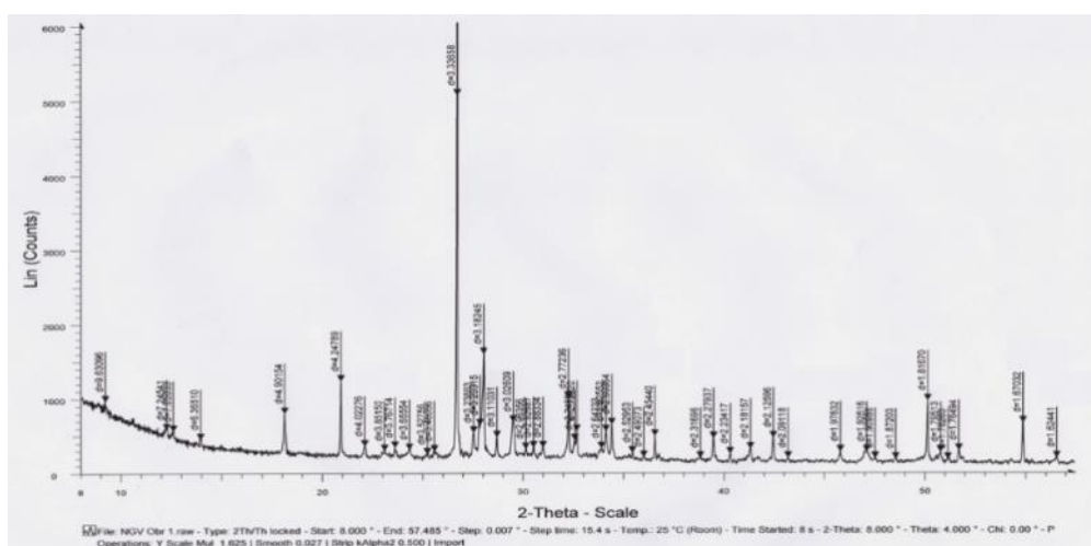
Рисунок 2. Дифрактограмма образцов состава твердой части смешанного стока.
