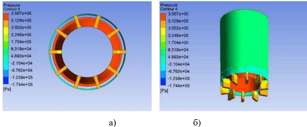
Рисунок 2. результаты моделирования гидродинамики коронки со стандартной формой матрицы: а – торец матрицы; б – вид сбоку.
