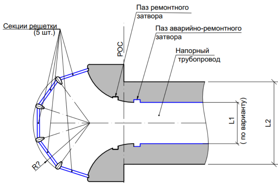
Рисунок. 1 Водоприемник гидросооружения
