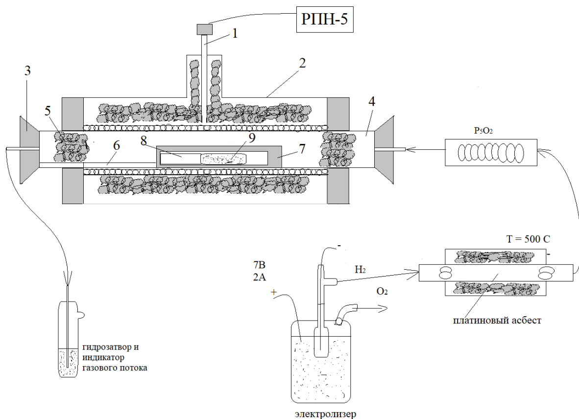
Рисунок 1. Схема ростовой установки (жидкость в гидрозатворе – серная кислота). 1 – регулирующая термопара с терморегулятором; 2 – печь; 3 – резиновые пробки; 4 –
