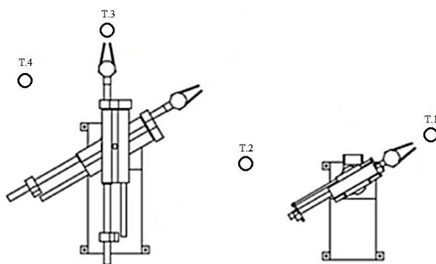
Рисунок 7 – Вторая траектория движения промышленных роботов
