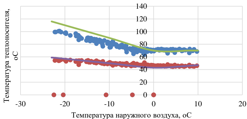
Рисунок 1. График зависимости температуры теплоносителя от температуры наружного воздуха
