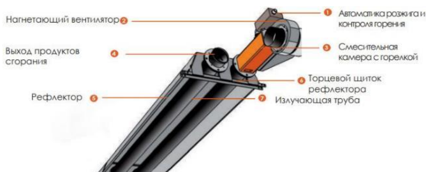
Рисунок 2. Схема ГИИ закрытой конструкции.
