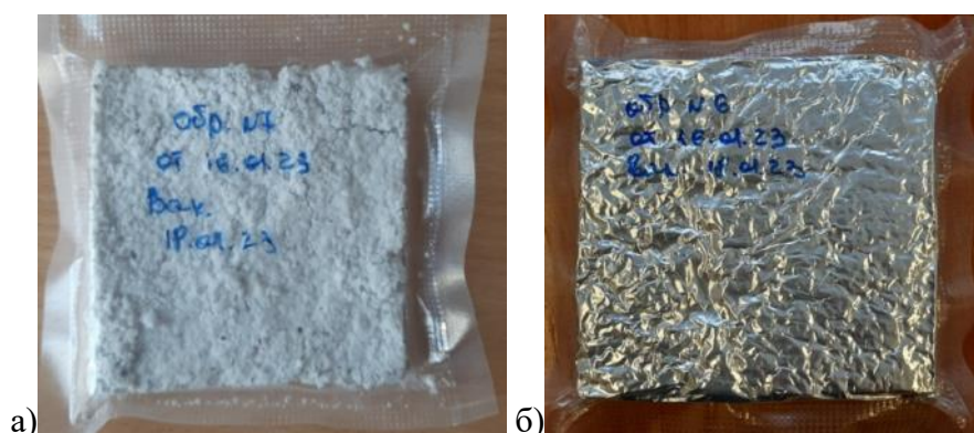
Рисунок 2. Лабораторные образцы вакуумированной плитки утеплителя
