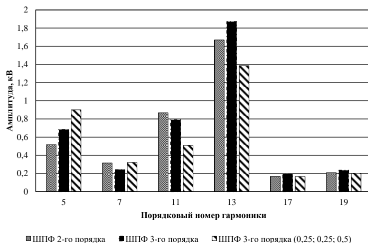
Рисунок 4. Спектры напряжения при установке многозвенных ФКУ
