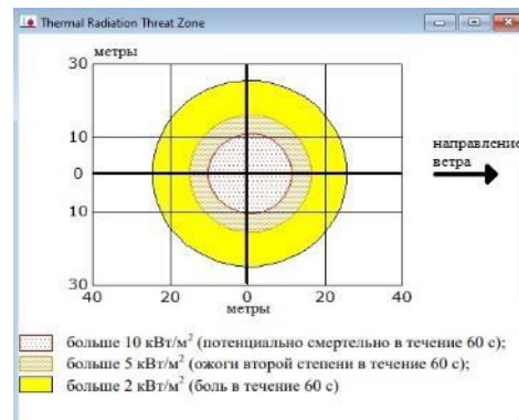
Рисунок 2. Зоны опасности при условной разгерметизации резервуара (газгольдера)
