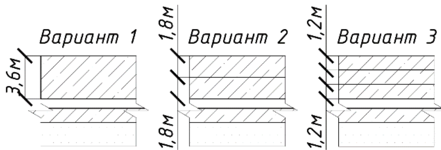
Рисунок 2. Варианты деления массивной фундаментной плиты ВЭУ на блоки бетонирования
