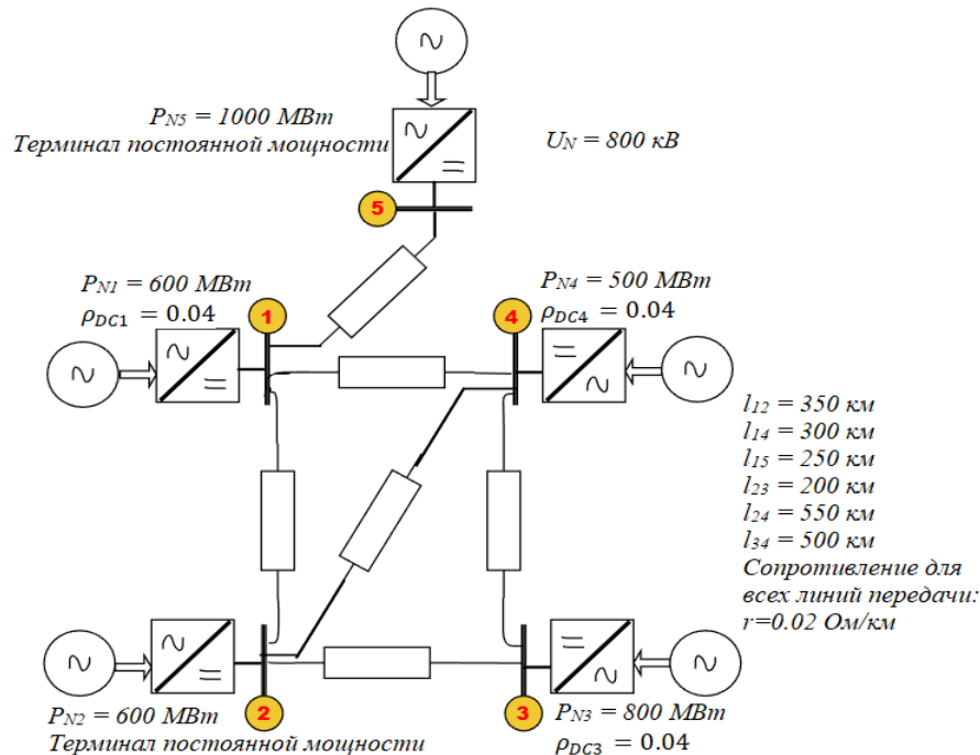
Рисунок 2. Схема МППТ, используемая при моделировании и симуляции
