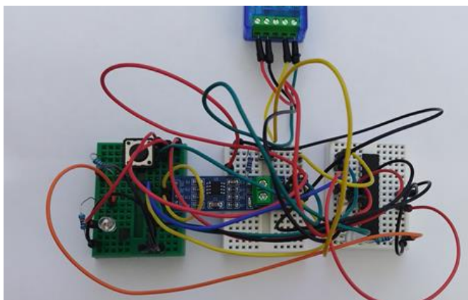
Рисунок 2. Прототип RS-485-совместимого ИК-передатчика
