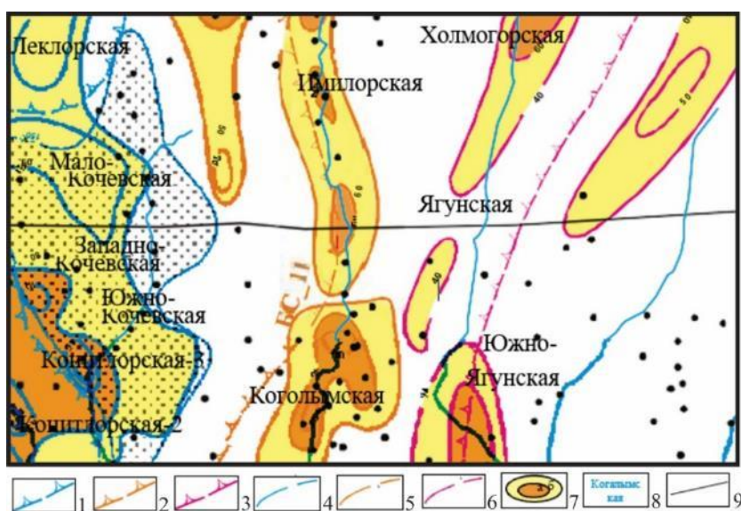
Рисунок 2. Фрагмент прогнознй схемы зон литологических резервуаров в клиноформах нижнего мела Сургутского района [2].
