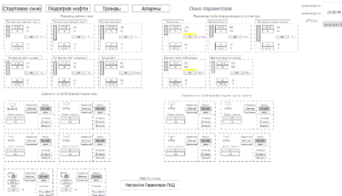
Рисунок 3. Окно параметров
