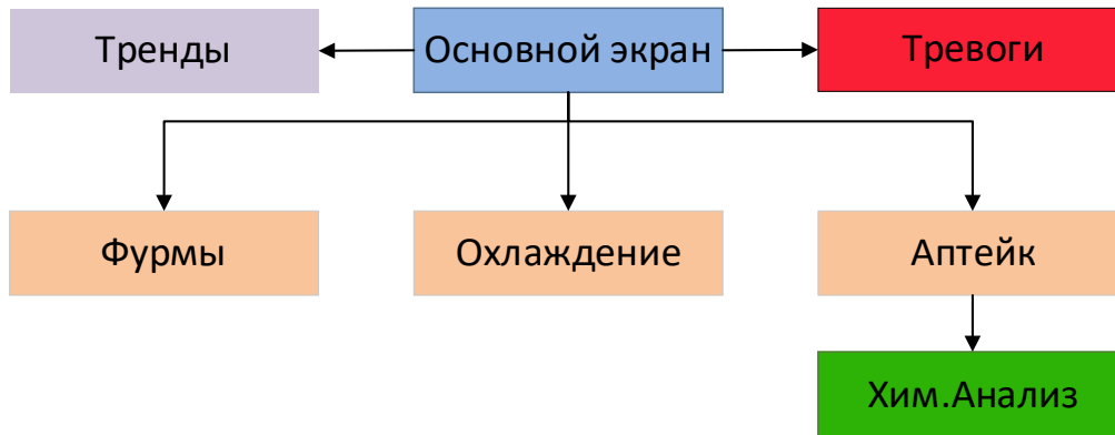
Рисунок 1. Иерархия экранов
