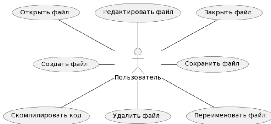
Рисунок 2. Диаграмма прецедентов
