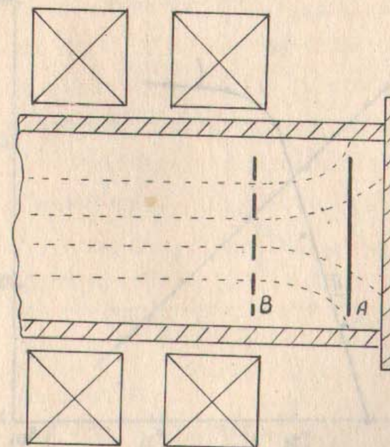
Рис.1б. Силовые линии магнитного поля в торце камеры. Расстояние ионизатор-экран в положении А-31 см, В-28 см.
