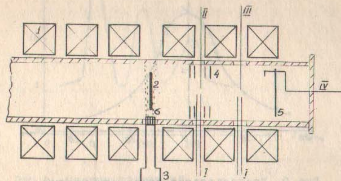
Рис.1а. Схема установки. I-катушки магнитного поля; 2-ионизатор; 3-испаритель; 4-измеритель диффузии; 5-экран; I-двойные зонды; II, III-одиночные зонды; IV-подвижный зонд.
