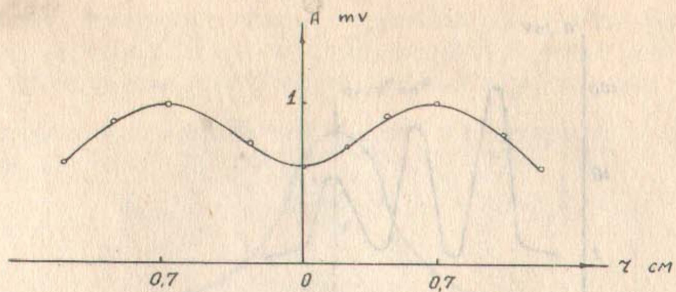
Рис.6. Зависимость амплитуды колебаний от радиуса.
