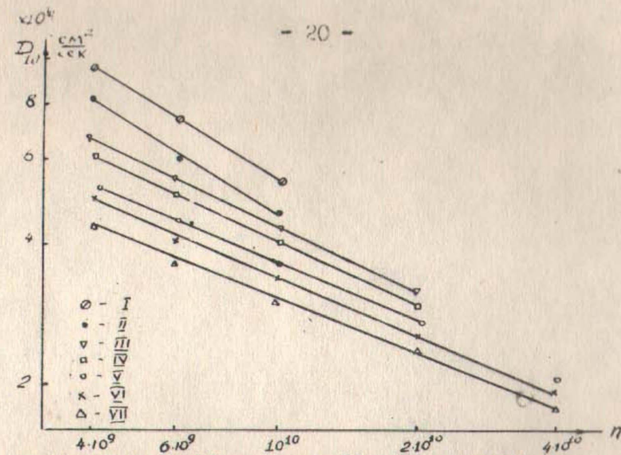
Рис. 12. Зависимость коэффициента диффузии от плотности. Магнитное поле H : I-100; II-200; III-400; IV-600; V-800; VI-1000; VII-1200 эрст.
