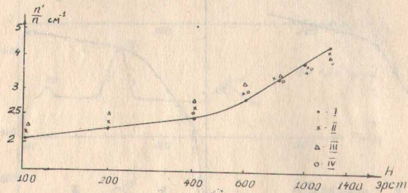
Рис. 11. Зависимость \frac{n'}{n} от магнитного поля (в логарифмическом масштабе). I- n = 4 \cdot 10^9 \text{ см}^{-3} ; II- n = 6 \cdot 10^9 \text{ см}^{-3} ; III- n = 1 \cdot 10^{10} \text{ см}^{-3} ; IV- n = 2 \cdot 10^{10} \text{ см}^{-3} .
