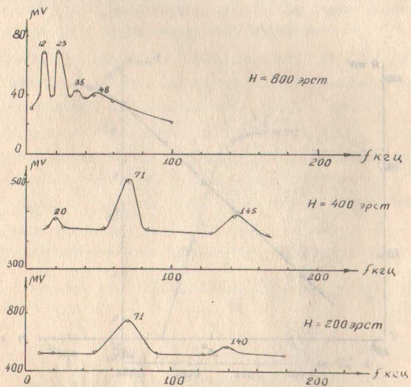
Рис.7. Спектр колебаний. Радиус плазменного столба \sim 10^{-3} см.
