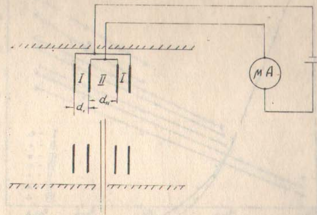
Рис.8. Измеритель диффузии. I-область разделения зарядов; II-область измерения \frac{dn}{dz} ; d_1 = 0,3 см; d_2 = 0,7 см.
