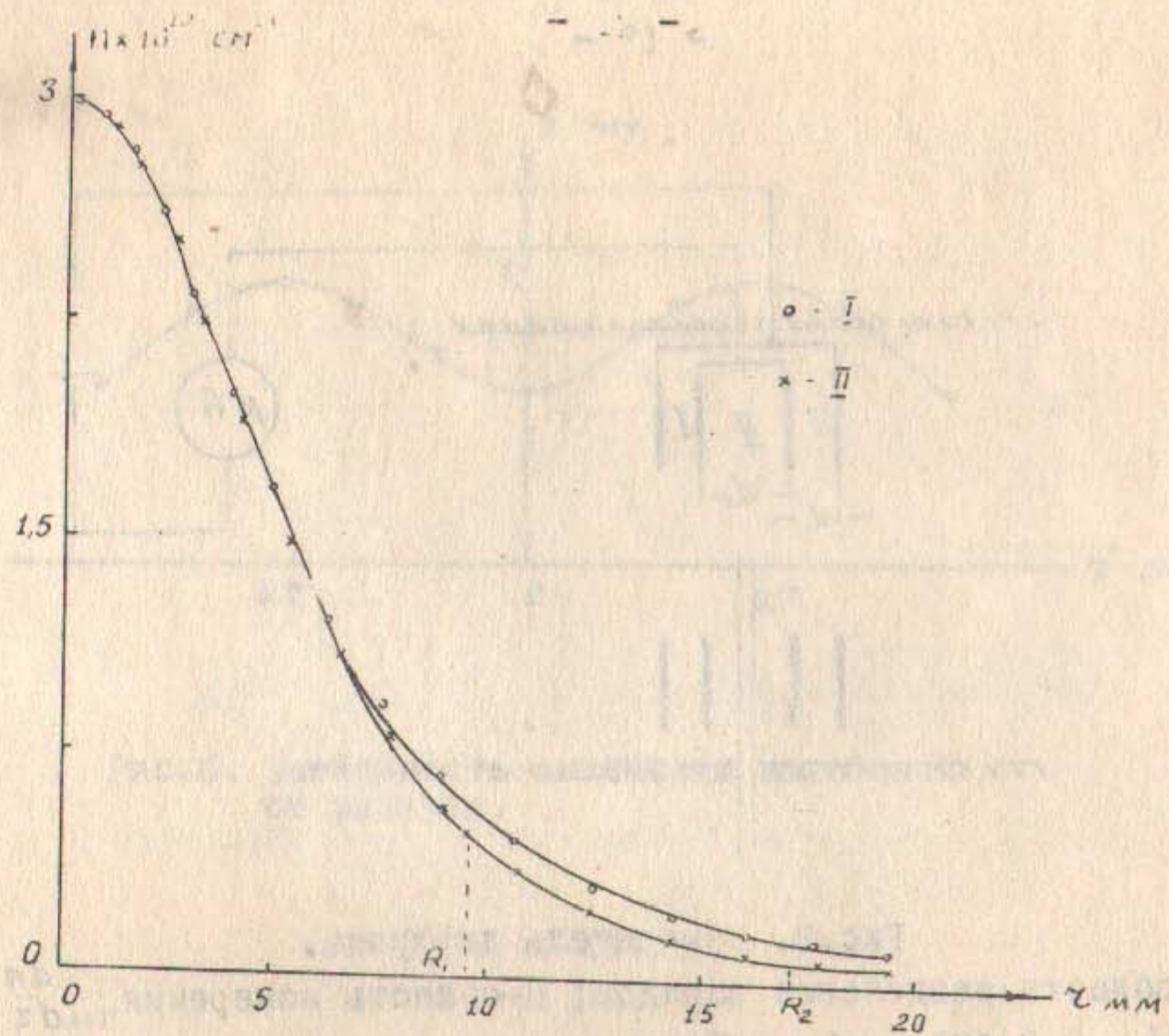
Рис. 10. Распределение плотности плазмы по радиусу. I-без колец; II-с кольцами H = 1000 эрстед.
