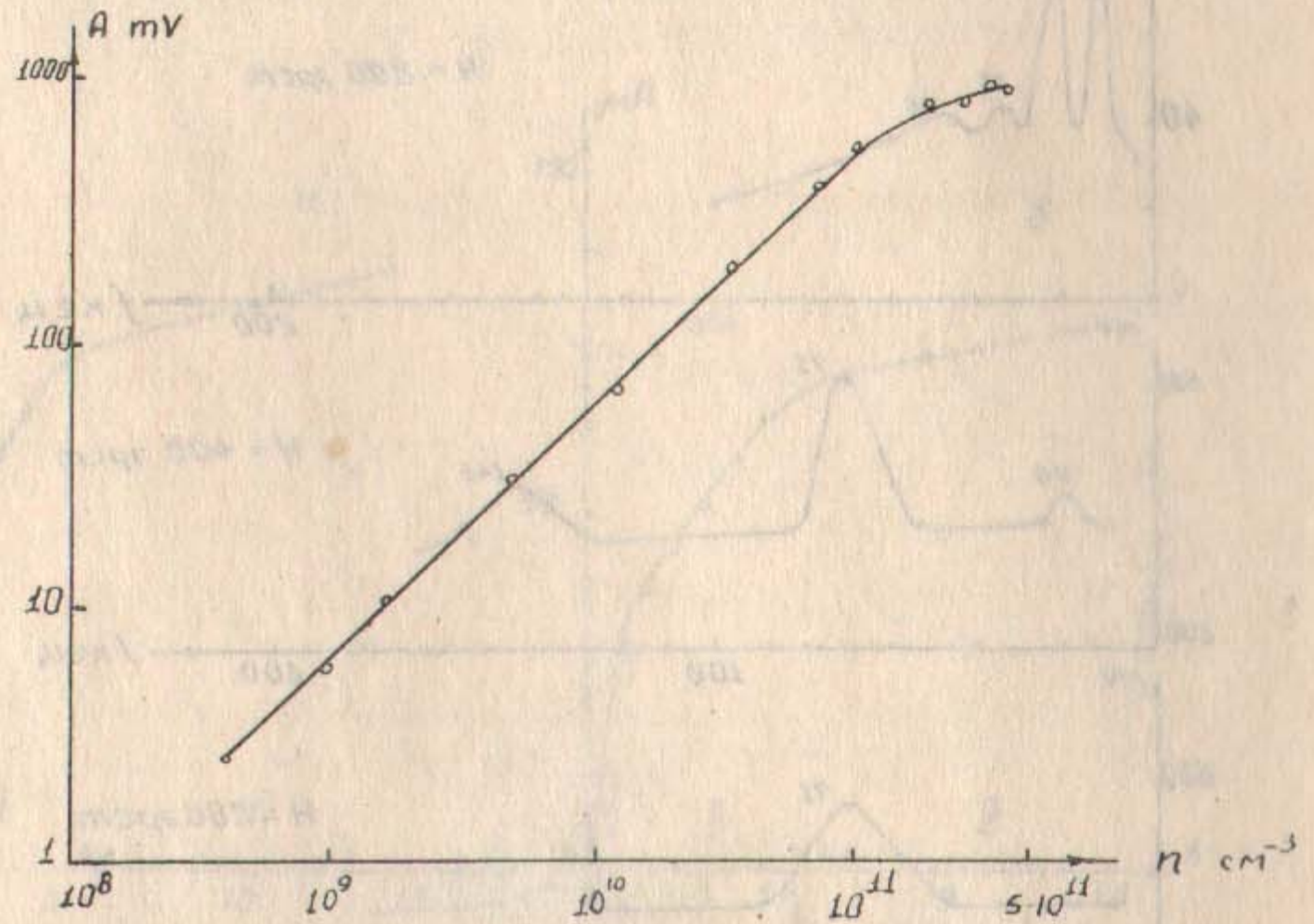
Рис.5. Зависимость амплитуды колебаний от плотности на оси.
