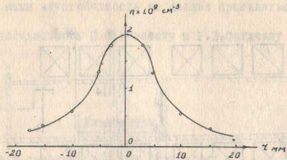
Рис.2. Распределение плотности плазмы по радиусу. H = 600 эрстед.
