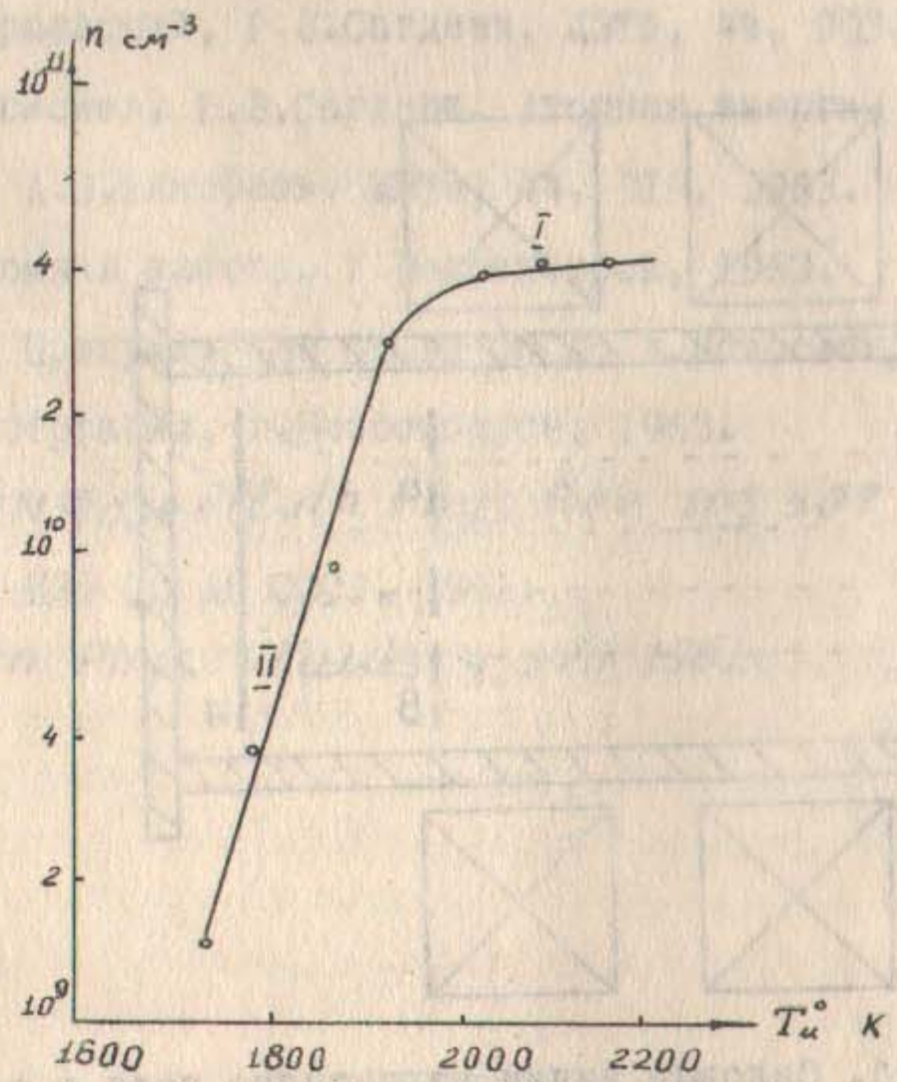
Рис.3. Зависимость плотности на оси от температуры ионизатора.
