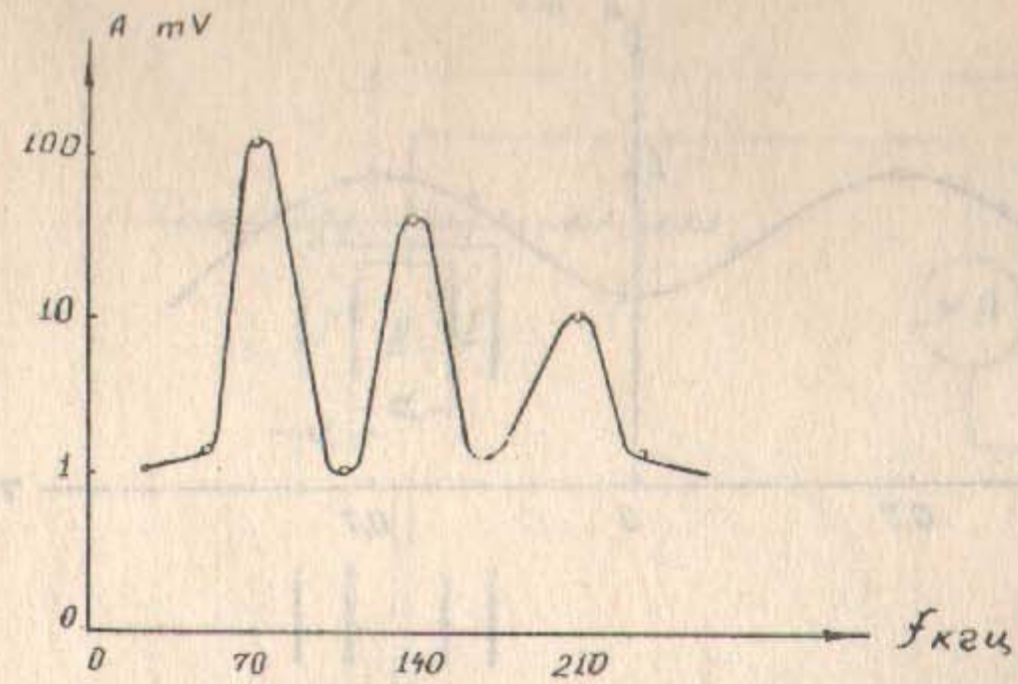
Рис.4. Спектр колебаний. n = 3 \cdot 10^{10} \text{ cm}^{-3} , H = 1000 эрстед.
