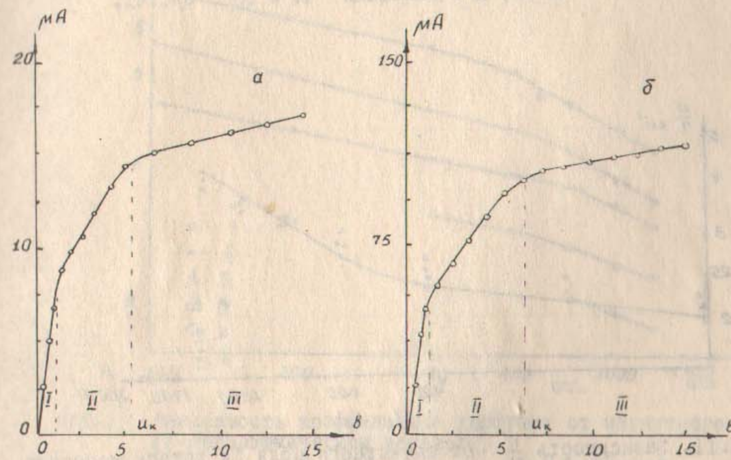
Рис.9. Вольт-амперная характеристика колец. H = 1000 эрст. а. n = 2 \cdot 10^8 см ^{-3} ; б. n = 2 \cdot 10^{10} см ^{-3} .
