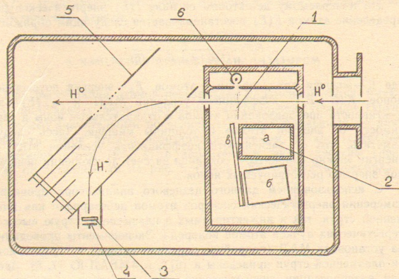
Рис. 3. Цезиевый анализатор атомов низких энергий:
