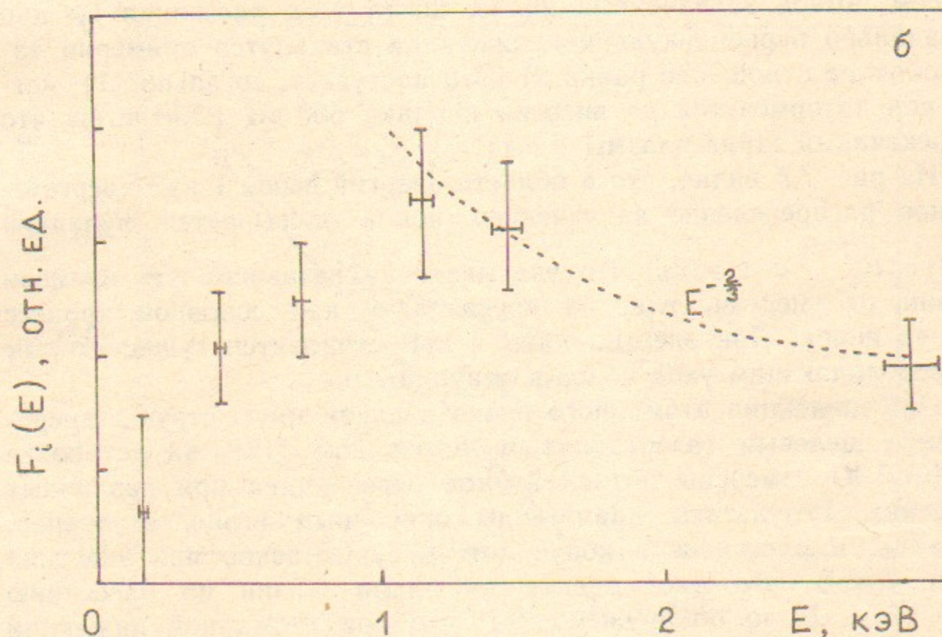
Рис. 7. Энергетические распределения атомов перезарядки (а) и захваченных ионов (б) инжектируемого в плазму пучка атомов водорода энергией 4 кэВ.
