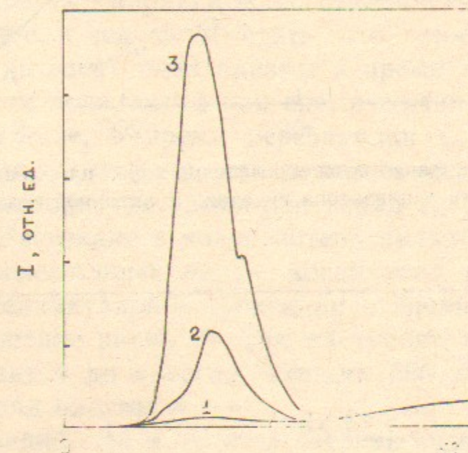
Рис. 4. Регистрируемый поток атомов перезарядки плазменной струи: 1 — напуск водорода в источник за \tau_3 = 2 мс до поджига разряда и в момент поджига вакуума в пробкотроне P \sim 5,5 \cdot 10^{-3} Па; 2 — \tau_3 = 3 мс, P \sim 10^{-1} Па; 3 — \tau_3 = 4 мс, P > 10^{-1} Па.
