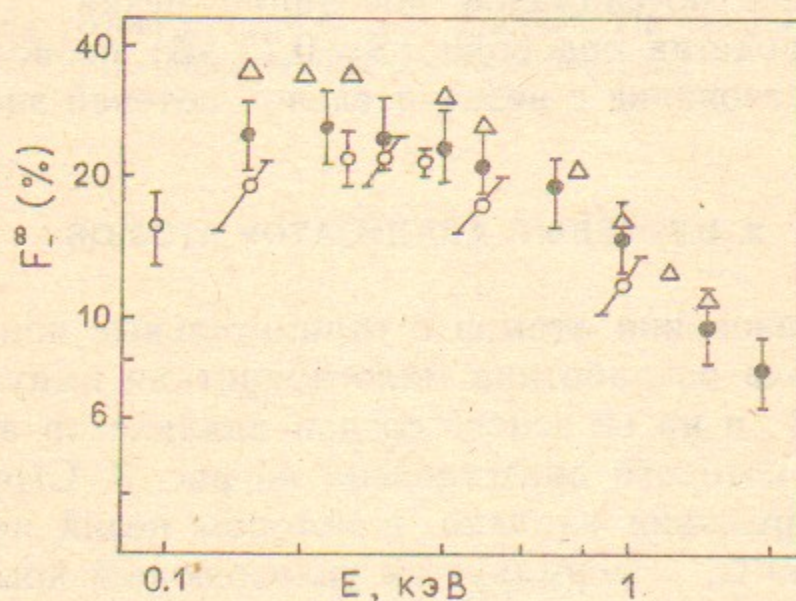
Рис. 2. Равновесный выход \text{H}^- в цезии F_{\infty} в зависимости от энергии: ● — [1]; ○ — [3]; △ — [4].
