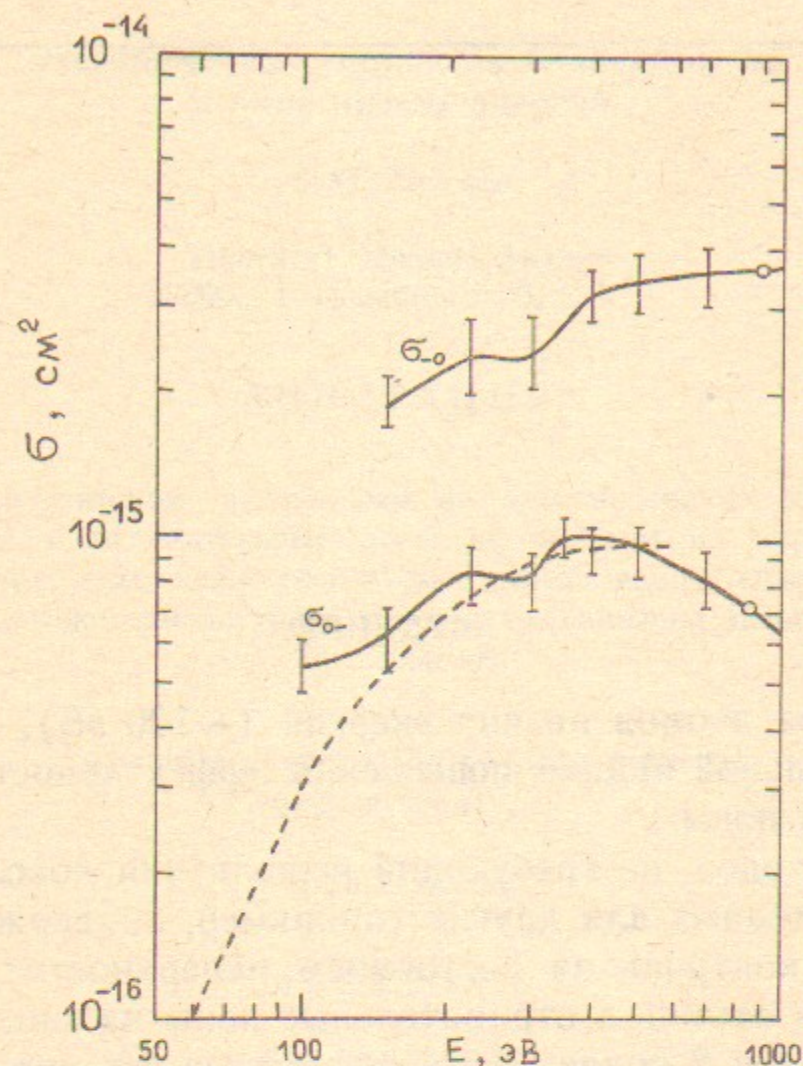
Рис. 1. Зависимость от энергии сечений потери электрона \sigma_{0-} для \text{H}^0 и захвата электрона \sigma_{00} для \text{H}^- . Сплошная кривая — экспериментальные результаты [1]; штриховая — расчетные [2].
