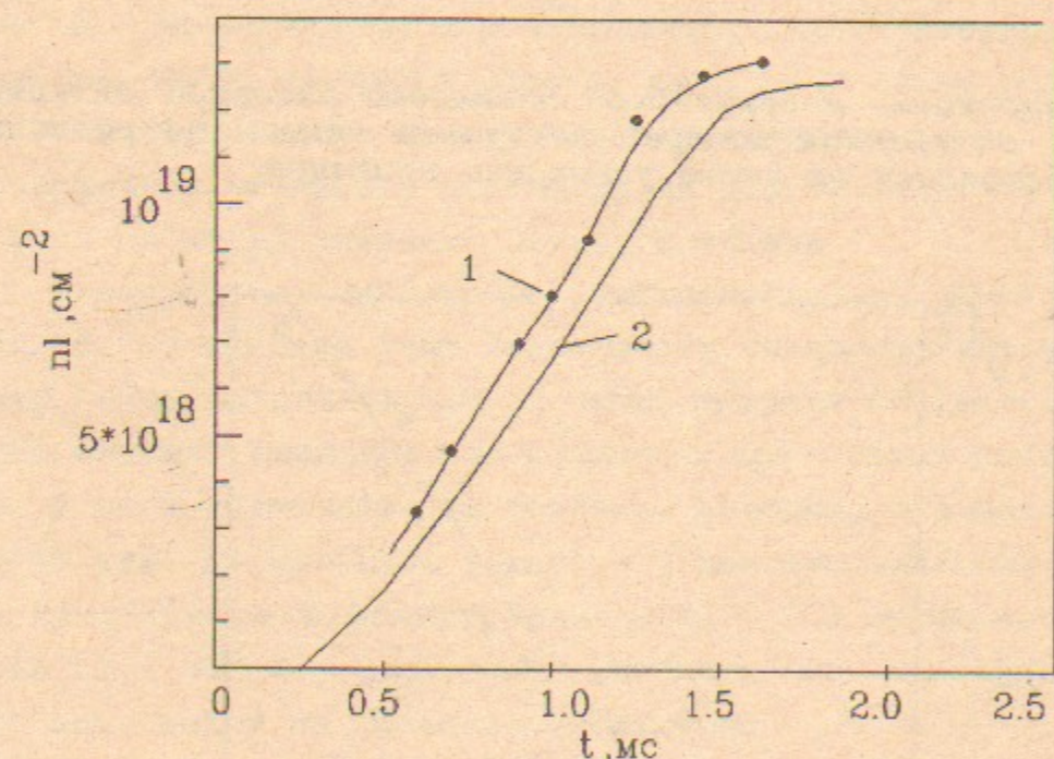
Рис. 26. Зависимость продольного n_1 от времени при давлении водорода в клапане 15 атм: 1 - вычислено по измерениям плотности поперёк вакуумной камеры; 2 - измерено интерферометром вдоль вакуумной камеры.
