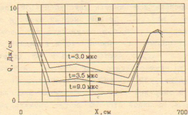
Рис. 22. Эксперимент с двумя сгустками плотной плазмы: а) распределение атомарной плотности водорода по длине установки при задержке срабатывания клапанов 1.6 мс (клапаны расположены на x = 12 см и 580 см); б) распределение диамагнетизма плазмы по длине установки (длительность пучка 3 мкс); в) удельное энергосодержание плазмы с учётом цены ионизации.
