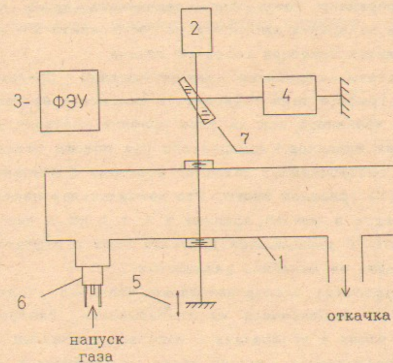
Рис. 23. Схема эксперимента по измерению параметров газового облака: 1 - вакуумная камера; 2 - He-Ne лазер с длиной волны 0,6328 \text{ мкм} ; 3 - детектор; 4 - система установки начальной фазы; 5 - система импульсной калибровки интерферометра; 6 - сборка импульсных клапанов.
