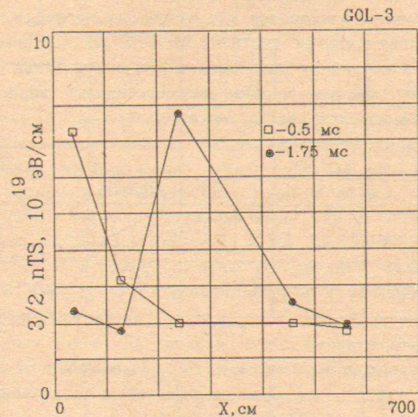
Рис. 7. Распределение поперечного давления плазмы (nT) по длине установки при различных длинах газового облака.
