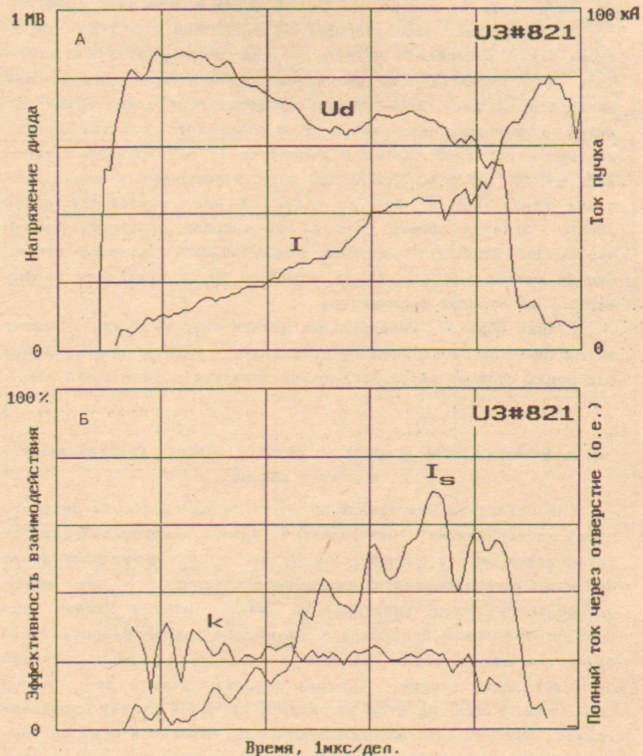
Рис. 16. Зависимость эффективности взаимодействия пучка с плазмой k от времени, определённая с помощью анализатора энергетического спектра пучка. Вверху: напряжение на диоде и ток пучка, внизу: эффективность взаимодействия и суммарный ток в анализатор.
