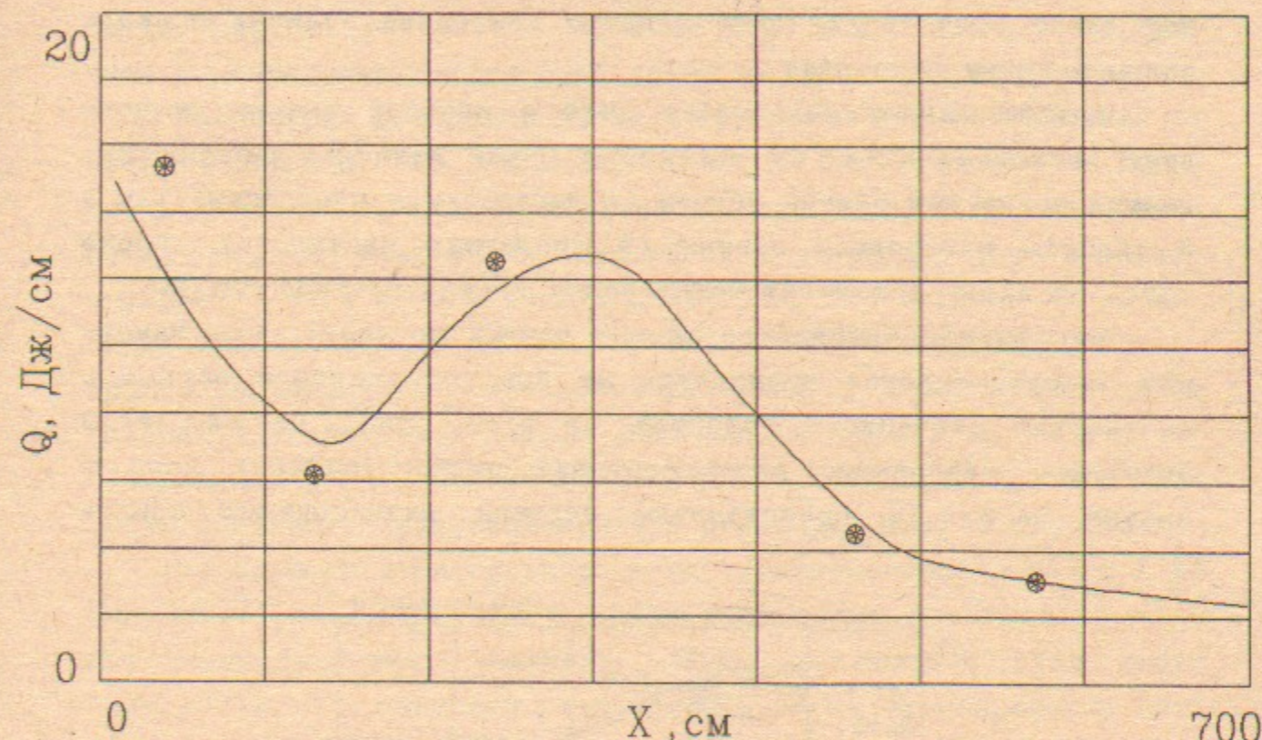
Рис. 17. Распределение удельного энергосодержания плазмы по длине установки с учётом цены ионизации при задержке срабатывания клапана 1.75 мс. Точки - измеренный диамагнетизм плазмы, сплошная линия - расчёт по модельной функции распределения.
