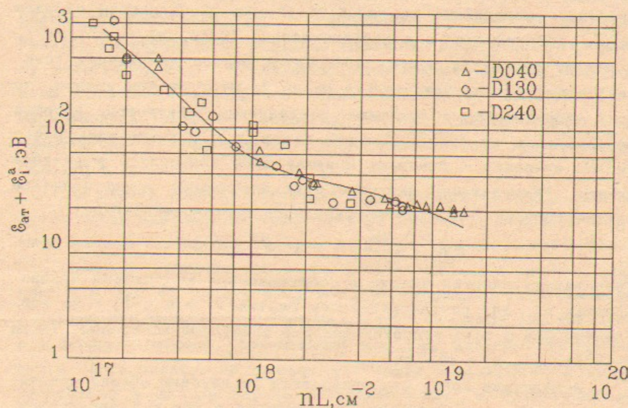
Рис. 14. Зависимость средней энергии, приходящейся на один атом водорода в облаке, переданной к моменту 3.2 мкс, от глубины облака с учётом цены ионизации. Точки соответствуют измерениям различными диамагнитными зондами; линия - расчёт характера энергосвечения от модельной функции распределения электронного потока.
