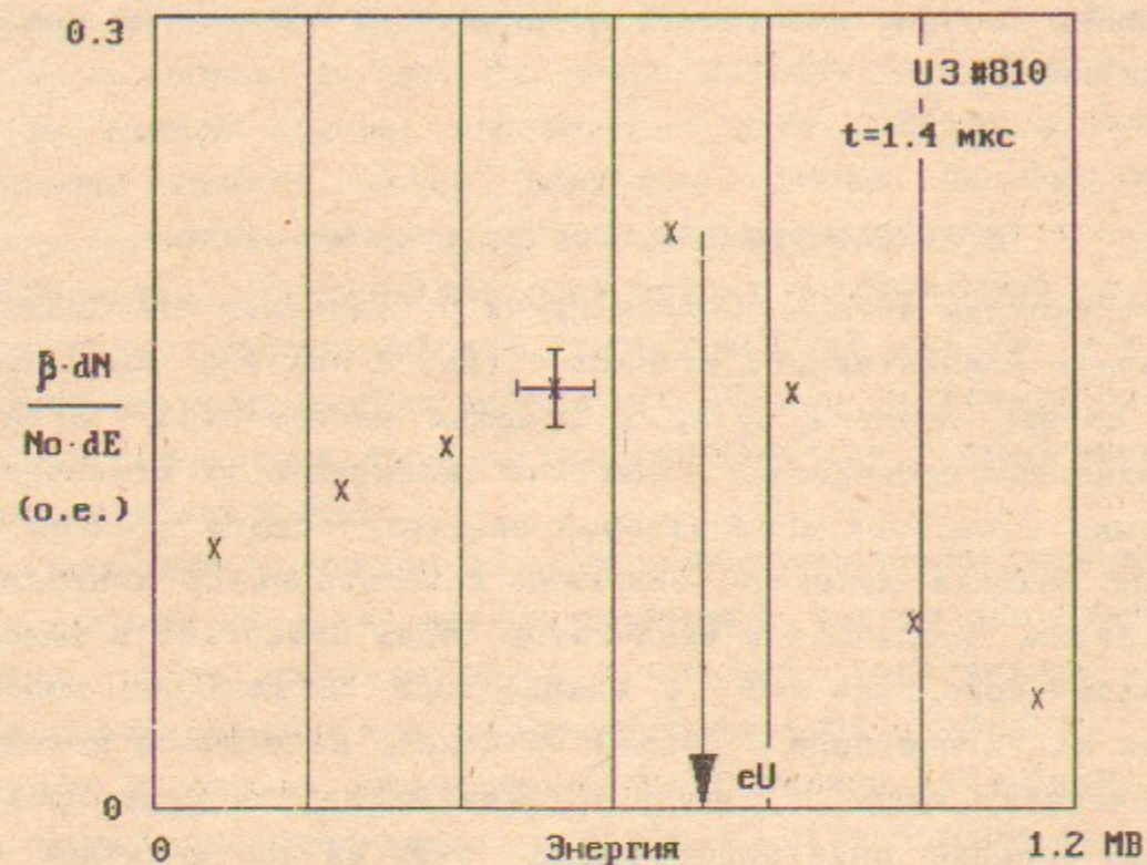
Рис. 15. Типичная форма энергетического спектра пучка после прохождения через плазму с n = 5 \cdot 10^{14} \text{ см}^{-3} на однородном участке. Стрелкой показана величина, соответствующая eU_d в этот момент времени (1.4 мкс от начала инжекции).
