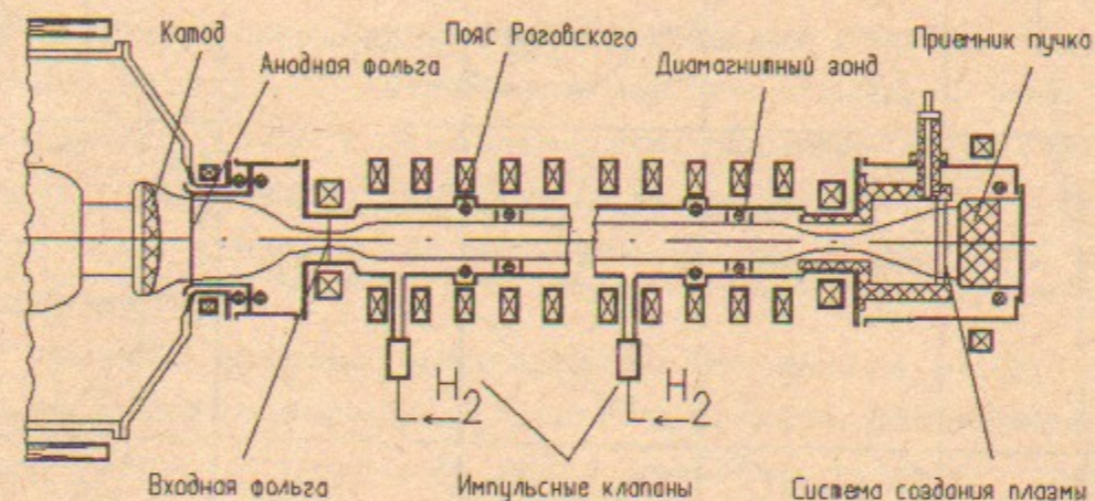
Рис. 1. Схема эксперимента.
