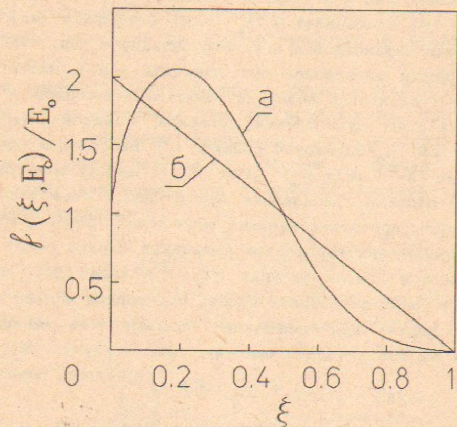
Рис. 28. Функция поглощения энергии в водородной мишени при изотропном падении на неё электронов с энергией E_0 . а) аппроксимация по формуле (П4) точного решения, полученного многошаговым методом; б) вычисления по простой модели (П3).
