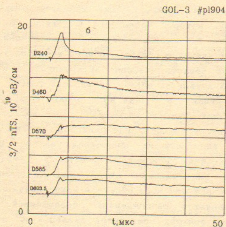
Рис. 21. а) распределение атомарной плотности водорода по длине установки при задержке срабатывания клапана 1.6 мс (клапан расположен в конце установки на x = 575 см) б) диамагнетизм плазмы в разных точках по длине плазменного столба.
