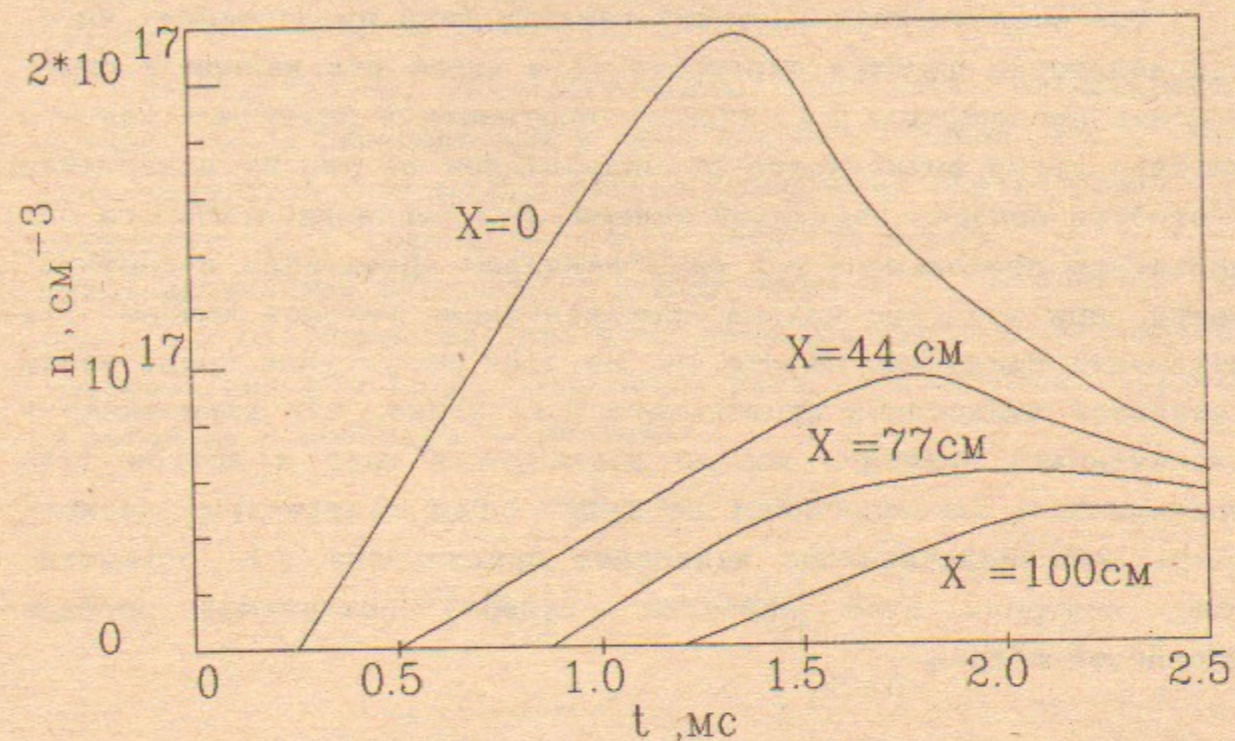
Рис. 24. Зависимость молекулярной плотности водорода от времени, измеренная поперёк вакуумной камеры на различных расстояниях от места установки клапанов.
