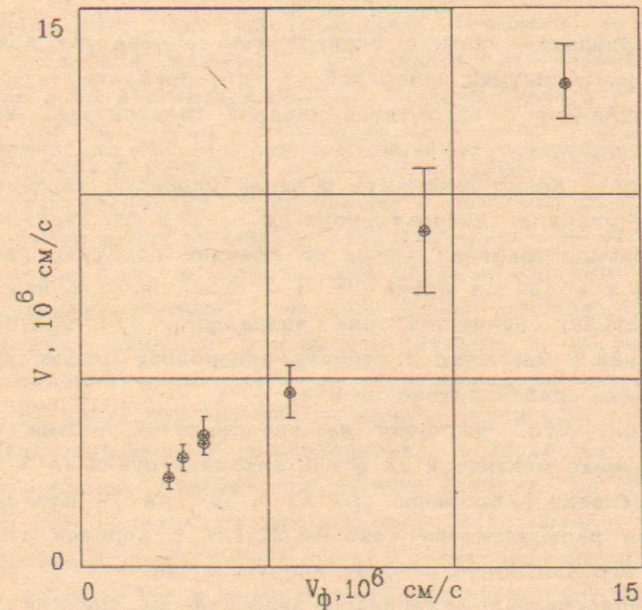
Рис. 20. Зависимость скорости волны v , вычисленной по времени появления всплеска на диамагнитных сигналах от скорости, полученной по теории ударных волн v_\phi .
