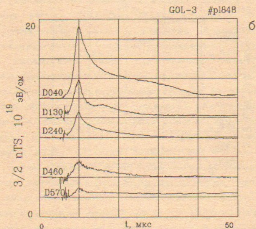
Рис. 6. а) распределение атомарной плотности водорода по длине установки при задержке инъекции пучка относительно срабатывания клапана 0.5 мс; б) диамагнетизм плазмы в разных точках по длине плазменного столба.
