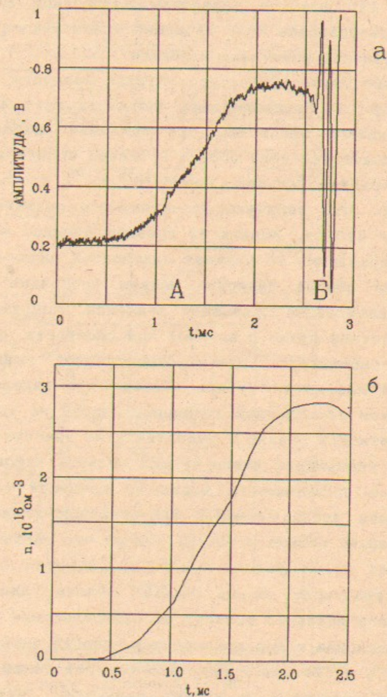
Рис. 4. а) интерферограмма на длине волны 0.63 мкм, измеренная поперёк вакуумной камеры на расстоянии 44 см от места установки клапана; б) зависимость плотности молекулярного водорода от времени.
