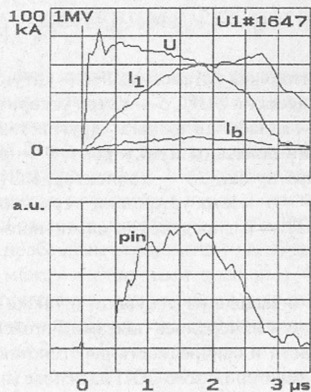
Рис.2. Вверху: U — напряжение на диоде ускорителя, I_1 — ток инжектируемого в ловушку пучка, I_b — ток пучка на выходе из ловушки. Мишень — 30 мкм Та в середине ловушки. Внизу — сигнал pin-диола.
