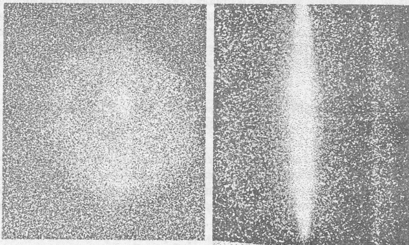
Рис. 4. Снимки мишени полученные рентгеновским ЭОП. Длительность экспозиции 0.3 мкс. Справа приведен снимок полученный через боковое окно, на котором более слабое изображение соответствует отражению рентгеновского излучения от боковой поверхности окна.
