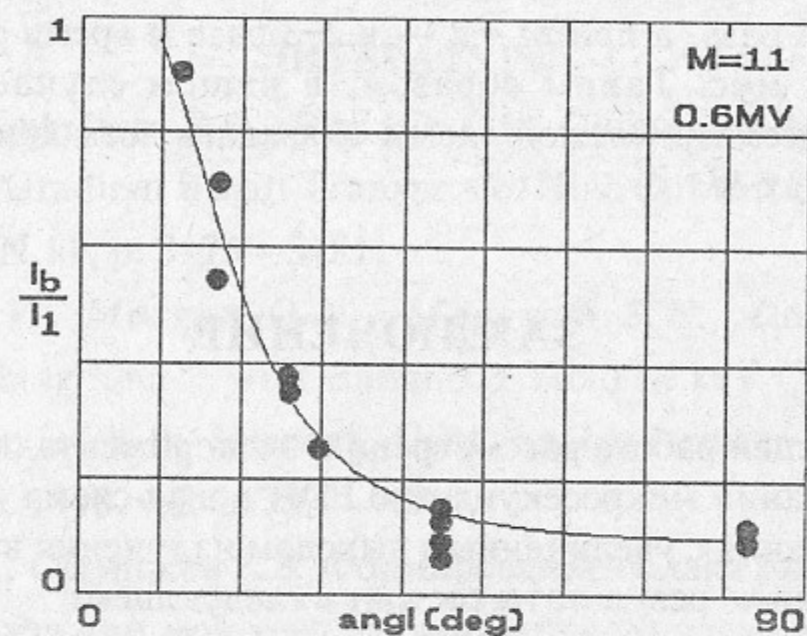
Рис. 7. Доля тока пучка, проходящего на коллектор в зависимости от среднеквадратичного угла рассеяния электронов пучка в мишени фольге. Точки — результаты измерений, сплошная линия — расчетный коэффициент прохождения при однократном рассеянии в фольге. Энергия электронов пучка 0.6 МэВ.
