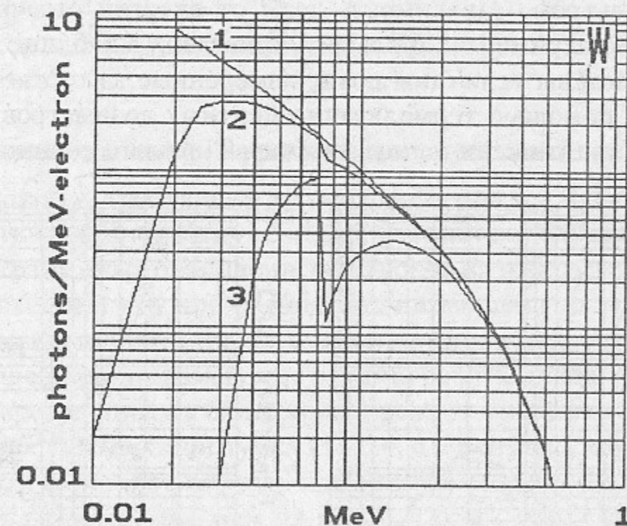
Рис. 5. Спектральный выход тормозного излучения из вольфрамовой мишени: 1 — без учета самопоглощения; 2, 3 — эффективная толщина мишени 15 мкм и 150 мкм, соответственно. Энергия электронов 0.6 МэВ.
