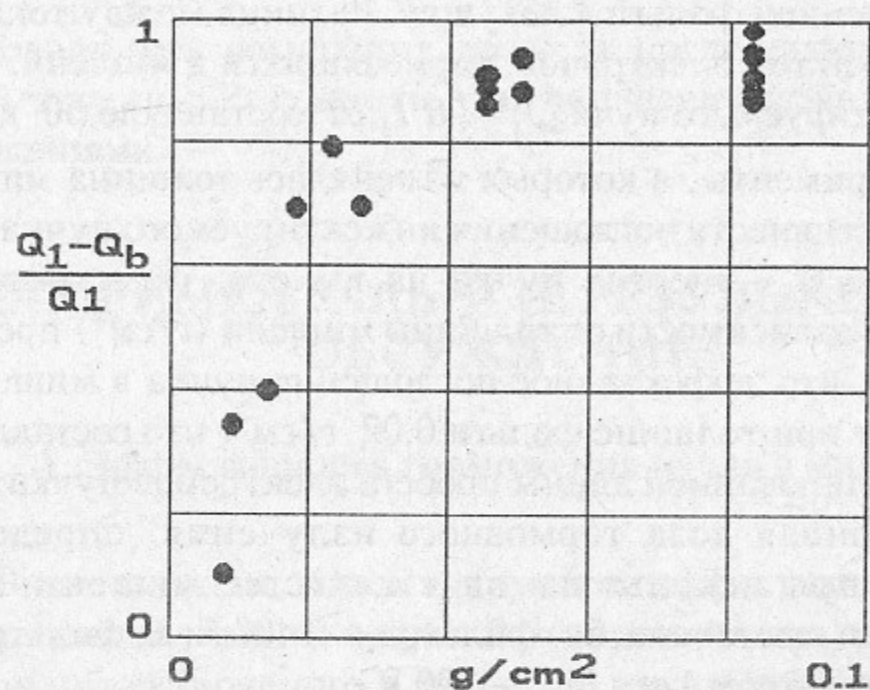
Рис. 3. Зависимость эффективности поглощения инжектируемого пучка в мишени от толщины мишени (Ta, Ti, Al).
