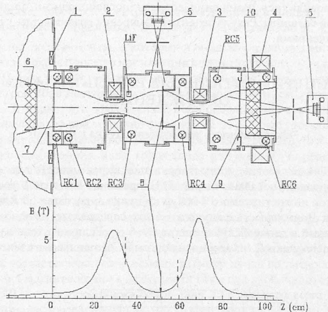
Рис. 1. Схема экспериментальной установки: 1–4 — катушки магнитного поля, 5 — рентгеновский ЭОП, 6 — катод ускорителя, 7 — анодная фольга, 8 — мишенная фольга (другие возможные места установки мишени показаны пунктиром), 9 — разделительная фольга коллектора пучка, 10 — коллектор, RC1–RC6 — пояса Роговского, "LiF" — место установки термолюминесцентных дозиметров. Внизу — распределение магнитного поля вдоль оси установки.
