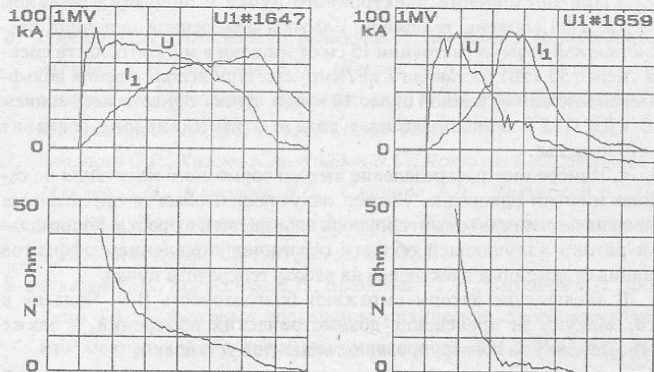
Рис. 8. Влияние положения мишени на работу диода ускорителя. Слева — пробочное отношение H_{\max}/H_t=8 , справа H_{\max}/H_t=2 . Внизу показано изменение импеданса диода во времени.
