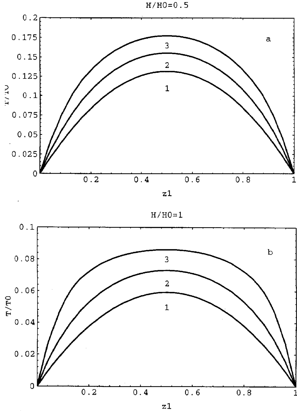
Рис. 4: Зависимость амплитуды расщепления фотона от энергии одного из конечных фотонов ( z_1 = \omega_1/\omega ) для H = H_0/2 (рисунок а) и H = H_0 (рисунок б) для разных энергий начального фотона: \omega/m = 0.1 (1), \omega/m = 1.5 (2) и \omega/m = 1.9 (3). Амплитуда T нормирована на амплитуду T_0 , формула (3.4).
