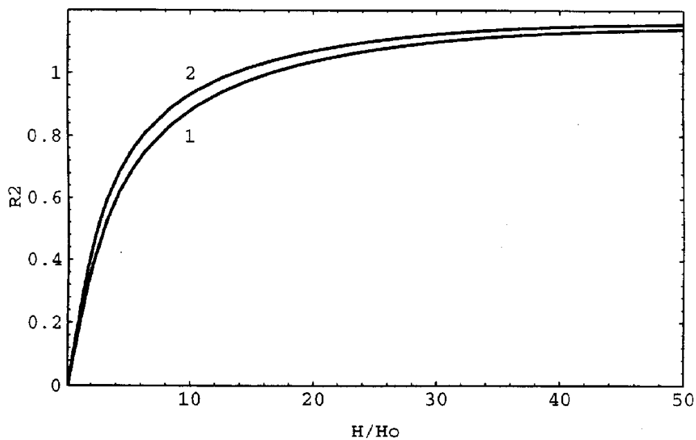
Рис. 2: Функция R_2 в зависимости от b = H/H_0 при разных значениях w = \omega\sigma/m : w = 0.1 – кривая 1 и w = 1.9 – кривая 2.
