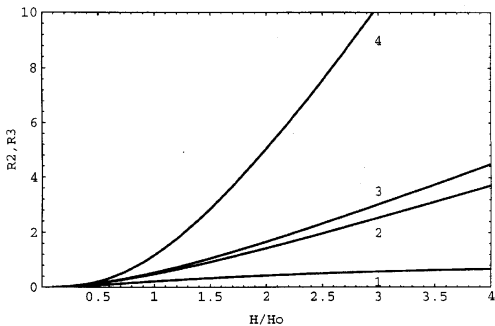
Рис. 3: Функция R_2 при w = 1.9 (кривая 1) и функция R_3 при w = 0.1 (кривая 2); при w = 1 (кривая 3) и при w = 1.9 (кривая 4) в зависимости от b = H/H_0 .
