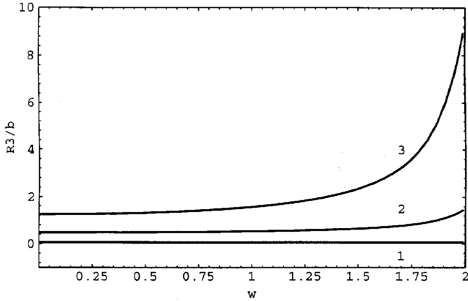
Рис. 1: Функция R_3/b в зависимости от w = \omega\sigma/m при разных значениях параметра b = H/H_0 : b = 0.1 – кривая 1; b = 1 – кривая 2; b = 30 – кривая 3.
