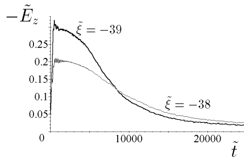
Рис. 4: Временная зависимость электрического поля на оси в точках \tilde{\xi} = -38 (максимум поля в начальный момент времени) и \tilde{\xi} = -39 (максимум поля при \tilde{t} \sim 2000 ).
