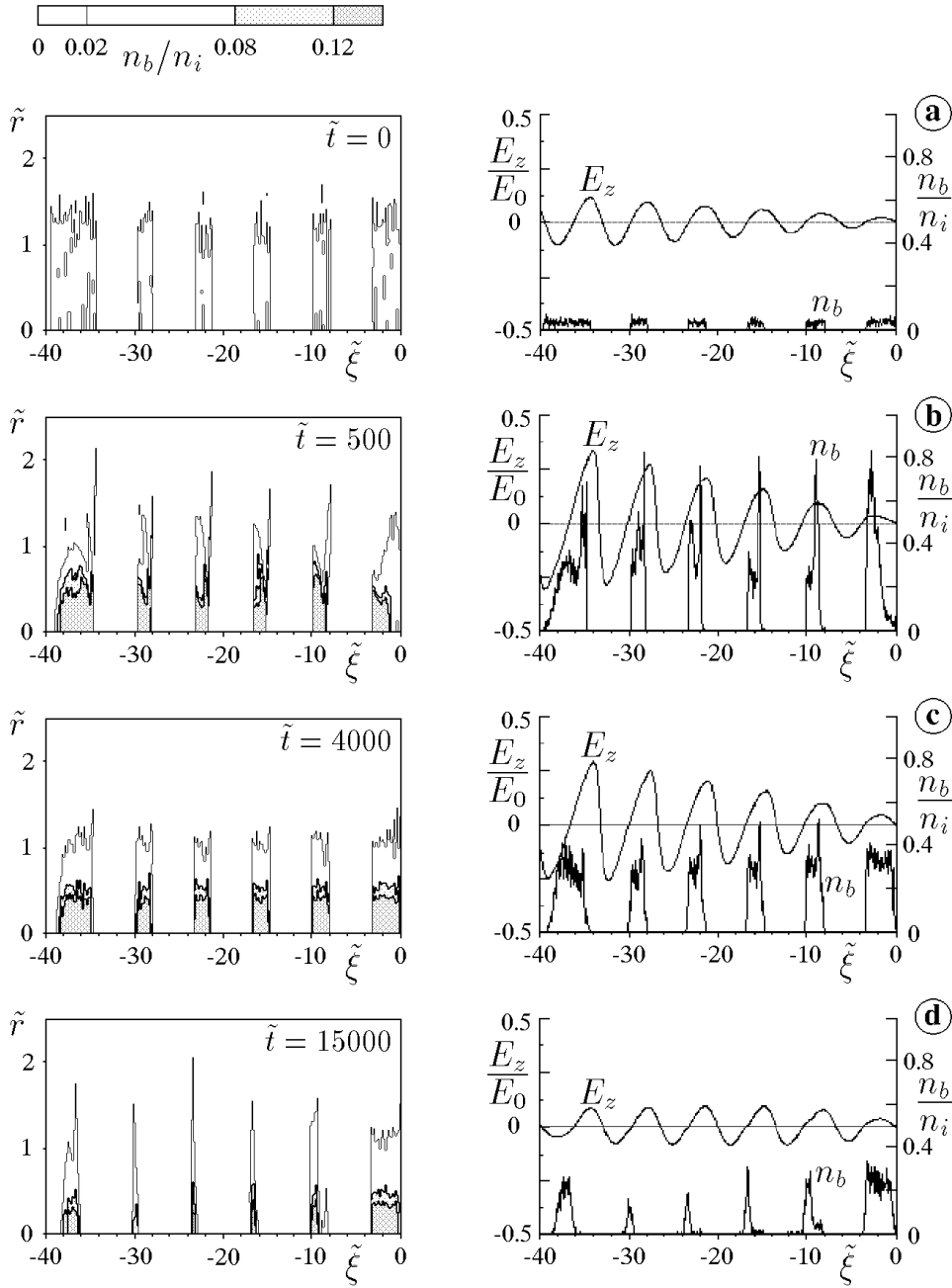
Рис. 2: Пространственное распределение плотности драйвера (слева; показаны линии постоянной плотности), электрическое поле и плотность драйвера на оси (справа) в различные моменты времени.
