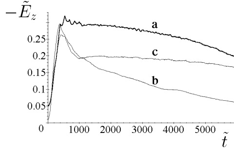
Рис. 10: Электрическое поле в месте оптимального расположения ускоряемых частиц для различных драйверов: (a) оптимизированный драйвер (19) с малым угловым разбросом, (b) драйвер (19) с угловым разбросом \Delta\alpha = \sqrt{2} \cdot 10^{-3} , (c) строго периодический драйвер (24) с малым угловым разбросом.
