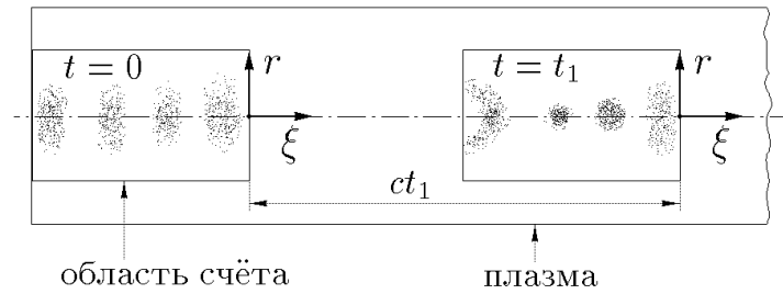
Рис. 1: Геометрия задачи.
