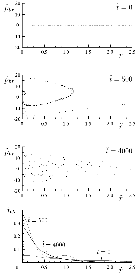
Рис. 3: Фазовые портреты драйвера в сечении \tilde{\xi} = -22.5 в различные моменты времени; соответствующие радиальные распределения плотности драйвера в том же сечении.
