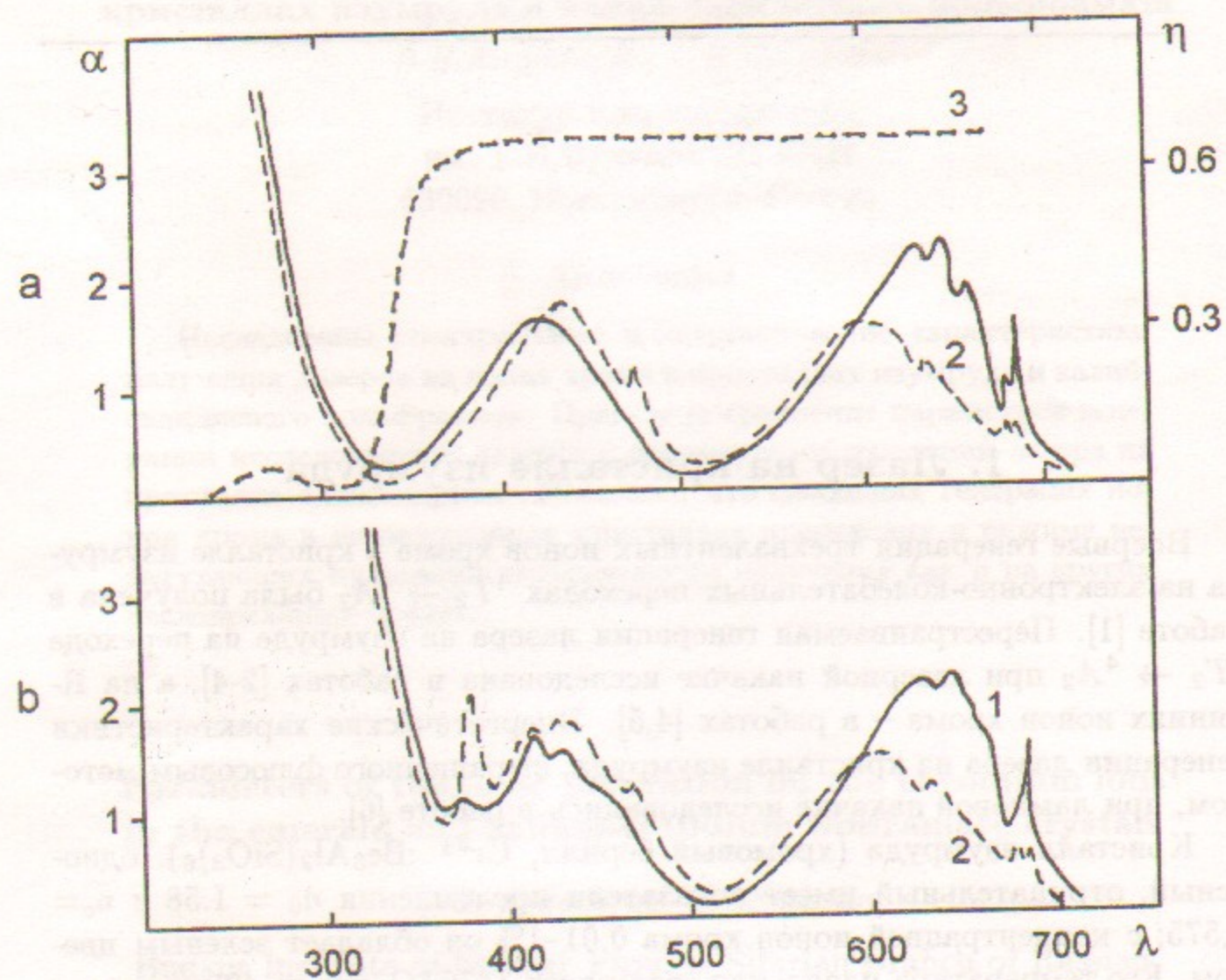
Рис. 1: Зависимости коэффициентов поглощения \alpha ( \text{см}^{-1} ) (1,2) и квантового выхода люминесценции \eta (нм) для флюсового (а) и гидротермального (б) изумрудов при T = 300 \text{ K} , 1 - E \parallel C , 2 - E \perp C .
