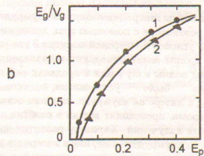
Рис. 4: a - зависимости удельных энергий генерации E_g/V_g (Дж·см ^{-3} ) (1,3) и пороговых энергий накачки E_t (2,4) лазеров на изумруде (1,2) и александрите (3,4) от коэффициента пропускания выходного зеркала резонатора T_2 , E_p = 0.4 кДж, L = 0.4 м, T = 70^{\circ}\text{C} ; b - зависимости удельных энергий генерации E_g/V_g (Дж·см ^{-3} ) лазеров на изумруде (1) и александрите (2) от энергии накачки E_p (кДж), L = 0.4 м, T = 70^{\circ}\text{C} .
