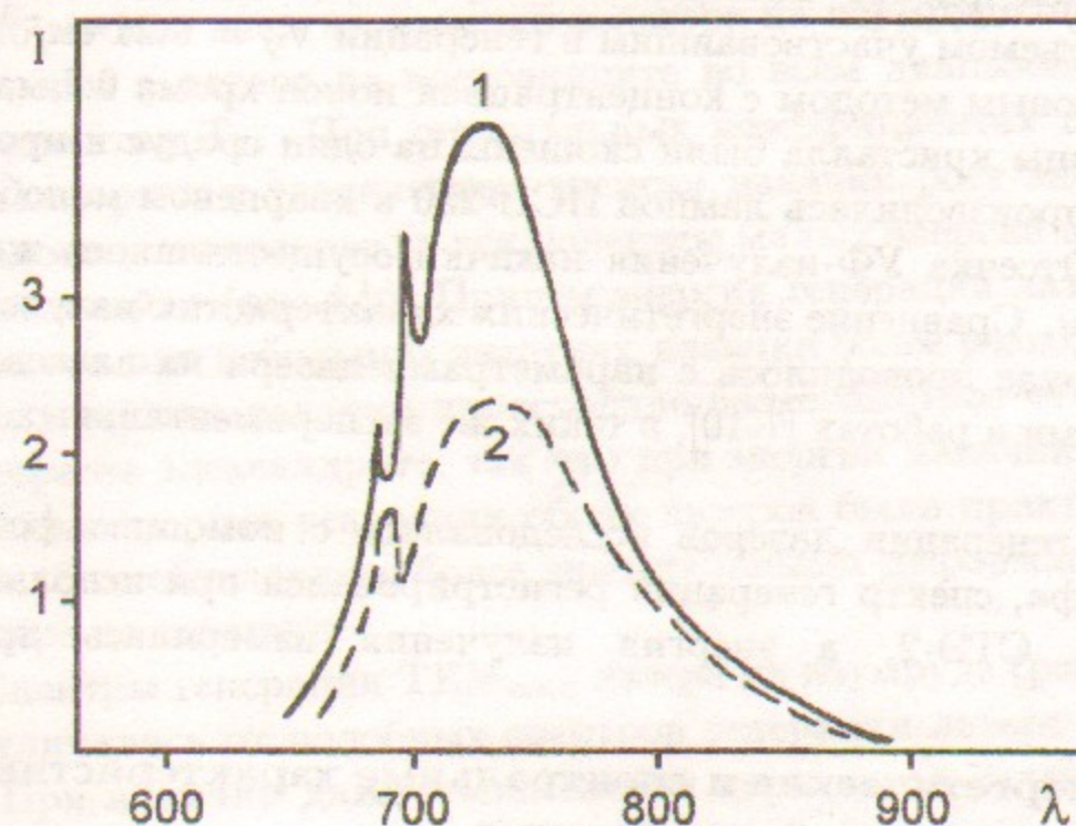
Рис. 2: Зависимости интенсивностей люминесценции I (отн.ед.) кристалла изумруда от длины волны \lambda (нм) при T = 300 \text{ K} , 1 - E \parallel C , 2 - E \perp C .
