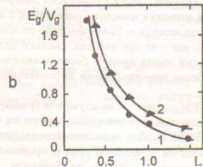
Рис. 3: a - зависимости удельных энергий генерации E_g/V_g (Дж·см ^{-3} ) (1,3) и пороговых энергий накачки E_t (кДж) (2,4) лазеров на изумруде (1,2) и александрите (3,4) от температуры кристалла T^{\circ}\text{C} , E_p = 0.4 кДж, L = 0.4 м; b - зависимости удельных энергий генерации E_g/V_g (Дж·см ^{-3} ) лазеров на изумруде (1) и александрите (2) от длины резонатора L (м), E_p = 0.4 кДж, T = 70^{\circ}\text{C} .
