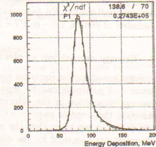
(d) Group 0.810–0.960 GeV
