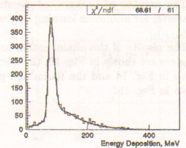
(d) \pi^- , 425 < E_\pi < 435 \text{ MeV}
