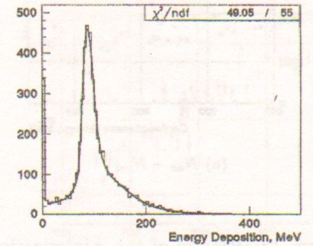
(b) \pi^- , 345 < E_\pi < 355 \text{ MeV}
