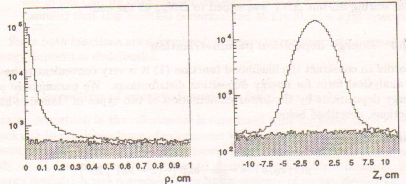
(b) Z -distribution
