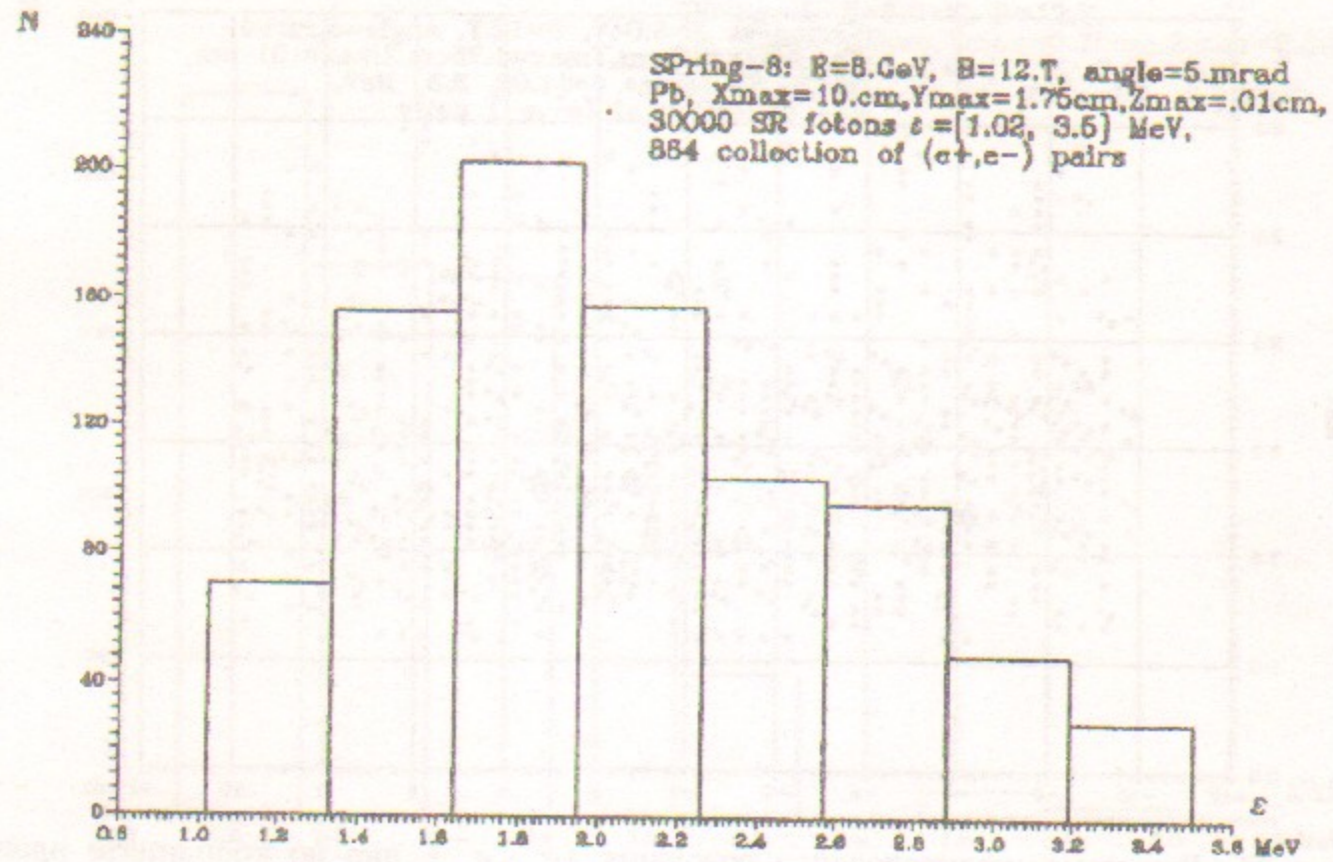
Рис. 33. Распределение рождения (e^+, e^-) пар по энергии исходных фотонов СИ.
