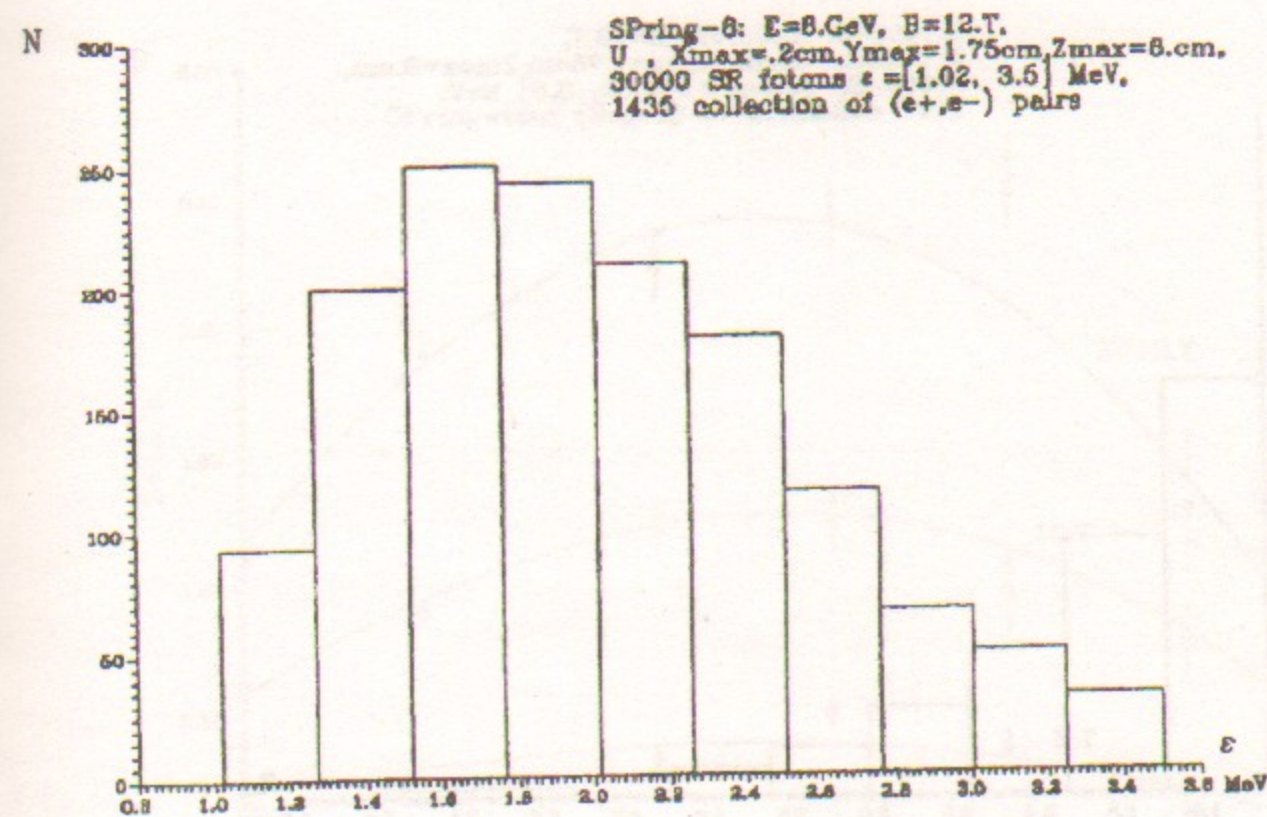
Рис. 20. Распределение рождения (e^+, e^-) пар в урановой мишени в функции энергии фотонов СИ.
