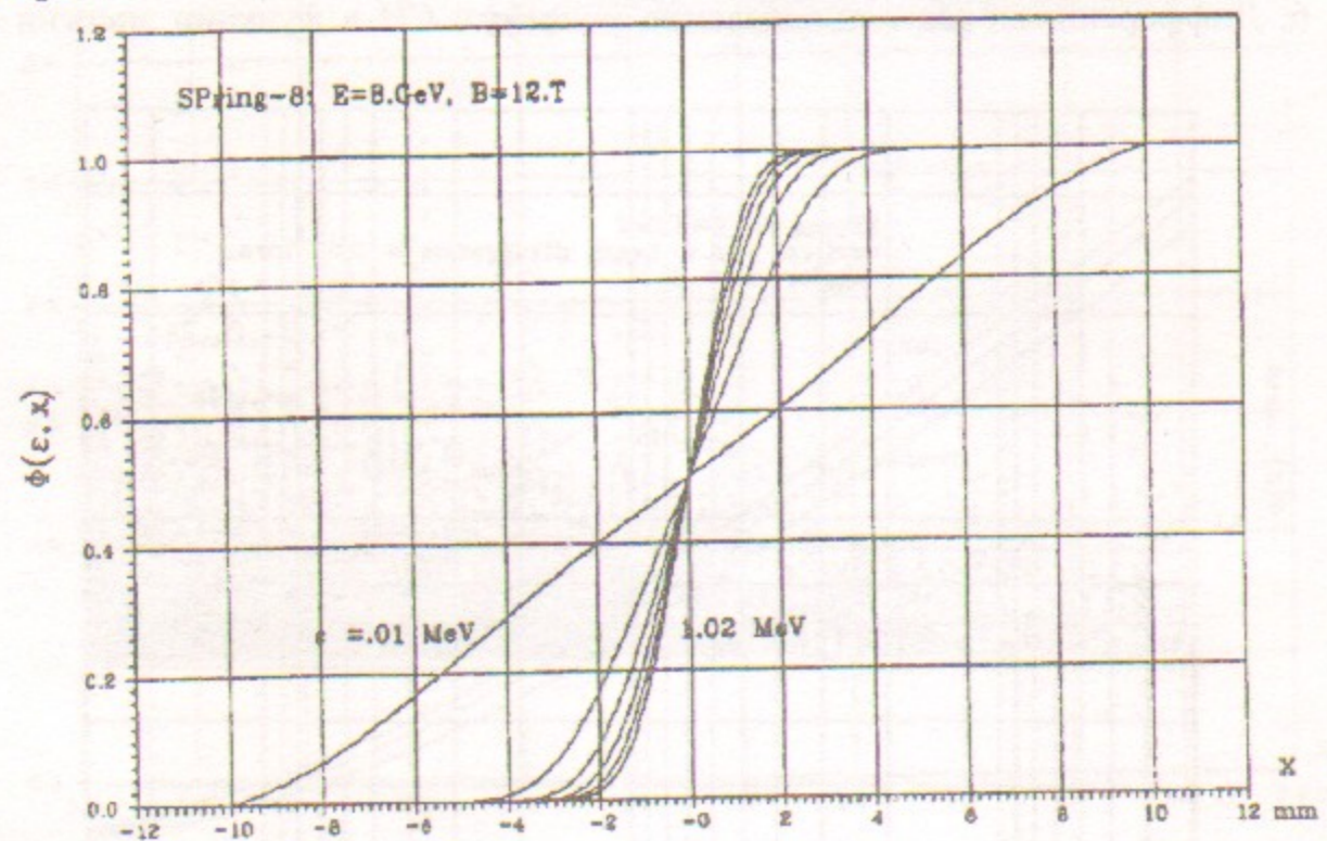
Рис. 9. Интегральное распределение мягкой части спектра фотонов СИ по вертикальной координате.
