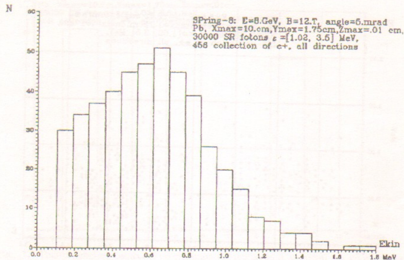
Рис. 41. Распределение эмиссии позитронов из наклонной мишени по кинетической энергии.
