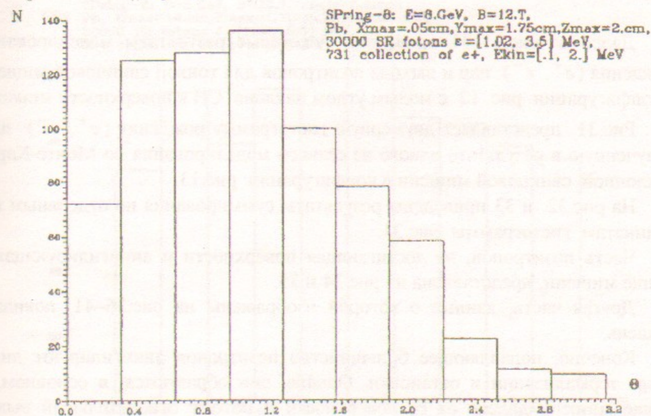
Рис. 29. Распределение позитронов по углу между направлением исходных фотонов СИ и лучем в точку остановки позитронов.
