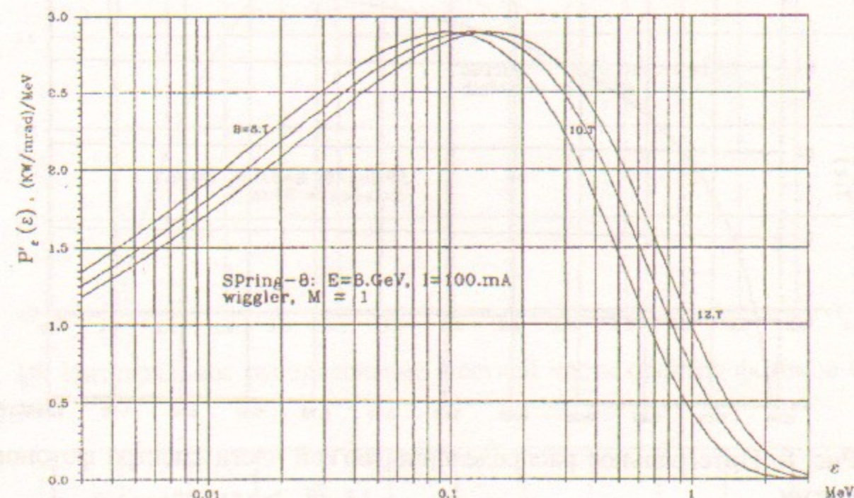
Рис. 6. Дифференциальное распределение мощности СИ в функции энергии фотонов.
