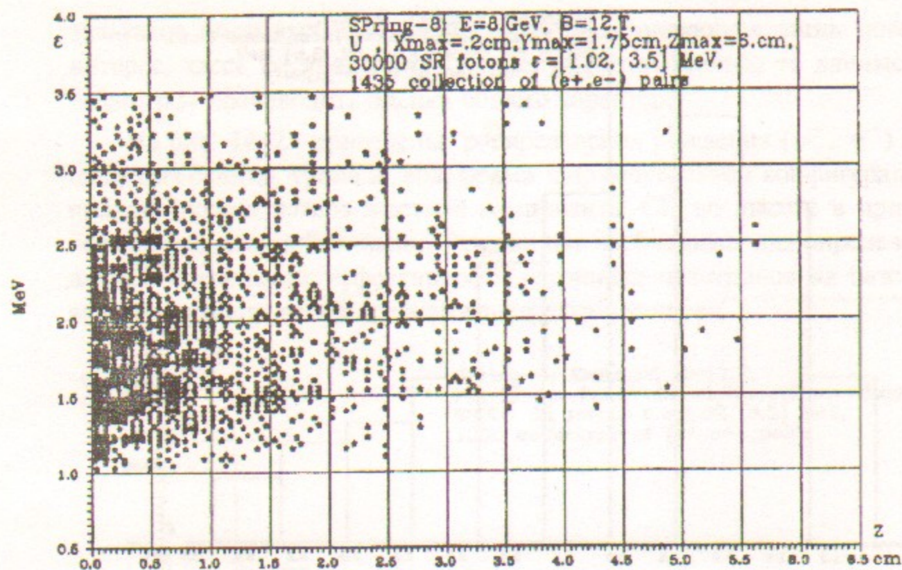
Рис. 18. Двумерное распределение рождения (e^+, e^-) пар в урановой мишени в функции расстояния от места входа СИ и энергии фотонов СИ.
