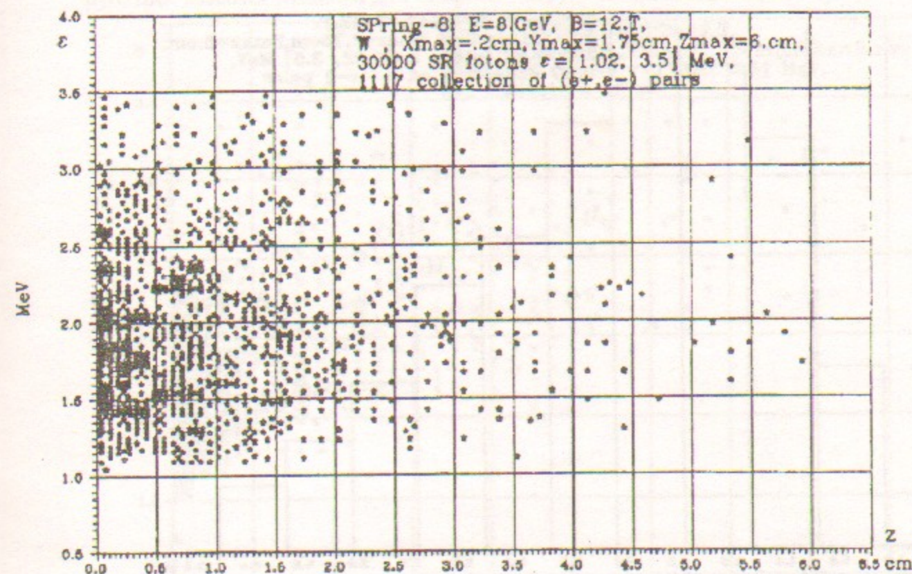
Рис. 21. Двумерное распределение рождения (e^+, e^-) пар в вольфрамовой мишени в функции расстояния от места входа СИ.
