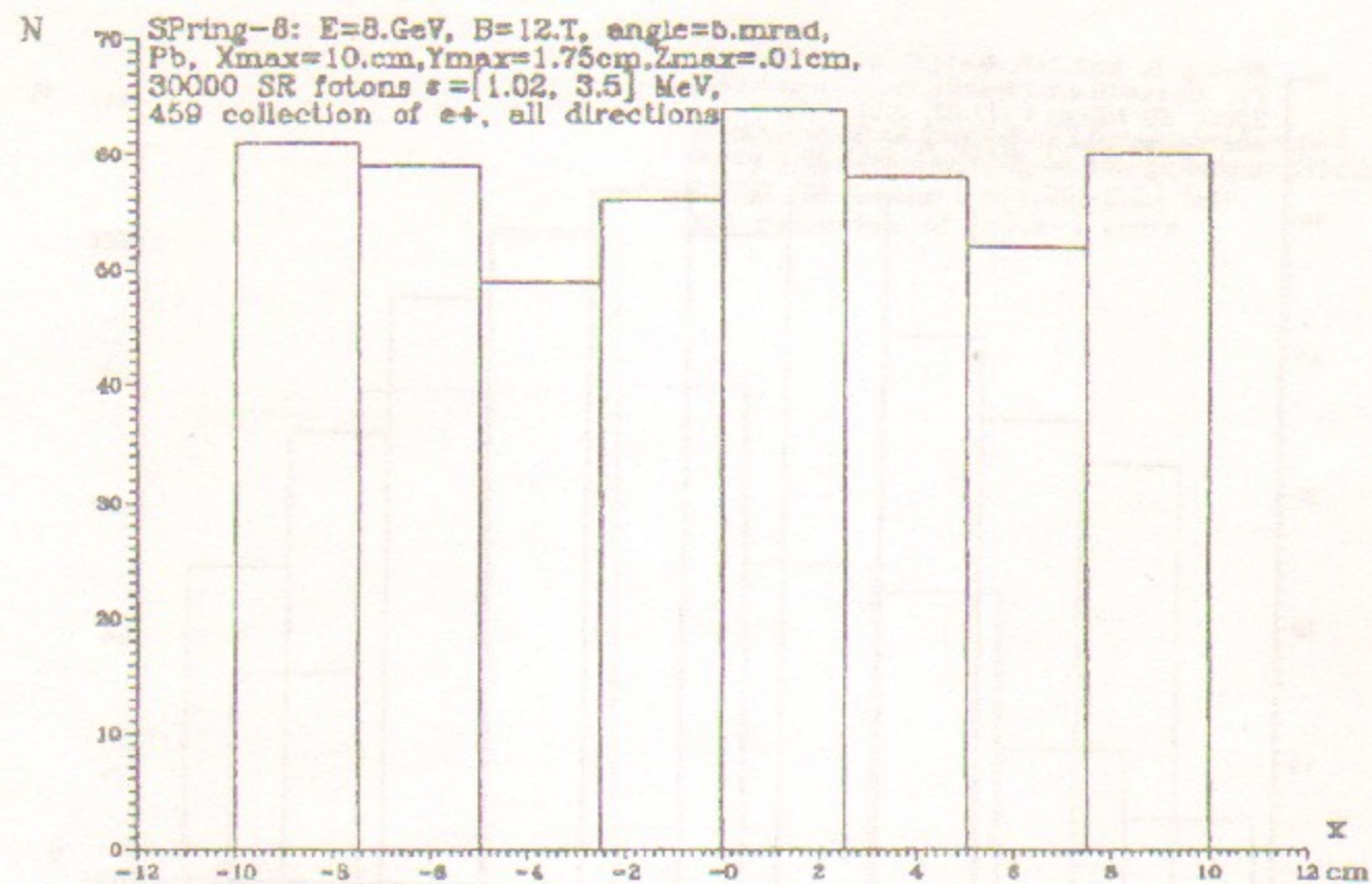
Рис. 37. Распределение эмиссии позитронов из наклонной мишени по координате вдоль поверхности наклонной мишени.
