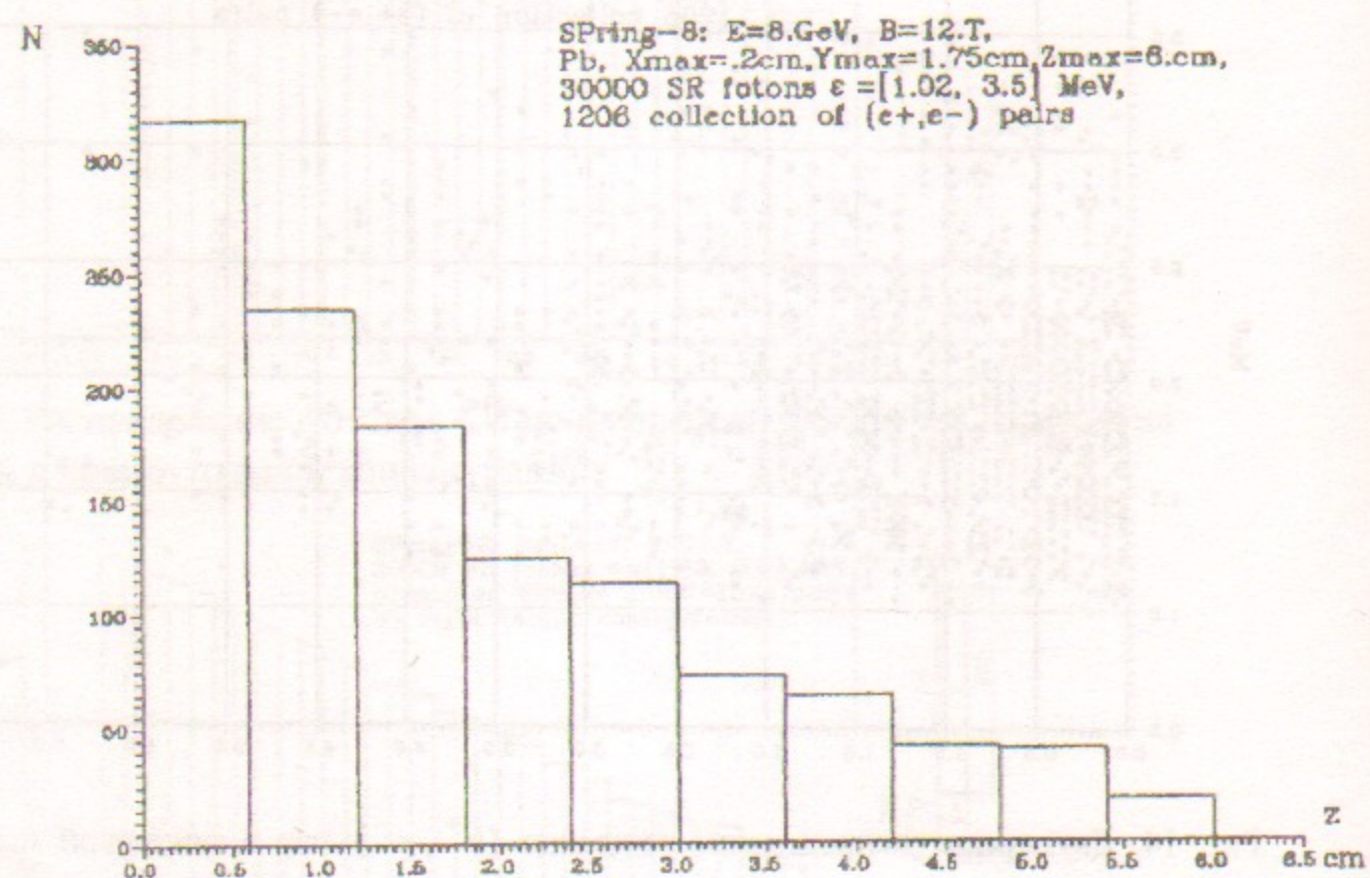
Рис. 15. Распределение рождения ( e^+ , e^- ) пар в свинцовой мишени в функции расстояния от места входа СИ.
