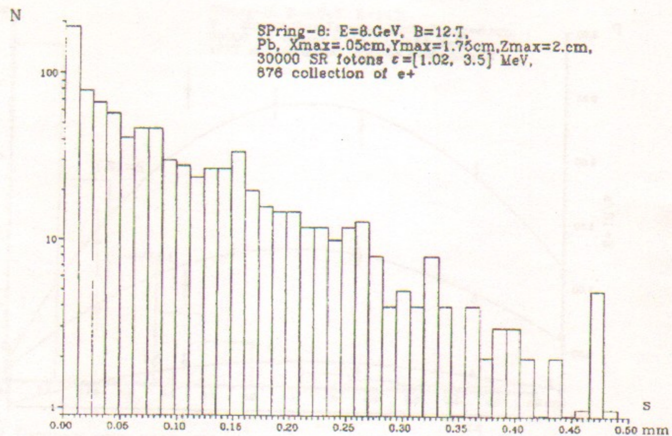
Рис. 26. Распределение позитронов по расстоянию от места рождения до остановки.
