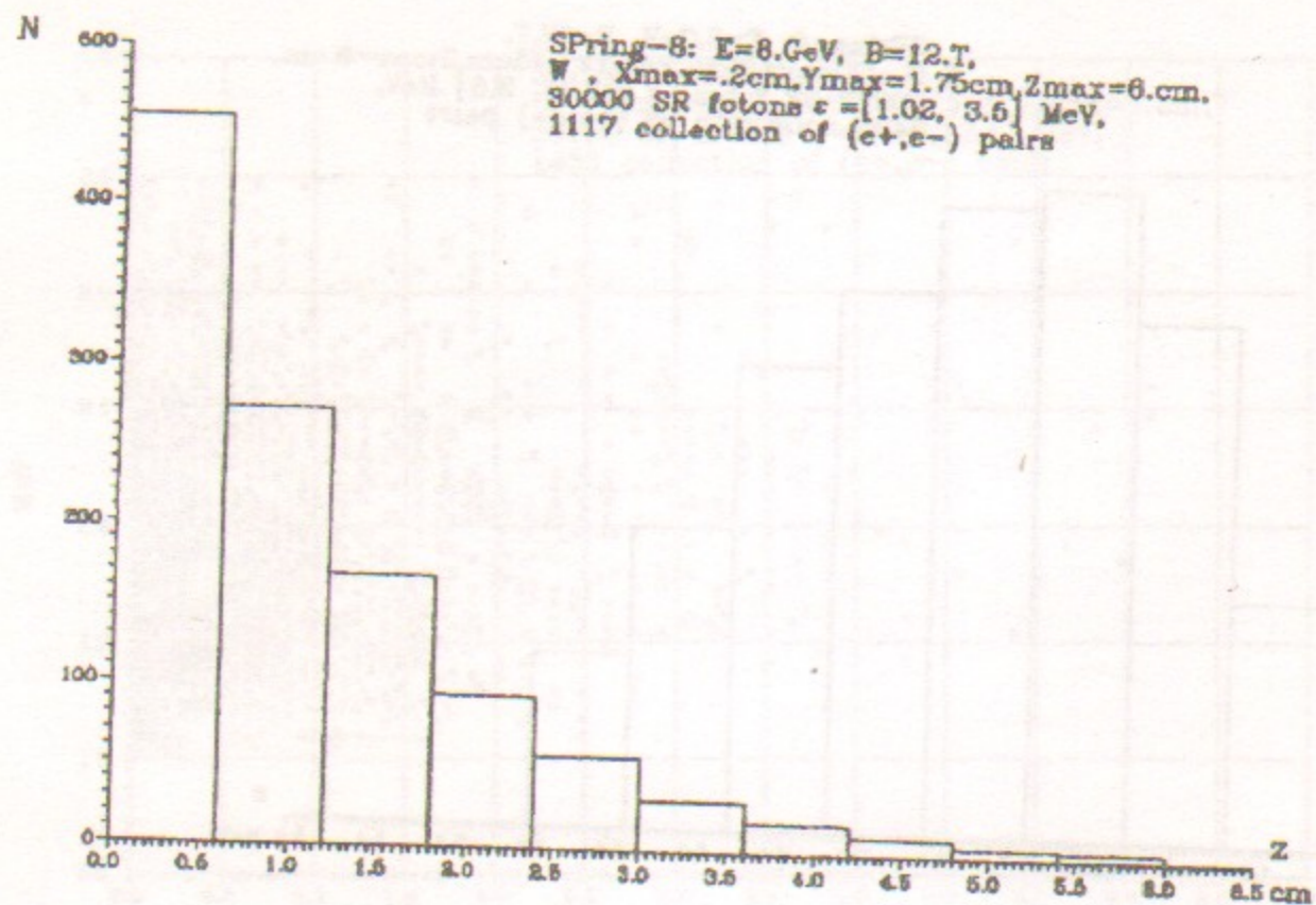
Рис. 22. Распределение рождения (e^+, e^-) пар в вольфрамовой мишени в функции расстояния от места входа СИ.
