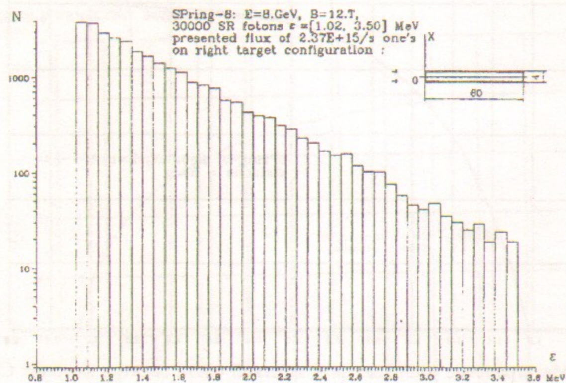
Рис. 12. Распределение фотонов СИ по их энергии для случая падения на мишень в прямоугольной конфигурации.
