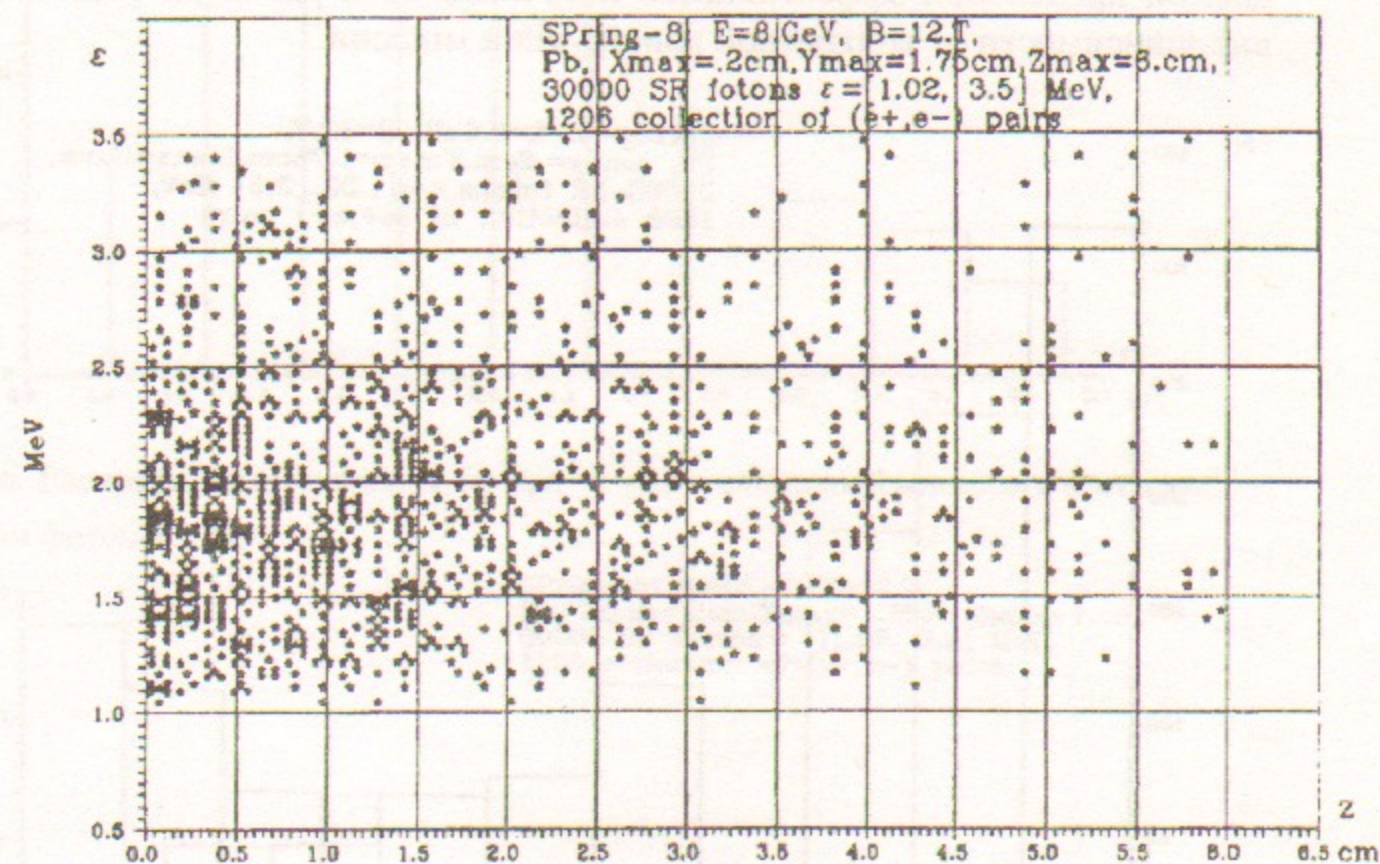
Рис. 14. Двумерное распределение рождения ( e^+ , e^- ) пар в свинцовой мишени в функции расстояния от места входа СИ и энергии фотонов СИ.
