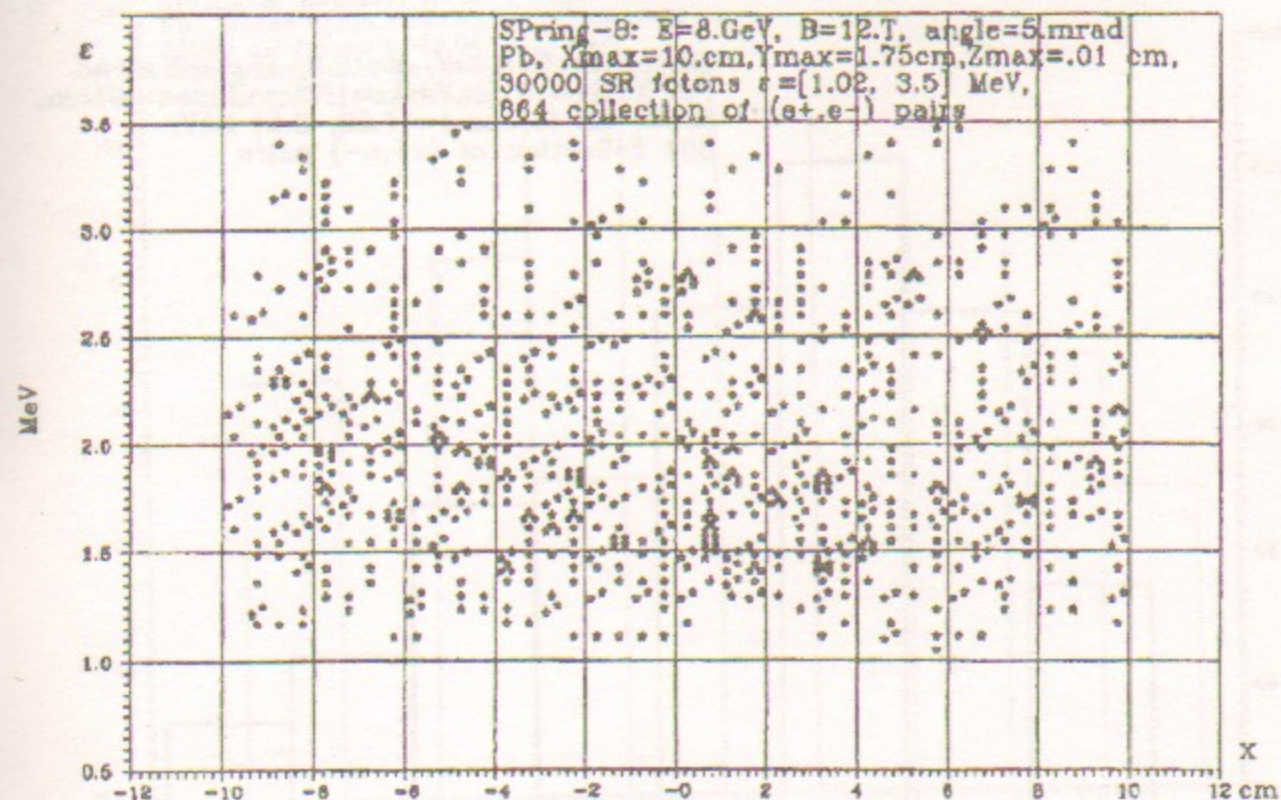
Рис. 31. Двумерное распределение рождения (e^+, e^-) пар по координате вдоль поверхности наклонной мишени и по энергии фотонов СИ.
