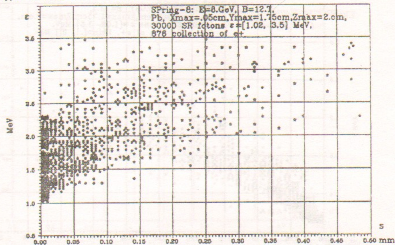
Рис. 25. Двумерное распределение позитронов по расстоянию от места рождения до остановки и по энергии фотонов СИ.
