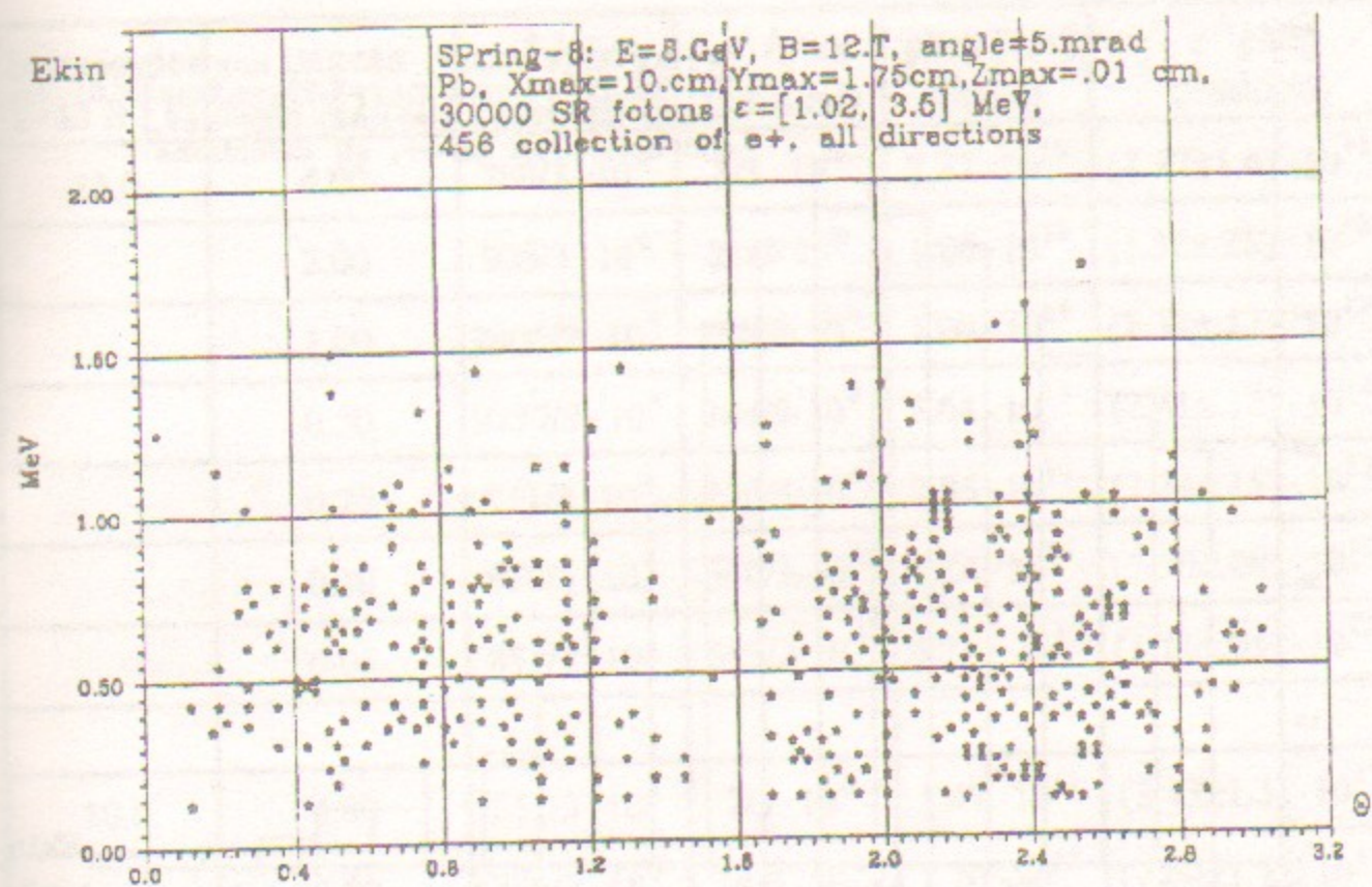
Рис. 39. Распределение эмиссии позитронов из наклонной мишени по кинетической энергии и по углу вылета.
