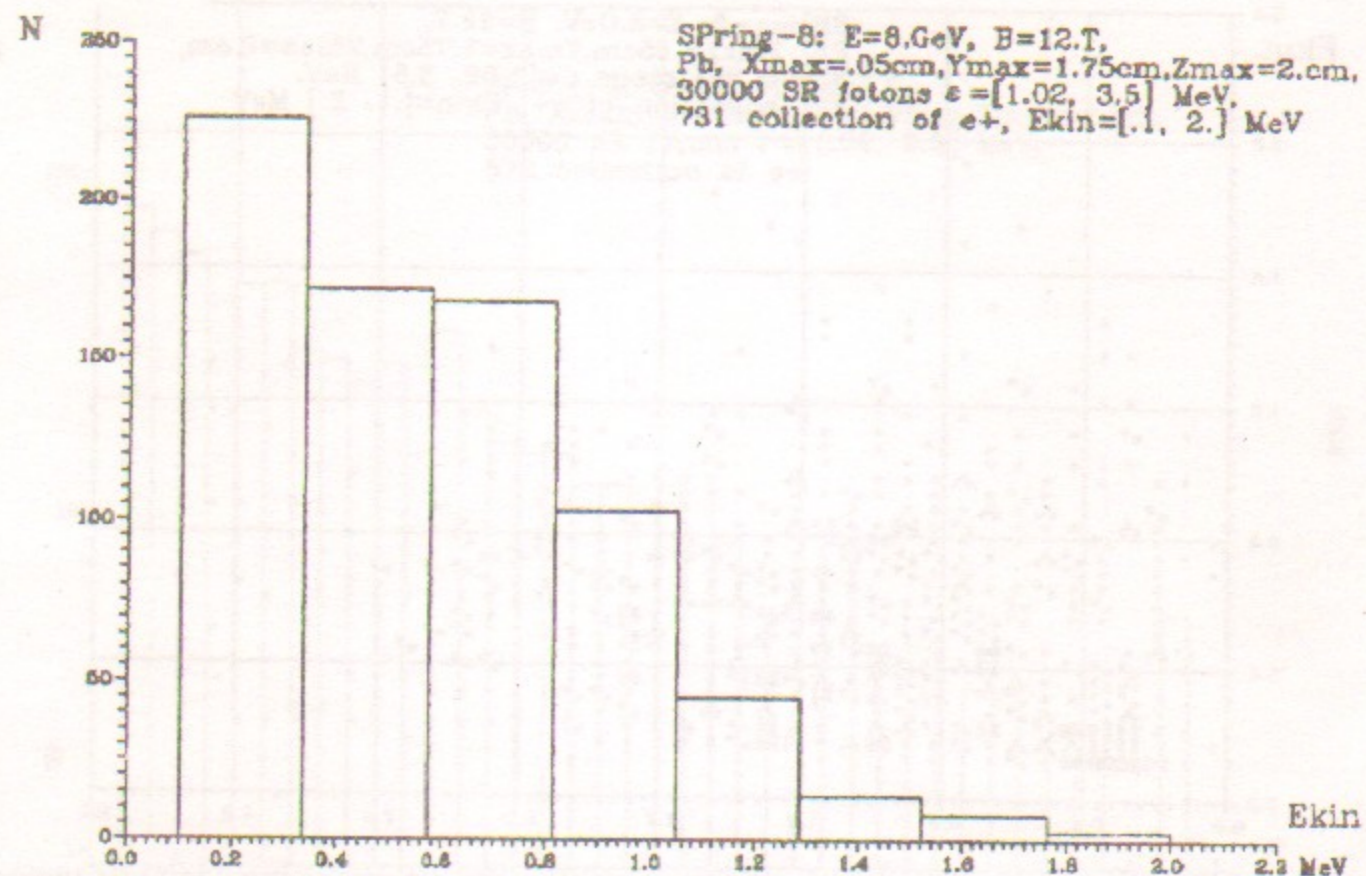
Рис. 30. Распределение позитронов по их кинетической энергии в момент рождения позитронов.
