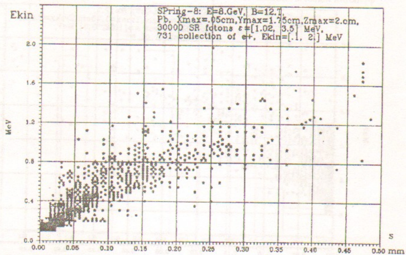
Рис. 27. Двумерное распределение позитронов по расстоянию от места рождения до остановки и по их кинетической энергии в момент рождения.
