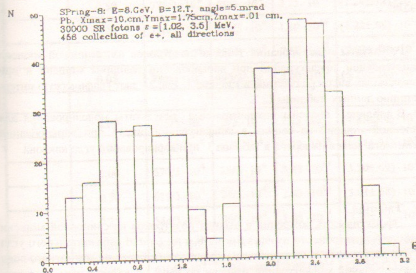
Рис. 40. Распределение эмиссии позитронов из наклонной мишени по углу вылета.
