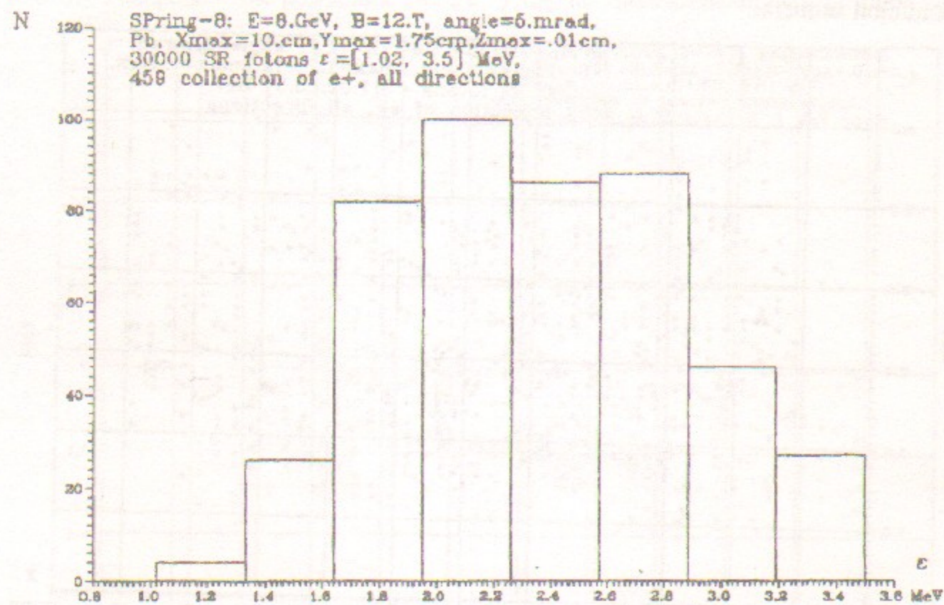
Рис. 38. Распределение эмиссии позитронов из наклонной мишени по энергии фотонов СИ.
