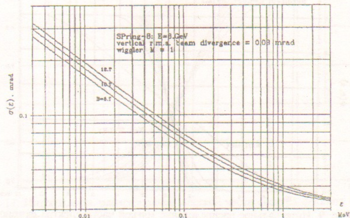
Рис. 7. Среднеквадратичный угол мощности СИ от энергии фотонов.
