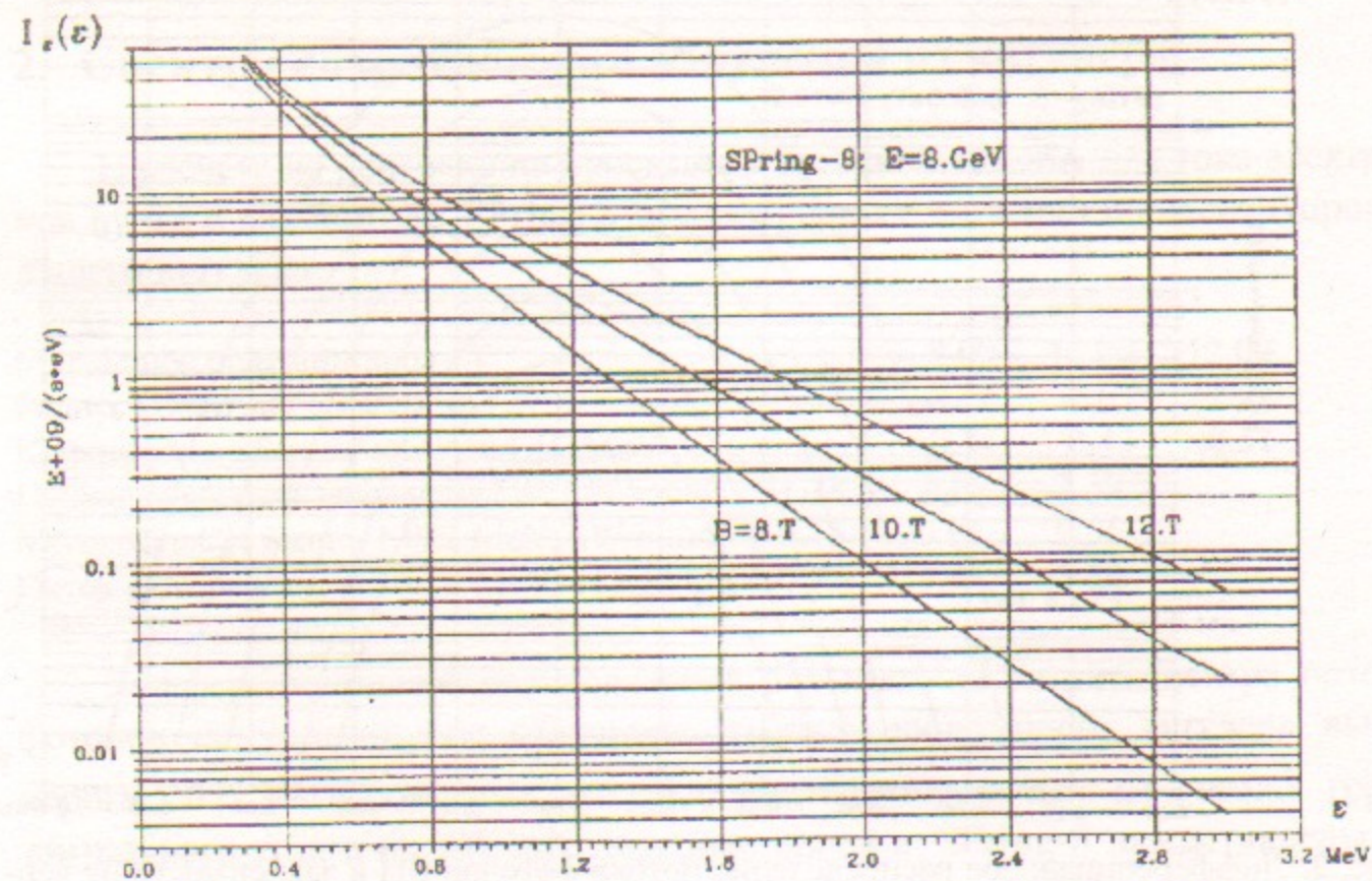
Рис. 4. Дифференциальное распределение потока фотонов СИ от их энергии, просуммированное по всем вертикальным углам.
