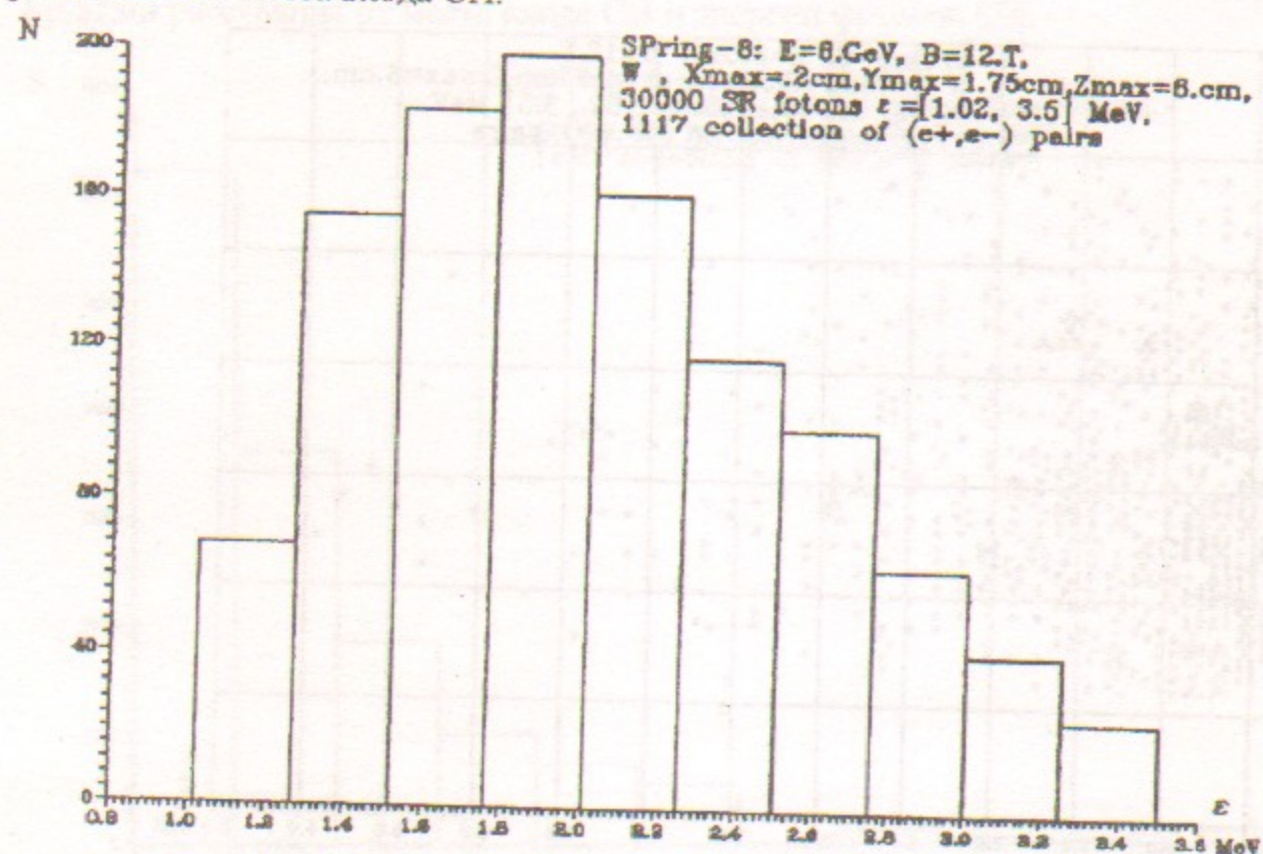
Рис. 23. Распределение рождения (e^+, e^-) пар в вольфрамовой мишени в функции энергии фотонов СИ.
