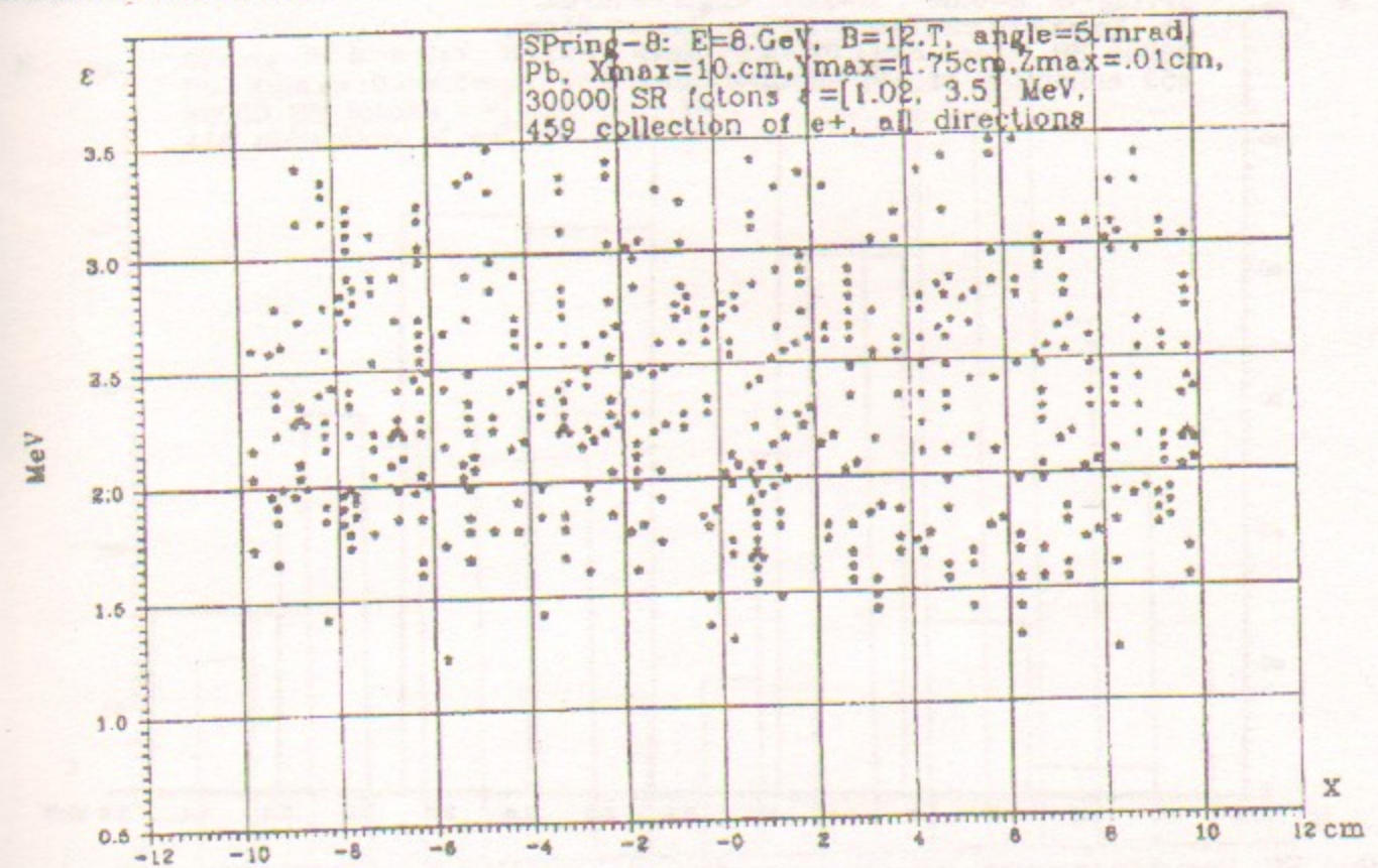
Рис. 36. Распределение эмиссии позитронов из наклонной мишени по координате вдоль поверхности наклонной мишени и по энергии фотонов СИ.
