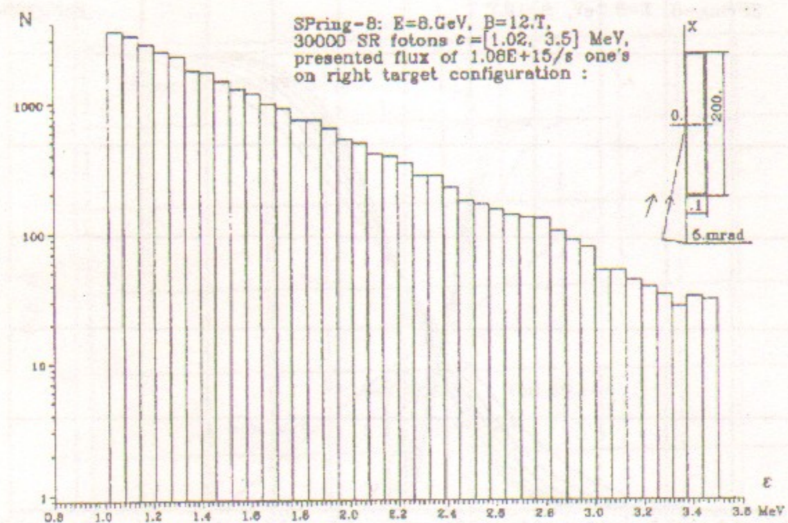
Рис. 13. Распределение фотонов СИ по их энергии для случая падения на наклонную тонкую мишень.
