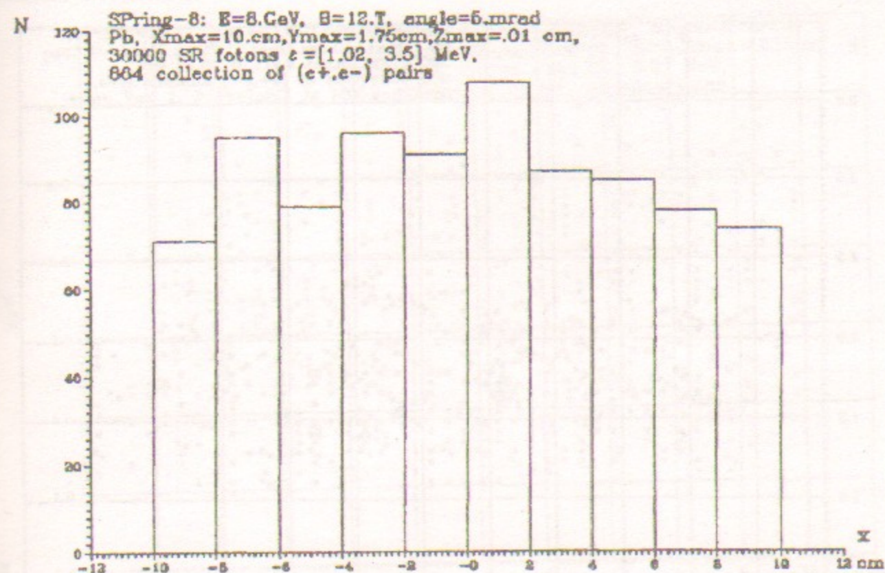
Рис. 32. Распределение рождения (e^+, e^-) пар по координате вдоль поверхности наклонной мишени.
