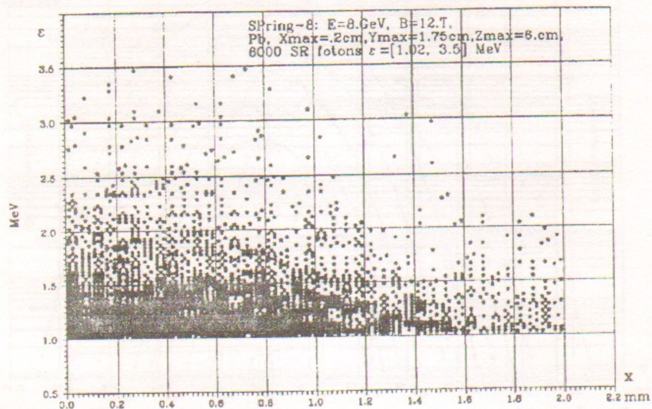
Рис. 5. Двумерное распределение жесткой части спектра фотонов СИ по высоте и энергии на расстоянии 35 м от вивглера.
