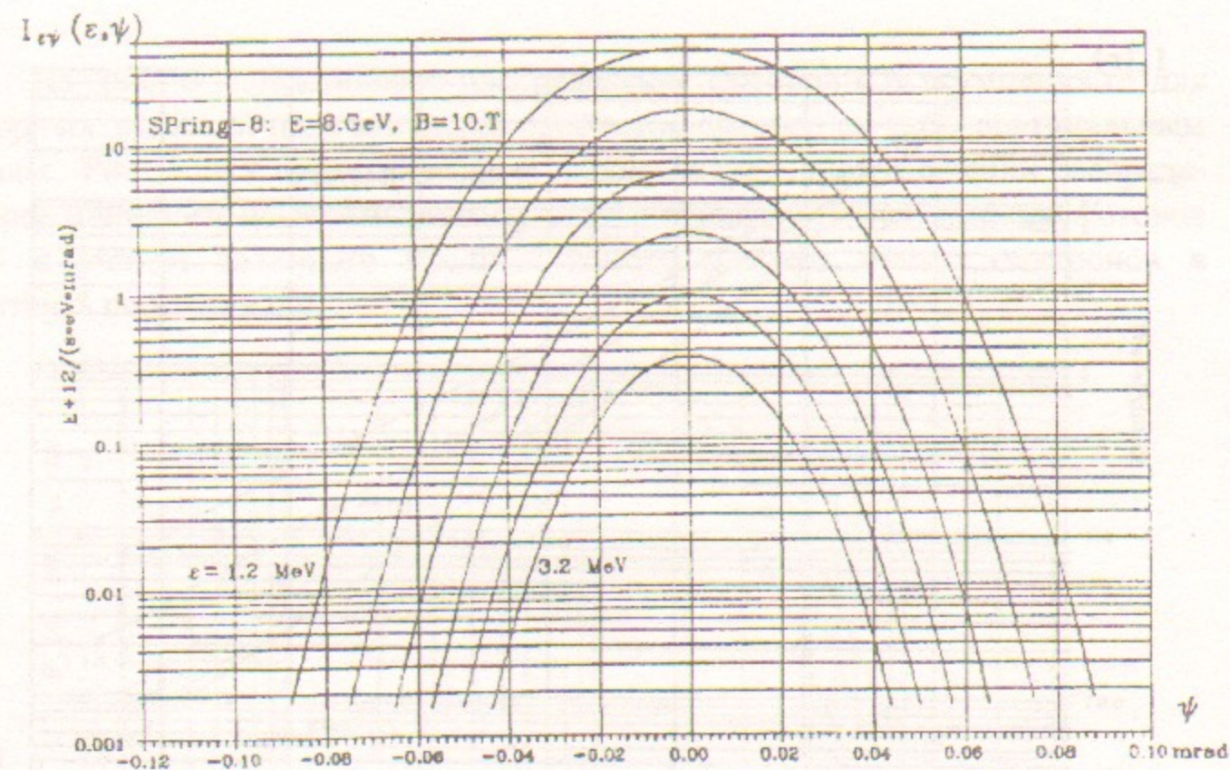
Рис. 2. Дифференциальное распределение потока фотонов СИ в зависимости от вертикального угла для поля B = 10 Т.
