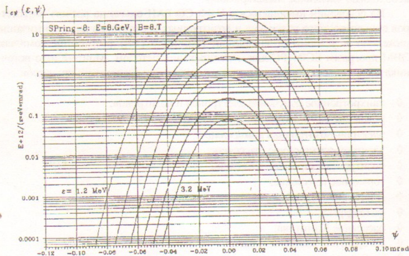
Рис. 1. Дифференциальное распределение потока фотонов СИ в зависимости от вертикального угла для поля B = 8 Т.
