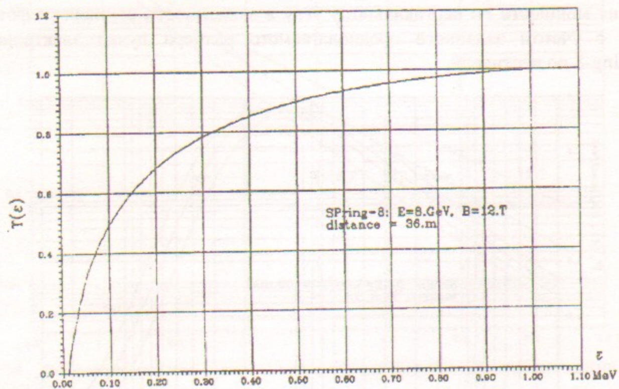
Рис. 8. Интегральное распределение мягкой части спектра фотонов СИ по энергии.
