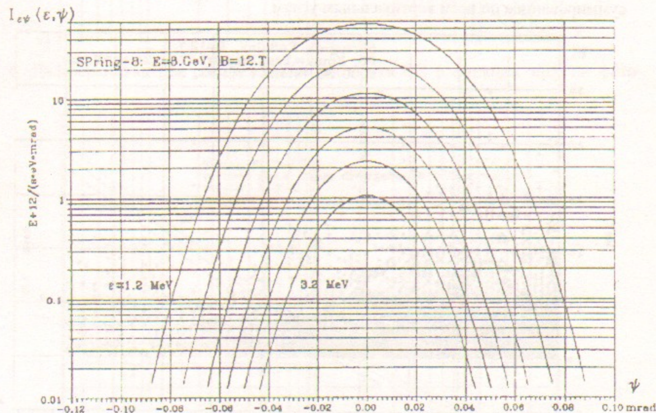
Рис. 3. Дифференциальное распределение потока фотонов СИ в зависимости от вертикального угла для поля B = 12 Т.
