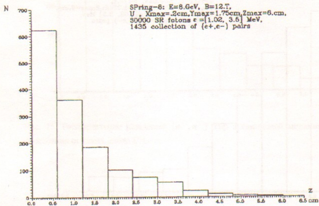
Рис. 19. Распределение рождения (e^+, e^-) пар в урановой мишени в функции расстояния от места входа СИ.
