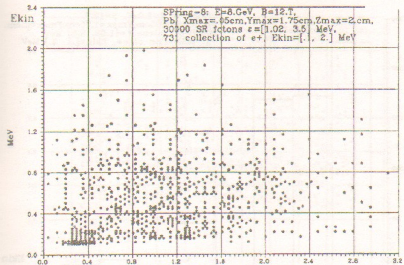
Рис. 28. Двумерное распределение позитронов по углу между направлением исходных фотонов СИ и лучем в точку остановки позитронов и по кинетической энергии позитронов в момент рождения.
