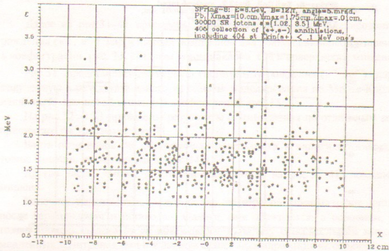
Рис. 34. Распределение аннигиляции позитронов в наклонной мишени по координате вдоль поверхности наклонной мишени и по энергии фотонов.
