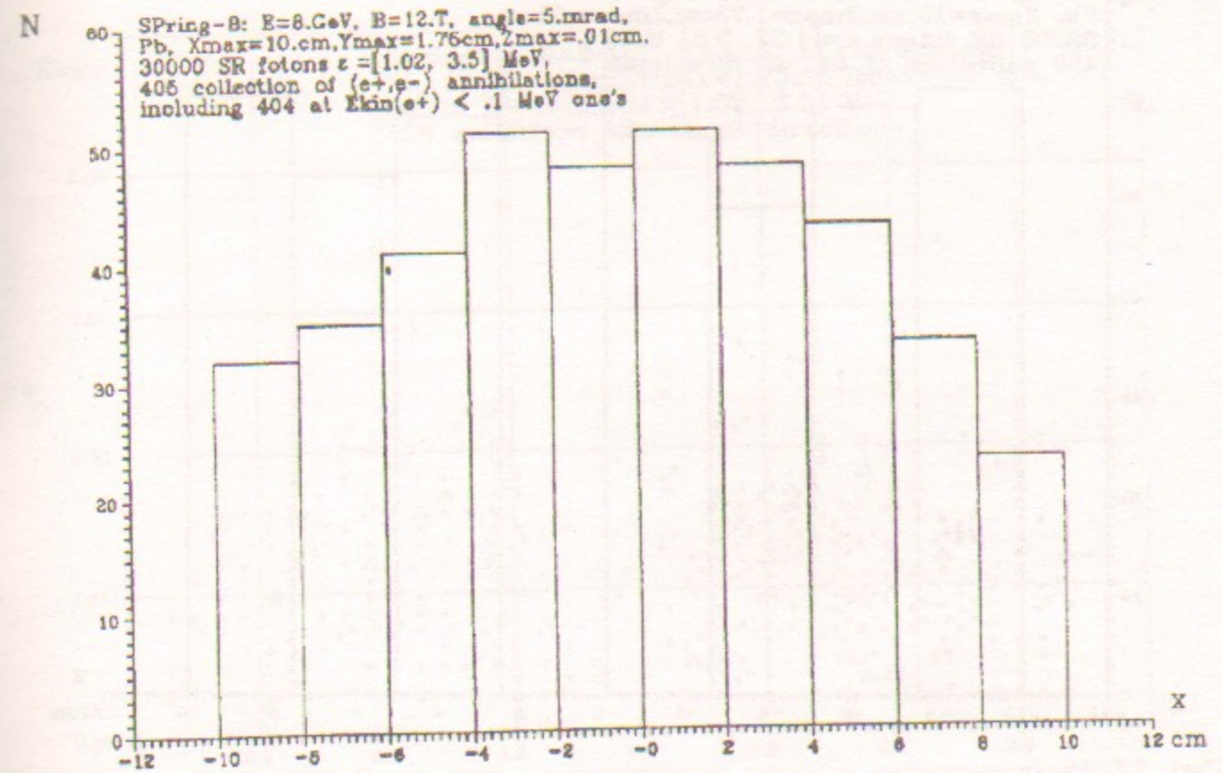
Рис. 35. Распределение аннигиляции позитронов по координате вдоль поверхности наклонной мишени.
