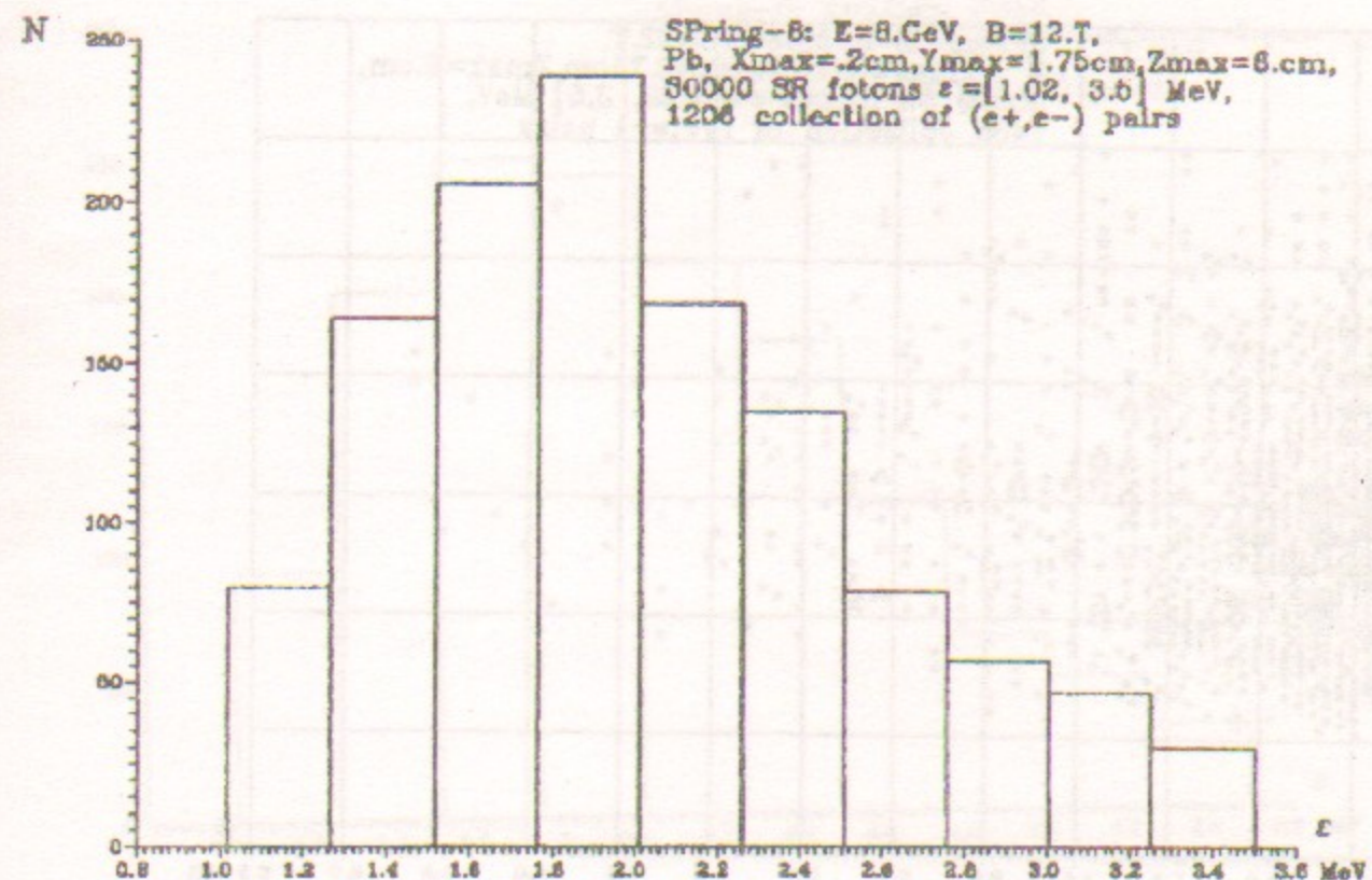
Рис. 16. Распределение рождения ( e^+ , e^- ) пар в свинцовой мишени в функции энергии фотонов СИ.
