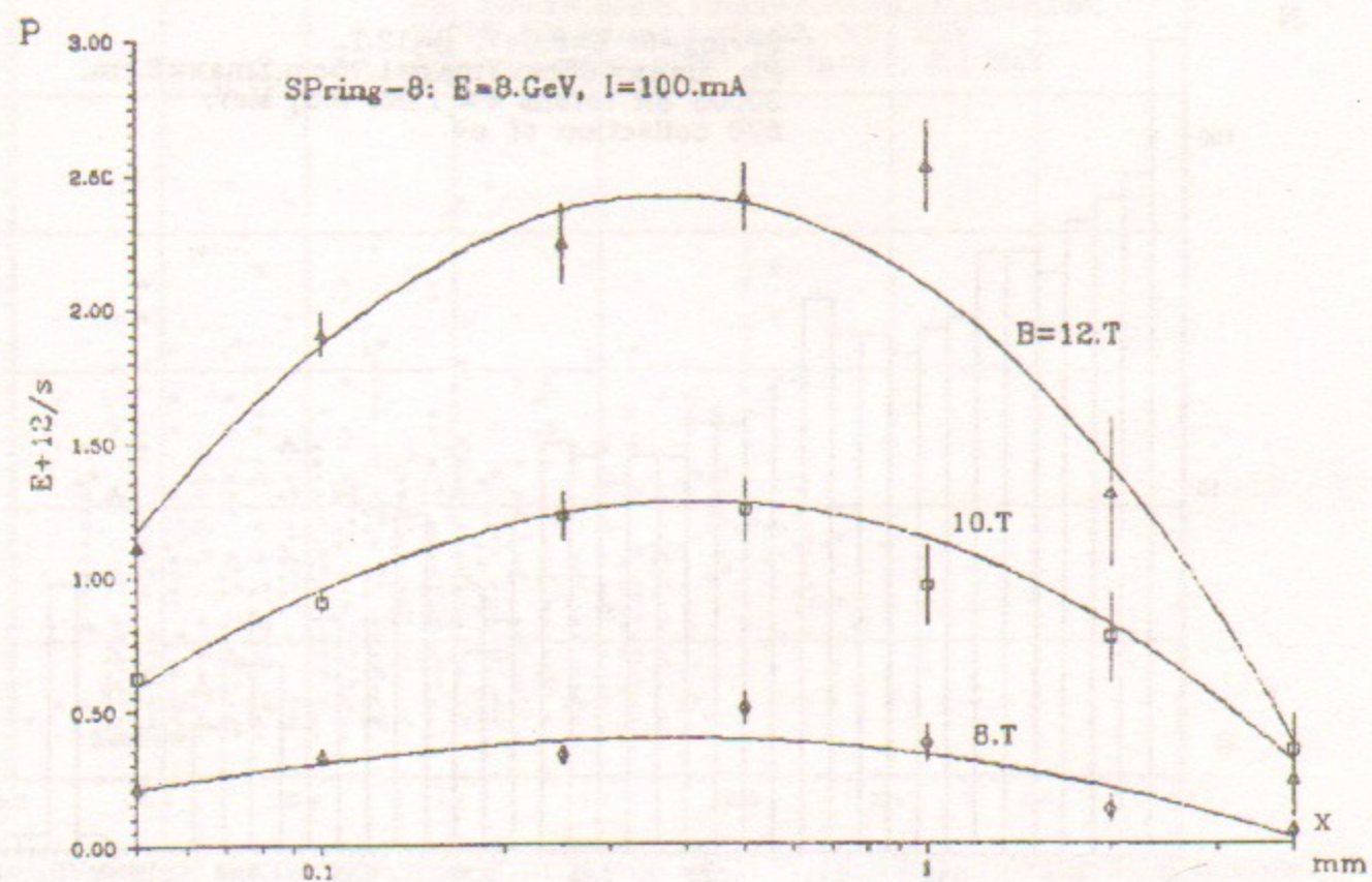
Рис. 24. Эмиссия позитронов из свинцовой мишени в прямоугольной конфигурации в функции высоты мишени для опорных значений поля витлера.
