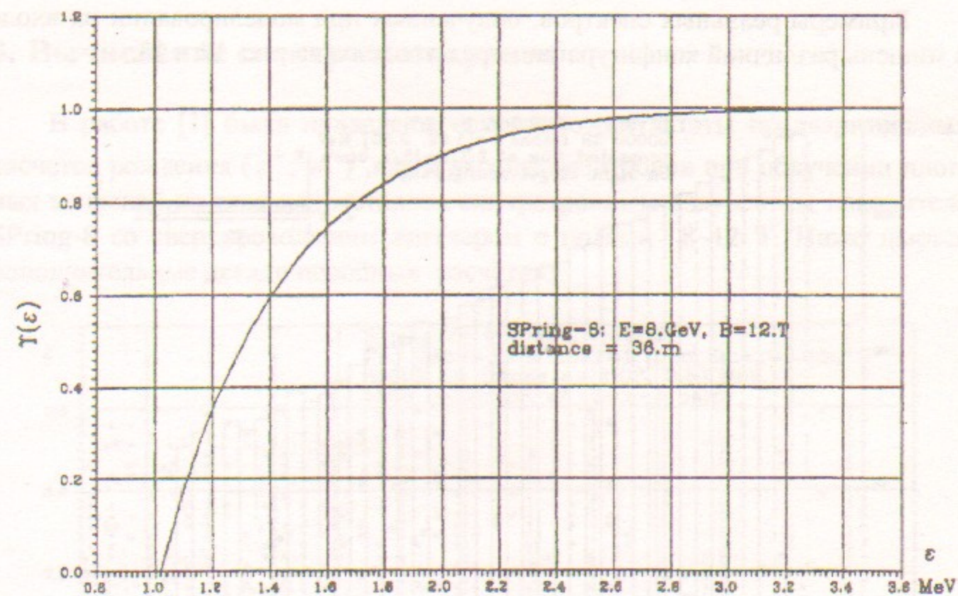
Рис. 10. Интегральное распределение жесткой части спектра фотонов СИ по энергии.
