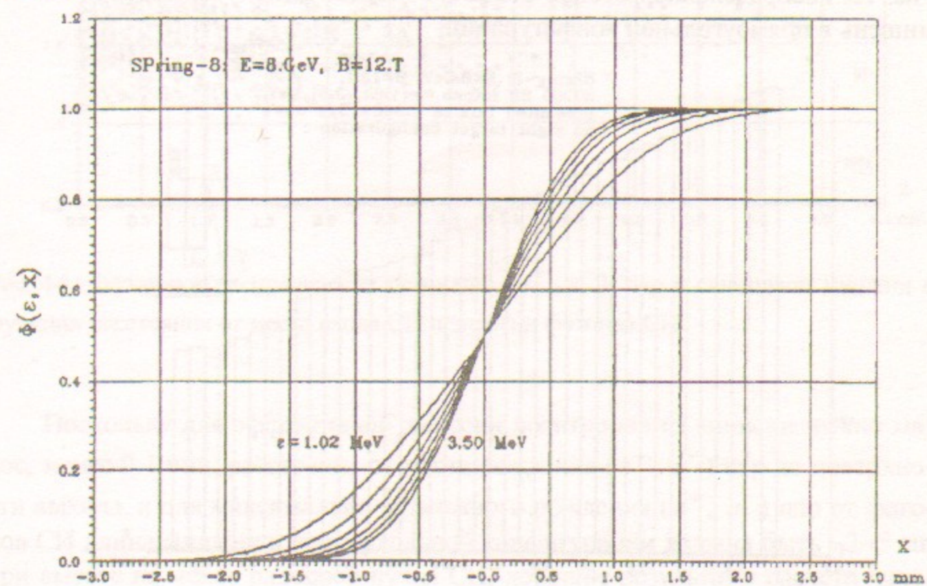
Рис. 11. Интегральное распределение жесткой части спектра фотонов СИ по вертикальной координате.
