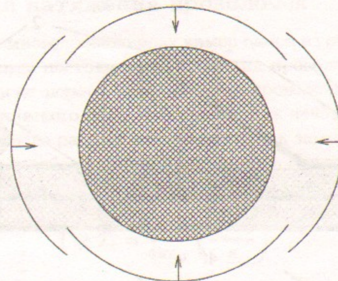
Рис. 4: Сборка цилиндрического катода из четырех листов СТЭФа. Листы, показанные на рисунке сверху и снизу, закрепляются на оправке, образуя цилиндр, поверх которого прижимаются оставшиеся два листа с нанесенным на них слоем эпоксидного клея.
