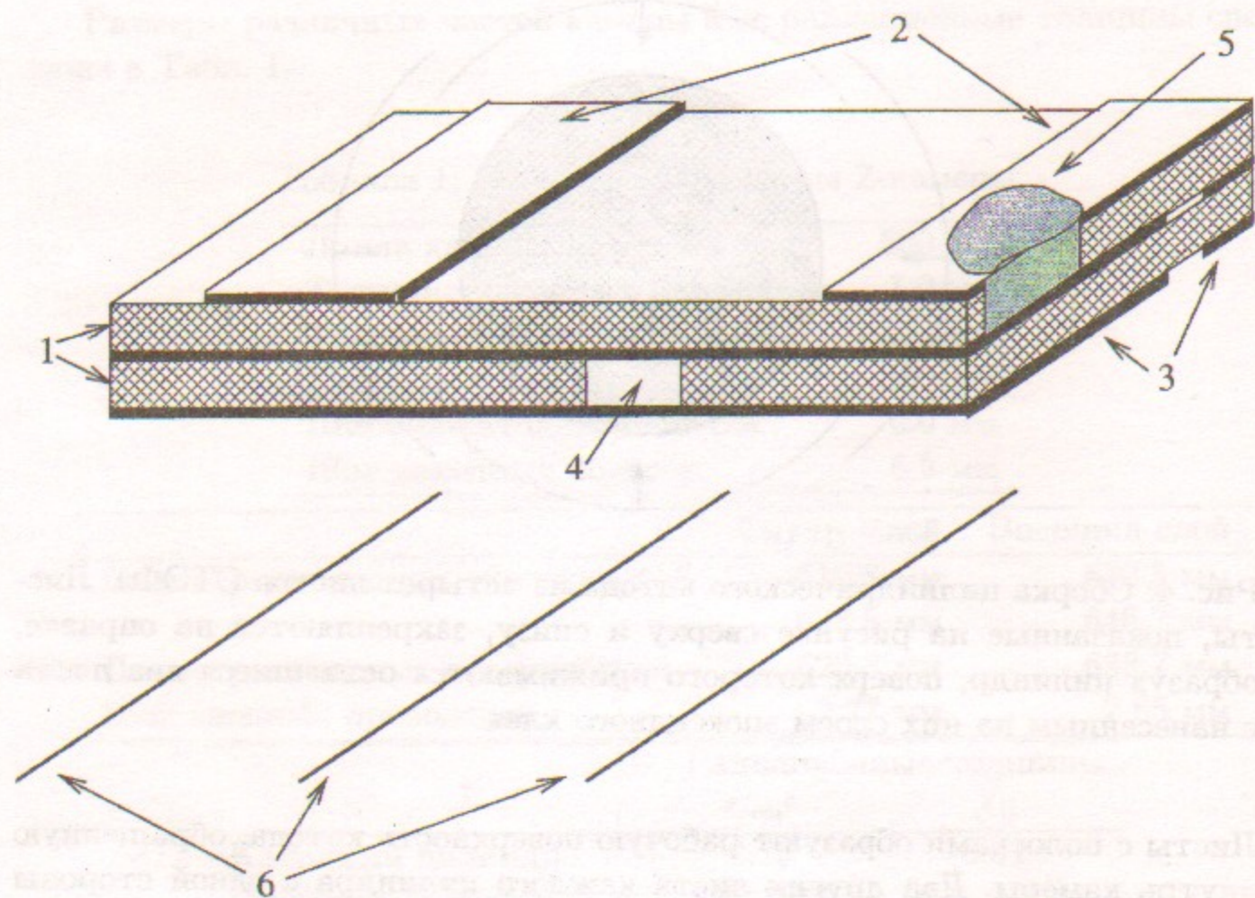
Рис. 5: Устройство катодных цилиндров. 1-листы стеклотекстолита, 2-печатный монтаж для съема сигналов, 3-катодные полосы, 4-никелевая заклепка с серебряной краской, 5-пайка.
