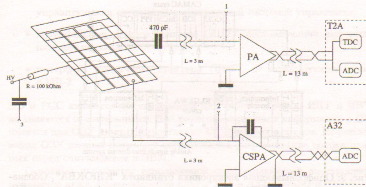
Рис. 8: Электронный тракт Z-камеры. 1 — вход калибровки электронного тракта анодных каналов, 2 — вход калибровки электронного тракта катодных каналов, 3 — вход калибровки камеры через разводку высоковольтного напряжения.
