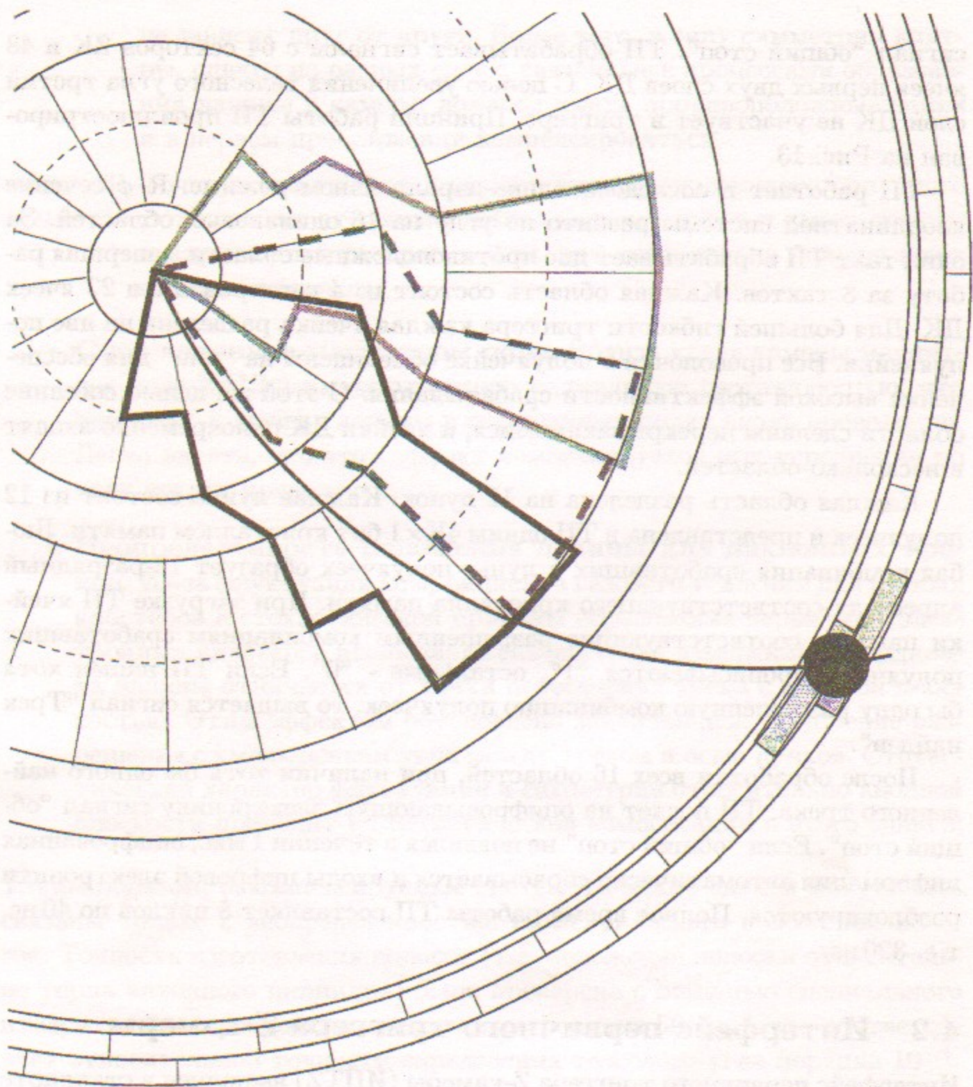
Рис. 13: Информация, используемая в работе ТП: полулунки первого и второго слоя ДК и анодные сектора Z-камеры. Показаны контуры "лунок" из 12 полулунки каждая, для опорной точки, являющейся пересечением секторов Z-камеры и изображенной на рисунке кружком.
