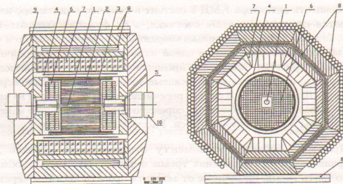
Рис. 1: Продольный и поперечный разрезы детектора КМД-2. 1 — вакуумная камера; 2 — дрейфовая камера; 3 — Z-камера; 4 — основной сверхпроводящий соленоид; 5 — компенсирующий соленоид; 6 — торцевой калориметр на основе BGO; 7 — цилиндрический калориметр на основе CsI; 8 — пробегная система; 9 — ярмо магнита; 10 — квадрупольные линзы.
