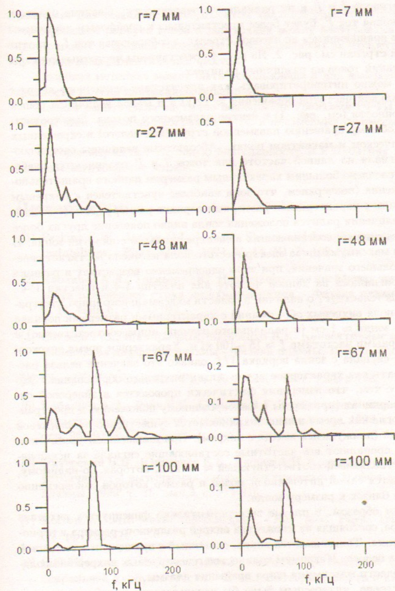
Рис. 5: Радиальные зависимости спектров токов I и I' .
