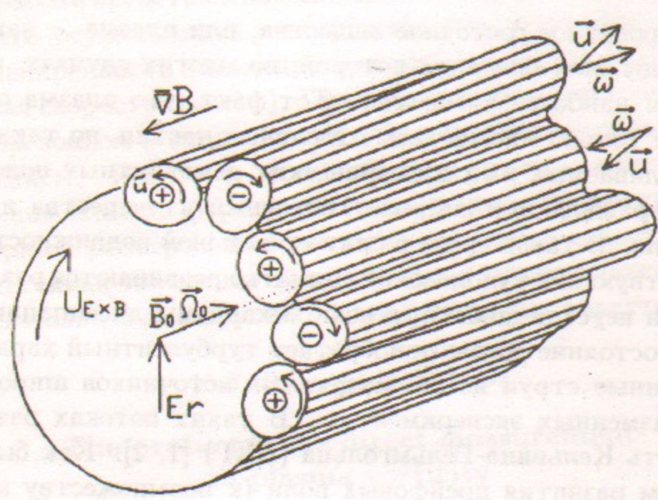
Рис. 1: Нелинейная стадия развития неустойчивости Кельвина-Гельмгольца.
