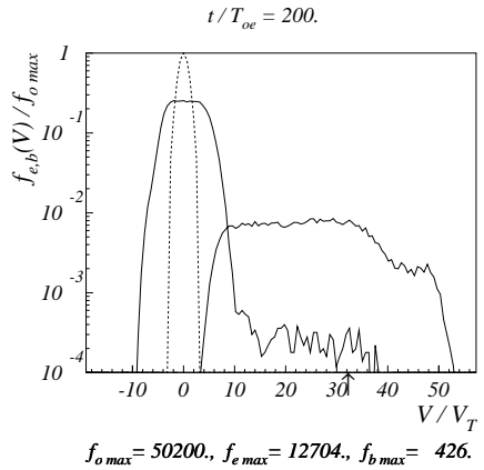
Рис. 37: Функции распределения по скоростям электронов плазмы и пучка. Пунктир – начальная функция распределения. Случай 25.
