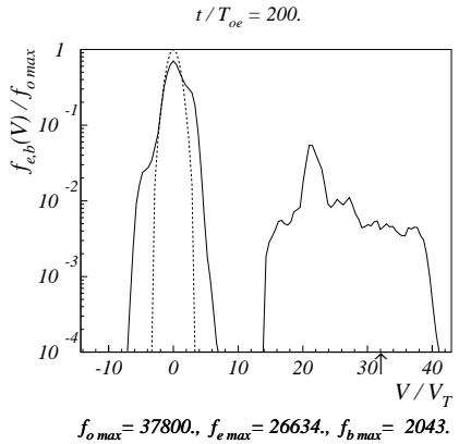
Рис. 5: Функции распределения по скоростям электронов плазмы и пучка. Пунктир – начальная функция распределения. Случай 20.
