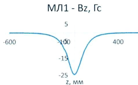
Рисунок 3.1. Геометрические параметры (а) и распределение магнитного поля МЛ1 (б). Количество витков N = 777 , ток I = 0.49 А.
