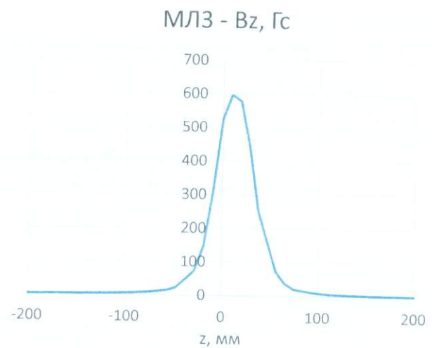
Рисунок 3.3. Геометрические параметры (а) и распределение магнитного поля МЛ3 (б). Количество витков N = 1000 , ток I = 2.5 А.
