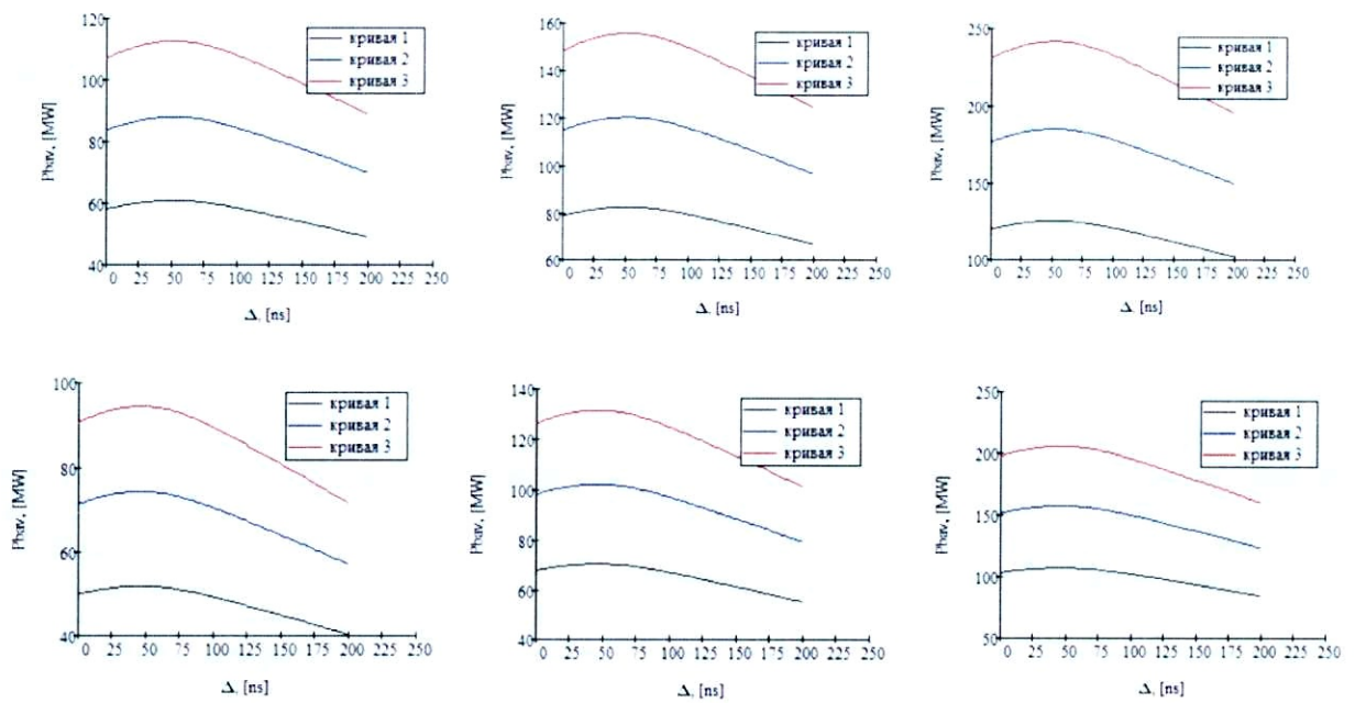
Рисунок 2.13. Средняя мощность пучка в импульсе с длительностью 100 нс в зависимости от сдвига времени инжекции по отношению к времени заполнения СВЧ ускоряющей структуры: слева направо 17 МВт, 30 МВт, 67 МВт, соответственно. Сверху вниз: для коэффициента усиления по мощности системы SLED K_p = 7.5 ; для коэффициента усиления по мощности системы SLED K_p = 5 ; для коэффициента усиления по мощности системы SLED K_p = 3 . Кривая 1 – ток пучка 1 А, 2 – 1.5 А, 3 – 2 А.
