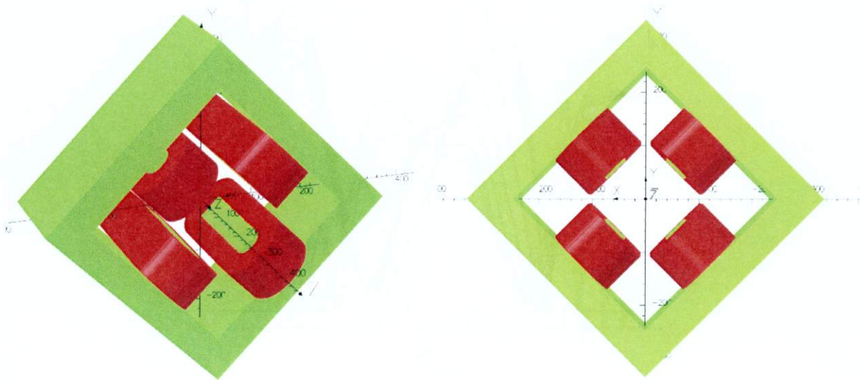
Рис. 3.10. Квадруполи типа Q2
