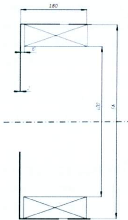
Рисунок 3.4. Геометрические параметры (а) и распределение магнитного поля КГ (б). Количество витков N = 56 , ток I = 300 А.
