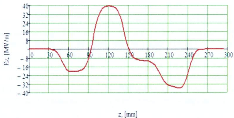
Рисунок 2.3. Расчетное распределение продольного электрического поля на оси группирователя при запасенной энергии 1 Дж.
