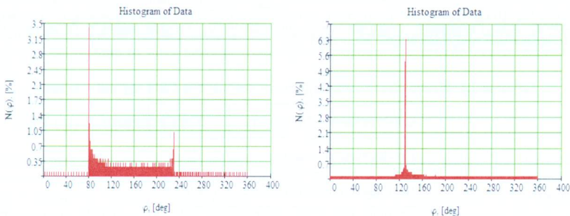
Рисунок 2.4. Распределение частиц в пучке по фазам после пролета через группирователь: слева – при входной мощности 100 кВт, справа – при входной мощности 10 кВт.
