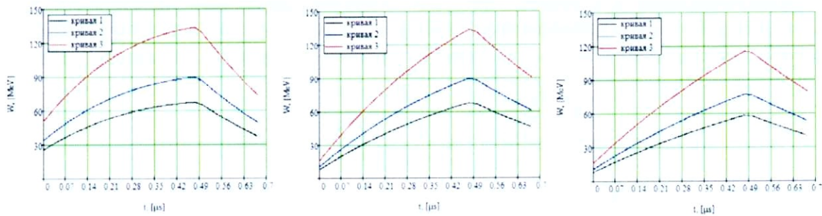
Рисунок 2.9. Набор энергии частицами пучка при пролете ускоряющей структуры с клистронами разной мощности при нулевом токе пучка в зависимости от времени инъекции. Слева направо: для коэффициент усиления по мощности системы SLED K_p = 7.5 ; для коэффициента усиления по мощности системы SLED K_p = 5 ; для коэффициента усиления по мощности системы SLED K_p = 3 . 1- мощность клистрона 17 МВт, 2 – 30 МВт, 3 – 67 МВт.
