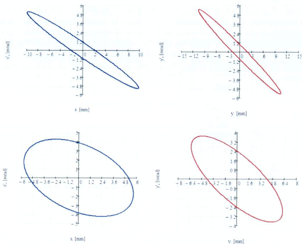
Рисунок 3.16. Начальные фазовые эллипсы для согласования каналов: сверху - для k = 1.2 , внизу - для k = 2.6 .
