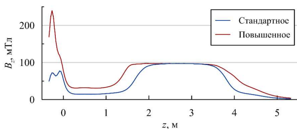
Рисунок 2. Конфигурация магнитного поля в экспериментах со стандартным (синяя кривая) и повышенным (красная кривая) ведущим магнитным полем. Амплитуда соответствует полю в транспортной секции 100 мТл.
