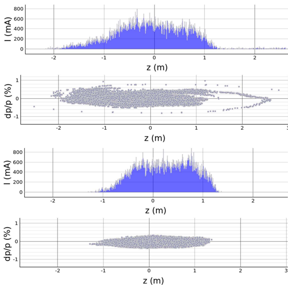
Рисунок 12. Профиль пучка на 40 000 (сверху) и 200 000 обороте (снизу).
