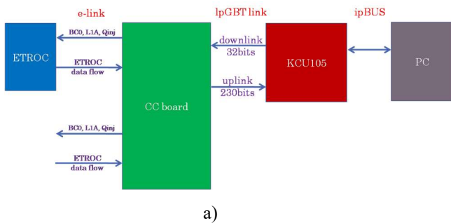
Рисунок 11. Стенд для проверки чипа ETROC: а) блок диаграмма, б) фотография стенда.
