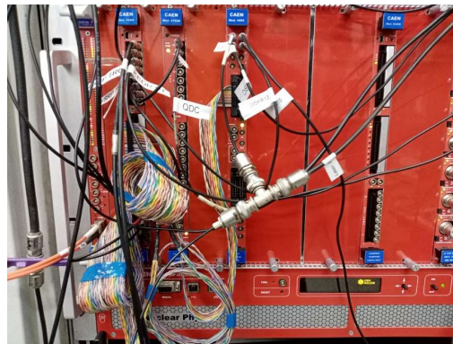
Рисунок 28. Управляющая и диагностическая электроника установки «Лазерный поляриметр»: программируемый логический блок, ЗЦП и дискриминаторы.
