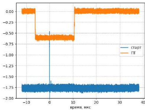
(а) Дрейфовая камера
