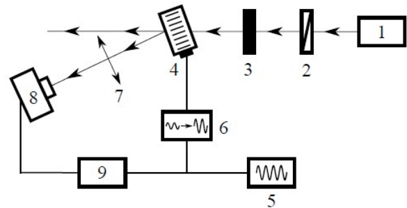
Рисунок 29. Принципиальная схема экспериментальной установки: 1 – ЛСЭ, 2 - проволочно-сеточный поляризатор, 3 - комплект калиброванных аттенуаторов излучения, 4 - АО ячейка, 5 - генератор сигналов, 6 - электрический усилитель, 7 – линза, 8 - ячейка Голя, 9 - синхронный усилитель.
