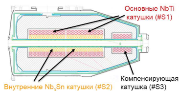
Рисунок 12. Поперечное сечение соленоида финального фокуса. Эффективная длина основной катушки равна 55,7 см.
