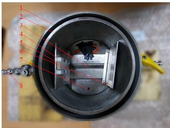
Рисунок 30. Вид АО камеры изнутри: 1 - внешняя стенка, 2 - внутренняя стенка; 3 - входное окно, 4 - держатель звукового преобразователя, 5 - преобразователь звука, 6 - звуковой отражатель, 7 - вход / выход элегаза, 8 - вход / выход охлаждающей воды.
