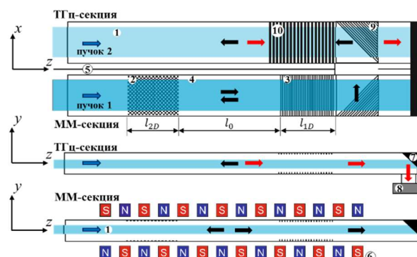
Рисунок 4. Схема электродинамической системы двухканального МСЭ с однопроходным рассеянием 4-мм волны в волну субмм диапазона. Верх рисунка – поперечные сечения ТГц-секции и ММ-секции генератора по ширине ленточного канала, ниже – сечение ТГц-секции в перпендикулярной плоскости по отношению к ширине, внизу – сечение ММ-секции также в перпендикулярной плоскости. Черные стрелки – направления движения 4-мм излучения, красные – ТГц-излучения, рассеянного на ленточном пучке. Обозначения на рисунке: 1- ленточные релятивистские электронные пучки, 2 и 3 – двумерный и одномерный брэгговские отражатели планарного резонатора ММ-секции генератора, 4 - участок гладкого волновода, 5 – проводящая стенка между ТГц-секцией и ММ-секцией, 6 – активный магнитный ондулятор, 7 – отражатель излучения для вывода его в окно 8, 9 – брэгговский планарный дефлектор, 10 – волновой трансформатор бегущей волны в квазикритическую волну.
