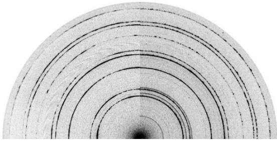
Рисунок 40. Фрагменты дифракционных картин, полученных от участка сварного соединения сплава В-1424 во время термообработки при различных температурах
