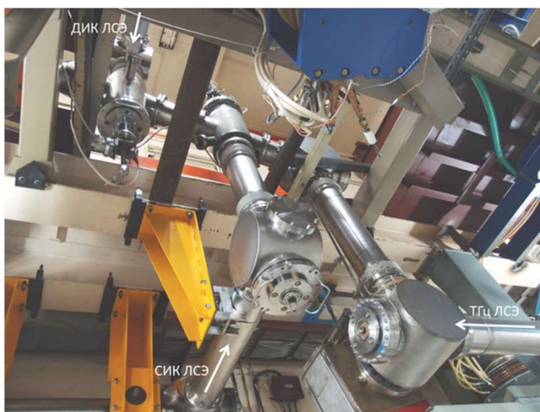
Рисунок 22. Оптический коммутатор с двумя подвижными зеркалами. Белыми стрелками показаны направления распространения внутри труб излучения первого (ТГЦ), второго (ДИК) и третьего (СИК) ЛСЭ.
