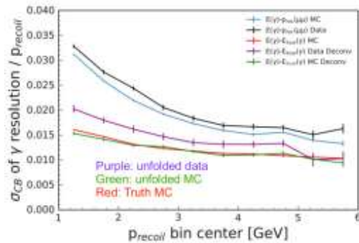
Рисунок 6. Энергетическое разрешение калориметра.
