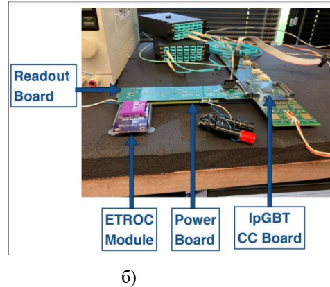
Рисунок 11. Стенд для проверки чипа ETROC: а) блок диаграмма, б) фотография стенда.
