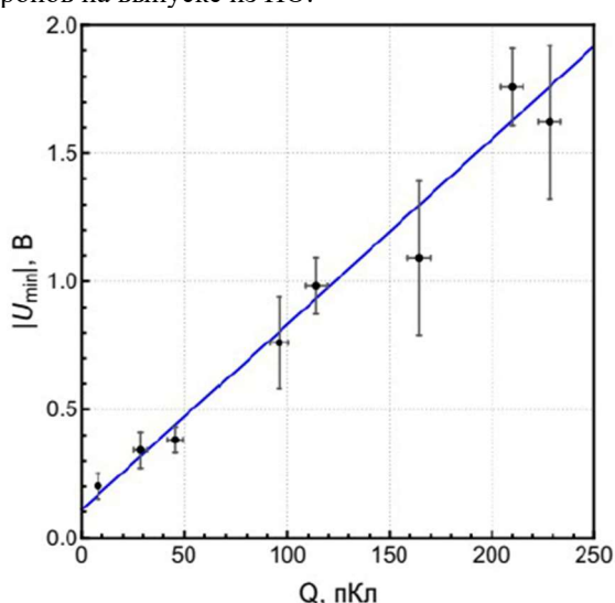
Рисунок 5. Зависимость амплитуды сигнала датчика от теряемого заряда пучка при одинаковом напряжении питания ФЭУ.
