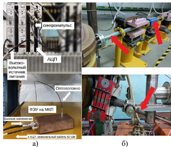
Рисунок 4. а) Элементы системы диагностики потерь в крейте КАМАК, б) Примеры расположения оптоволоконного датчика на поверхности вакуумной камеры.
