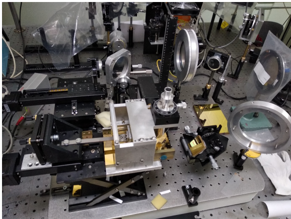
Рисунок 28. Интерферометры плазмонных и объёмных волн на экспериментальной станции «Фотоника».
