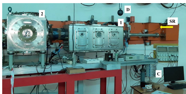
Рисунок 10. Внешний вид Технологической станции СИ. 1 – вакуумируемая камера монохроматора, 2 – вакуумируемый экспериментальный объем, С – контроллеры приводов и управляющий ПК, D – датчик АСМР.
