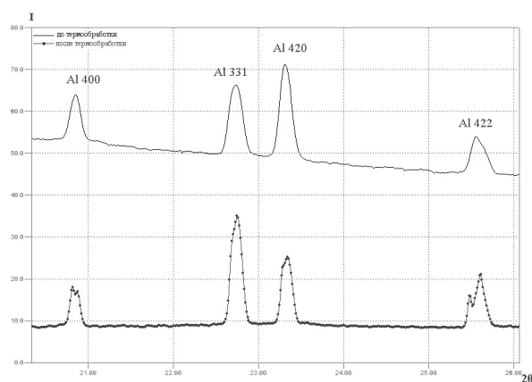
Рисунок 39. Фрагмент диффрактограммы от участка сварного соединения листов из сплава В-1424 до и после термической обработки.
