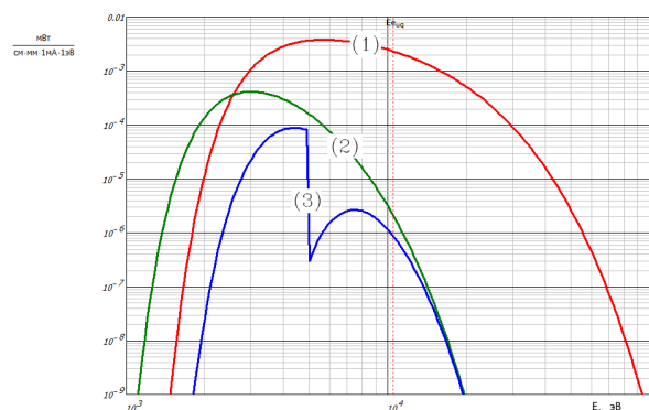
Рисунок 5. Мощность падающего на образец излучения на станции ЛИГА: 1) E=2 ГэВ, H=20 кГс, Ve окно 500 мкм; 2) актуальный режим облучения E=1,2 ГэВ, H=12 кГс, Ve окно 200 мкм; 3) E=1,2 ГэВ, H=12 кГс, Ve окно 200 мкм + Ti=20 мкм. Расстояние до образца 20130 мм.
