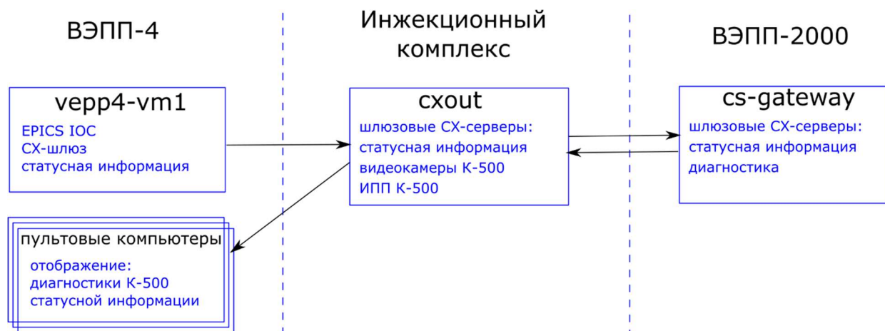
Рисунок 18. Схема передачи информации между компьютерами разных систем управления ускорительных комплексов.
