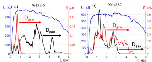
Рисунок 3. Сопоставление сигналов мощности субмм-излучения на длине волны в окрестности 1 мм с детектора в вакуумной камере D вак и с детектора потока излучения, выведенного в атмосферу D атм , для двух вариантов узла для вывода излучения в атмосферу: (а) – до модернизации узла; (б) – после его модернизации. Синей линией показано изменение во времени напряжения на диоде ускорителя.
