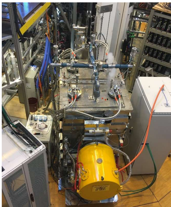
Рисунок 3. Инжектор на токамаке TCV.
