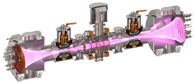
Рисунок 1. Разрез установки ALIANCE-T.
