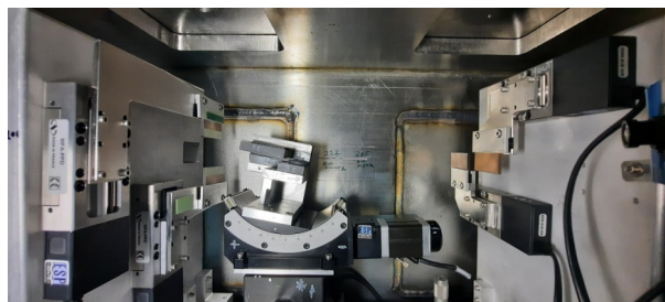
Рисунок 11. Монохроматор на Si(111) кристалле-бабочке и управляемые рентгеновские щели.
