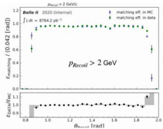
Рисунок 5. Эффективность реконструкции фотонов в зависимости от полярного угла.
