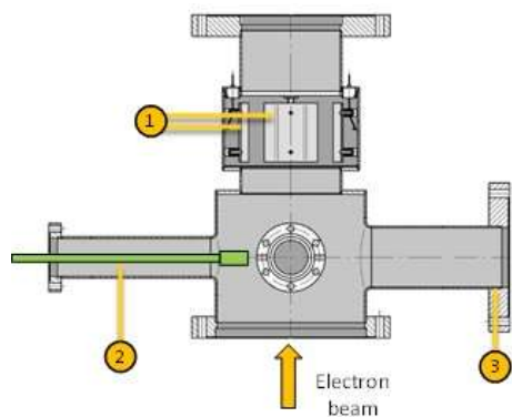
Рисунок 4. Схема диагностического узла (слева) и его фотография (справа). 1 – пикап-электроды, 2 – профилометр, 3 – вакуумное окно, 4 – манипулятор.
