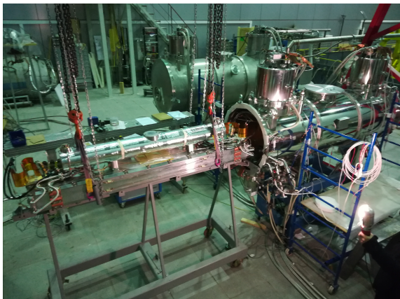
Рисунок 3. Процесс установки магнитной системы 119-периодного ондулятора с периодом 15,6 мм и полем 1,2 Тл в собственный криостат с косвенным охлаждением.
