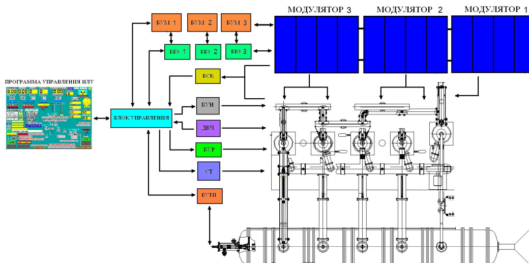
Рисунок 5. Блок-схема системы управления ускорителем ИЛУ-14.
