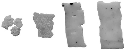
Рисунок 1. Фотографии образцов, подвергнутых воздействию потоков электронов различной плотностью мощности W .
