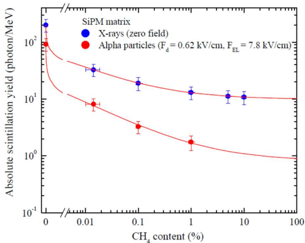
Рисунок 1. Абсолютный выход первичных сцинтилляций от рентгеновских фотонов и альфа частиц в чистом жидком Ar и его смесях с CH 4 в зависимости от содержания CH 4 , регистрируемый матрицей SiPM.
