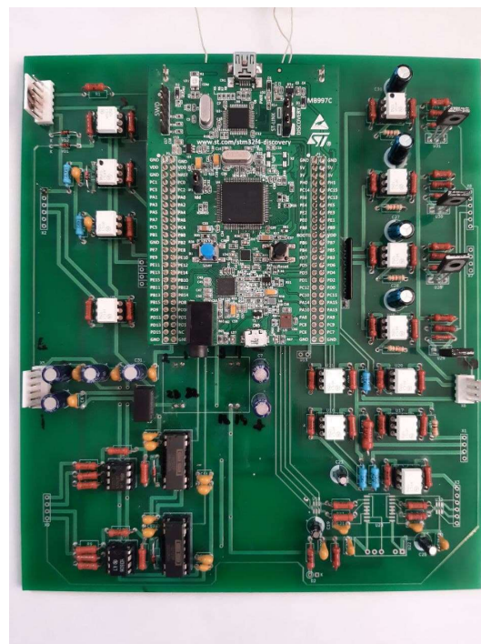
Рисунок 6. Новый БУМ – плата управления.
