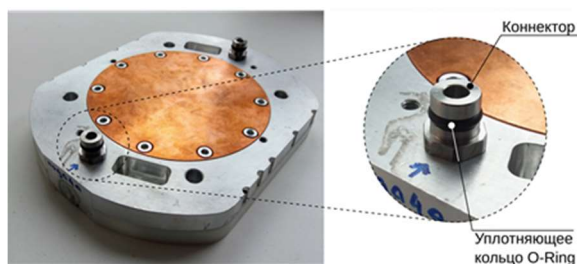
Рисунок 21. Общий вид медной подложки, установленной в основание мишенного узла.
