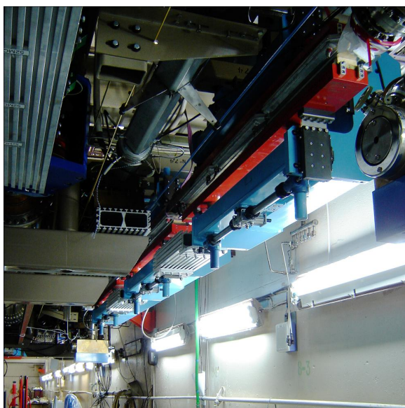
Рисунок 5. Ondулятор третьего ЛСЭ.
