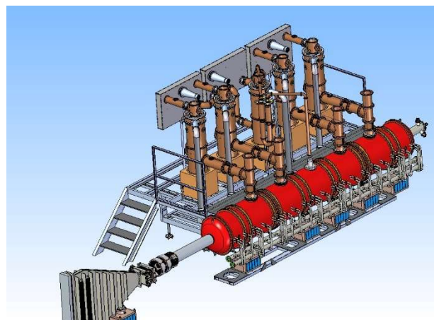
Рисунок 4. Виды ускорителя ИЛУ-14 с модернизированным ВЧ генератором.
