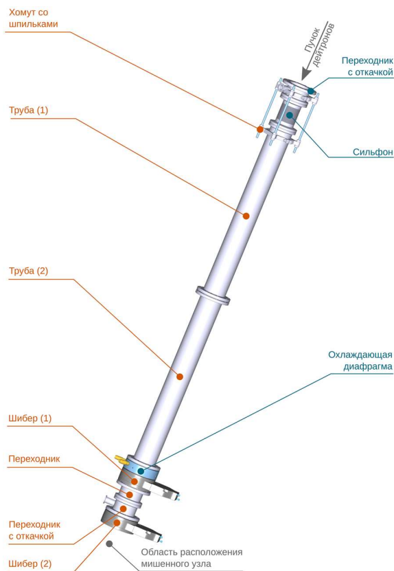
Рисунок 17. Вакуумная камера с обозначением ключевых элементов.
