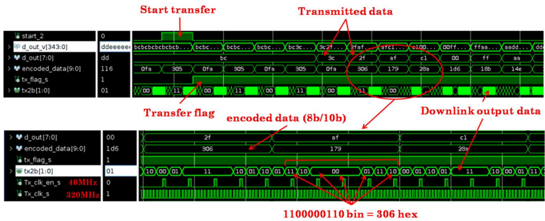
Рисунок 9. Моделирование работы модуля конфигурации (Tx Config module).
