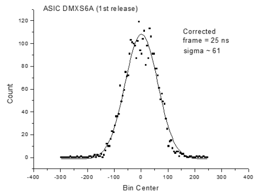
Рисунок 19. Распределение шумового сигнала для электроники регистрации на основе СБИС DMXS6A и DMXS6B.
