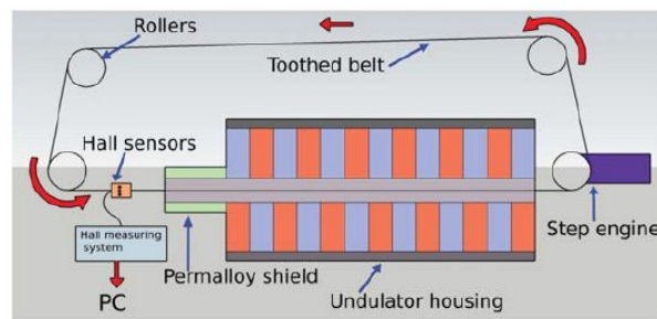
Рисунок 11. Схема устройства для измерения поля ондулятора.
