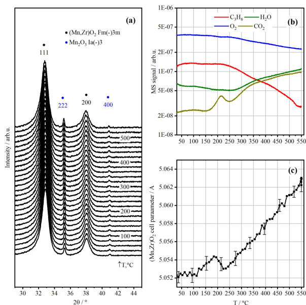
Рисунок 47. Рентгенограммы Mn-Zr-650 , записанные при нагреве в реакционной среде 1% C_3H_8 /6% O_2 /He от 30 до 550°C со скоростью 5°/мин, длина волны 1.6467 Å (а) и данные масс-спектрометрии полученные параллельно (б). Изменение параметра решетки (Mn,Zr) O_2 при изменении температуры (с).
