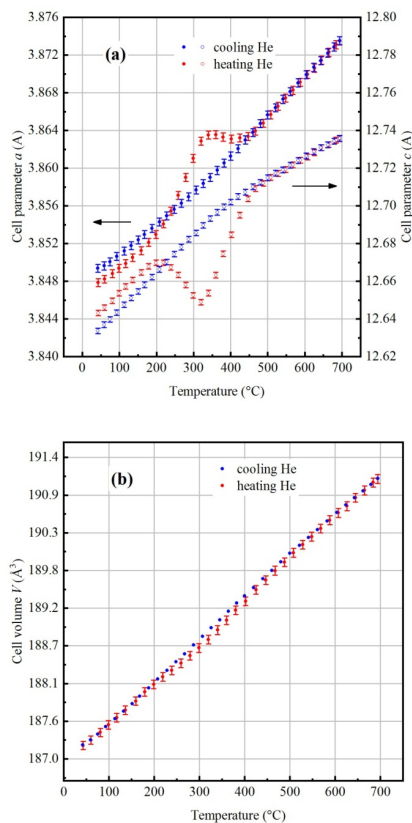
Рисунок 52. Зависимости параметров решетки a , c (а) и объема элементарной ячейки (б) от температуры, полученные для LCNO_01 при нагреве/охлаждении в He.
