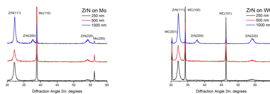
Рисунок 43. Изменение фазового состава покрытий ZrN с ростом толщины покрытия на поверхностях молибдена и карбида вольфрама.
