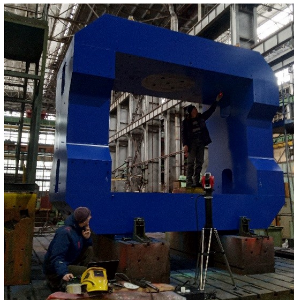
Рисунок 4. Процесс предварительной сборки железного ярма дипольного магнита СВМ, декабрь 2021.
