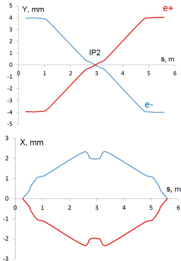
Рисунок 22. Электростатическое разведение орбит на участке вставки. Исходное разведение происходит по вертикали с амплитудой 4 мм.
