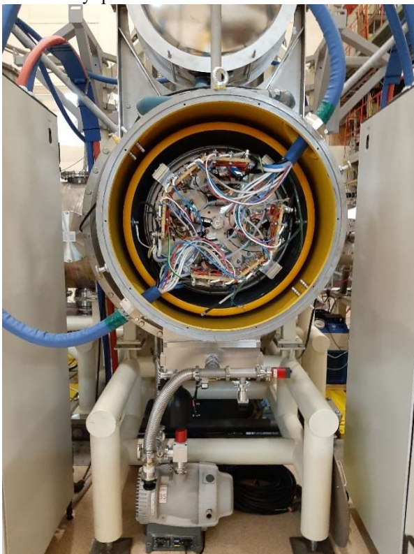
Рисунок 7. Инжектор атомарных пучков.
