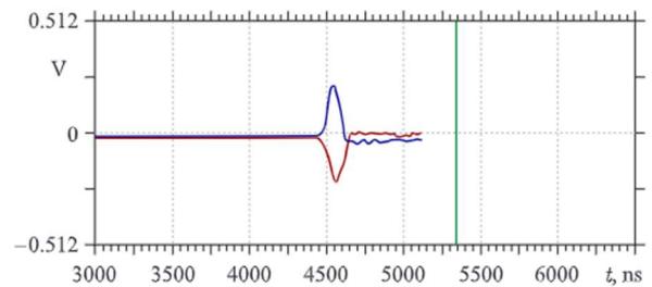
Рисунок 16. Импульсы генераторов инфлекторов.
