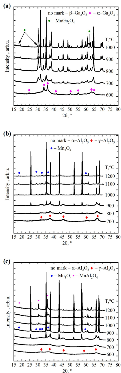
Рисунок 50. Рентгенограммы серий катализаторов 10Mn90Al(а), 10Mn90Ga(б) и 10Mn85Al5Ga(в), прокаленных в температурном диапазоне 600-1200°C.
