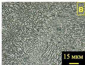
Рисунок 34. Макроструктура (а) и микроструктура (б) сварного соединения (оптическая металлография)
