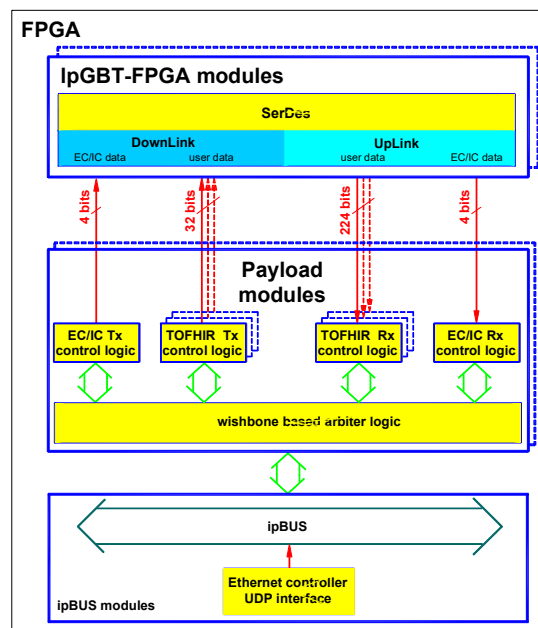
Рисунок 4. Блок-схема проекта для ПЛИС KCU105.
