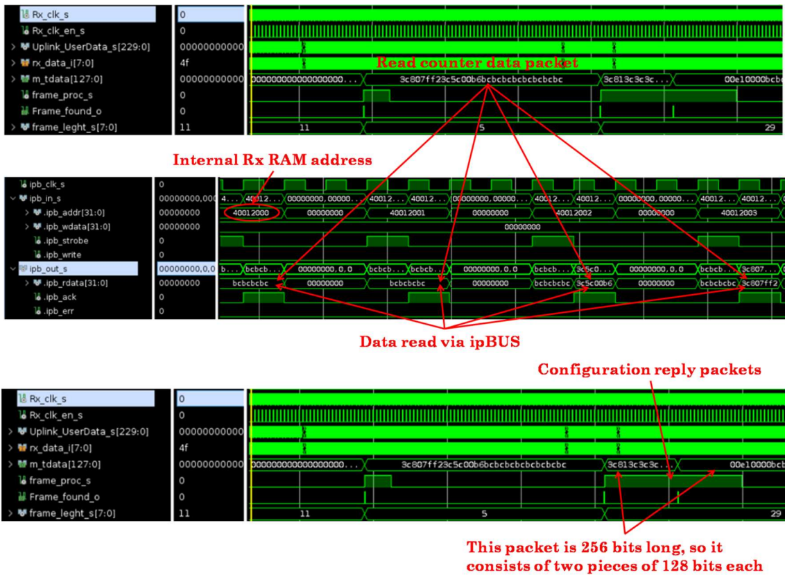
Рисунок 10. Моделирование работы модуля приема данных (Rx module).
