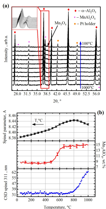
Рисунок 51. Рентгенограммы катализатора 10Mn5Ga85Al-1000 , снятые в условиях его постепенного охлаждения на воздухе от 1000 °C до 100 °C со скоростью 10 °/мин – (а); изменение параметра решётки, содержания (вес.%) и средних размеров ОКР для оксида со структурой шпинели при охлаждении – (б).
