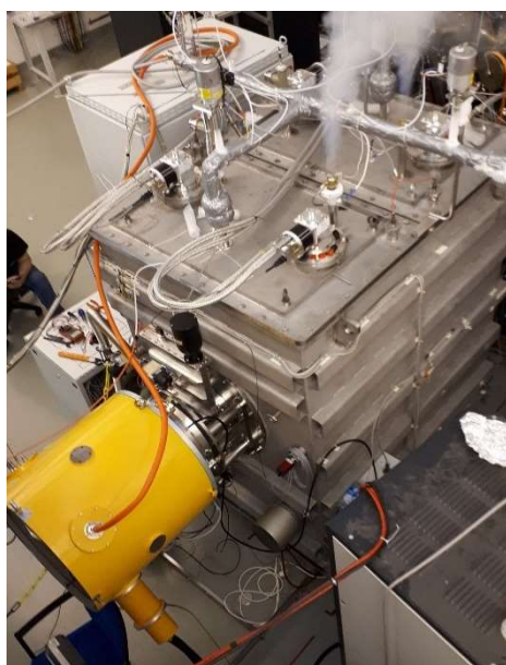
Рисунок 1. Инжектор на токамаке в Праге.
