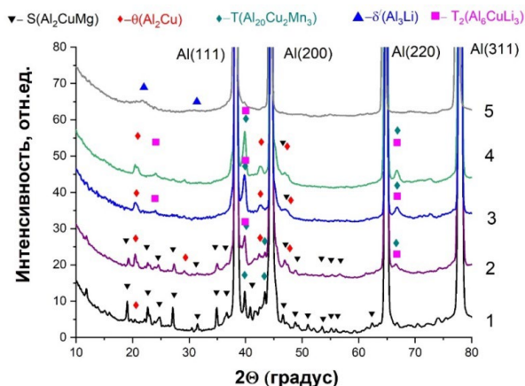
Рисунок 35. Рентгенограммы (на просвет) образца со сварным соединением: 1 – сплав Д16Т, 2 – зона плавления сплава Д16Т, 3 – центр сварного шва, 4 – зона сплавления около сплава 1420, 5 – сплав 1420.
