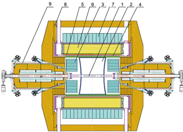
Рисунок 1. Криогенный магнитный детектор КМД-3: 1 – вакуумная камера; 2 – дрейфовая камера; 3 – калориметр ВГО; 4 – Z-камера; 5 – сверхпроводящий соленоид; 6 – жидкоксеноновый калориметр; 7 – калориметр CsI; 8 – ядро магнита; 9 – соленоиды ВЭПП-2000.
