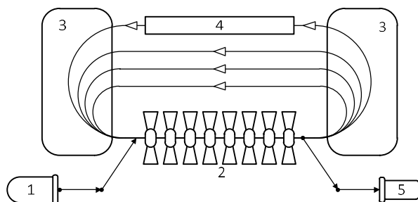
Рисунок 1. Упрощённая схема многооборотного УР: 1 – инжектор, 2 – ускоряющая структура, 3 – поворотные магниты, 4 – ондулятор, 5 – поглотитель.
