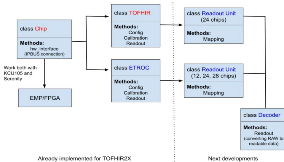
Рисунок 14. Блок-схема программного обеспечения DAQMTD.
