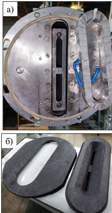
Рисунок 6. Фотография элементов ускорительного магнитно-изолированного диода, предназначенного для одновременной генерации двух ленточных пучков. (а) – место присоединения к ускорительному диоду вакуумного канала с миллиметровой и терагерцовой секциями, расположенными одна над другой по вертикали. (б) - графитовые детали анодной щели для двухпучкового диода.
