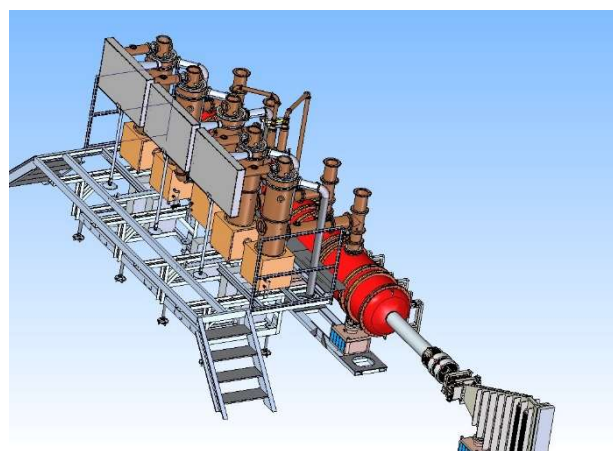
Рисунок 3. Ускоряющая структура ИЛУ-14 на несущей раме: 1 – ускоряющая структура, 2 – несущая рама, 3 – трубы и коллекторы системы водяного охлаждения, 4 – магниторазрядные высоковакуумные насосы.
