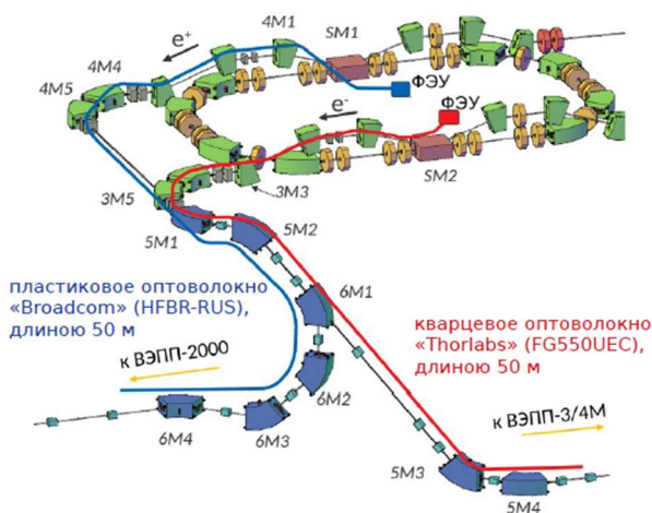
Рисунок 3. Схема расположения датчиков потерь пучка в каналах транспортировки К-500.
