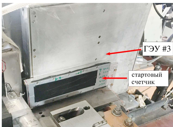
Рисунок 3. Стартовый сцинтилляционный счетчик.
