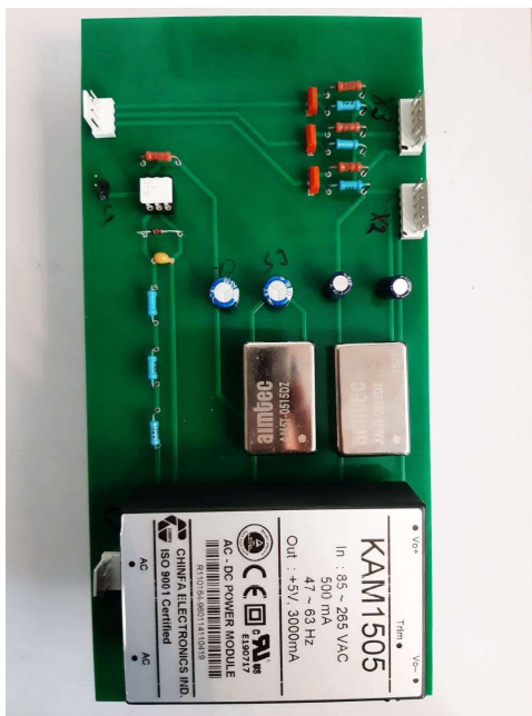
Рисунок 7. Новый БУМ – плата питания.
