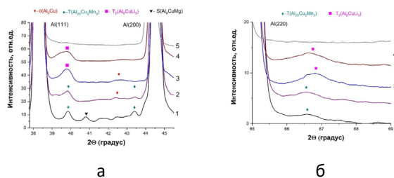
Рисунок 36. Рентгенограммы (на просвет) образца со сварным соединением: а) область углов 39\text{--}43^\circ ; б) область углов 66\text{--}68^\circ , 1 – сплав Д16Т, 2 – зона плавления сплава Д16Т, 3 – центр сварного шва, 4 – зона сплавления около сплава 1420; 5 – сплав 1420
