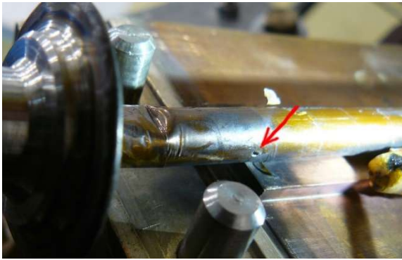
Рисунок 1. Отверстие в тонкостенной вакуумной камере импульсного магнита.
