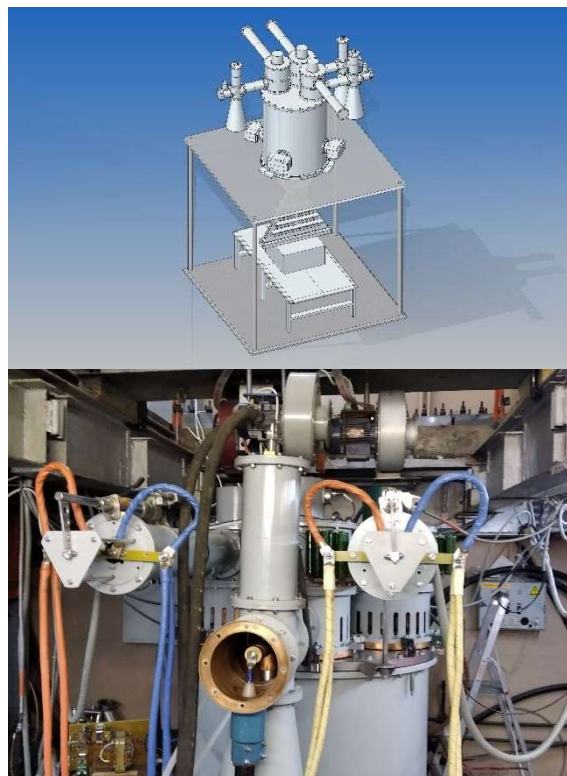
Рисунок 1. Концептуальный проект ИЛУ-10М2 и его верхняя часть с тремя ВЧ генераторами.
