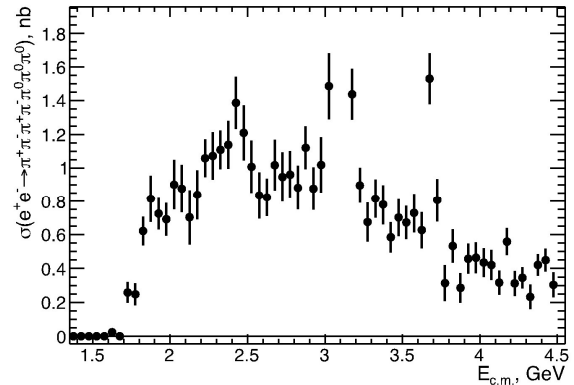
Рисунок 3. Измеренные в эксперименте ВАВАР сечения процессов e^+e^- \rightarrow \pi^+\pi^-\pi^0\pi^0\pi^0 (вверху) и e^+e^- \rightarrow 2(\pi^+\pi^-\pi^0\pi^0\eta) (внизу).
