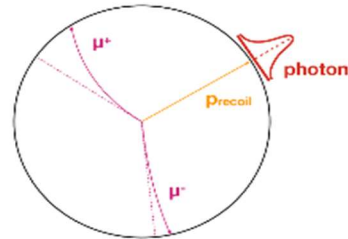
Рисунок 4. Кинематика процесса e^+e^- \rightarrow \mu^+\mu^-\gamma .
