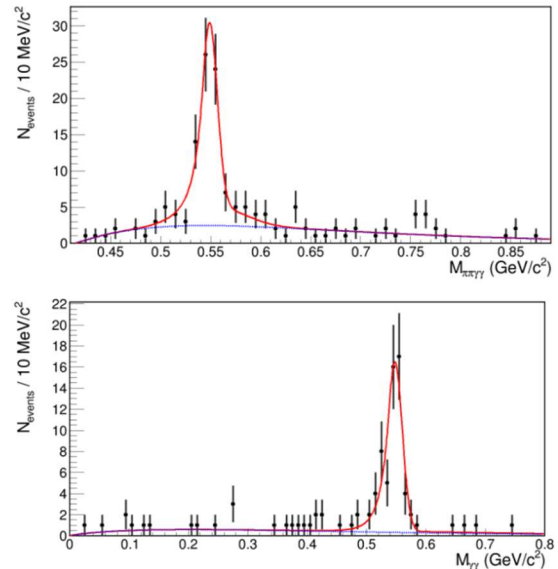
Рисунок 1. Распределение по инвариантной массе восстановленного \eta -мезона в процессе Y(5S) \rightarrow Y(2S)\eta . Сверху – сигнал в канале распада \eta \rightarrow \pi^+\pi^-\pi^0 , снизу – в канале \eta \rightarrow \gamma\gamma . Точками показаны распределения экспериментальных данных со статистическими неопределенностями, линиями – результаты аппроксимации вклада сигнальных и фоновых событий.
