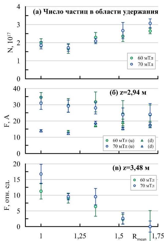
Рисунок 4. Зависимость числа частиц и интегрального потока от средней глубины гофрировки при различных ведущих магнитных полях. (а) число частиц в области удержания, (б) интегральный поток в середине транспортной секции на сторонах зона Маха, обращённых к источнику (u) и приёмнику (d) плазмы, (в) интегральный поток на выходе из транспортной секции.
