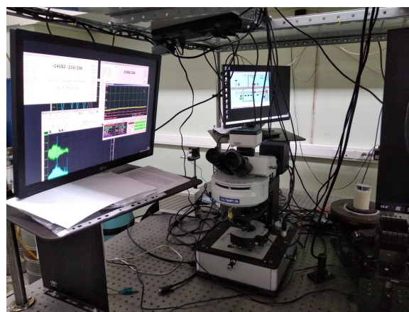
Рисунок 27. Атомно-силовой микроскоп на экспериментальной станции «Фотоника».
