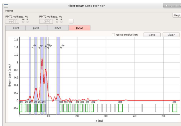
Рисунок 7. Окно вывода данных датчика потерь пучка для позитронов направлении ВЭПП-2000, показано распределение потерь до наладки выпуска.
