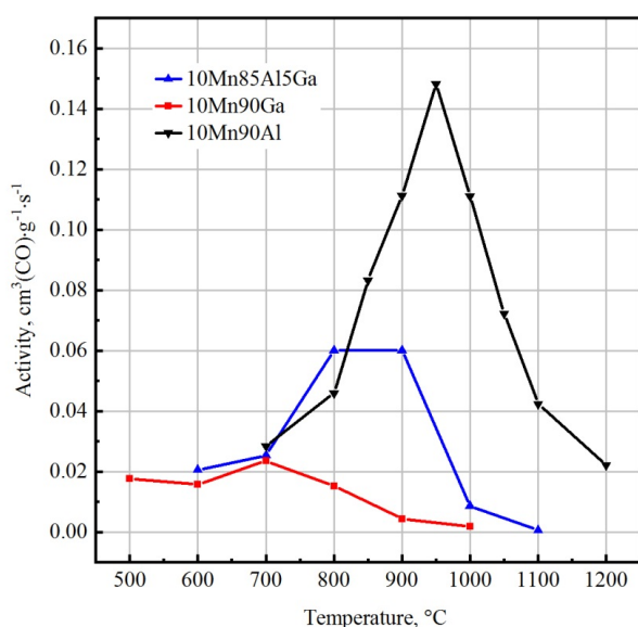
Рисунок 49. Зависимость каталитической активности в реакции окисления CO двухкомпонентных систем состава 10Mn90Ga и 10Mn90Al и трехкомпонентной системы состава 10Mn85Al5Ga от температуры прокаливания образцов в реакции окисления CO.
